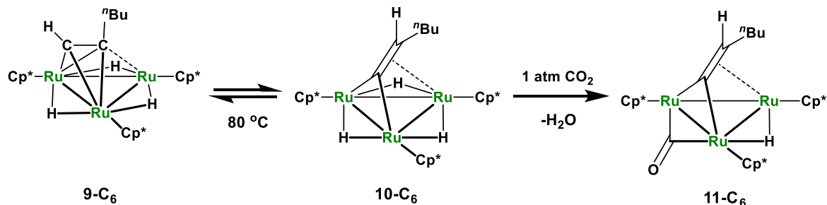
Scheme 3-1-6. 錯体 9 , 10 の平衡混合物と二酸化炭素との反応
