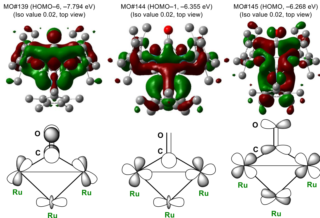
Figure 2-3-8. 錯体 2'-symm の特徴的な分子軌道
