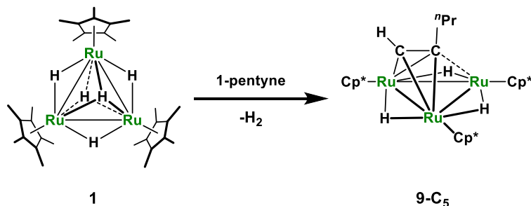
Scheme 3-1-3. 錯体 1 と 1-ペンチンとの反応
