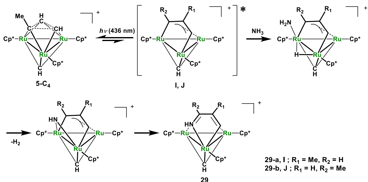
Scheme 4-2-3. 錯体 29 の生成機構
