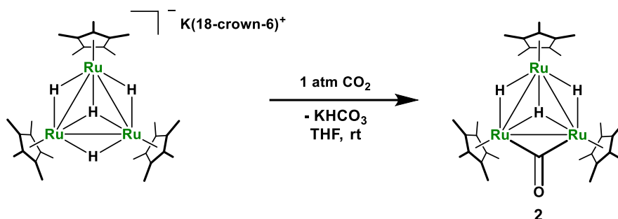
Scheme 1-6-1. アニオン性テトラヒドリドクラスターと二酸化炭素との反応による錯体 2 の合成
