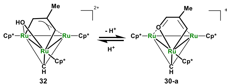
Scheme 4-2-6. 脱プロトン化によるオキサルテナシクロペンタジエン錯体の形成
