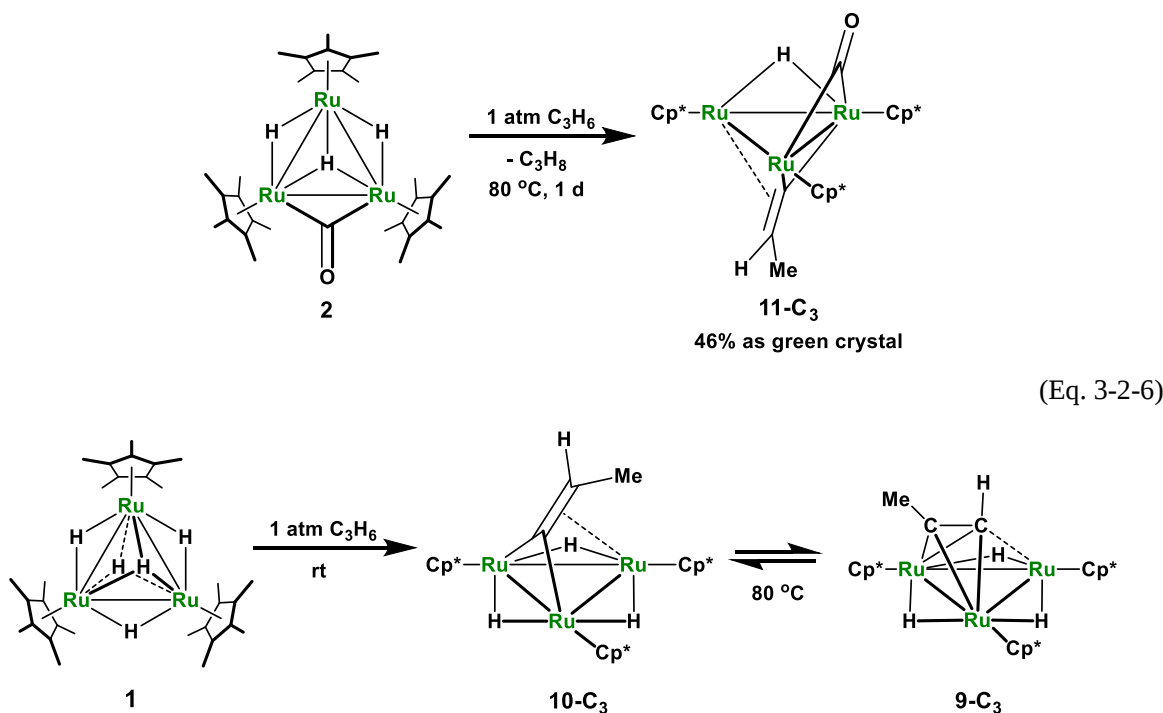
Scheme 3-2-8. 錯体 1 とプロペンとの反応
