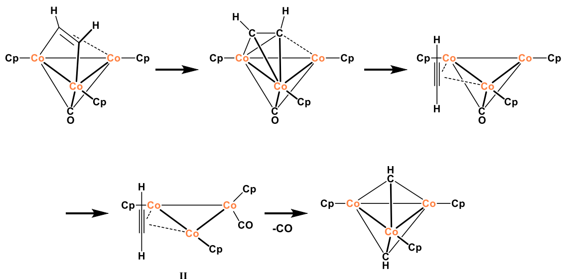
Scheme 1-5-3. 三核コバルトクラスターを用いた C\equiv C 結合切断反応 (a). カルボニル配位子を持たない場合 (b). カルボニル配位子を持つ場合
