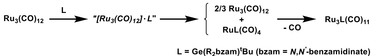
Scheme 1-2-1. \text{Ru}_3(\text{CO})_{12} とアミジナートゲルミレンとの反応
