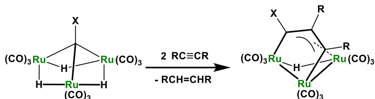
Scheme 3-5-3. アルキリジン錯体と内部アルキンとの反応によるジルテナリル錯体の形成
