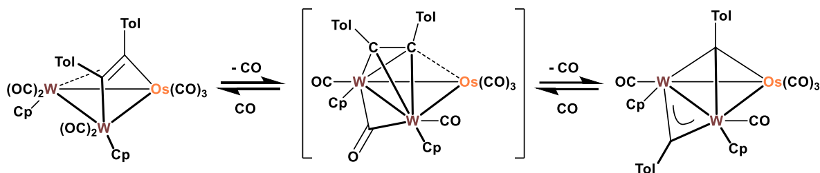
Scheme 3-2-7.2 種類のアリキジン配位子のカップリング
