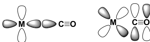
Figure 1-5-2. 末端配位における軌道の相互作用
