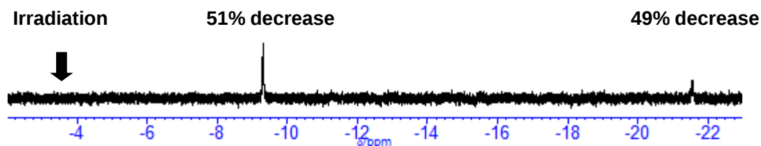
Figure 2-3-4. -70\text{ }^\circ\text{C} での錯体 2 の照射実験 (a) 照射なし (b) \delta -3.59 に照射 (400 MHz, \text{THF-d}_8 )
