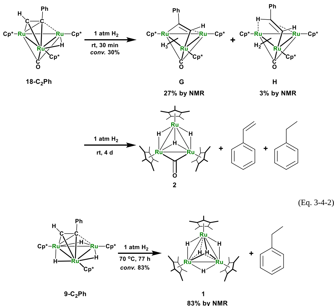
Scheme 3-4-3. 錯体 9-C 2 Ph と水素との反応
