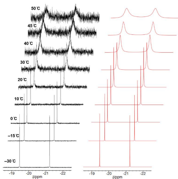
Figure 3-7-15. 錯体 21-CO の温度可変 ^1\text{H} NMR (左 : 測定データ (400 MHz, \text{THF-}d_8 )、右 : シミュレーション、ヒドリド領域)
