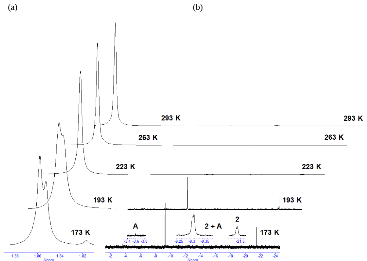
Figure 2-3-3. 錯体 2 の温度可変 ^1\text{H} NMR (a) \text{Cp}^* 領域 (b) ヒドリド 領域 (400 MHz, \text{THF-d}_8 )
