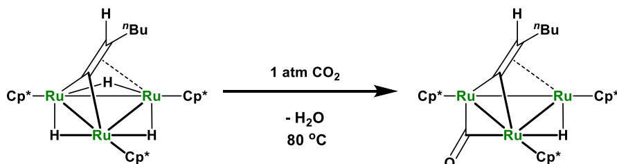
Scheme 2-1-4. 二酸化炭素由来のカルボニル配位子の形成
