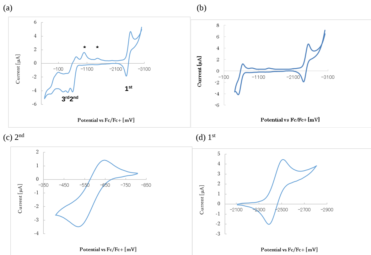
Figure 2-3-9. 錯体 2 のサイクリックボルタモグラム (錯体 1.00 \text{ mM} , 支持電解質 \text{TBAPF}_6 0.1 \text{ M} , 設定温度 25 \text{ }^{\circ}\text{C} , 作用極 Pt, 対極 Pt, 参照極 \text{Ag}/\text{Ag}^+ ( \text{TBAPF}_6/\text{MeCN} ), 内部標準 フェロセン, 掃引速度 50 \text{ mVs}^{-1} , 測定範囲 (a) -3.01 - +0.39 \text{ V} , (b) -3.01 - -0.41 \text{ V} , (c) -0.81 - -0.41 \text{ V} , (d) -2.81 - -2.11 \text{ V} )
