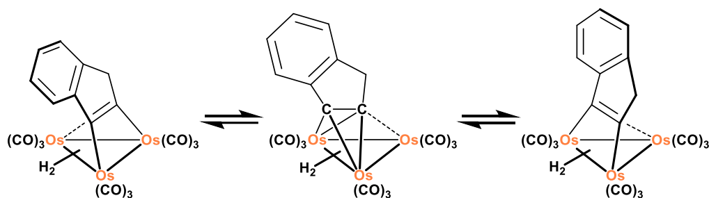
Figure 1-1-3. カルボニルクラスター上での三重架橋インデン配位子の動的挙動
