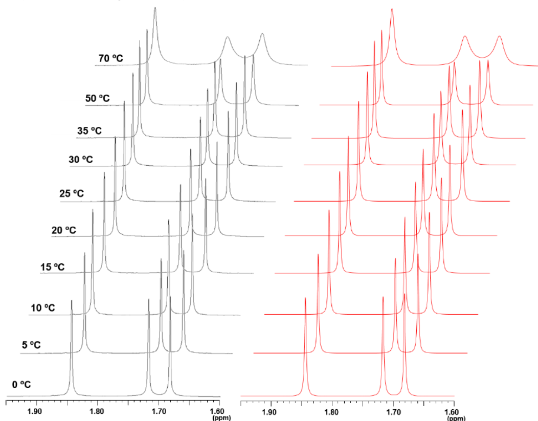
Figure 3-7-10. 錯体 18-C 2 Ph の温度可変 ^1\text{H} NMR (左 : 測定データ (400 MHz, \text{C}_6\text{D}_6 )、右 : シミュレーション、 \text{Cp}^* 領域)
