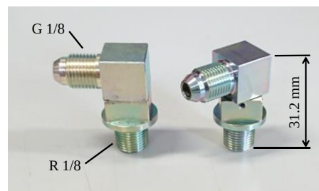
図9 1/8 インチ規格小型スィベルジョイント
