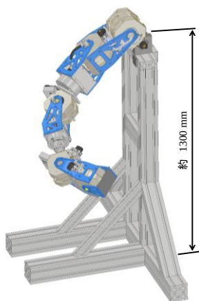
図8 開発した油圧脚ロボットー肢モデルのCAD図
