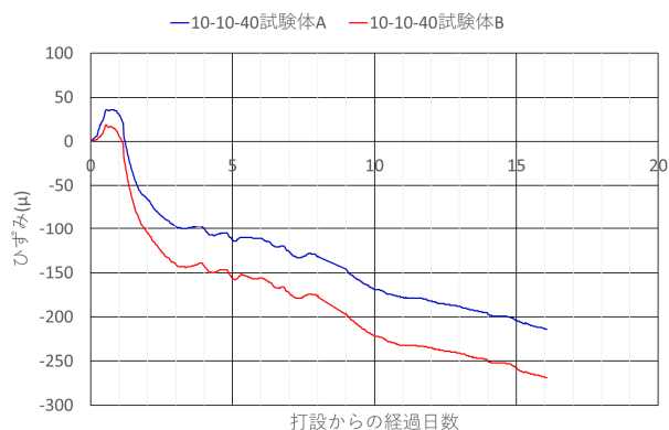
図－１ 材料のひずみ経時変化
