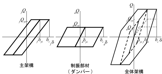
図2 復元力特性
