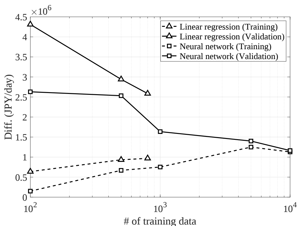
図 4.1 学習データ数に対する達成し得る最大の平均利益からの差
