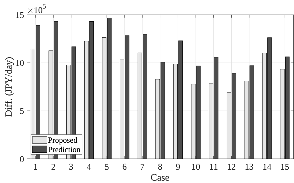
図 3.2 達成し得る最大の平均利益からの差
