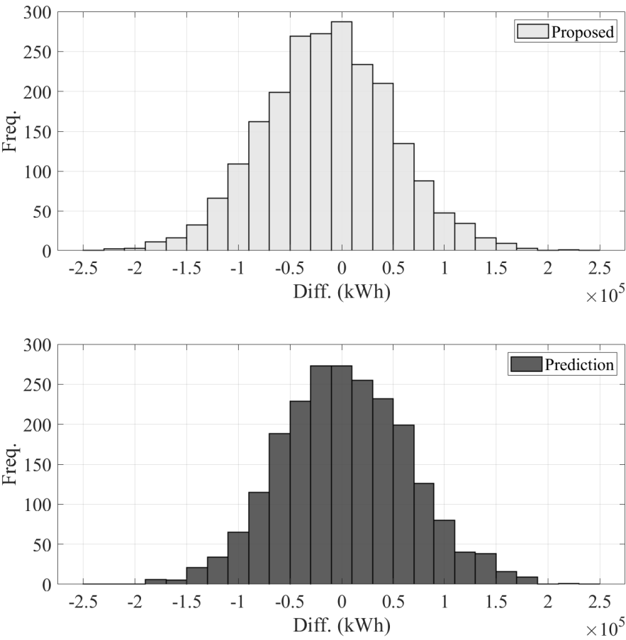
図 3.4 理想的な計画値からの差分に対するヒストグラム
