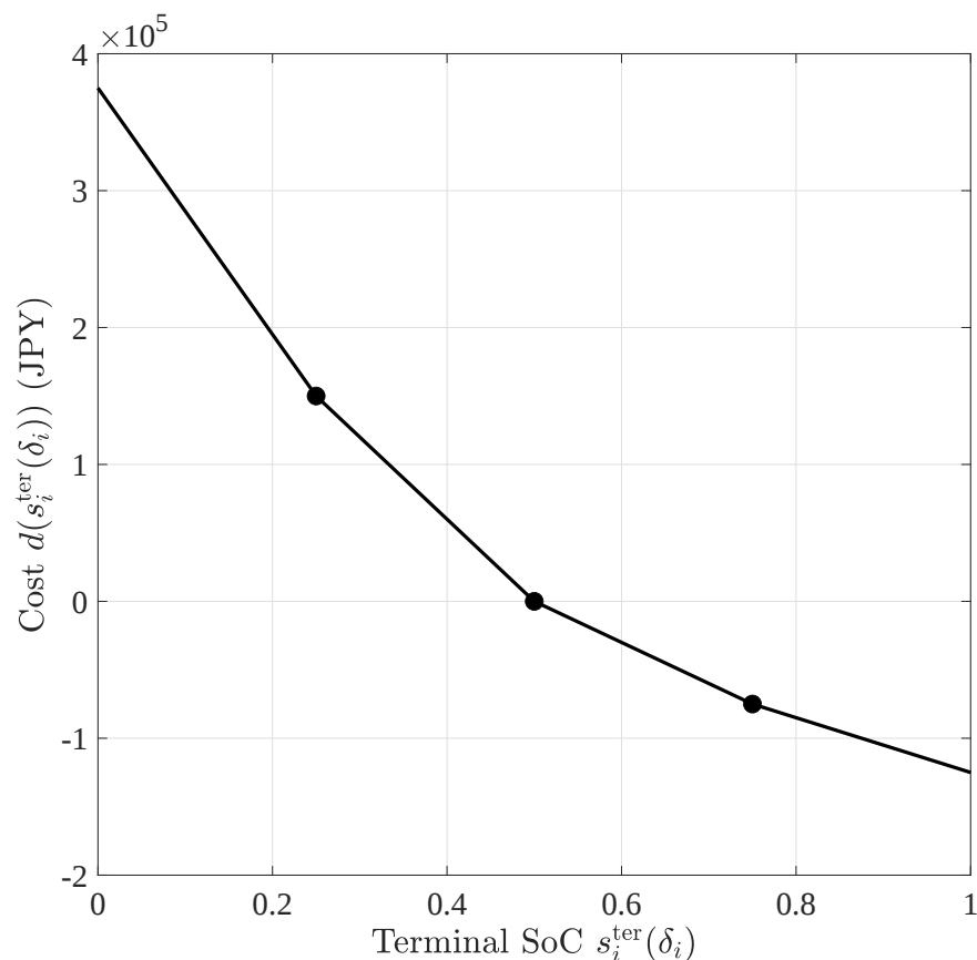
図 3.1 蓄電池の充放電量に関するコスト関数
