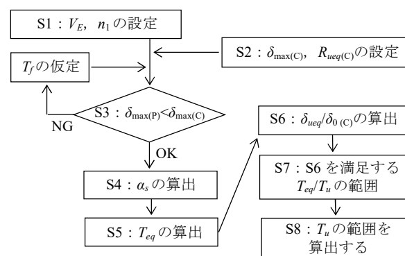
図1 設計フロー
