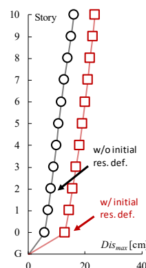
Fig. 2 Max. displacement (NS)
