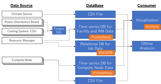
図 2 ABCI におけるジョブ情報蓄積の構成
