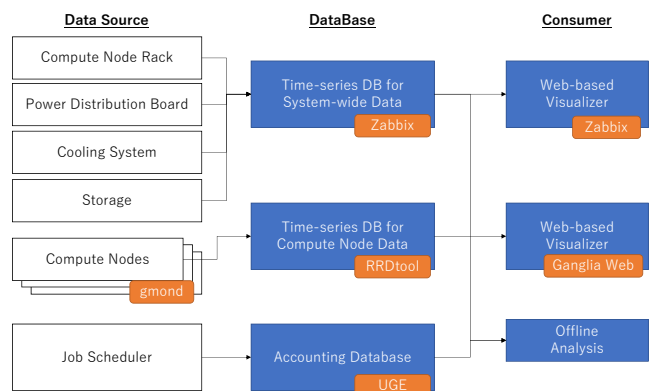
図 1 TSUBAME3 におけるジョブ情報蓄積の構成
