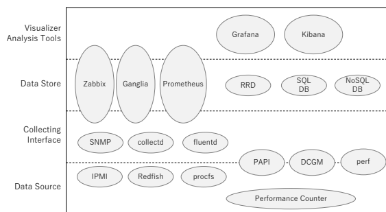
図 3 モニタリングツールと階層関係
