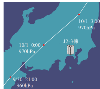
図 5 台風経路 7)
