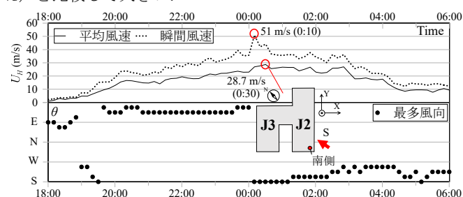
図 6 風速風向の時系列変化
