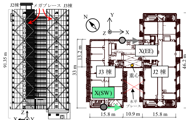
図 4 20 階平面 (加速度計位置)
