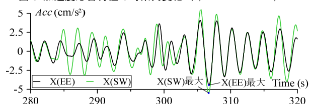
図 9 最大応答時(2018/10/1 0:10 - 0:20)の加速度時刻歴 (最大値発生時周辺)
