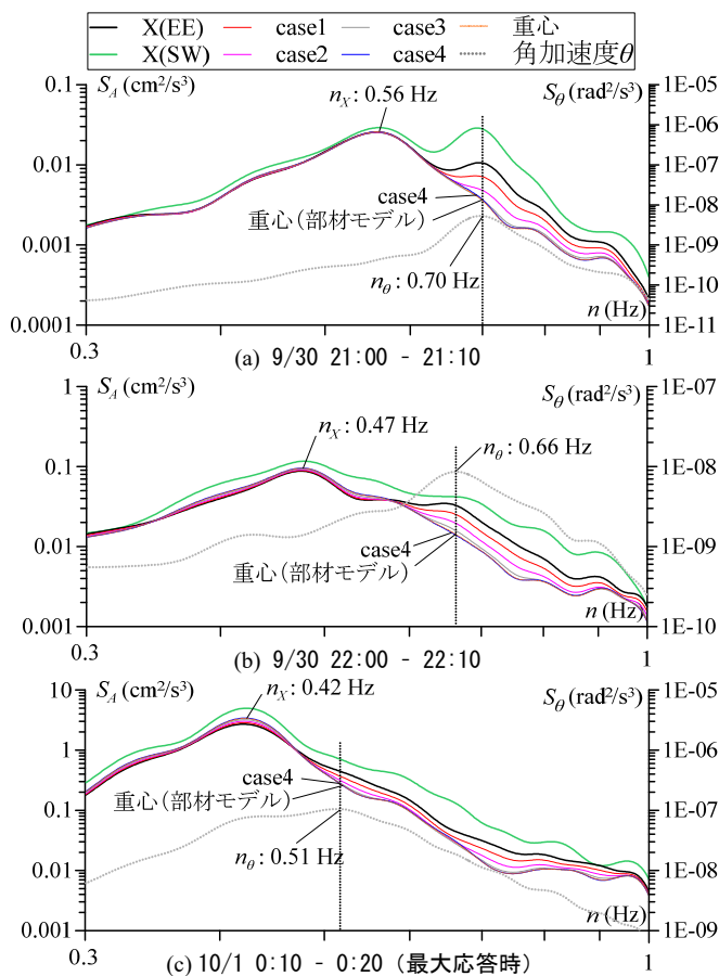
図2 並進成分XのPSD
