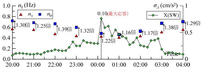
図3 固有振動数の時系列変化
