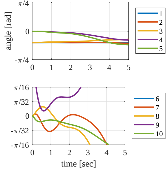
図9 ケース2での関節角時系列は発散.
