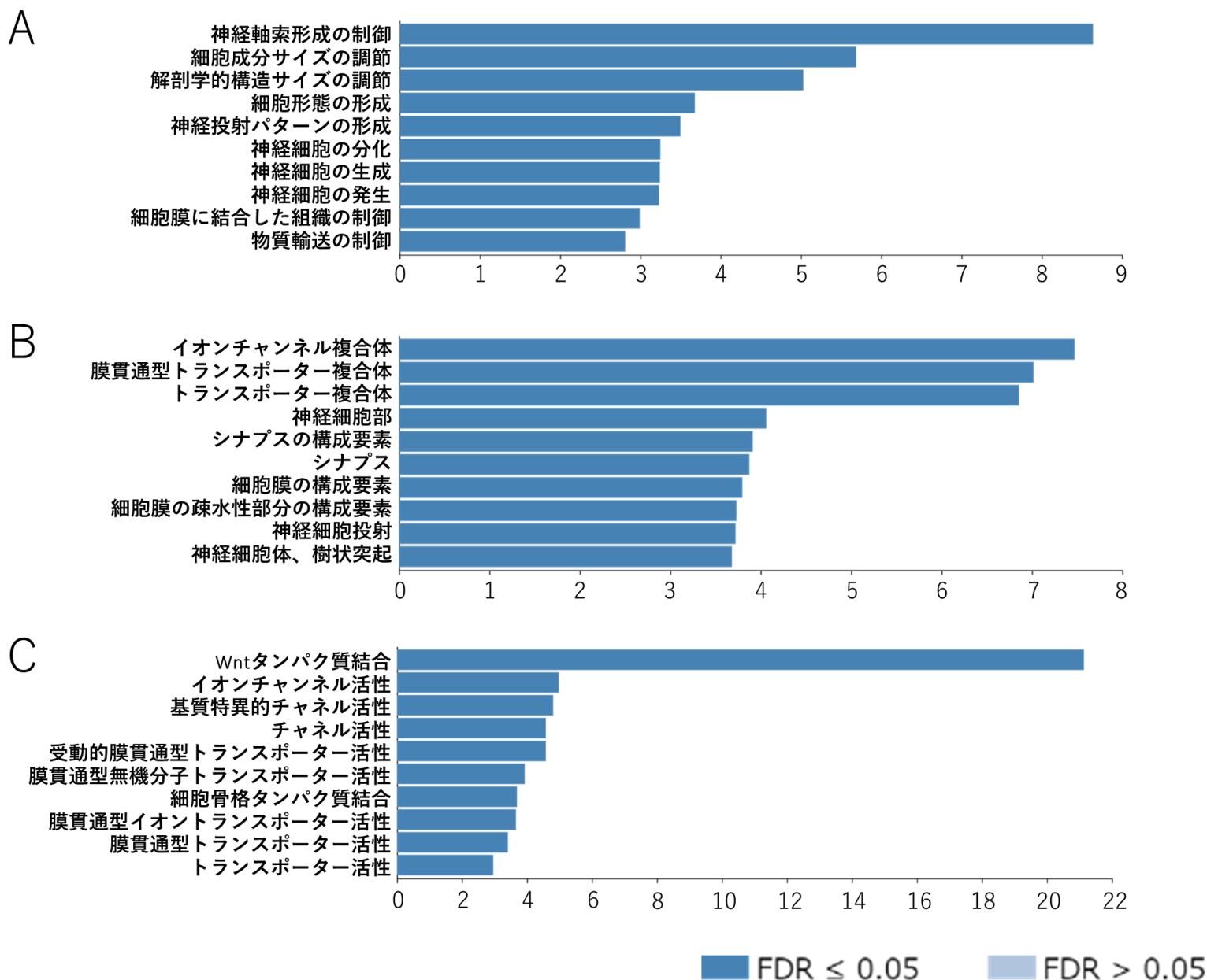
図 10. ポリプテルスの MOO で有意に多く発現していた DEG の Gene ontology (GO) 解析結果。それぞれ(A)生体内作用、(B)細胞構成要素、(C)分子機構に関する DEG の GO を示している。これらの結果は WebGestalt を用いて得られた。各グラフの縦軸は遺伝子カテゴリー、横軸はエンリッチメント率を表す（濃紺色のバーは FDR \leq 0.05 、水色のバーは FDR > 0.05 を示す）。
