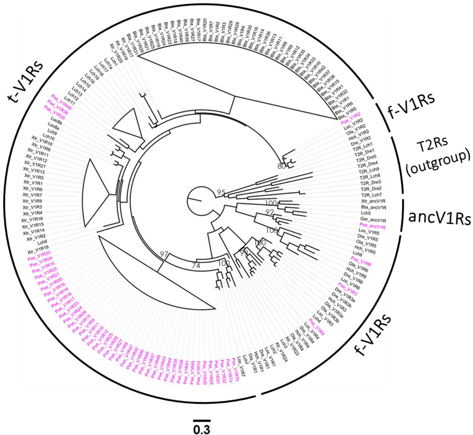
図 7. ポリプテルスを含む 8 種の脊椎動物の V1R の系統樹。図に示した脊椎動物 7 種の略式名は以下の通り。Pse (ポリプテルス)、Loc (スポッテッドガー)、Ola (メダカ)、Hch または Oni (シクリッド)、Dre (ゼブラフィッシュ)、Lch (シーラカンス)、Xtr (ネッタイツメガエル)、Bta (ウシ)。ポリプテルス V1R はマゼンダ色で示した。ブートストラップ値は各枝の根元に部分的に示されている。スケールバーは各枝におけるアミノ酸置換数を表す。
