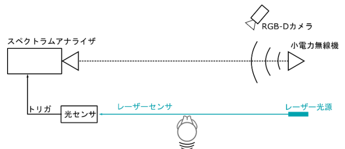
図 1 動的遮蔽特性と動体の同時測定系
