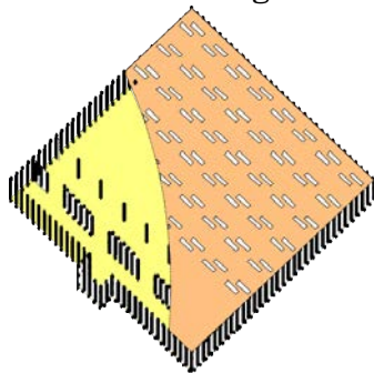
(d) Post-wall waveguide
