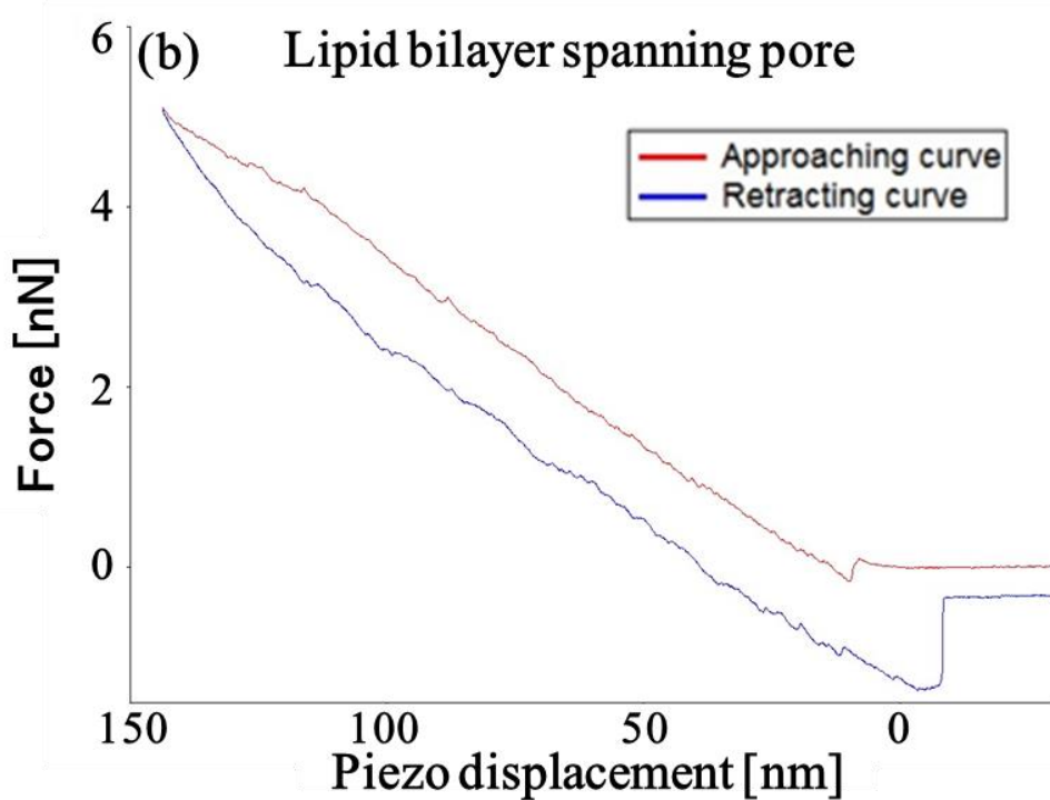
図 5.8 自発展開を行ったサンプルのそれぞれのフォースカーブ. (a)メンブレンフィルタ表面 (b)メンブレンフィルタ小孔.
