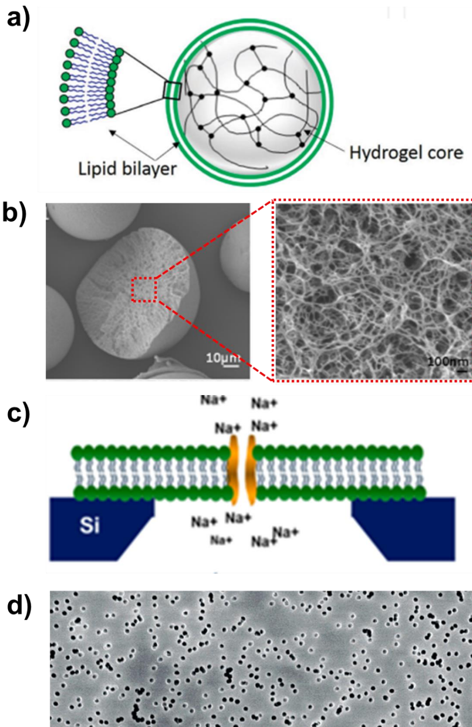
図 1.5 小孔支持型脂質二重膜の概略図. (a) 小孔支持型 GUV の概略図. 脂質二重膜内にハイドロゲルが内包されている[Kazakov 2017]. (b) agarose ゲルの電子顕微鏡写真[Nwekw 2017(一部改編)]. (c) 小孔支持型 SLB の概略図. 脂質二重膜が小孔上に形成される[Khan 2017]. (d) ポリカーボネート基板の電子顕微鏡写真[Favero 2005].
