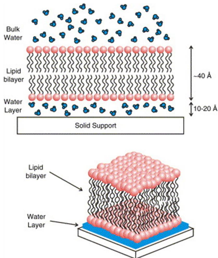
図 1.4 人工脂質二重膜の概略図. (a) ベシクルの概略図. サイズによってさらに分類でき, 1000 nm 以上の巨大なものは giant unilamellar vesicle (GUV)と呼ばれる. [Mozafari 2021]. (b) 支持型平面脂質二重膜(SLB)の概略図. 脂質二重膜が固体基板に支持され, 間に 1-2 nm の水層を挟む[Castellana 2006].
