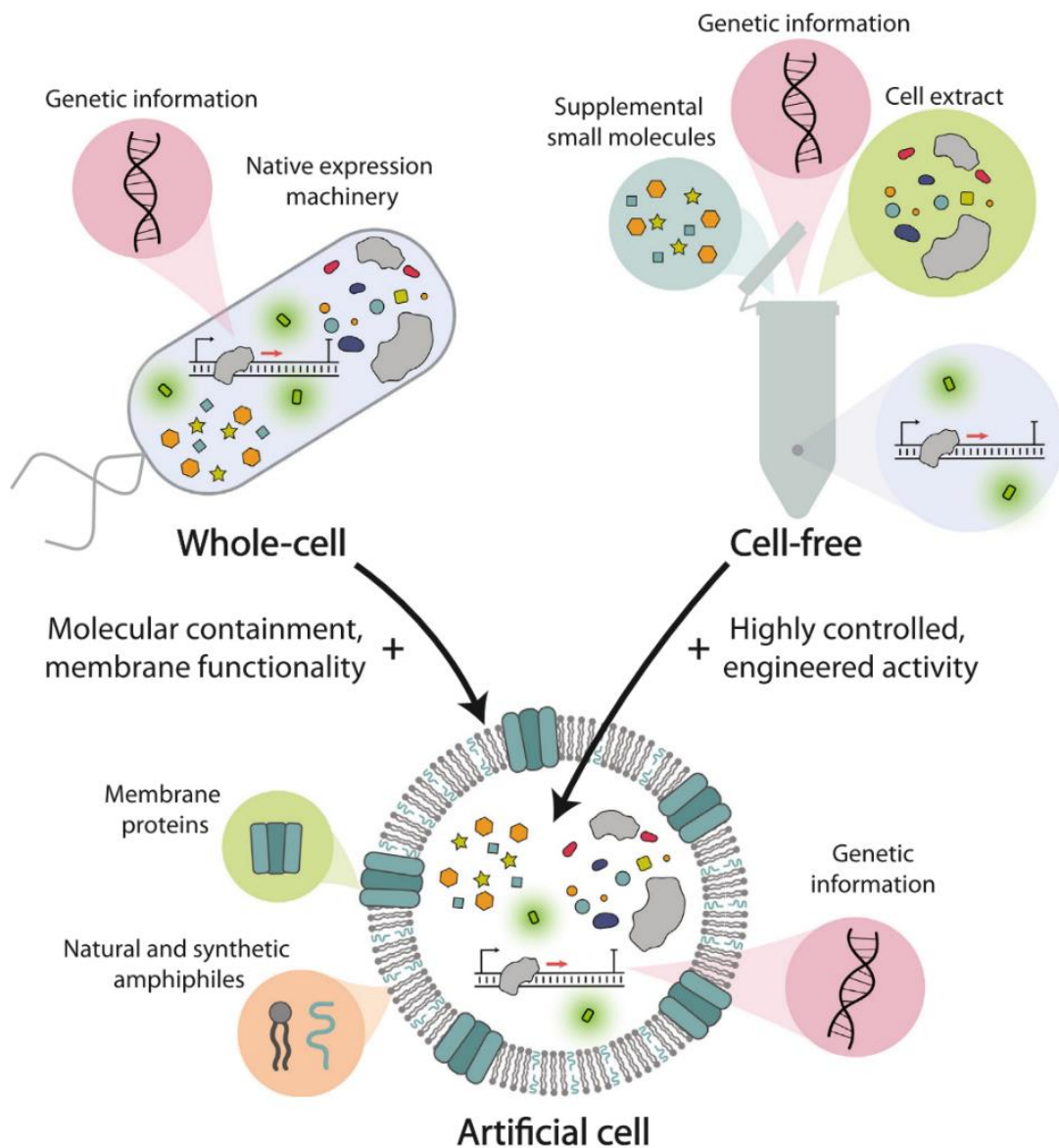
図 1.1 人工細胞の概要図. 脂質二重膜, DNA やタンパク質などの生体分子を組み合わせることで機能を実現する[Boyd 2021].
