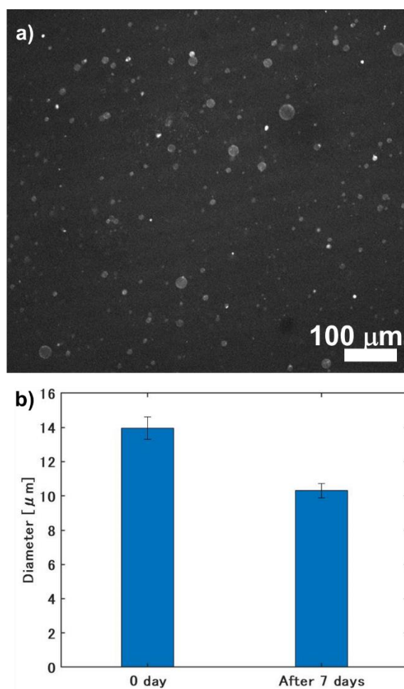
図 3.6 小孔支持型 GUV の寿命. (a) 4℃の冷蔵庫内で 7 日間保存した小孔支持型 GUV の蛍光画像. (b) 小孔支持型 GUV の直径変化.
