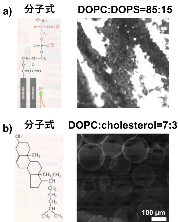
図 3.7 脂質の種類の検討. (a) PS の分子式と、形成した小孔支持型 GUV. (b) cholesterol の分子式と、形成した小孔支持型 GUV. 分子式は[ Alberts 2014]より引用.
