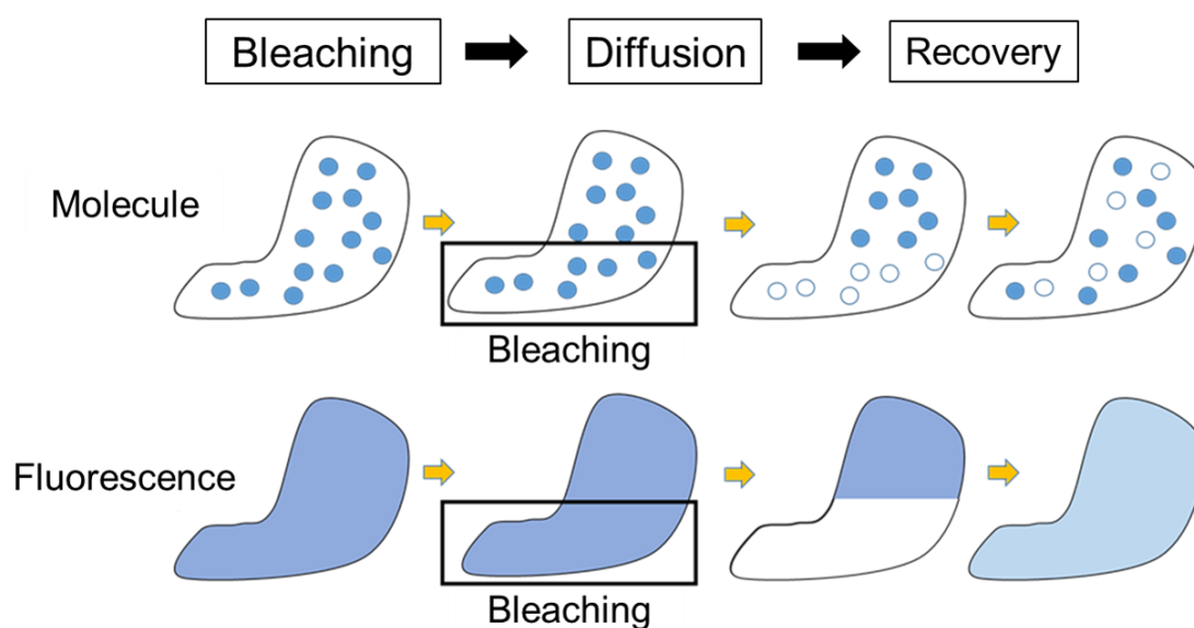
図 4.5 FRAP の模式図
