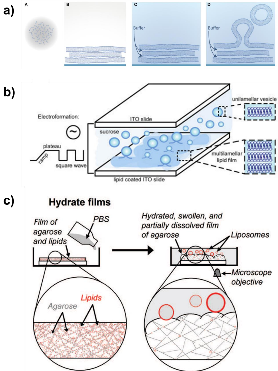
図 2.1 オイルフリーの GUV 形成法. (a) 静置水和法 [Stein 2017]. (b) Electroformation 法 [Schmid 2017]. (c) ポリマーフィルム水和法 [Horger 2019].
