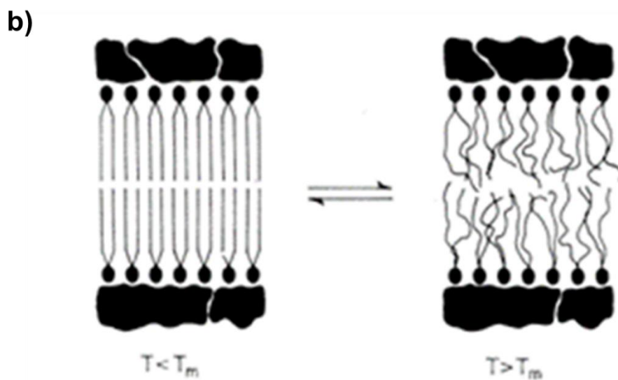
図 5.3 小孔支持型 SLB の展開速度. (a)それぞれの条件下での SLB の展開速度. ▲ : メンブレンフィルタ, 22℃. ◆ : メンブレンフィルタ, 33℃. ■ : ガラス, 22℃. ● : ガラス, 33℃. (b) 温度の上昇とリン脂質分子の流動性の関係[坂本明郎 1998].
