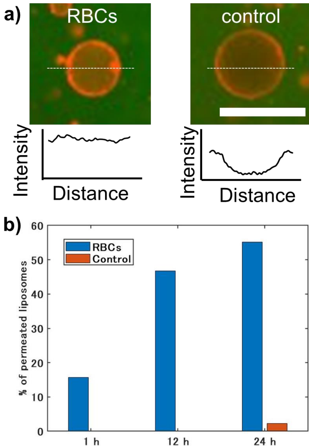
図 3.5 膜タンパク質の導入. (a) 膜タンパク質が導入された小孔支持型 GUV (RBCs) と導入されていない小孔支持型 GUV(control)の蛍光画像. スケールバー : 20 \mu\text{m} (b)calcein に侵入された小孔支持型 GUV の割合の時間変化.
