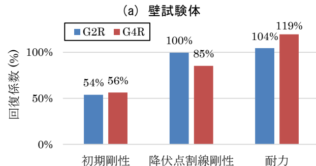
図 3 各性能値の回復係数
