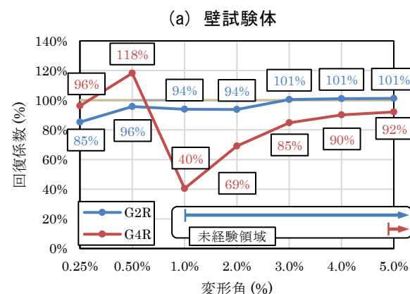
図 4 等価粘性減衰定数の回復度推移
