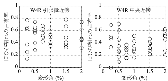
図 5 試験体 W4R のひび割れの旧ひび割れ占有率
