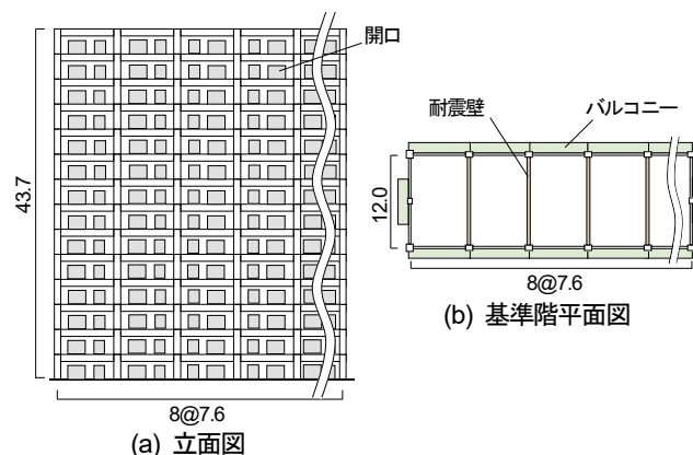
図2 14Model 概要 (単位: m)
