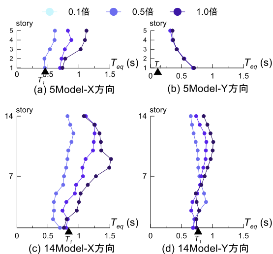
図 10 T_{eq} の高さ方向分布
