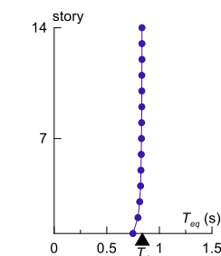
図 A-1 T_{eq} の高さ方向分布
