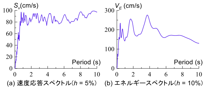
図7 入力地震動スペクトル(1.0倍)
