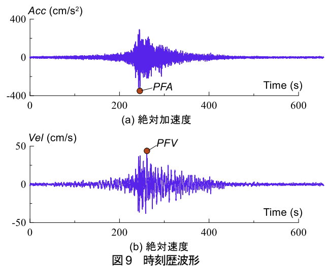
図9 時刻歴波形
