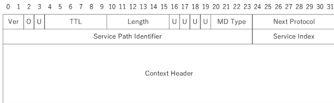
図 2.2 NSH ヘッドフォーマット
