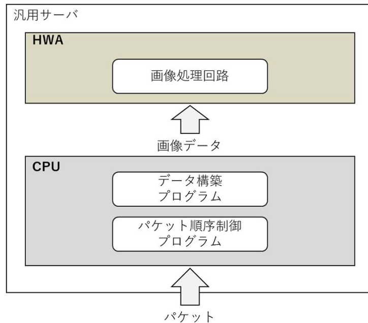
図 1.2 典型的な CPU-HWA サーバアーキテクチャにおける処理手順
