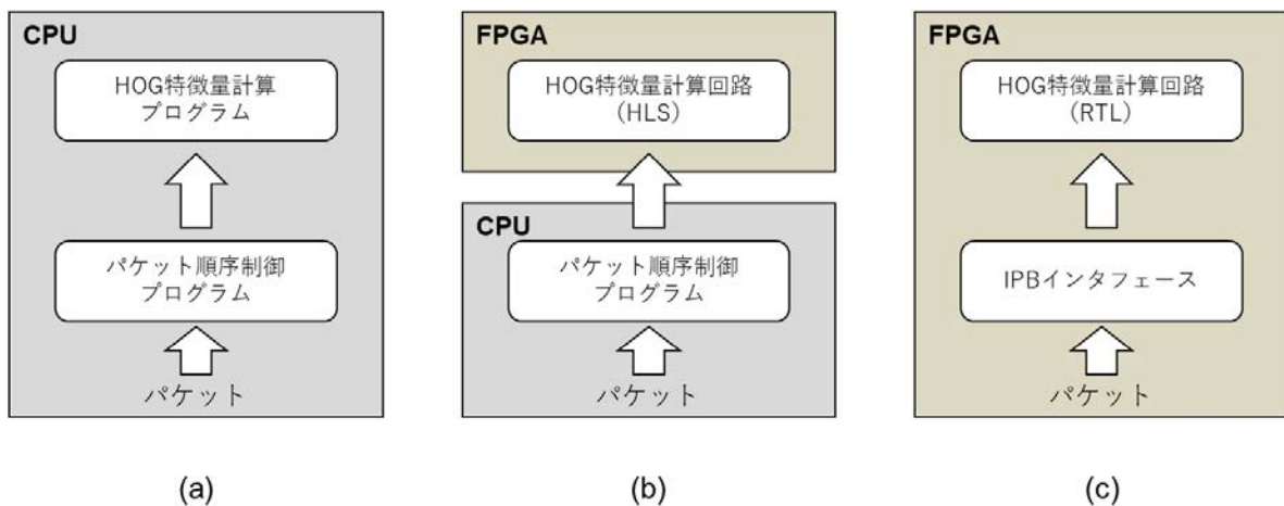
図 3.11 (a)SW-SW 構成, (b)SW-HW 構成, (c)HW-HW 構成の HOG 特徴量計算機能
