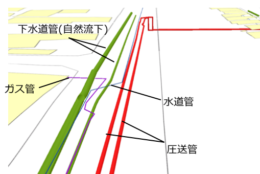
図-1 圧送管と周辺埋設管の3次元モデル
