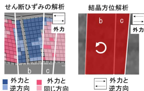
図5 外力に逆らったせん断が働いたキンクバンドの存在
