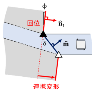
図4 せん断されたキンク界面で生じる回位と連携変形
