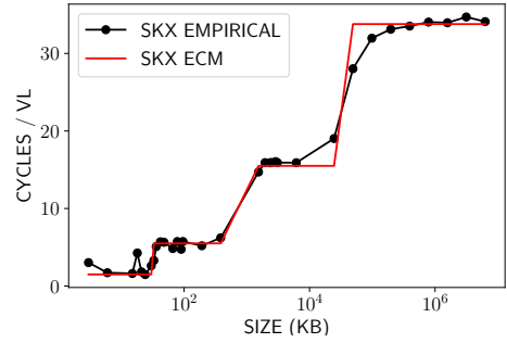
(b) Intel Xeon Gold 6148
