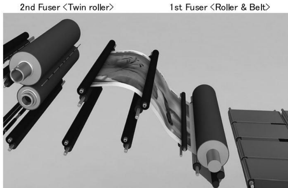
Fig. 1-20 imagePRESS C7000VP に搭載のデュアル定着システム[1-14]
