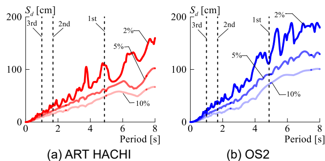
図2 変位応答スペクトル
