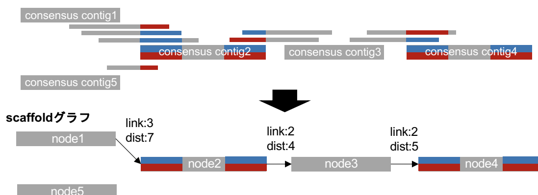
図 13 scaffold グラフの構築
