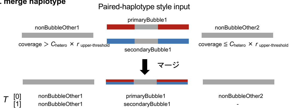
図 9 Merge haplotype
