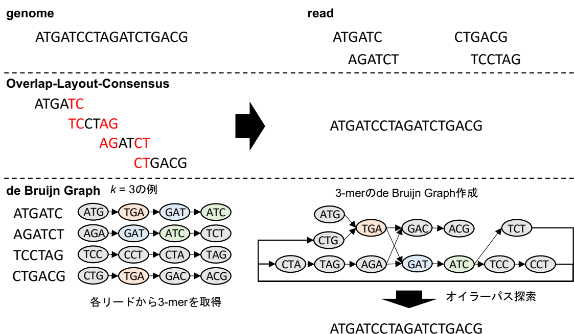
図 3 contig assembly の方法の比較
