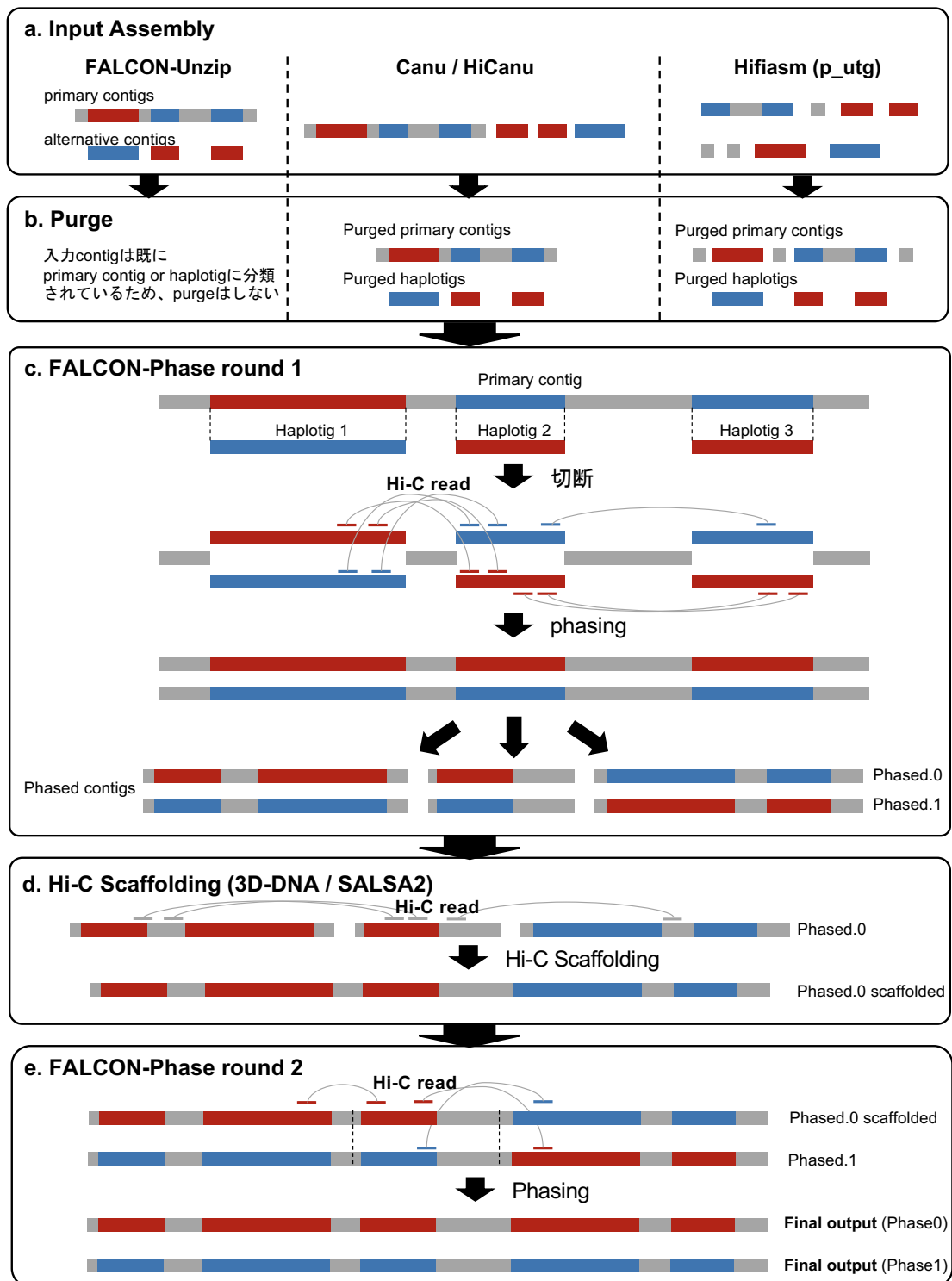
図 23 FALCON-Phase と Hi-C Scaffolding ツールの実行方法
