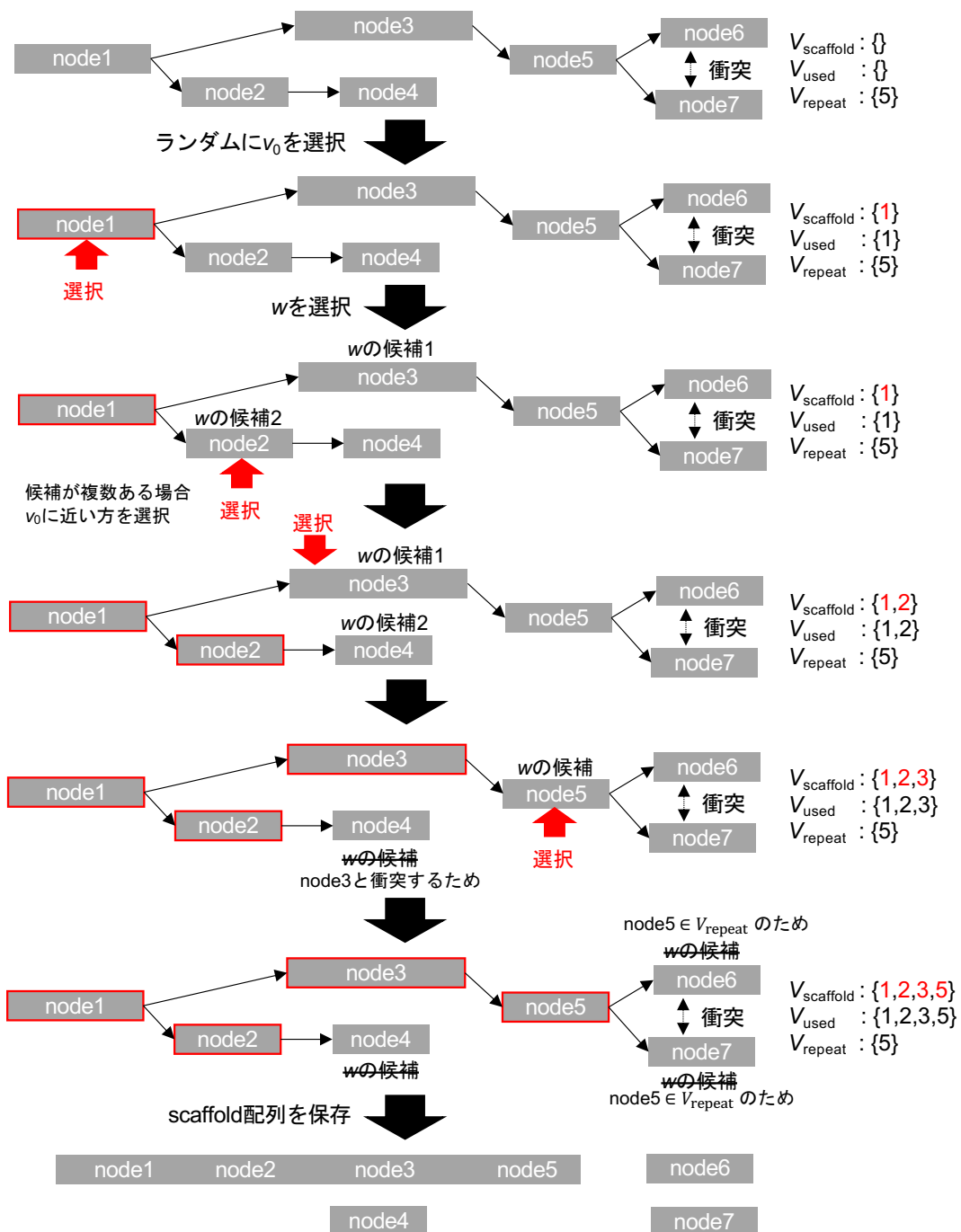
図 17 scaffold 構築
