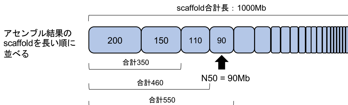
図 24 N50 の説明
