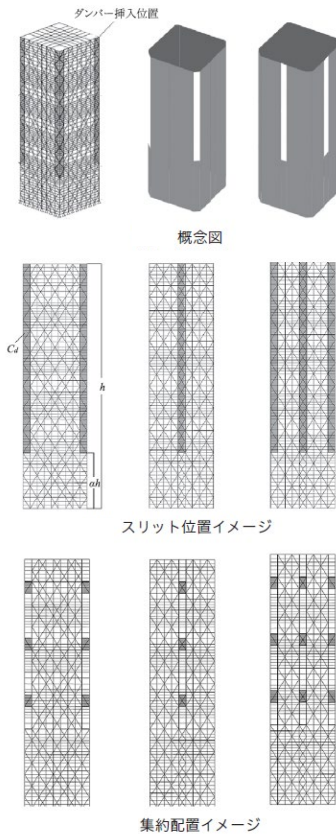
Figure 5.2.3 Damped braced tube のバリエーション
