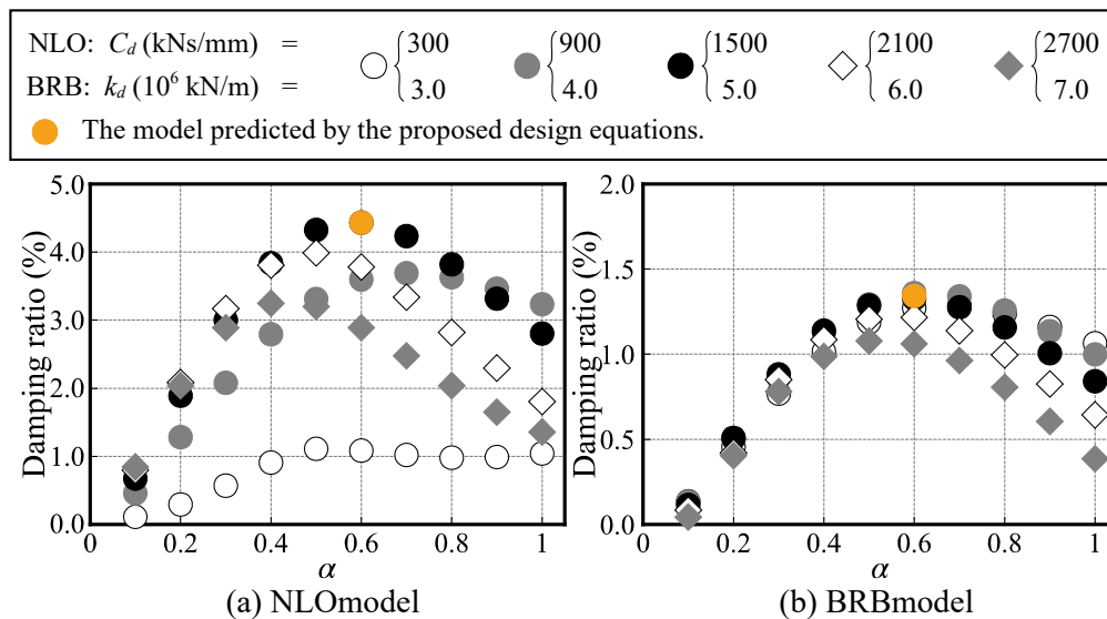
Figure 4.4.2 1次モード減衰比と \alpha の関係（XX-Lv.2）
