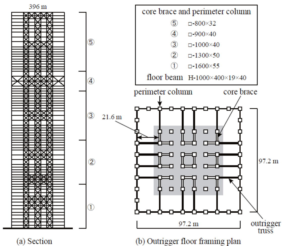
Figure 4.4.1 検討対象建物（高さ 396m, 70 層）
