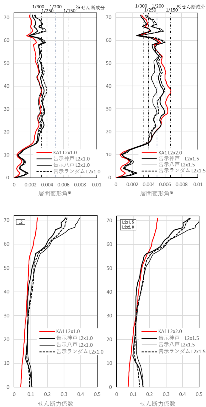
Figure 6.6.2 地震応答解析結果
