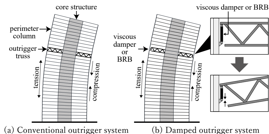
Figure 1.2.1 アウトリガー構造の概念図
