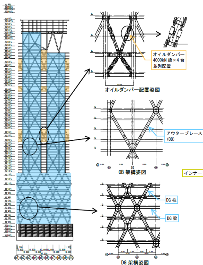
Figure 6.5.2 外殻構面軸組図
