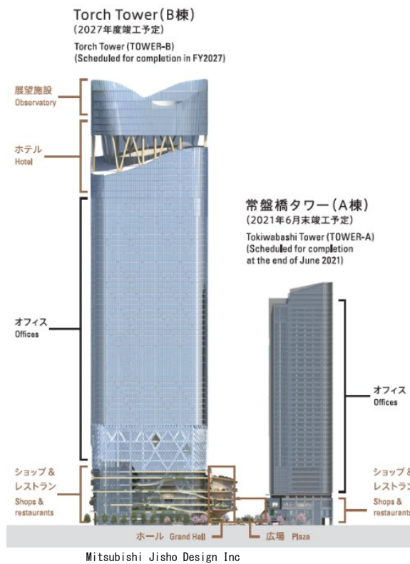
Figure 6.3.2 断面構成図
