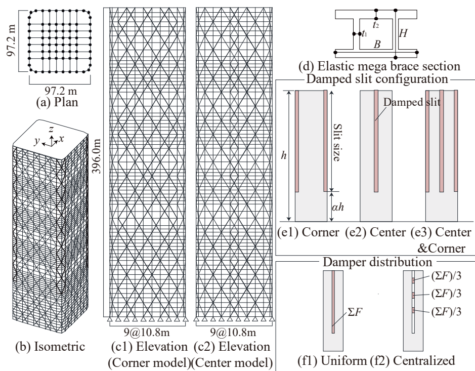
Figure 5.4.4 解析モデルとパラメータ
