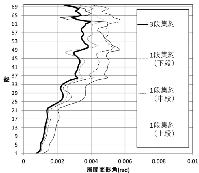
Figure 5.3.11 集約配置モデル（1 段・3 段）の比較
