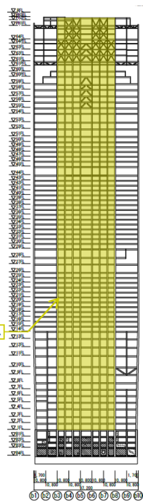
Figure 6.5.3 インナーフレーム軸組図
