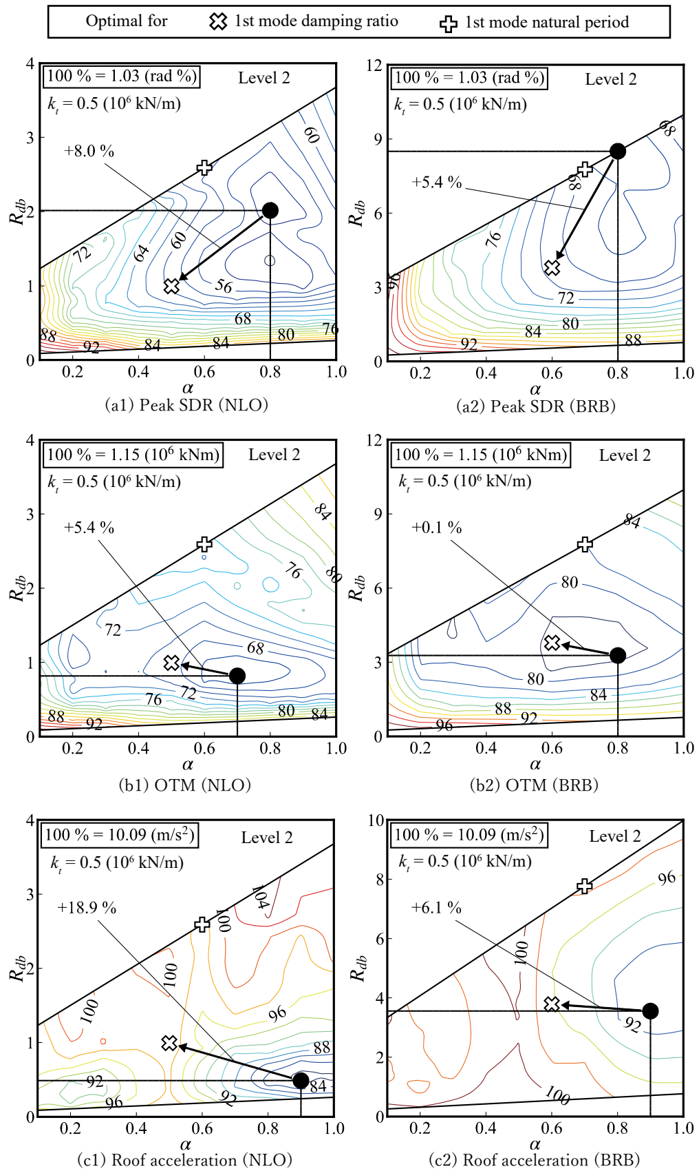
Figure 4.3.17 地震応答比の等値線図 (32 層モデル)
