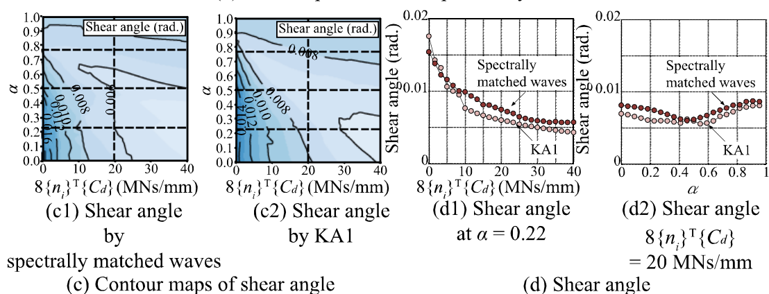
Figure 5.5.6 地震応答解析の結果の等値線図（線形オイルダンパー均等配置）
