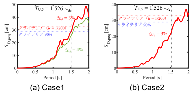
Fig. 6 HB (RC 造) の応答スペクトル
