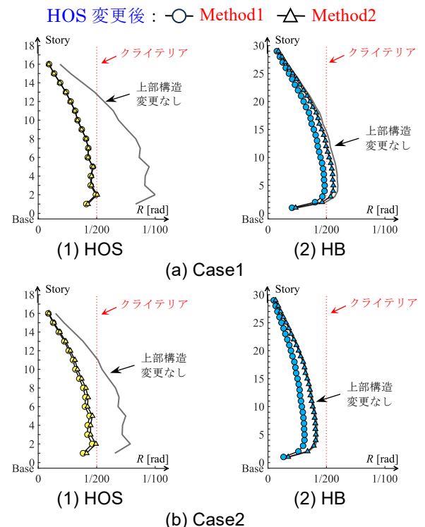
Fig. 8 層間変形角の高さ方向分布 (HOS のみ変更)
