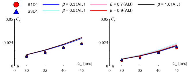
図4 免震建物と荷重指針の C_B の比較
