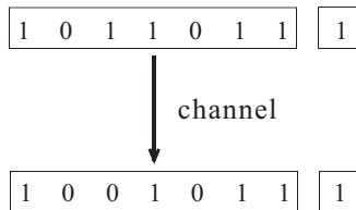
FIG. 5.1. Parity-check code
