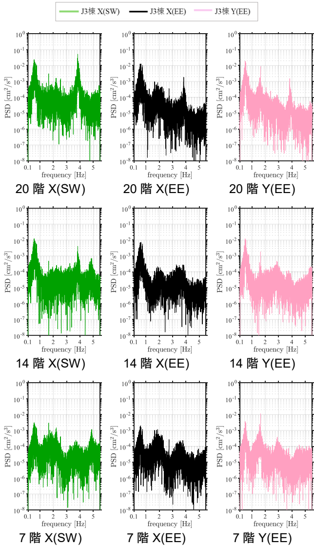
図 8 T2407 最接近時の加速度の PSD (2024/8/16 17:30 -17:40)
