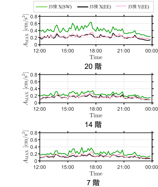
図 7 最大応答加速度の時系列変化
