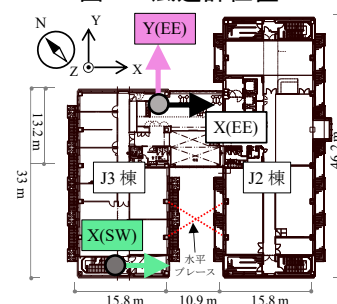
図3 J3 棟基準階 加速度計設置位置
