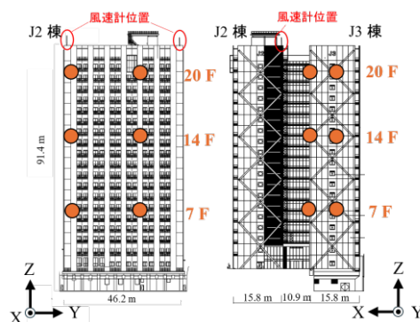
図1 J2-3 棟立面
