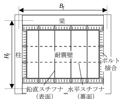
図1 鋼板耐震壁
