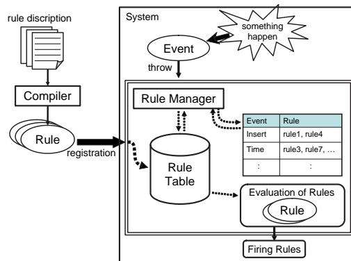
図1 全走査によるルール処理方法
