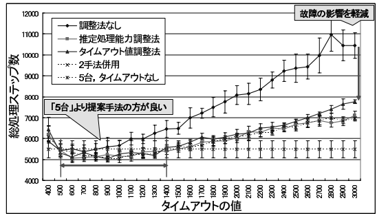
図 7 故障時における再割当手法の違いによる総処理ステップ数の比較
