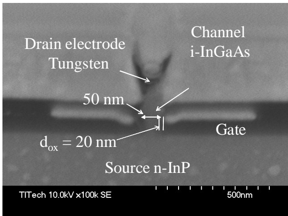
図 5 断面 SEM
