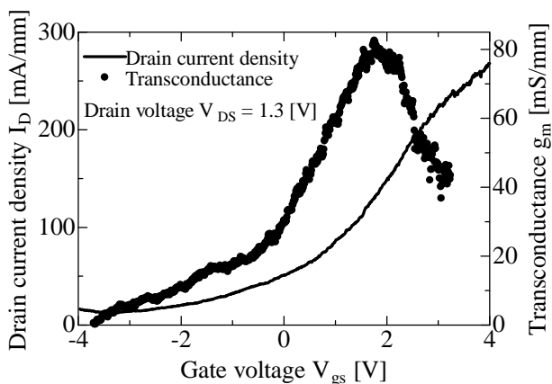
図8 新しく提案した素子の伝達特性
