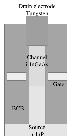
図 1 提案する素子構造
