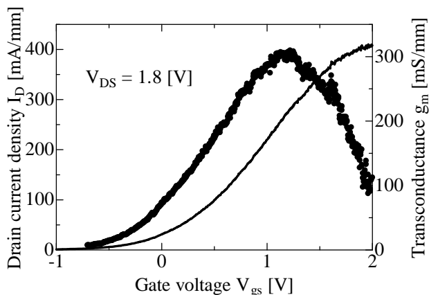
図 10 ゲート絶縁膜が 5 nm の素子の伝達特性
