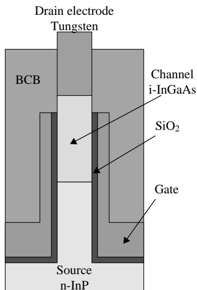
図 6 新しく提案する構造 Fig. 6 Schematic image of device
