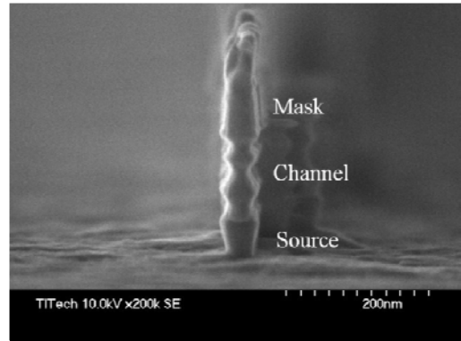
図 2 作製したメサ
