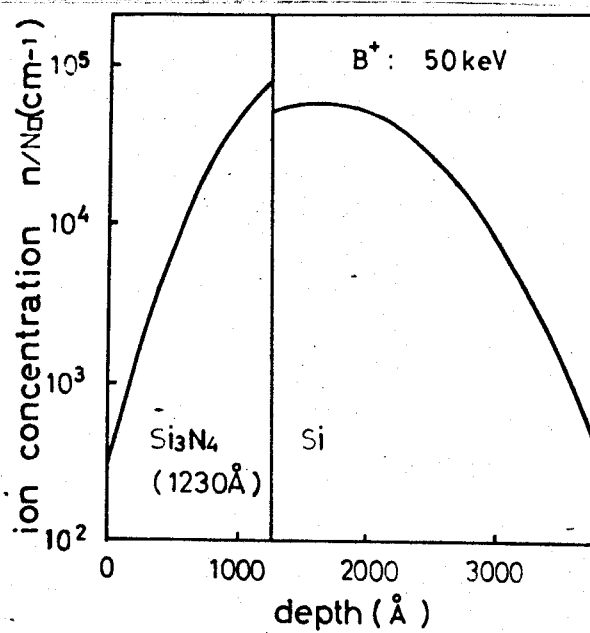
図5-9 \text{SiO}_2 、 \text{Al}_2\text{O}_3 およ び \text{Si}_3\text{N}_4 層の付いた Si 基板 中の 50 keV、 B^+ イオンの分 布。(等価厚みの層が付い た場合。) (T-F pot.)
