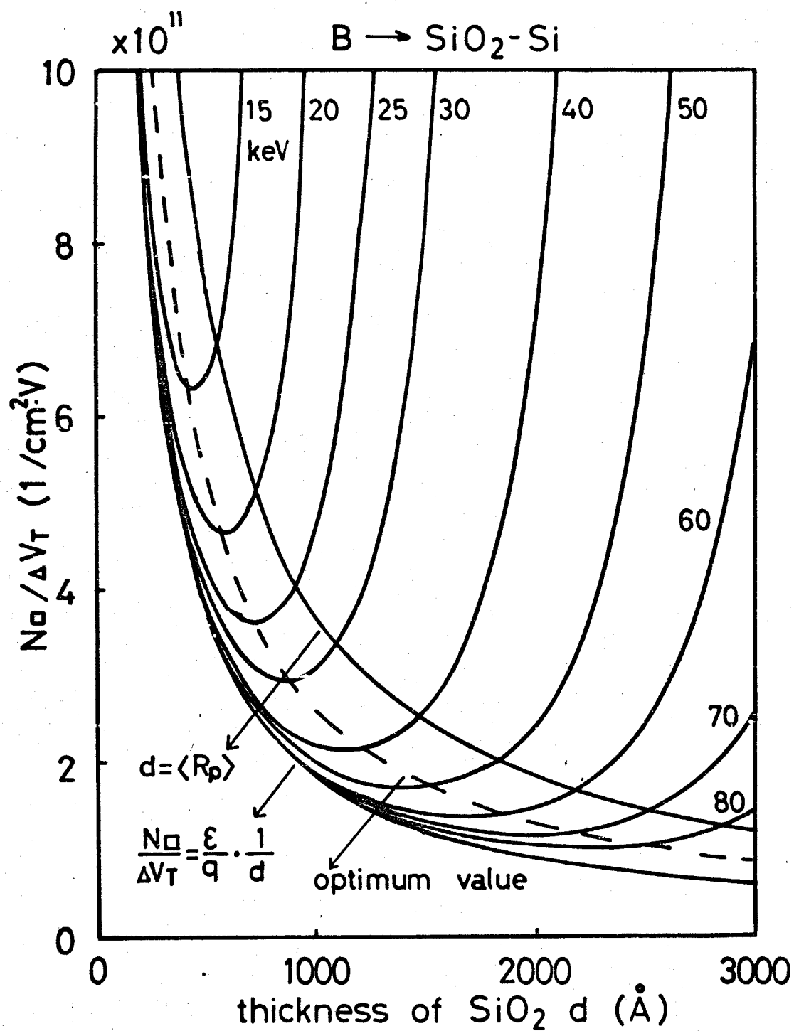
図5-11 MOSFETの閾値電圧制御のための最適打ち込み条件。(Bイオンを注入した場合。)
