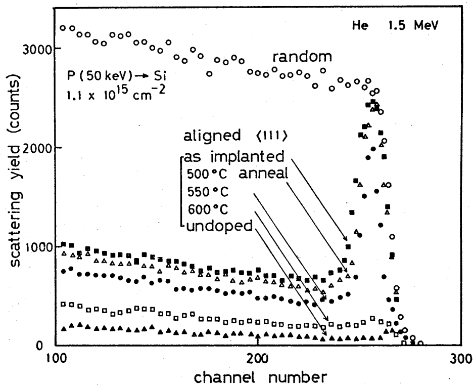
図 8-5 P 打ち込み試料のアニール特性
