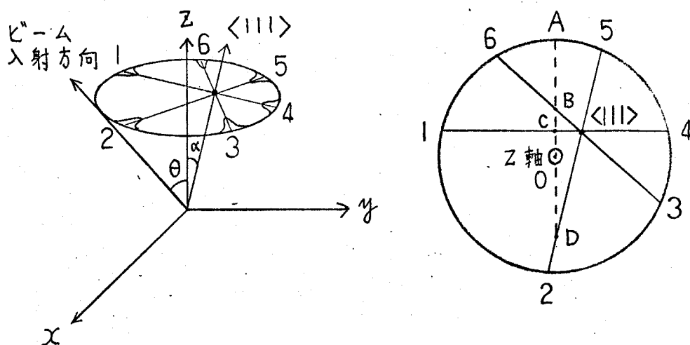
図8-3 結晶軸合わせの方法 (面心立方結晶 \langle 111 \rangle 軸)
