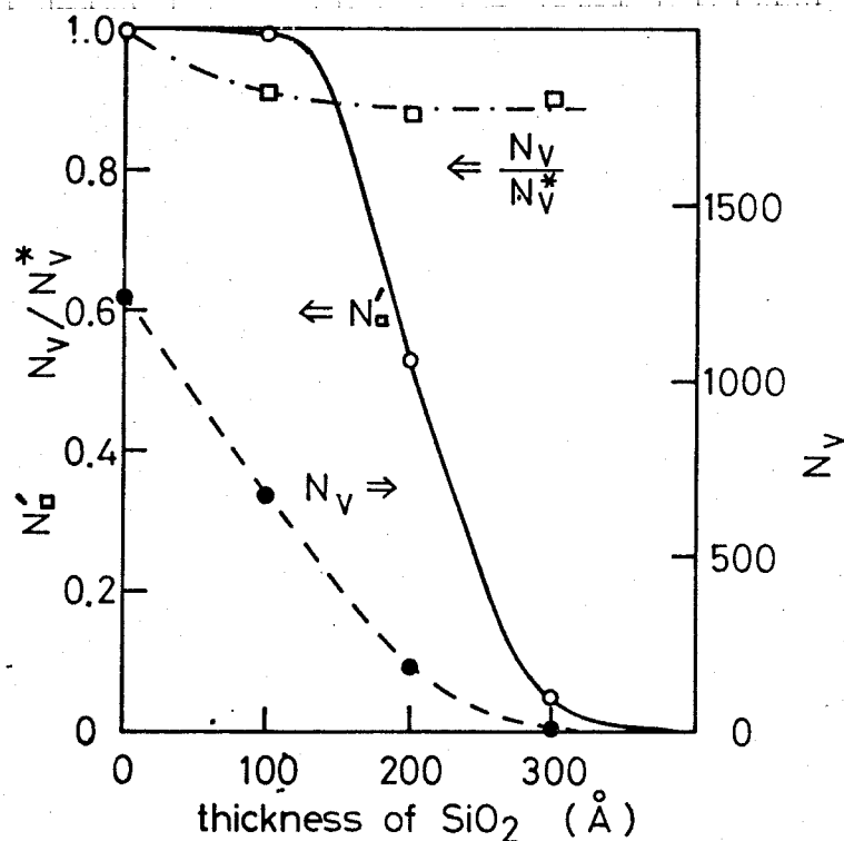
図 6-11 \text{Si} 中にできる格子欠陥数の \text{SiO}_2 膜厚による変化 ( r^{-2} pot.)
