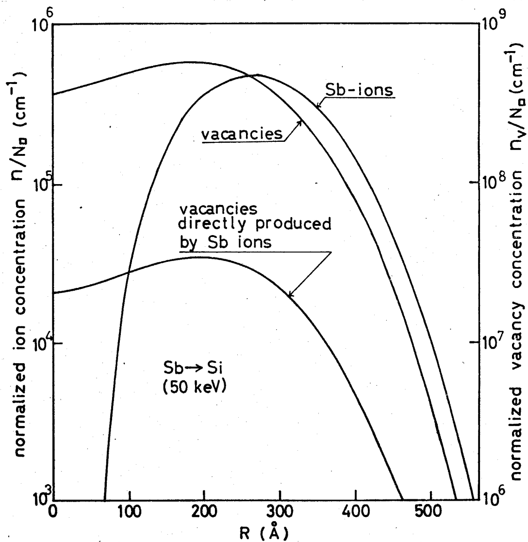
図 6-5 50 keV Sb イオンによる Si 基板中の 格子欠陥分布 ( r^{-2} pot.)
