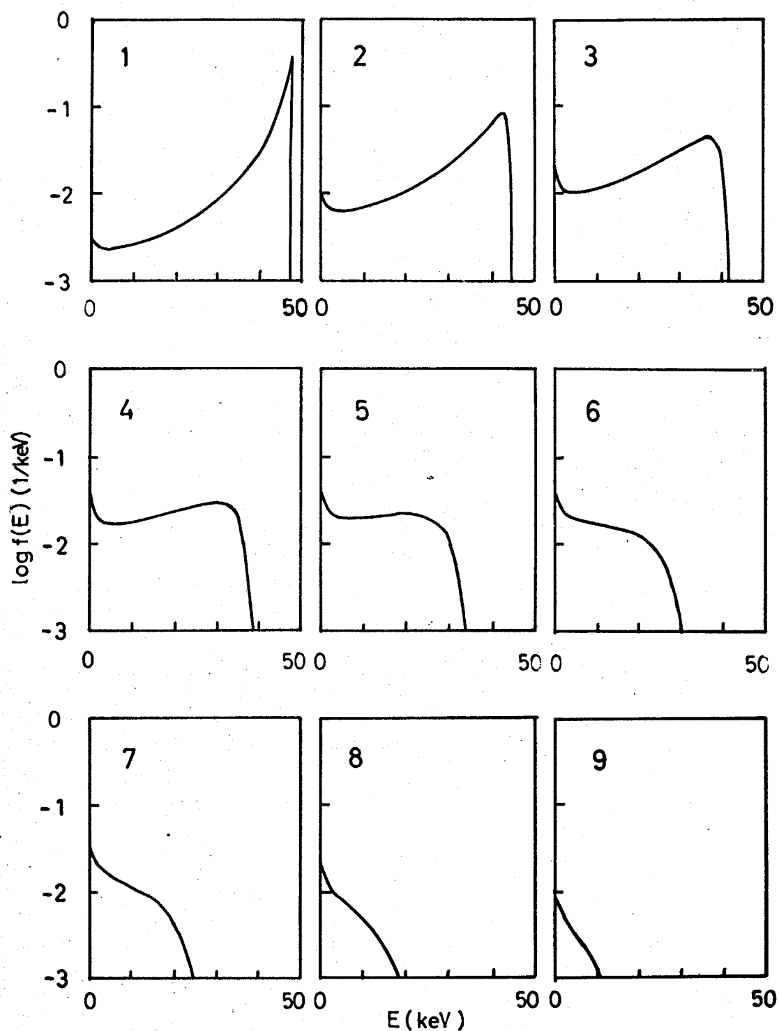
図 4-10 Thomas-Fermi ポテンシャルを用いた場合の基板中のイオンのエネルギー分布。(50 keV Ar \rightarrow Si) (T-F pot.)
