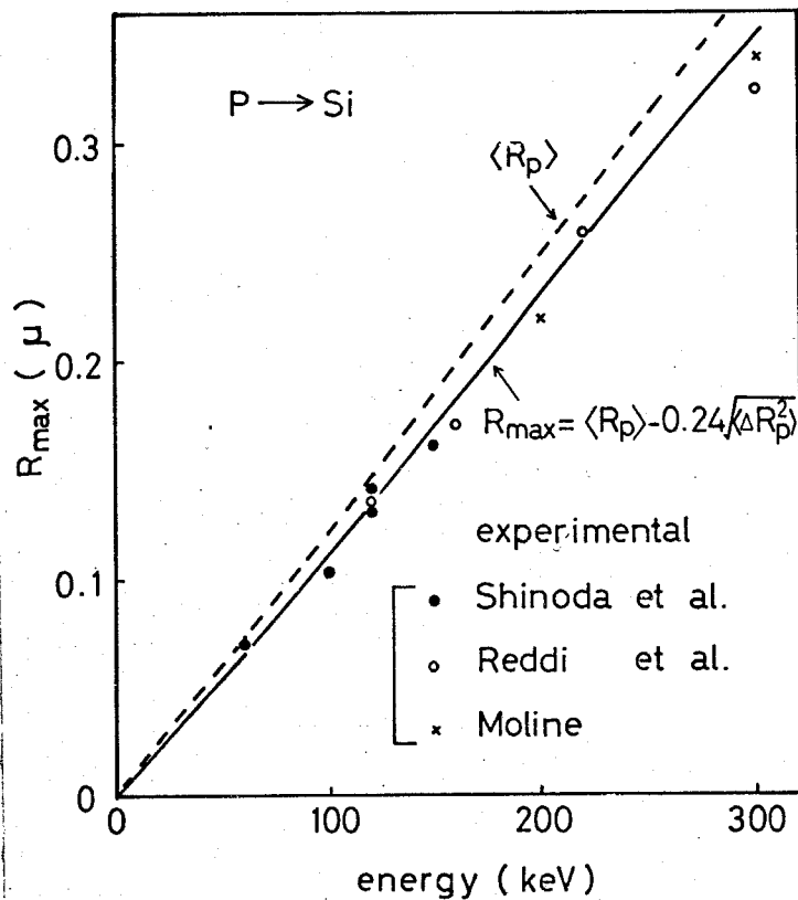
図3-9 Si中のPイオン濃度最大点と打ち込みエネルギーとの関係。 (T-Fpot. + r^{-2} pot.)
