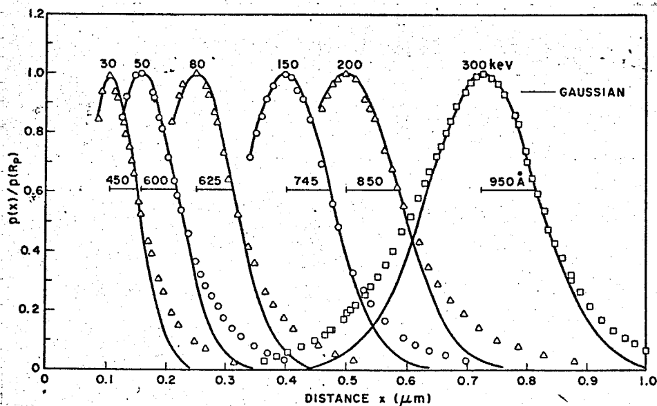
図 2-9. 非晶質基板中のイオン分布の一例*。(B イオンを Si 基板に注入した場合。) (122)
