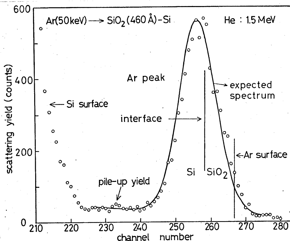
図 7-13 \text{SiO}_2 -Si 基板中の 50 keV Ar イオンを測定した後方散乱スペクトル。理論値に用いた pile up yield は、235~240 ch. および、273~278 ch. の pile up 量を、最小 2 乗法を用いて直線で近似したものである。
