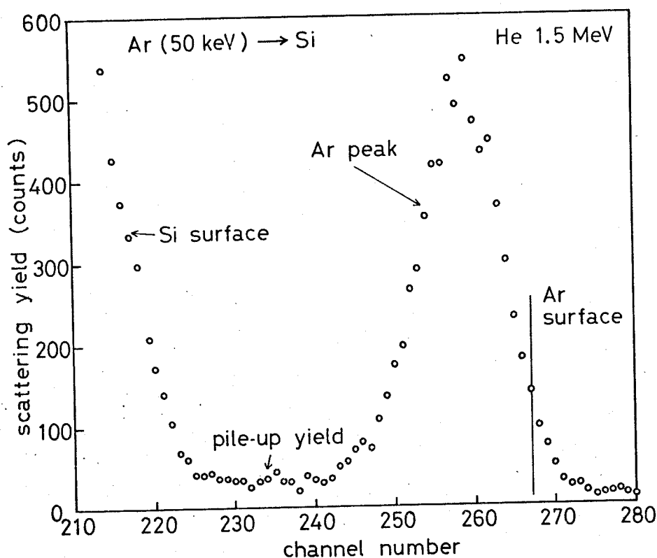
図 7-9 Si 基板中の 50 keV Ar イオン分布を測定した 後カ散乱スペクトル。
