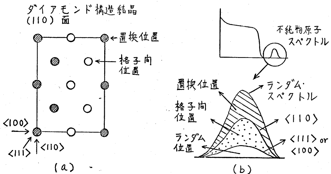
図8-2 後方散乱法による不純物原子位置の測定
