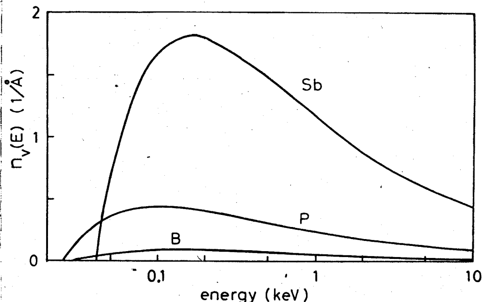
図6-1 F個のイオンによりSi基板中に作られる格子欠陥密度
