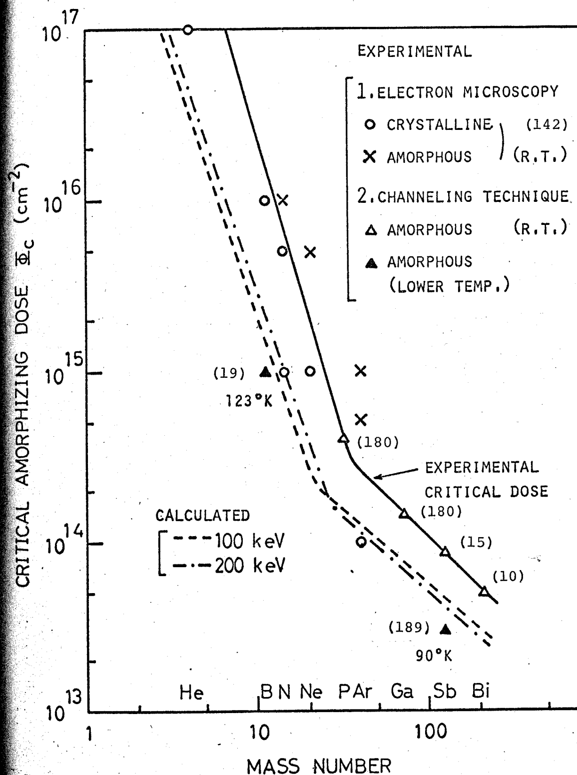
図 6-12 Si 基板が非晶質となる限界注入量 \Phi_c のイオン種依存性 図中の番号は参考文献を示している。
