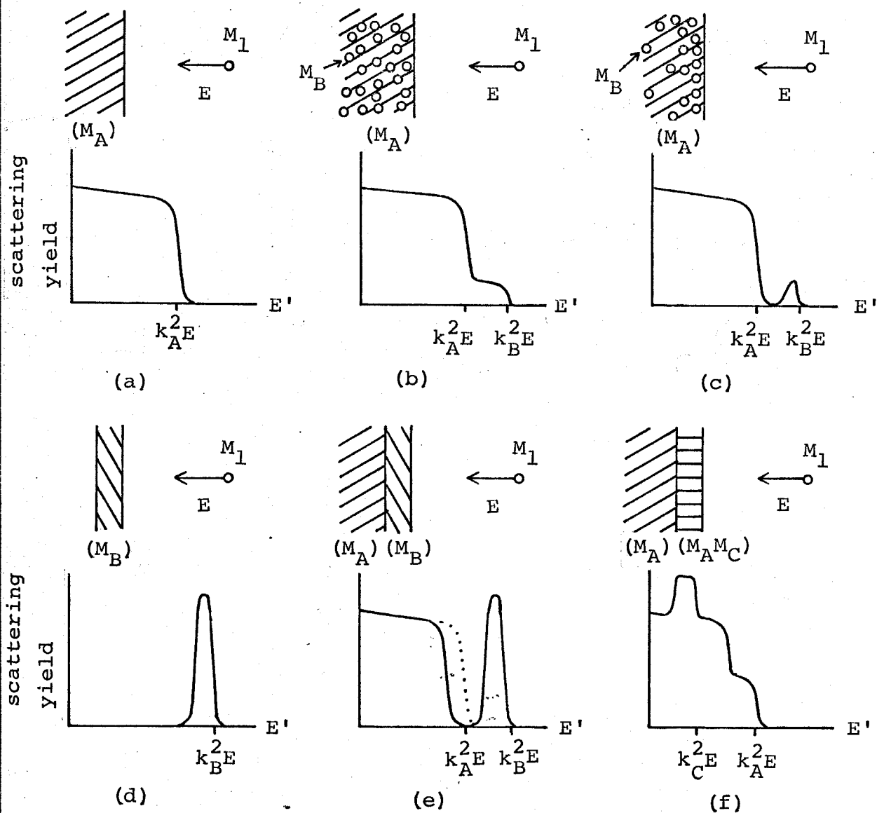
図 7-2 後方散乱法により測定できる基板の種類 および エネルギースペクトル
