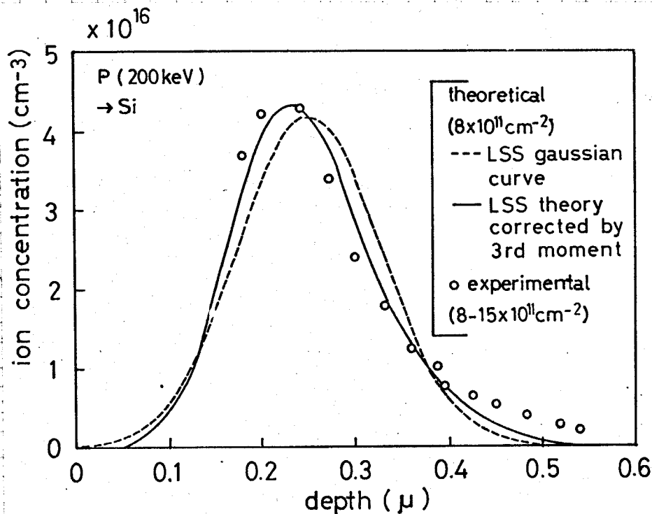
図 3-8 Si 中の P イオン濃度分布の理論値と実験値との比較。
