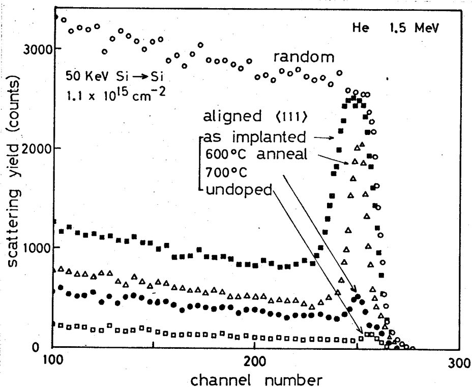
図 8-6 Si 打ち込み試料のアニール特性
