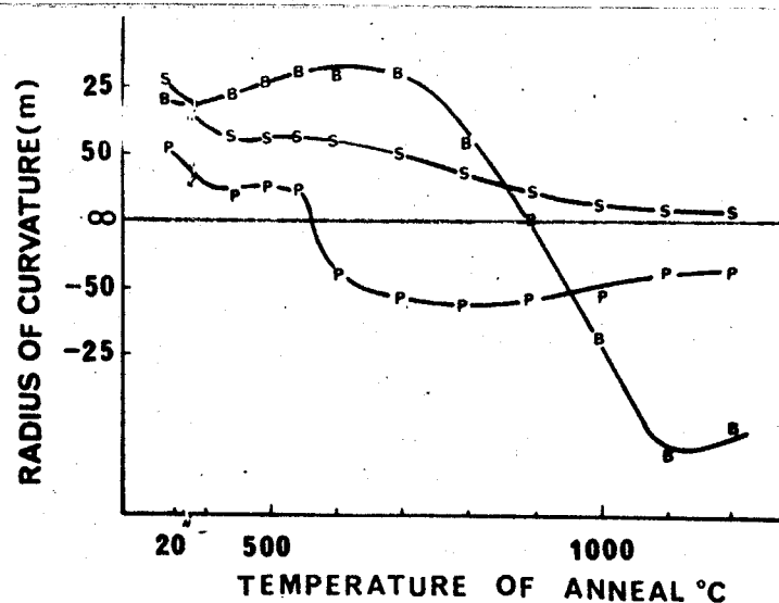
図 8-9 イオン注入層の歪の測定。B, S, P はそれぞれ B, Si, P 打込み試料を示す。
