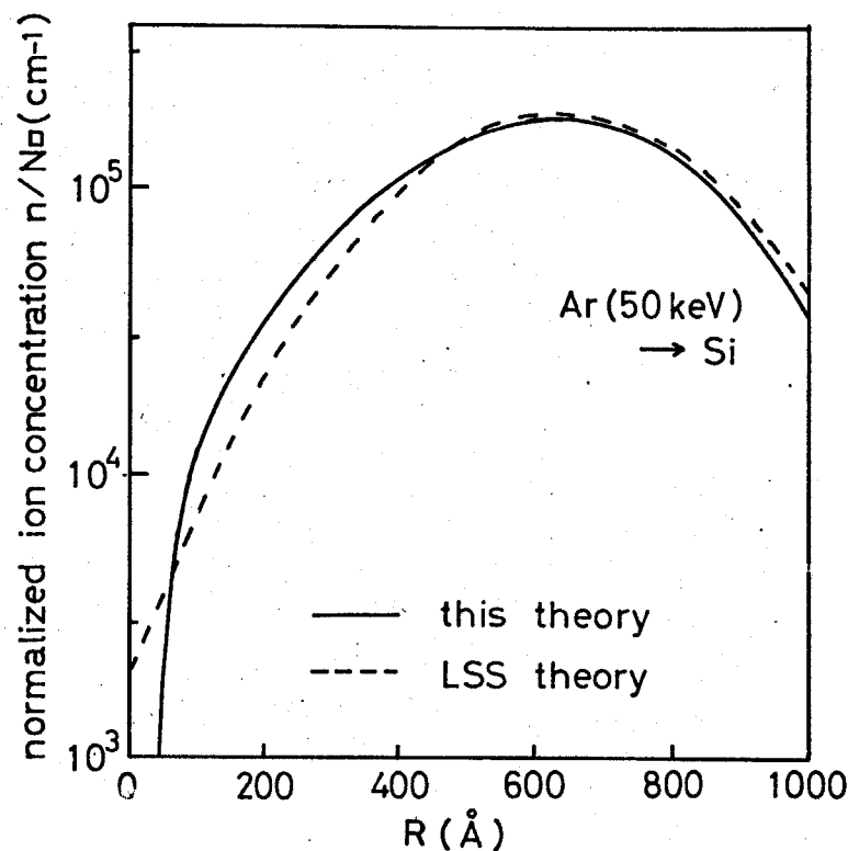
図 4-11 Thomas-Fermi ポテンシャルを用いて計算された Si 基板中の 50 keV、Ar イオンの飛程分布。(T-F pot.)
