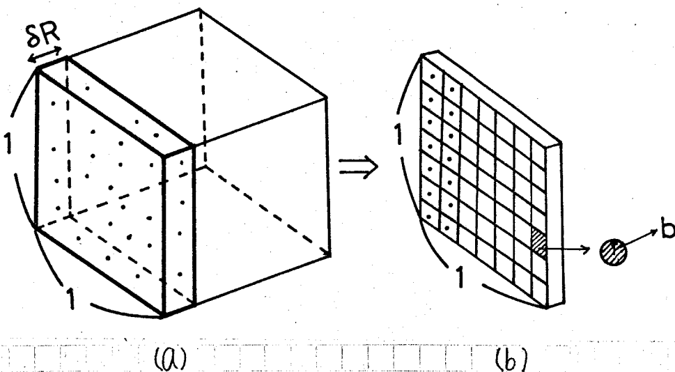
図 2-2 核阻止能 S_n(E) を求める概念図。
