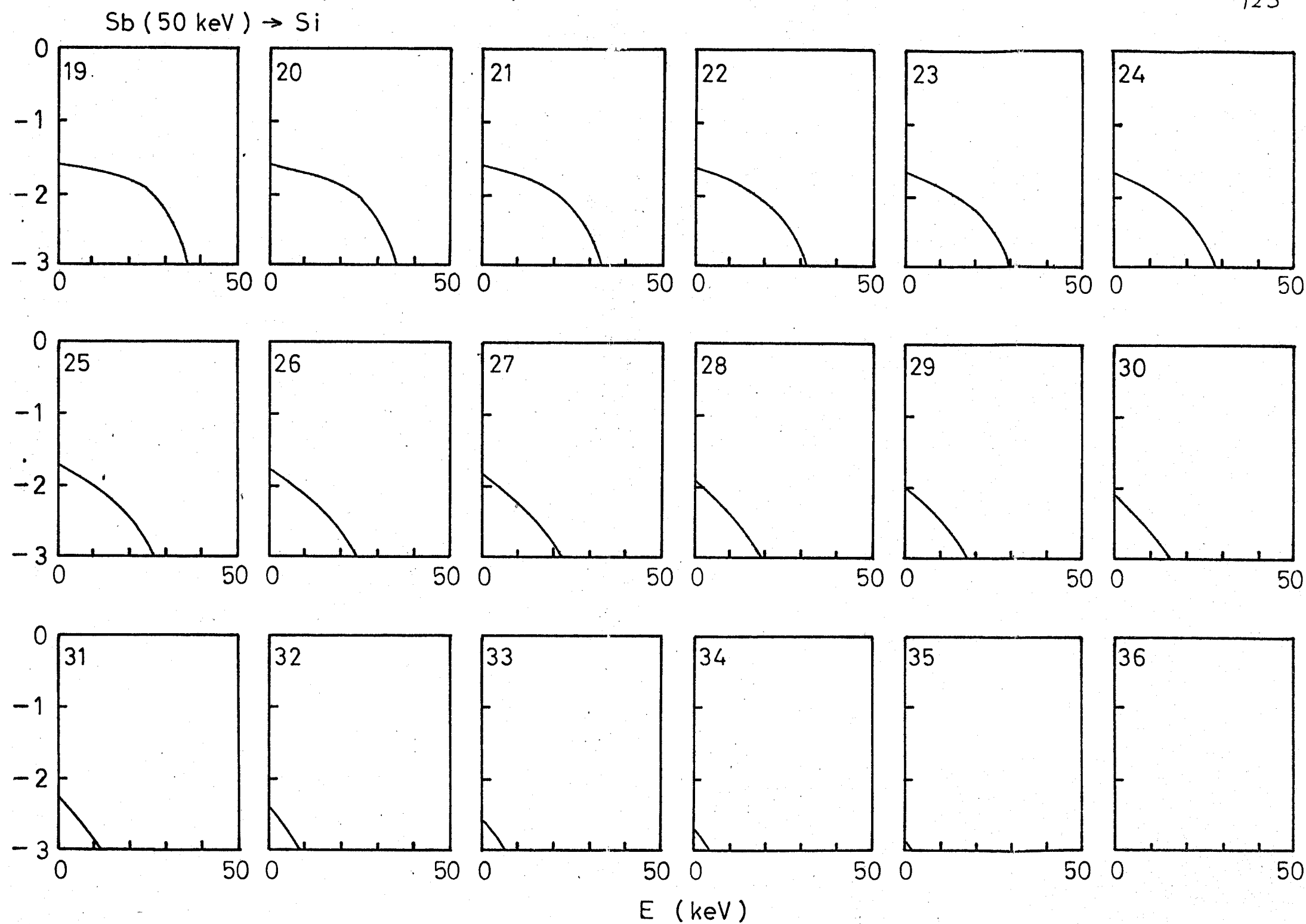
図 4-5 (b) Si 基板中の 50 keV Sb イオンのエネルギー分布 (II) ( r^{-2} pot.)
