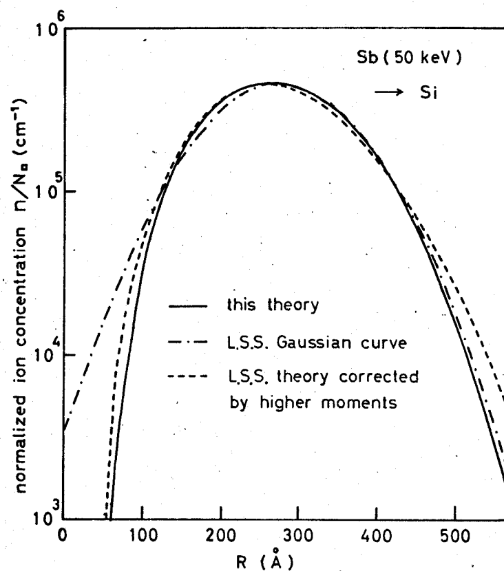
図4-9 高次モーメントを考慮したLSS理論と本解析法との比較。(50 keV, SbイオンをSiに注入した場合。) ( r^{-2} pot.)
