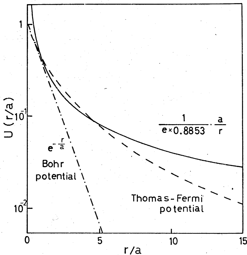
図 2-3 原子間の相互作用を表わす各種の遮蔽関数。
