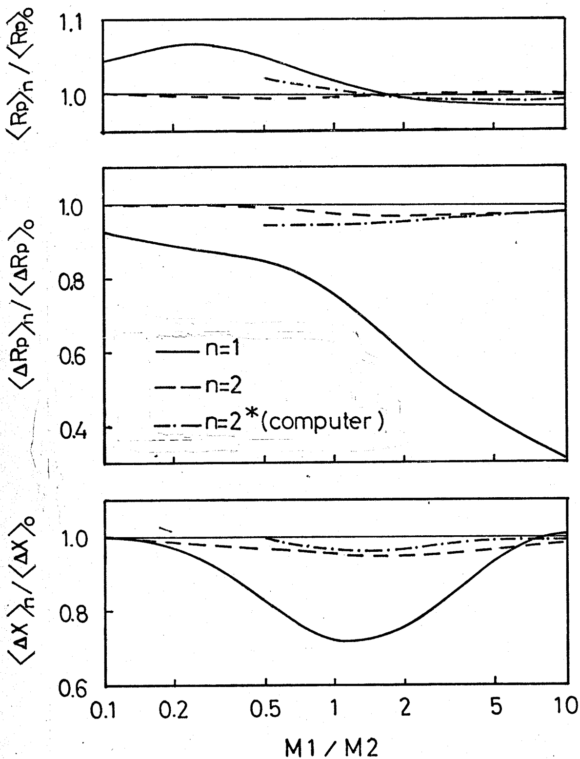
図3-4 平均射影半径、射影標準偏差、および横方向広がりに関する厳密解と、1階および2階微分方程式の解との比。(r -2 pot.)
