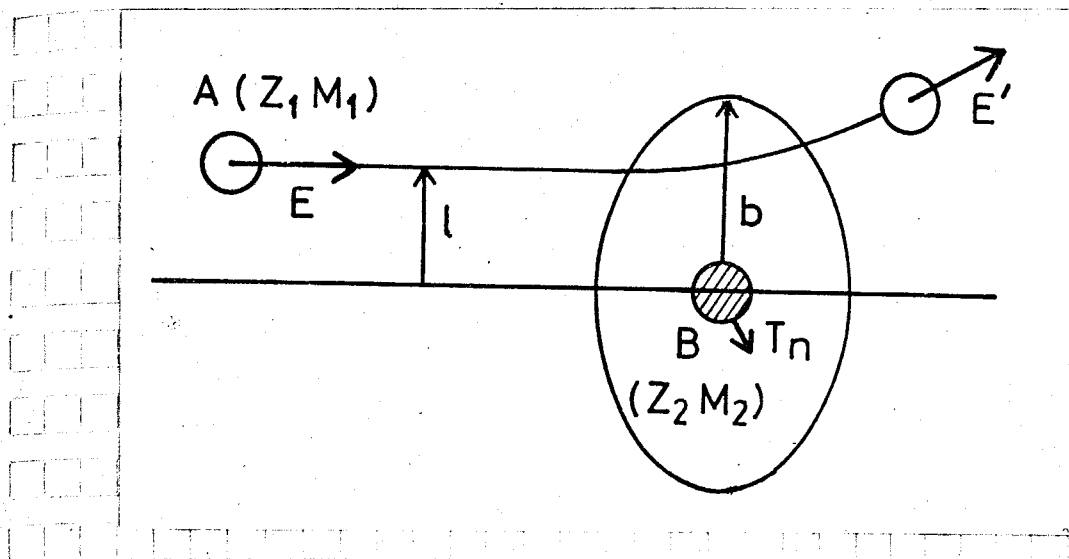
図4-3 入射イオン A と基板原子核 B との衝突。
