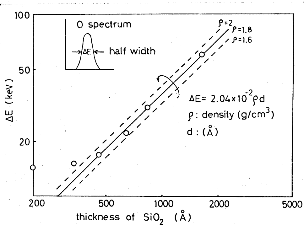
図 7-8 陽極酸化 \text{SiO}_2 の比重の測定。 \text{SiO}_2 中の He イオンのエネルギー損失の割合は、文献(106)を用いた。
