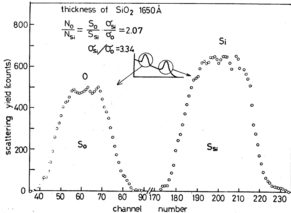
図 7-7 \text{SiO}_2 層からの後方散乱スペクトル
