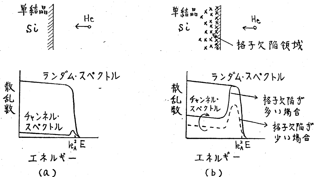
図8-1 完全結晶および格子欠陥の存在する結晶からの後方散乱スペクトル
