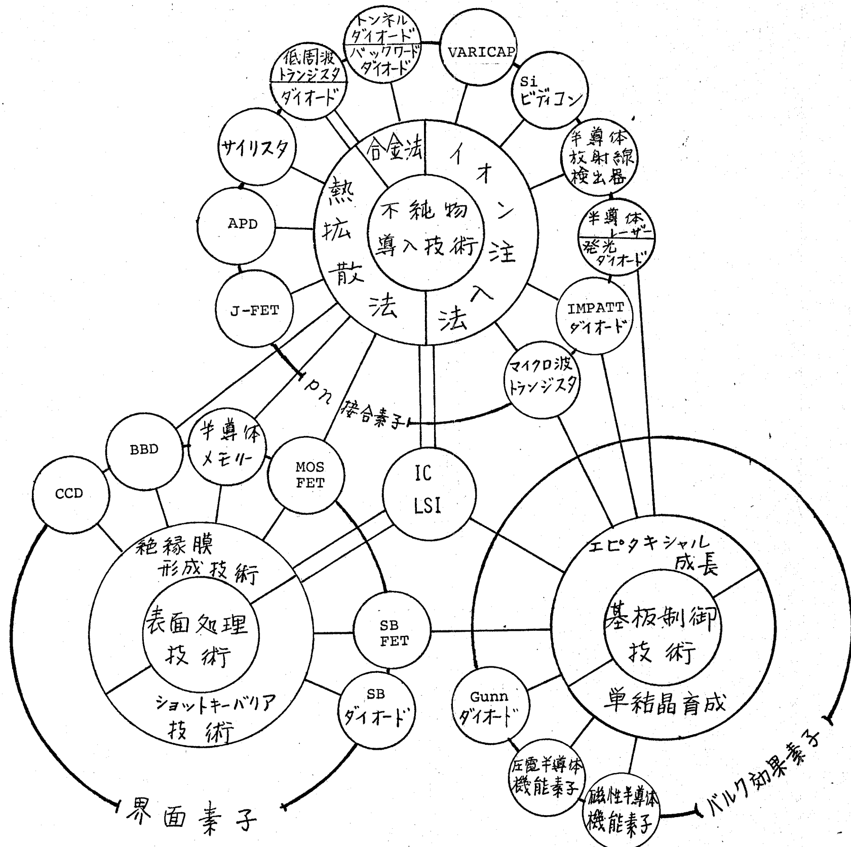
図 1-1 半導体素子製作技術の中でイオン注入法の占める位置
