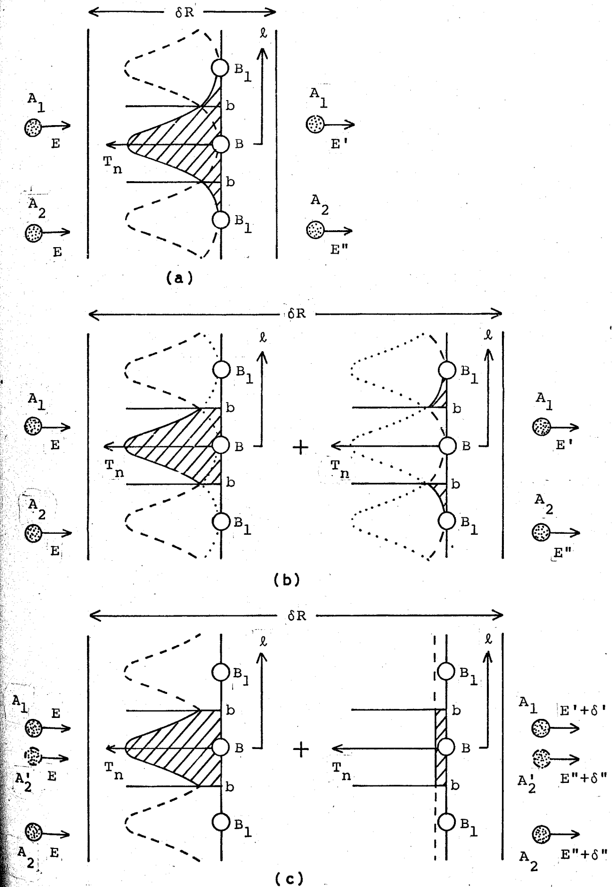
図4-2 薄層通過時イオンのエネルギー損失の導出
