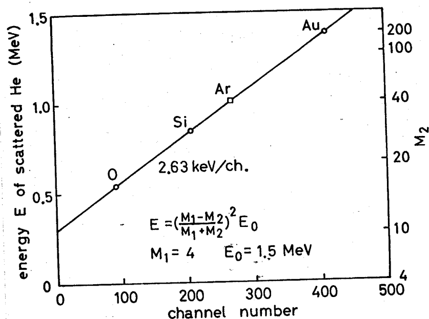
図 7-10 多重波高分析器チャンネル数の校正。 M_1 は He イオンの質量数, M_2 は測定対象物の元素の質量 数である。図中の式は, 180^\circ 後方散乱の場合である。
