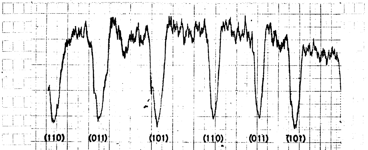
図 8-4 ゴニオメーターの回転による後方散乱数の変化。
