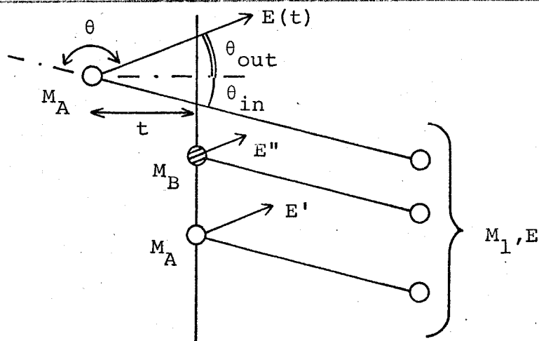
図 7-1 後方散乱法の原理
