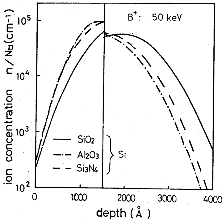
図5-7 \text{SiO}_2 , \text{Al}_2\text{O}_3 および \text{Si}_3\text{N}_4 層の付いた Si 基板中の 50 keV B^+ イオンの射影濃度分布 (T-F pot.)
