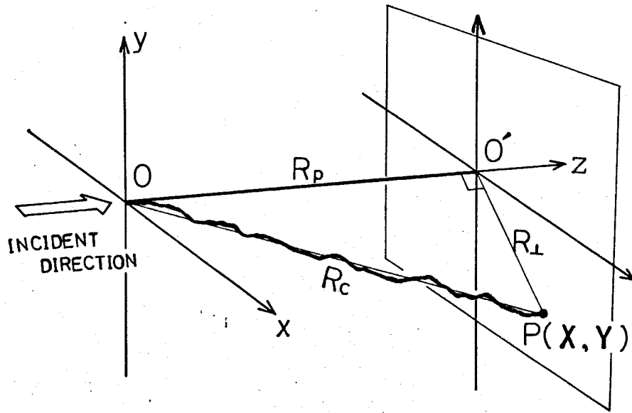
図 2-8 飛程に関する諸量の定義。
