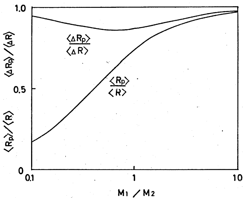
図3-2 平均値および標準偏差に関する 飛程と射影飛程の比 ( r^{-2} pot.) *
