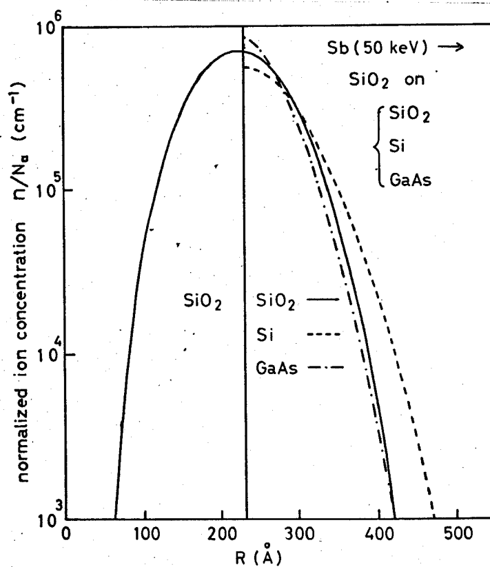
図5-2 SiO 2 -Si基板 および、SiO 2 -GaAs基板 中の 50 keV、Sbイオンの 飛程分布。(SiO 2 の厚み 230 Å.) (r -2 pot.)
