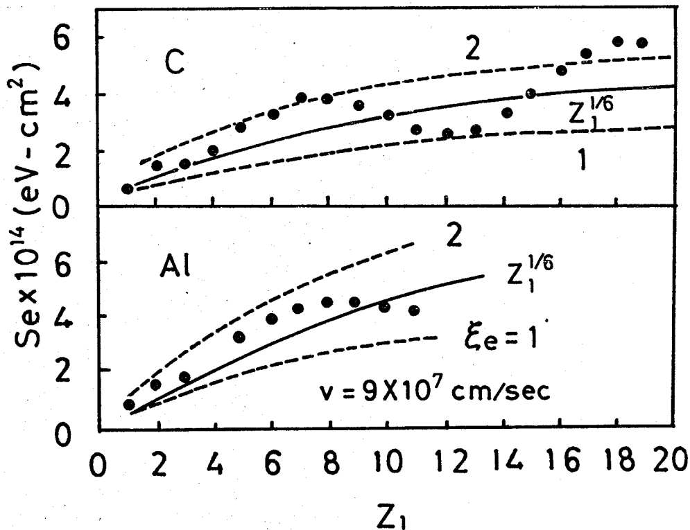
図2-6 電子阻止能の注入イオン原子番号 Z_1 への依存性。 (112)
