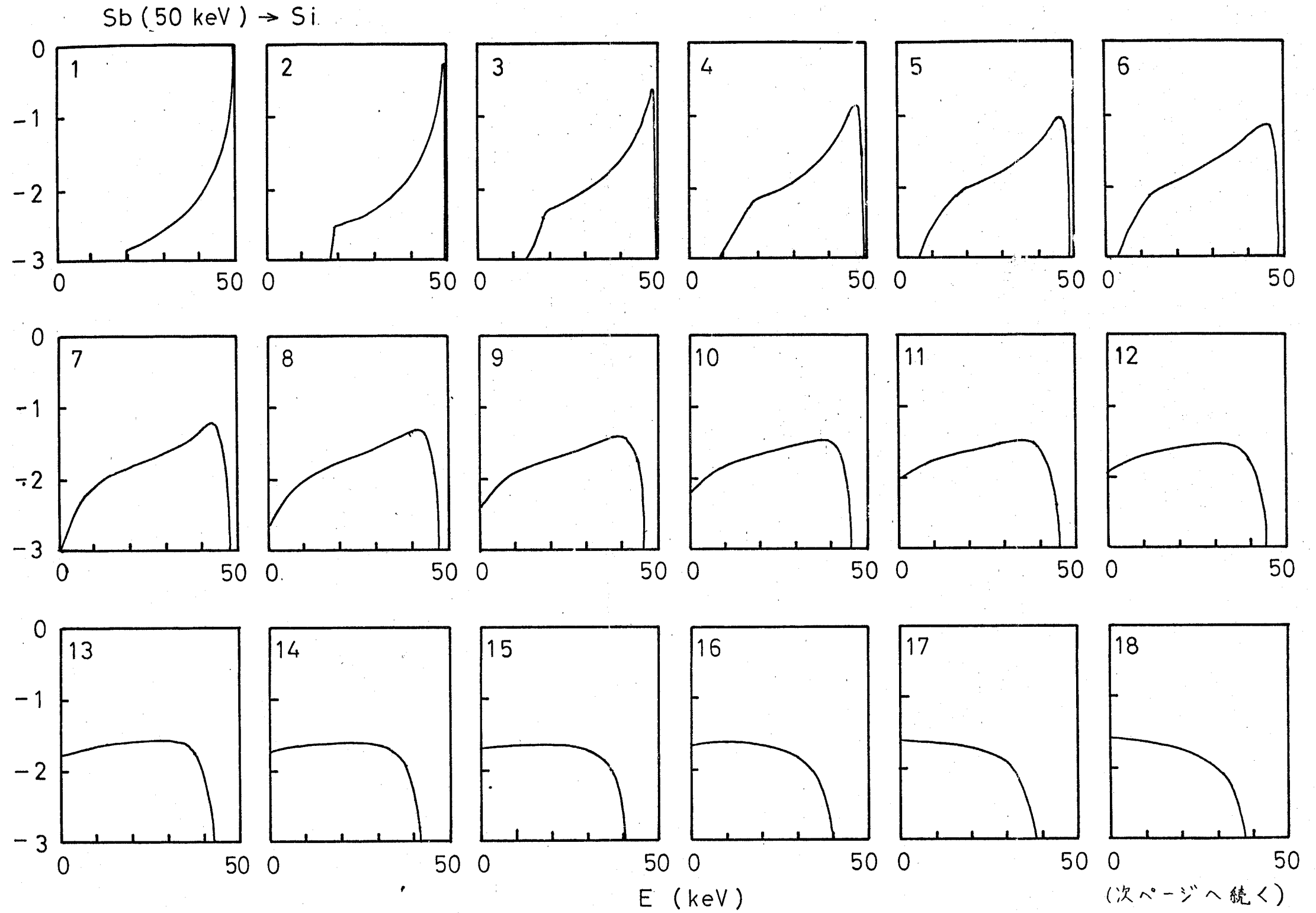
図 4-5(a) Si 基板中の 50 keV Sb イオンのエネルギー分布 (I) ( r^{-2} pot.)
