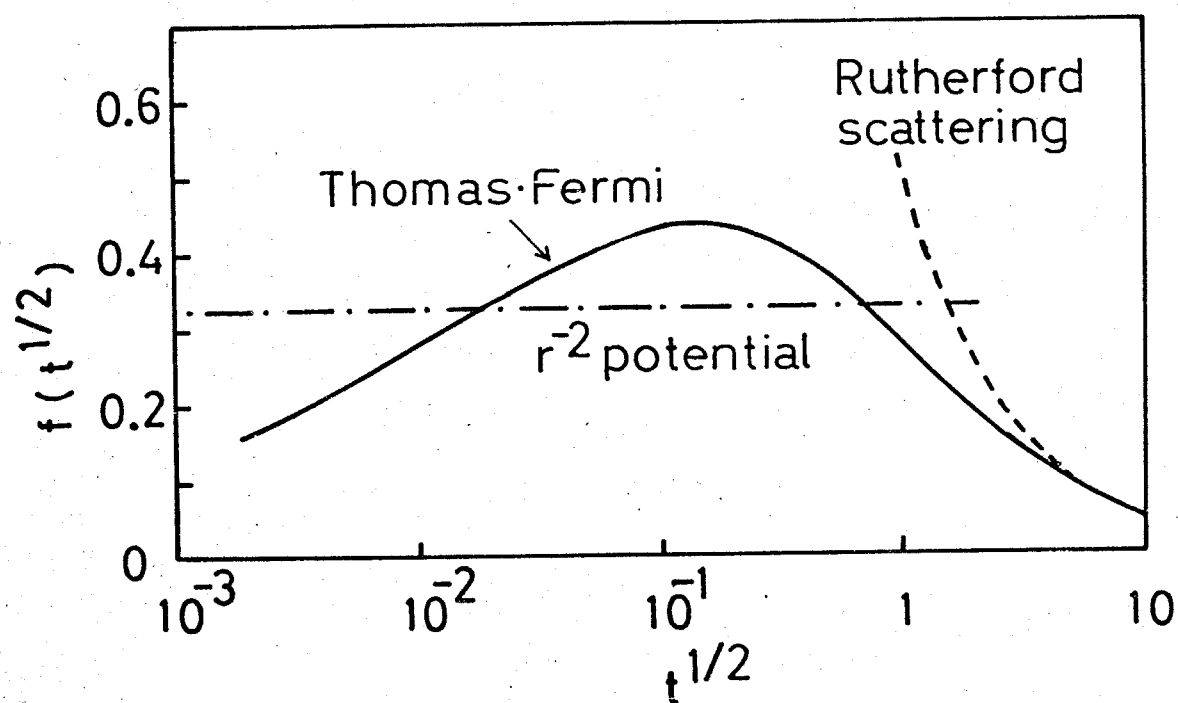
図2-4 各種遮蔽関数に対する f の値.
