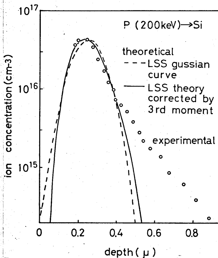
図3-10 Si中のPイオンの尾に及ぶ理論値と実験値との比較。実験結果はMoline (154) による。 (T-Fpot. + r^{-2} pot.)
