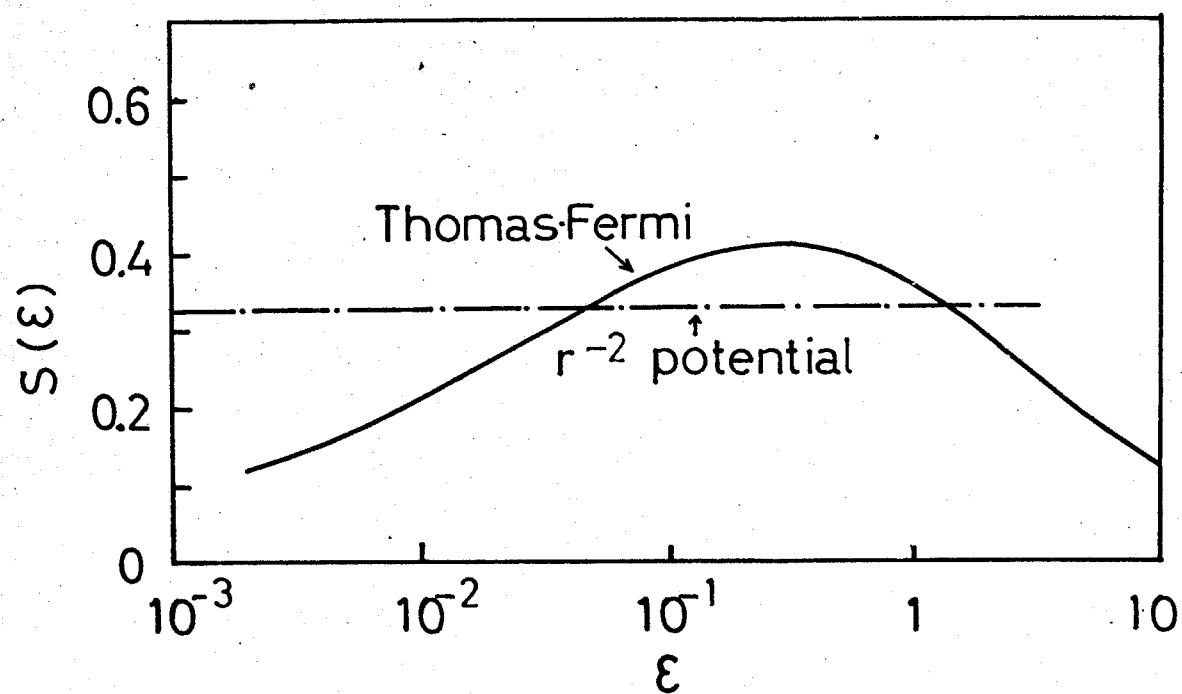
図2-5 核阻止能のエネルギー依存性.
