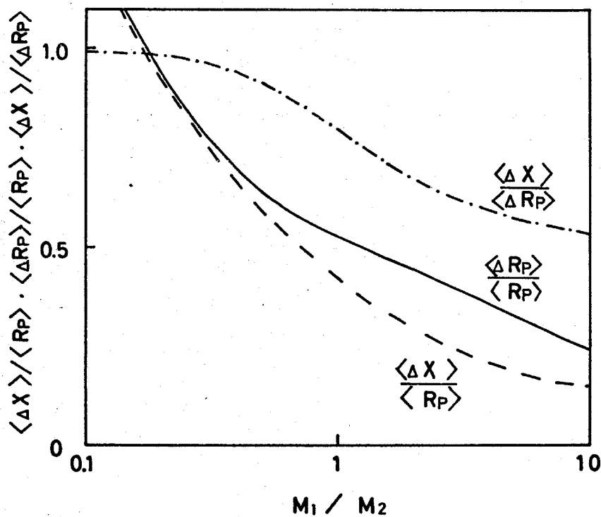
図3-3 射影飛程 分布に関する諸量 の関係 ( r^{-2} pot.) *
