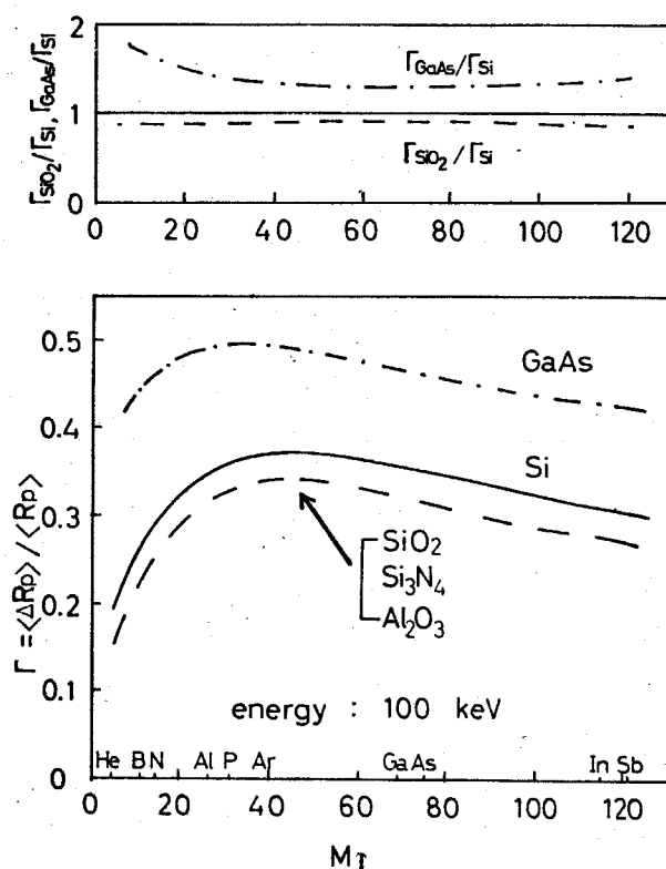
図 5-6 各種基板中における \langle \Delta R_p \rangle と \langle R_p \rangle の比。(打ち込みエネルギー 100 keV) (T-F pot.)
