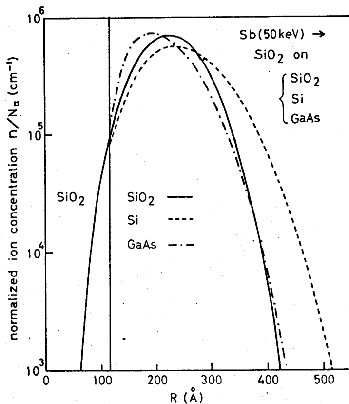
図5-1 SiO 2 -Si基板 および、SiO 2 -GaAs基板 中の 50 keV、Sbイオンの 飛程分布。(SiO 2 の厚み 115 Å.) (r -2 pot.)
