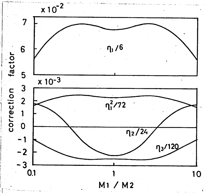
図3-5 Edgeworth の漸進形における補正項係数のイオン質量による変化 (r -2 pot.)
