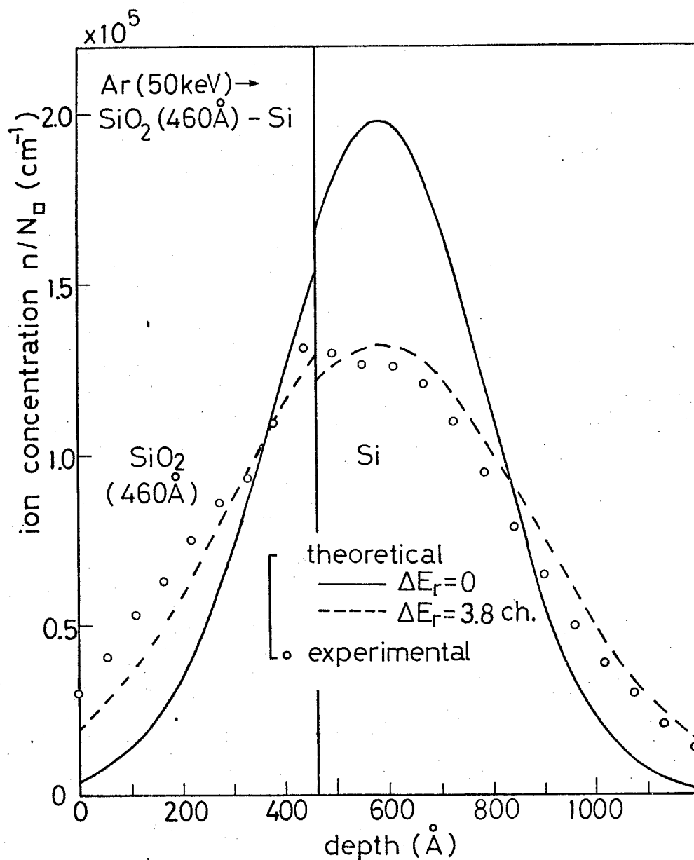
図 7-14 SiO 2 (460 Å) - Si 基板中の Ar イオン分布。
