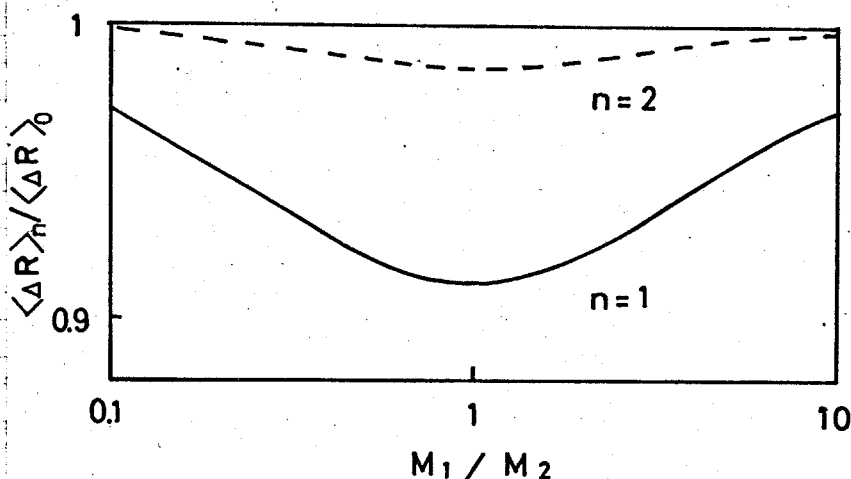
図3-1 1階および2階微分方程式の解と厳密解との比較。(飛程分布の標準偏差。) 図中の \langle \Delta R \rangle は \sqrt{\langle \Delta R^2 \rangle} を示している。(r -2 pot.)*
