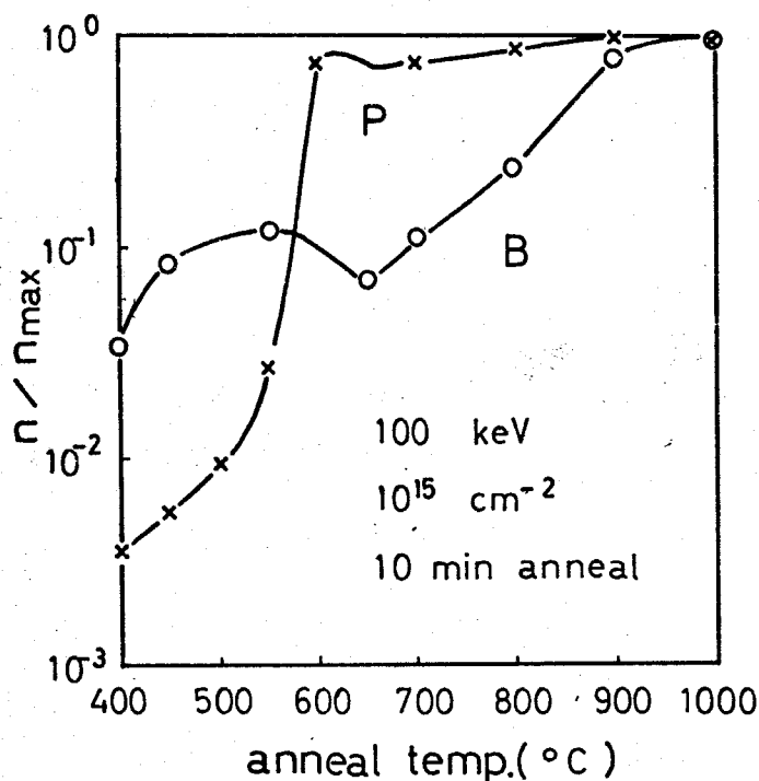
図2-12 Si基板中のBおよびPイオンの等時アニール特性。
