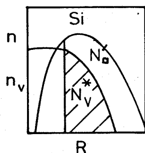
図 6-11 \text{Si} 中にできる格子欠陥数の \text{SiO}_2 膜厚による変化 ( r^{-2} pot.)
