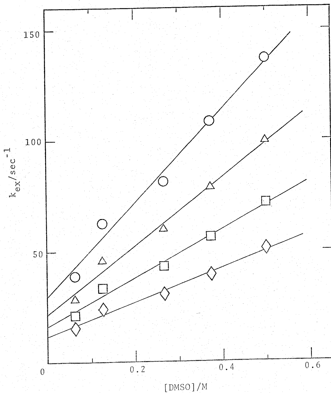
Fig. 16. Plots of k_{\text{ex}} vs. [\text{DMSO}] for the exchange of DMSO in \text{UO}_2(\text{dbm})_2\text{DMSO} in \text{CD}_2\text{Cl}_2 . ○ : -10\text{ }^{\circ}\text{C} ; △ : -15\text{ }^{\circ}\text{C} ; □ : -20\text{ }^{\circ}\text{C} ; ◇ : -25\text{ }^{\circ}\text{C} .
