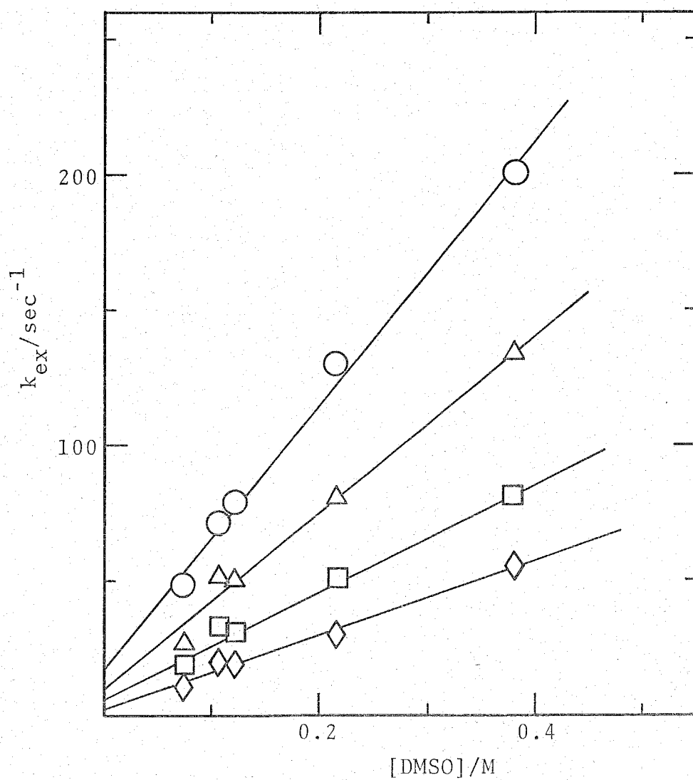
Fig. 11. Plots of k_{\text{ex}} vs. [\text{DMSO}] for the exchange of DMSO in \text{UO}_2(\text{DMSO})_5^{2+} . ○ : -35\text{ }^{\circ}\text{C} ; △ : -40\text{ }^{\circ}\text{C} ; □ : -45\text{ }^{\circ}\text{C} ; ◇ : -50\text{ }^{\circ}\text{C} .
