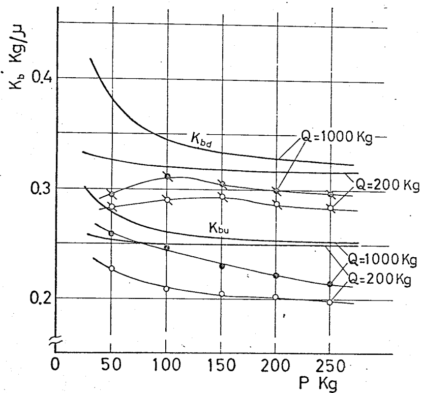
図5-23 多数ボルト締結時の曲げ荷重依存性の理論値と実験値の比較 d=M12, s_{ul}=30\text{ mm}, s_{ul}=60\text{ mm}, L_e=305\text{ mm}
