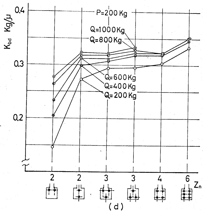
図 2-50 曲げ静剛性に及ぼす締結ボルト本数の効果
