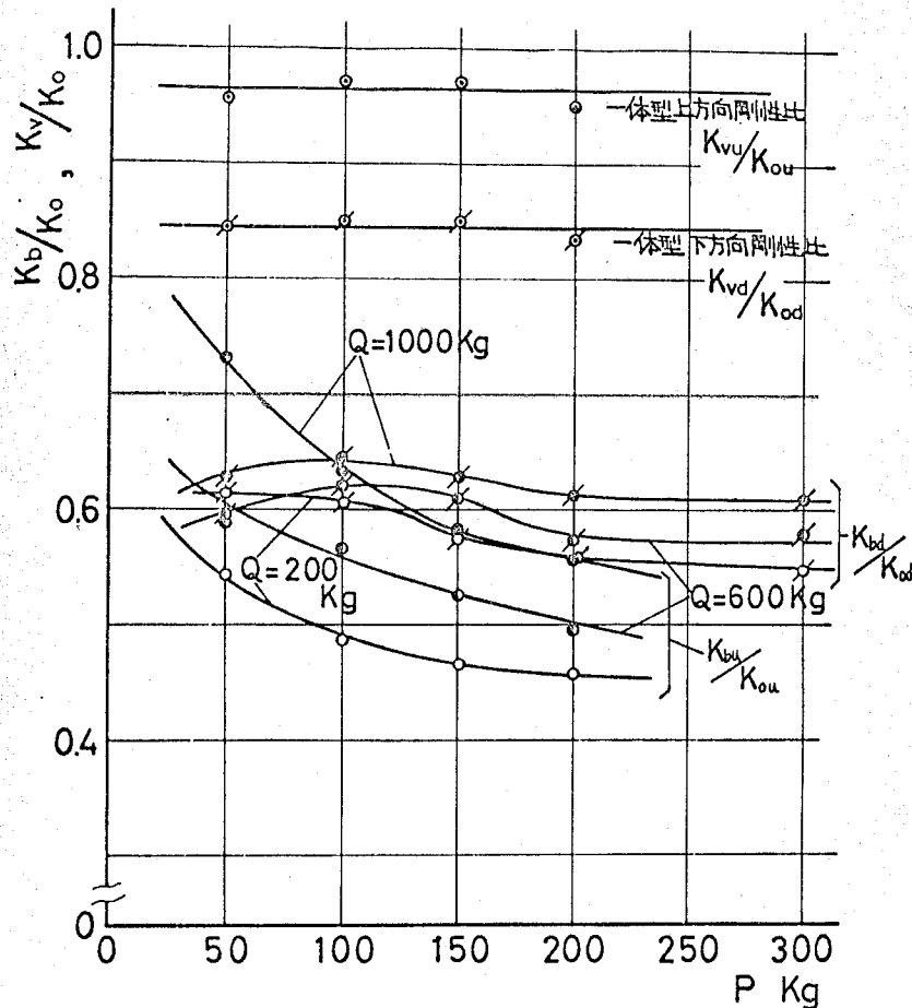
図 2-16 一体形とボルト締結の曲げ静剛性の比較
