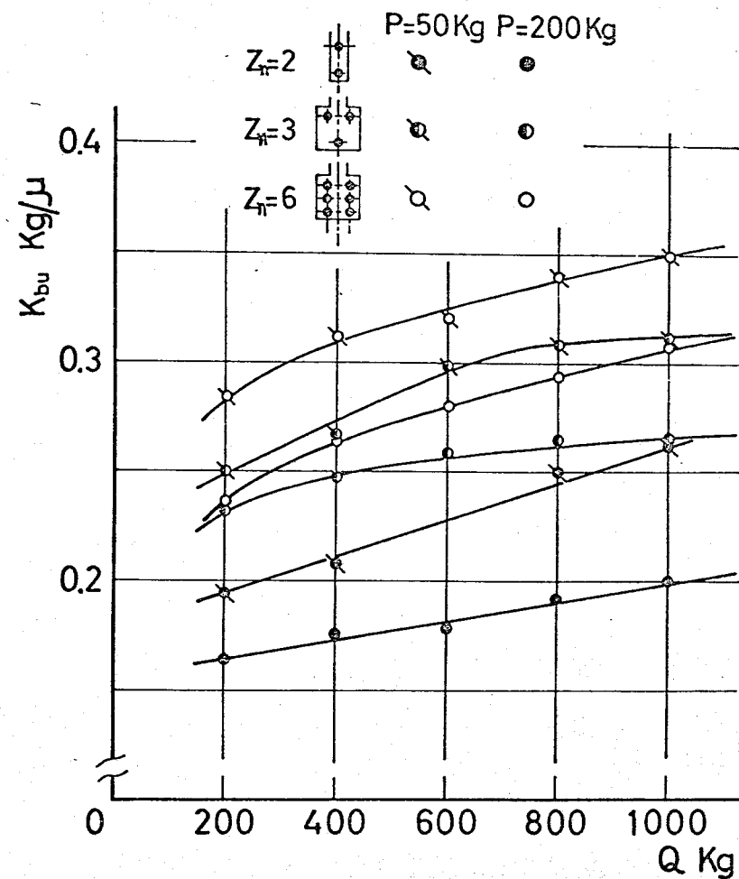
図 2-54 多数ボルト締結に於ける曲げ静剛性の 締結力依存性
