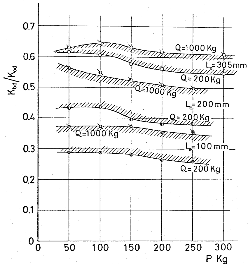
図 2-23 突出し長さによる下方向剛性比の変化 d=M12, s_a=60\text{mm}, b=40\text{mm}, h=40\text{mm}
