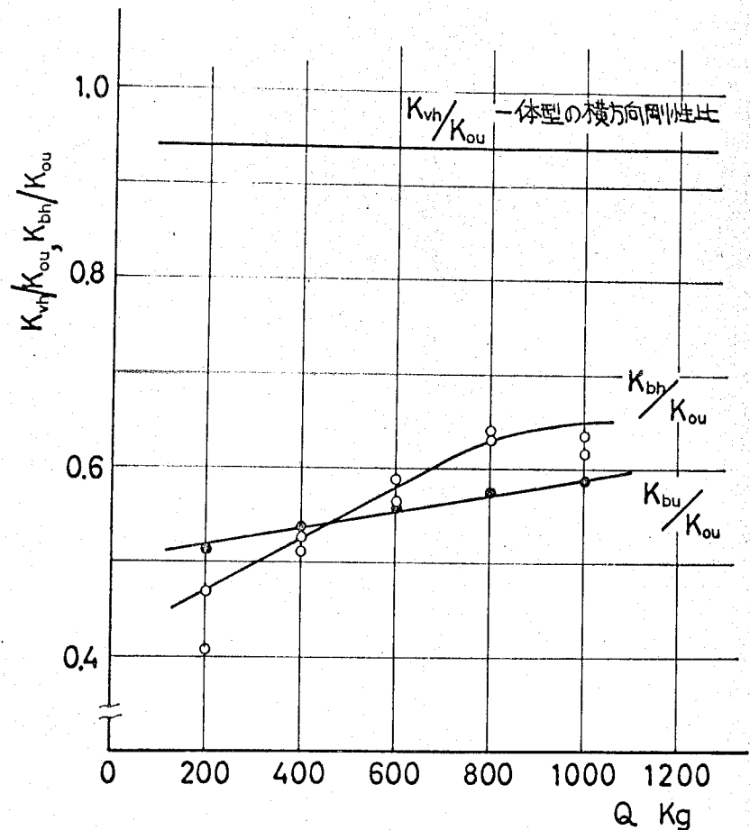
図2-37 一体型とボルト締結梁の横剛性値の比較 d=M12, s_a=60mm, h=40mm, b=40mm, L_e=305mm
