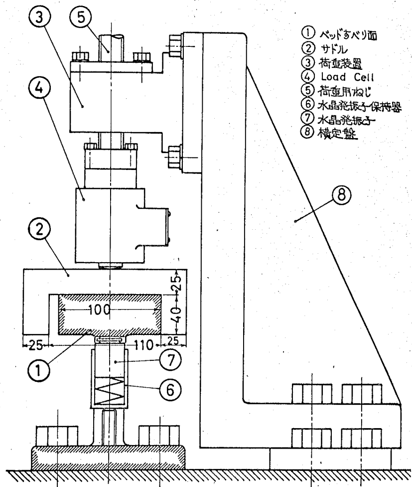
図3-5 実験装置概略図
