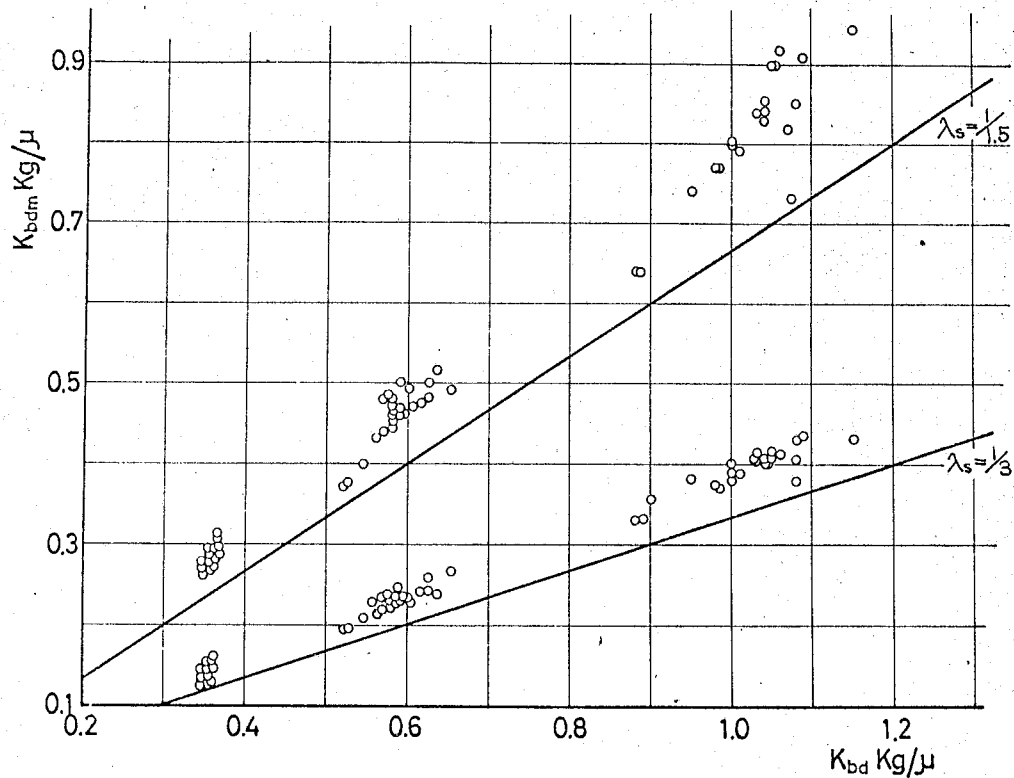
図6-4 模型則の理論値と実験値の比較（下方向曲げ静剛性）
