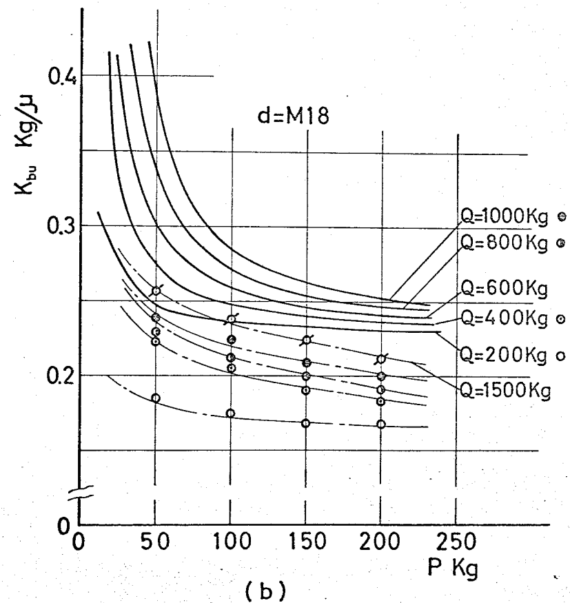
図5-30 締結ボルト径を変えたときの曲げ荷重依存性(1)
