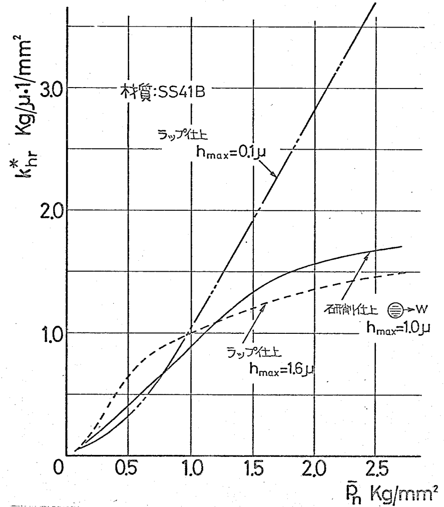
図 4-7 横方向接触剛性に及ぼす平均接触面圧力の影響
