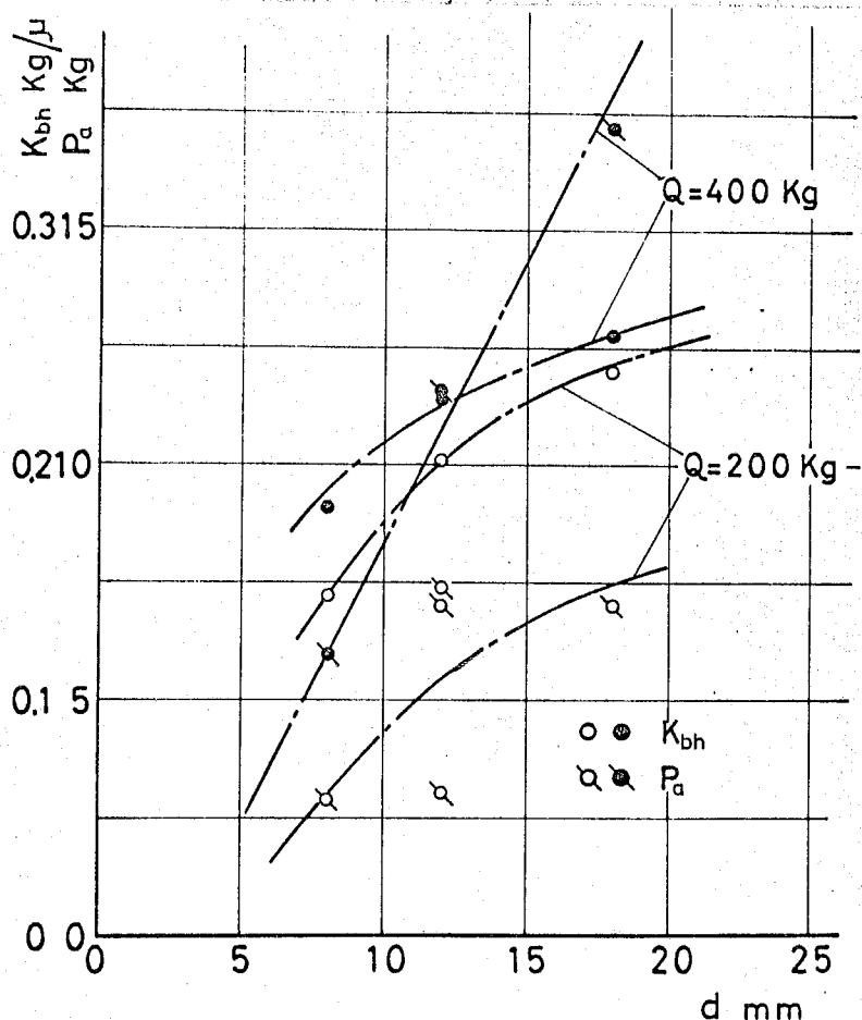
図 2-40 横曲げ静剛性に及ぼす締結ボルト径の影響 s_a=40\text{mm} , h=40\text{mm} , b=40\text{mm} , L_e=305\text{mm}
