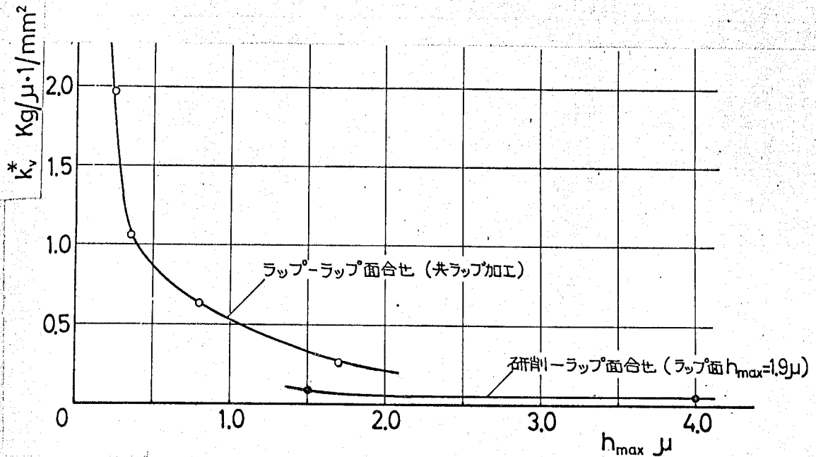
図3-18 床の弾性係数に及ぼす表面粗さの影響(材質FC25)
