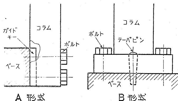
図 1-2 ボルト結合部の種類
