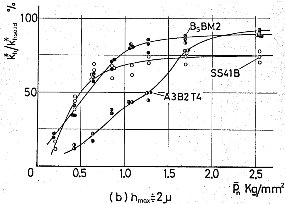
図 4-19 横方向接触剛性に及ぼす材質の影響 (研削仕上面, \odot \rightarrow W )
