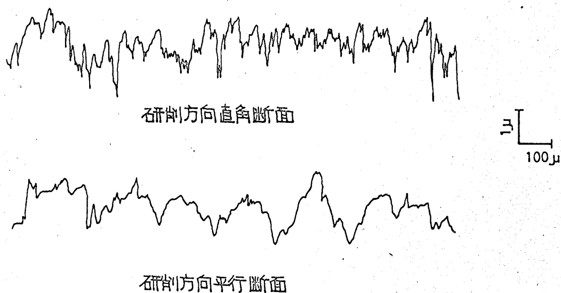
図4-13 研削仕上面の表面粗さ形状
