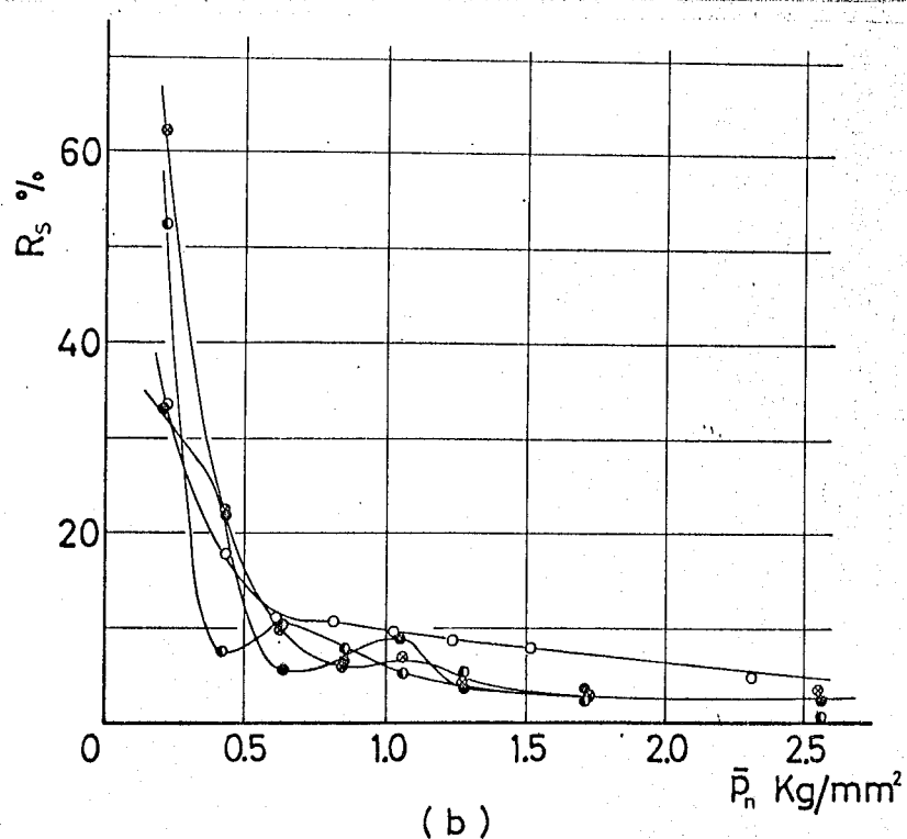
図 4-14 横方向接触剛性とすべり変位率に及ぼす研削方向の影響 (材質: SS41B, 研削仕上)
