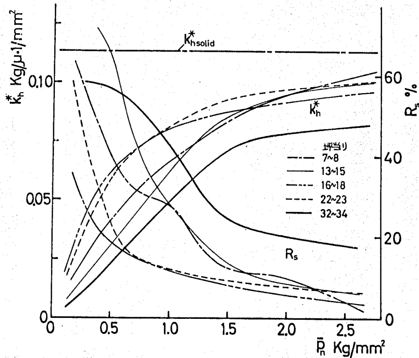
図4-18 きさげ仕上面の坪当りが横方向接触剛性および変位率に及ぼす影響(材質:FC25)
