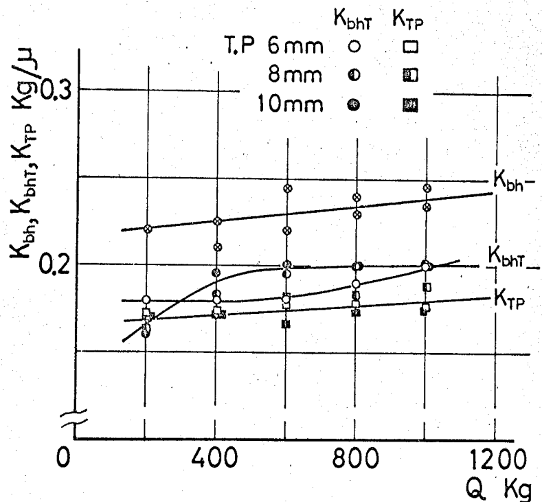
図2-45 横曲げ静剛性に及ぼすテーパピンの効果 (締結条件, テーパピンの位置は図2-43と同じ)
