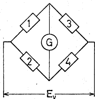
図 2-3 ボルト締付力測定用ブリッジ回路
