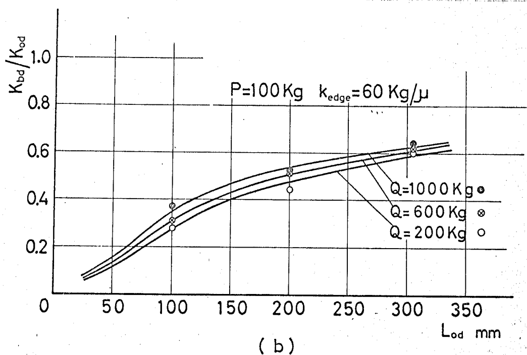
図5-33 突出し長さによる曲げ剛性比の変化 d=M12 , s_a=60\text{mm} , b=40\text{mm} , h=40\text{mm}
