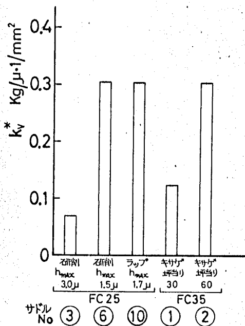
図3-15 床の弾性係数の測定値 (ベッドすべり面 No2: キサゲ仕上面)
