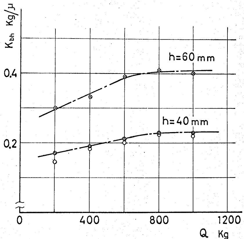
図 2-42 梁の厚さによる横剛性値の変化 d=M12 , s_a=60 mm, b=40 mm, L_e=305 mm
