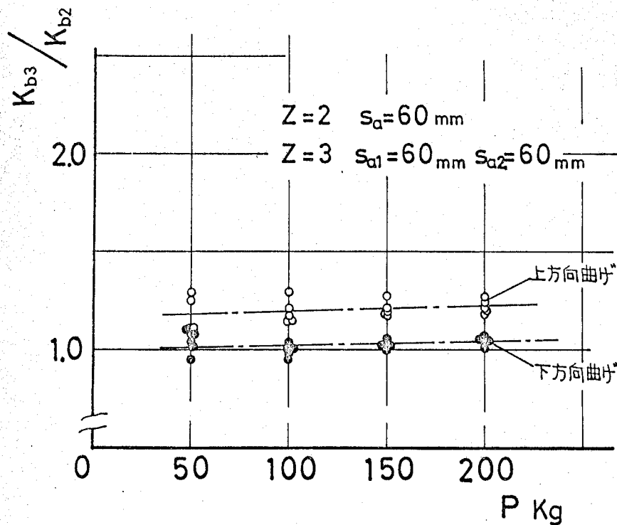
図 2-52 結合部面積が変化するときの中固ボルトの効果
