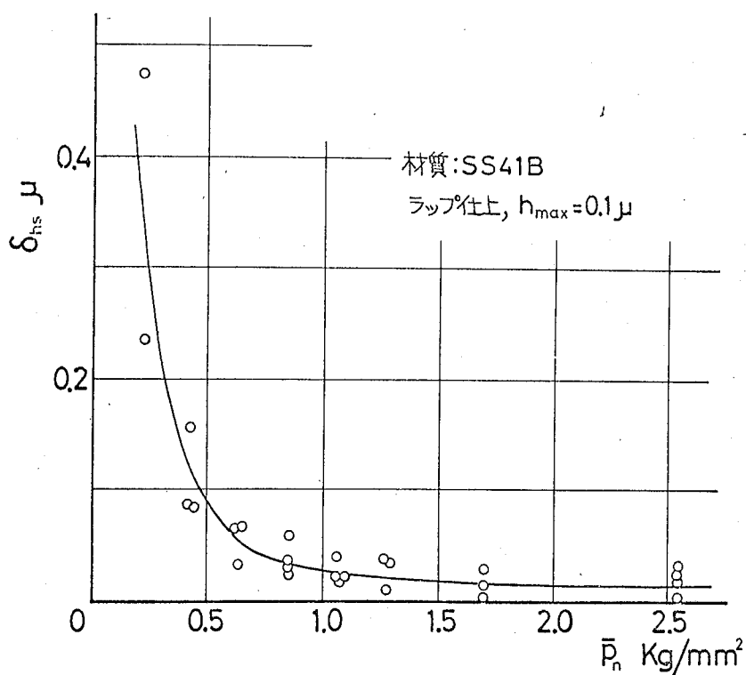
図4-9 すべり変位と平均接触面圧力の関係
