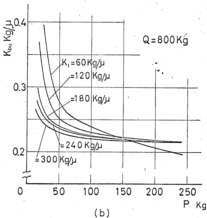
図5-21 Base edge部, Base部の等価ばね定数の曲げ静剛性に及ぼす影響 d=M12, s_a=60 \text{ mm}, b=h=40 \text{ mm}, L_e=305 \text{ mm}
