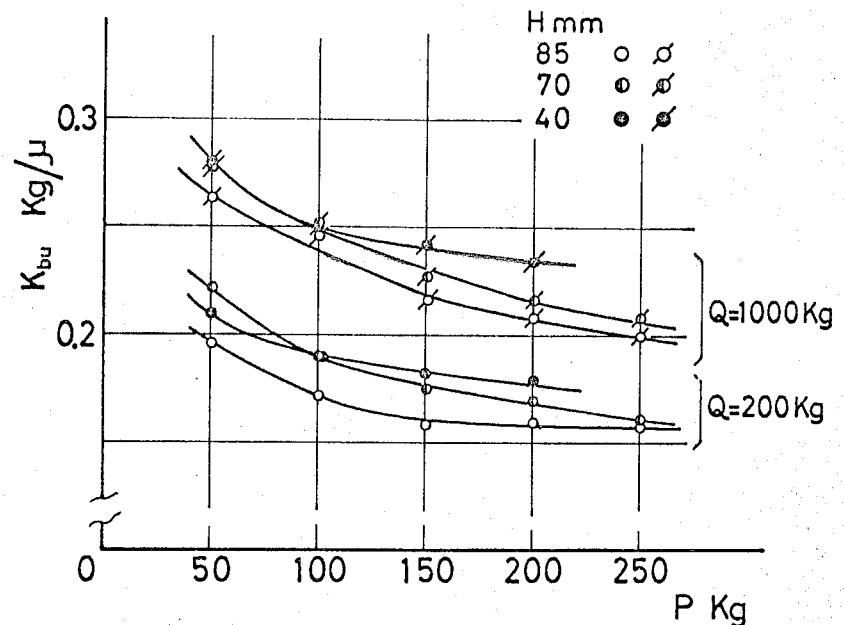
図 2-26 上方向曲げ静剛性に及ぼすベースの厚さの影響 d=M12 , s_a=60\text{mm} , b=h=40\text{mm} , L_e=305\text{mm}
