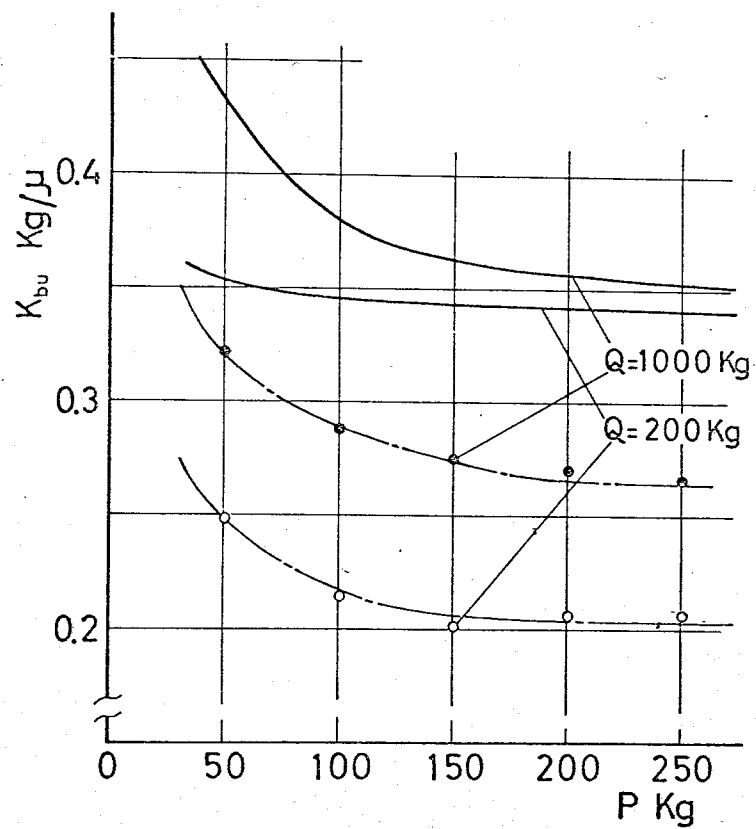
図 5-25 多数ボルト締結時の曲げ荷重依存性の理論値と実験値の比較 d=M12
