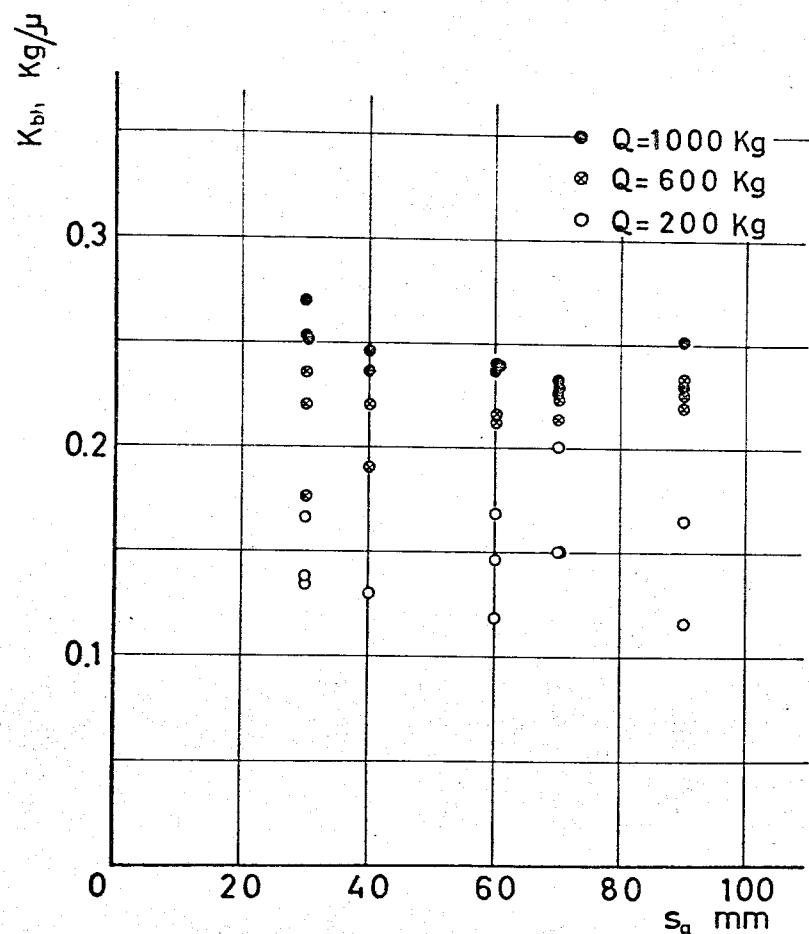
図 2-38 ボルト締付間隔による横剛性値の変化 d=M12 , h=40 mm, b=40 mm, L_e=305 mm
