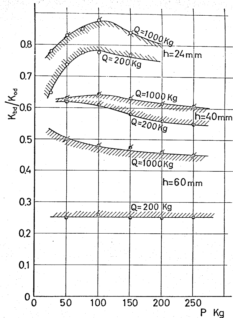
図 2-24 下方向曲げ剛性比の梁の厚さによる変化 d=M12, s_a=60\text{mm}, b=40\text{mm}, L_e=305\text{mm}
