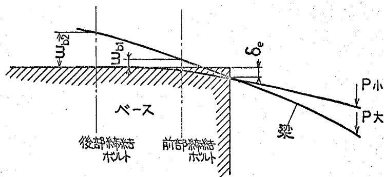
図 2-12 梁のベース部に於ける変形状態の模型図
