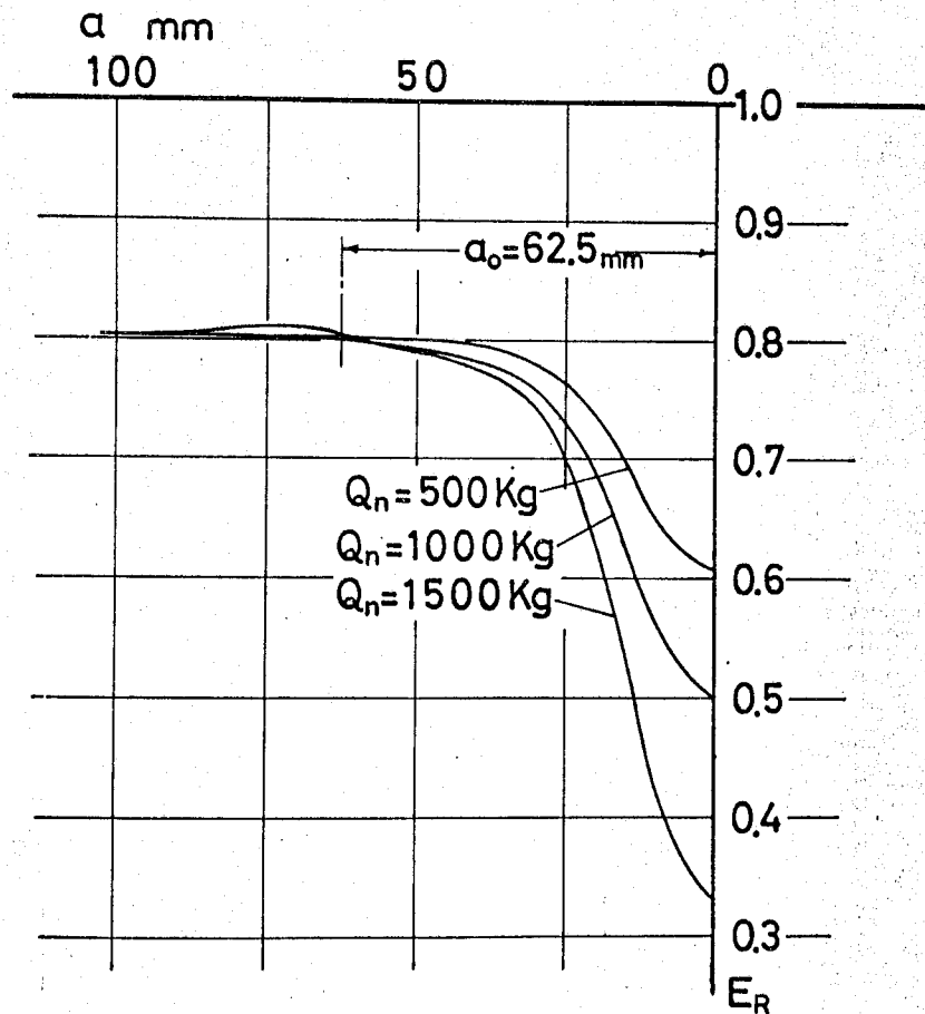
図3-12 補正した反射波高比分布
