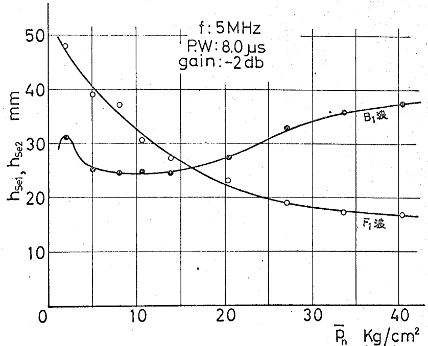
附図-8 F_1 波高 h_{se1} , B_1 波高 h_{se2} の特性 (Test piece: No.2)
