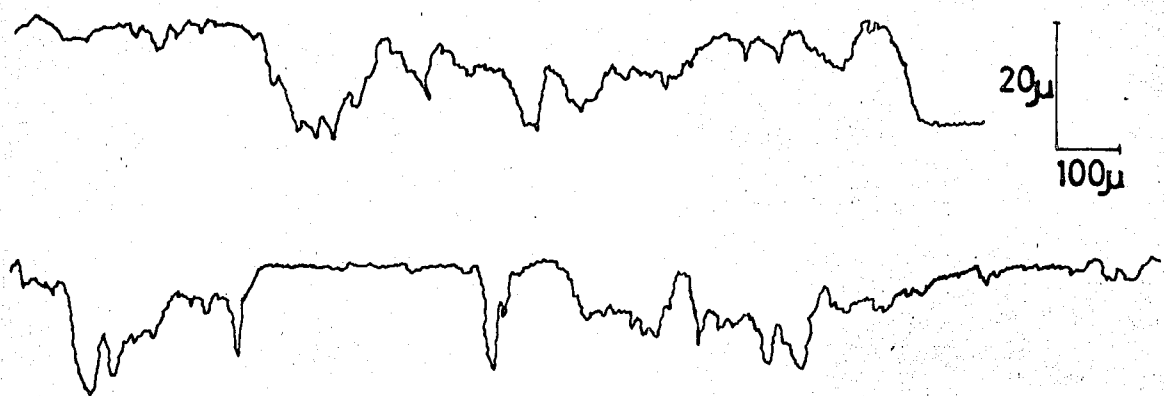
図4-21 きさげ仕上面の表面状態
