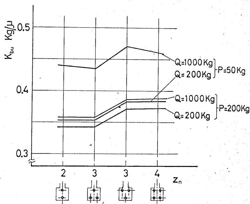
図5-27 締結ボルト本数の効果(計算値)
