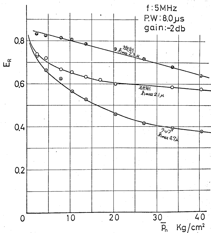
附図-16 表面粗さと反射波高比の関係 (Test piece: No.2, 但し上部試験片の粗さは図示のとおり)
