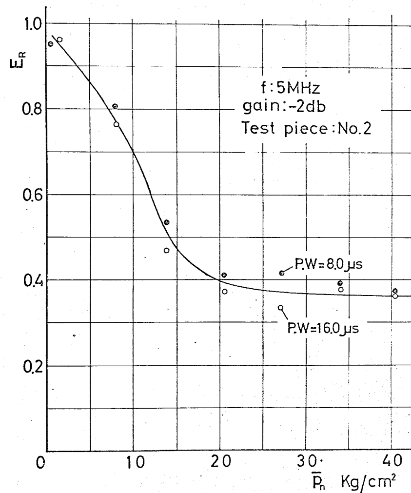
附図-12 送信パルス幅の反射波高比に及ぼす影響
