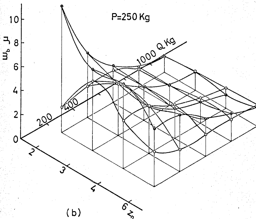
図 2-51 上方向曲げに於ける締結ボルトの伸び
