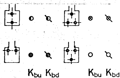
図 2-49 締結ボルトの位置と曲げ静剛性の関係
