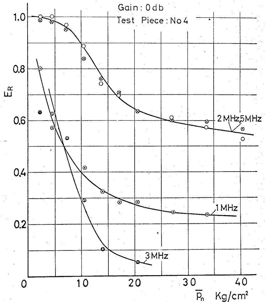
附図-13 発振周波数による反射波高比の変化
