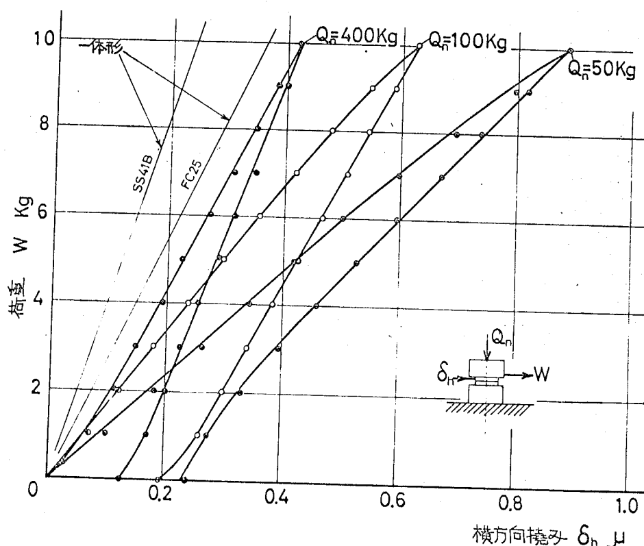
図4-4 横方向変位の測定例 (材質:SS41B, 研削仕上げ, 研削方向平行合せ (●))
