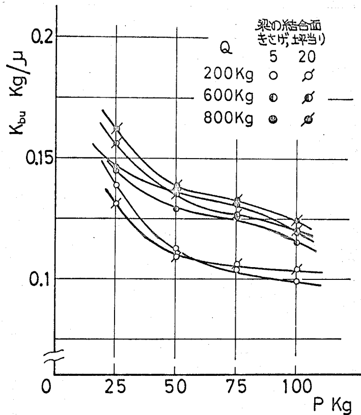
図 2-30 上方向曲げ静剛性に及ぼすきざげ仕上面の坪当りの影響
