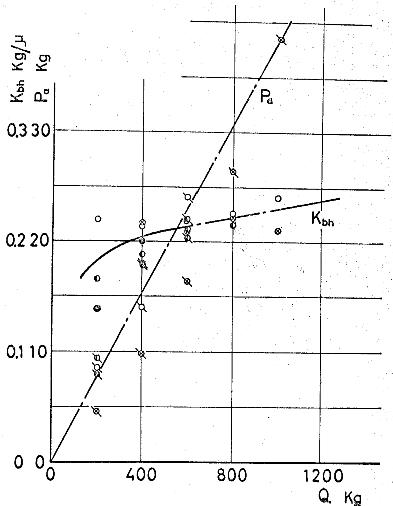
図 2-35 横曲げ静剛性の締付力依存性
