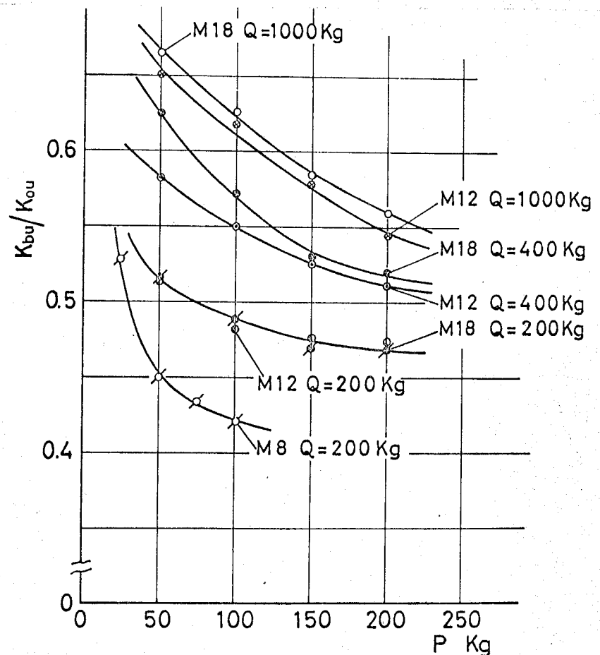
図 2-20 締付力，ボルト径による上方向曲げ剛性比の変化 s_d=40\text{mm} , h=40\text{mm} , b=40\text{mm} , L_e=305\text{mm}
