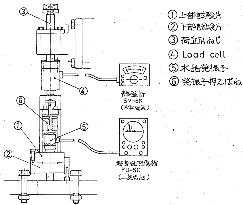
附図-5 実験装置
