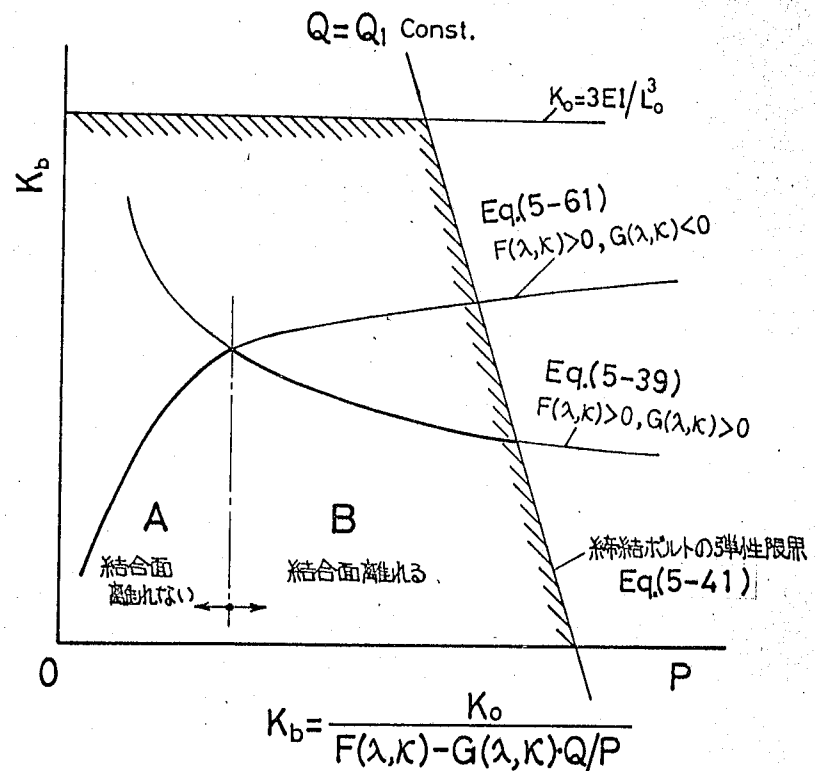
図5-37 曲げ静剛性の近似モデルによる理論解の適用範囲
