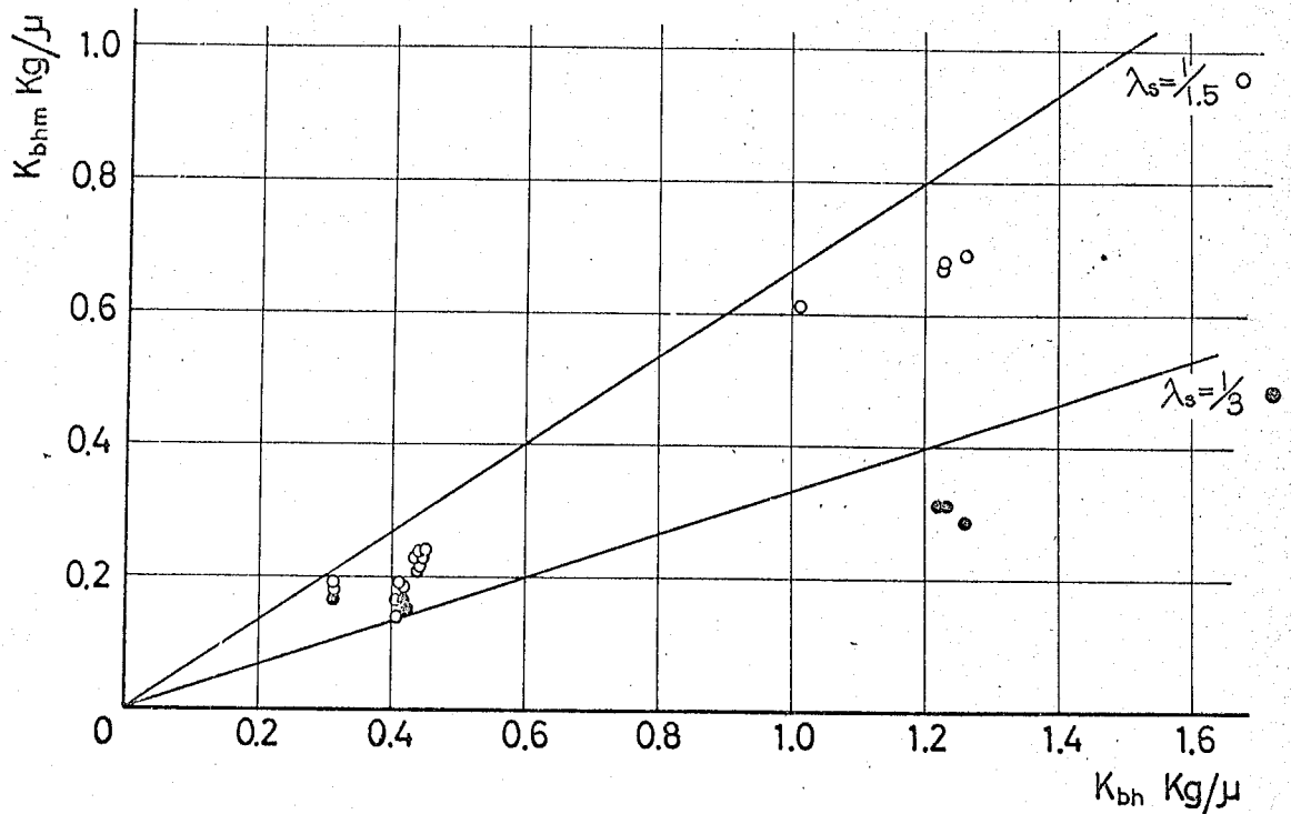
図6-9 模型則の理論値と実験値の比較 (横曲げ静剛性)
