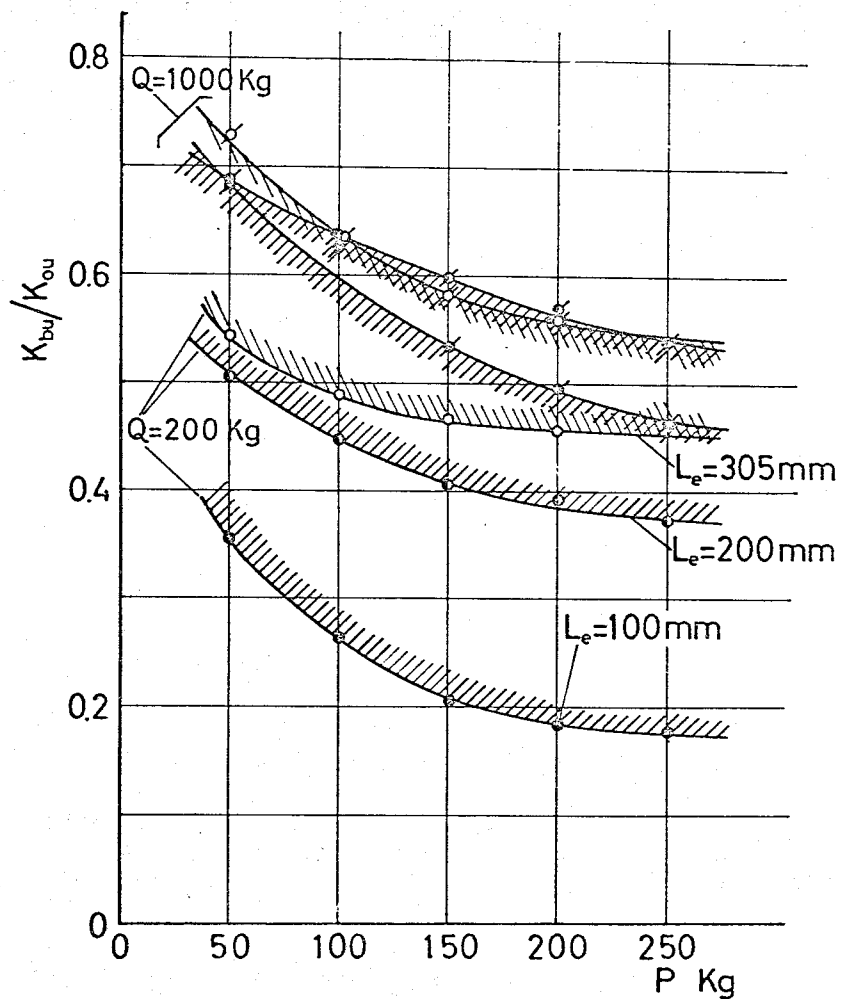
図 2-21 突出し長さによる上方向剛性比の変化 d=M12 , s_a=60\text{mm} , b=40\text{mm} , h=40\text{mm} .
