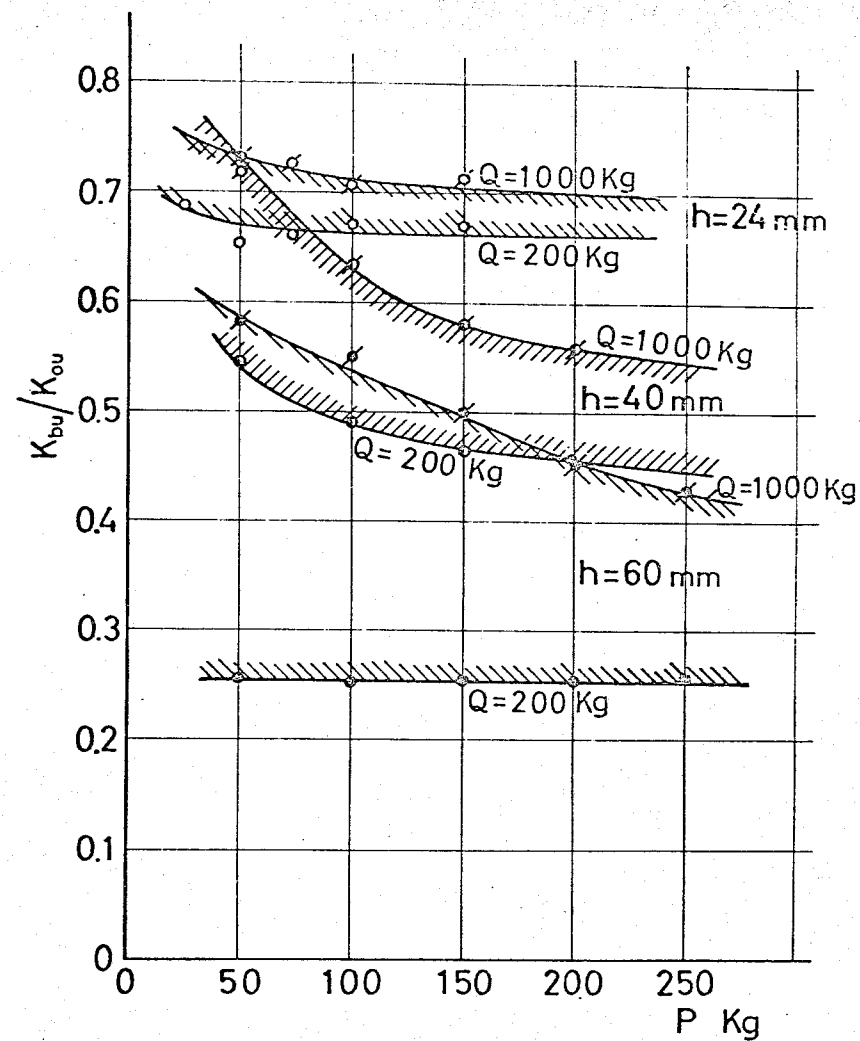
図 2-22 梁の厚さによる上方向曲げ剛性比の変化 d=M12 , s_a=60\text{mm} , b=40\text{mm} , L_e=305\text{mm}
