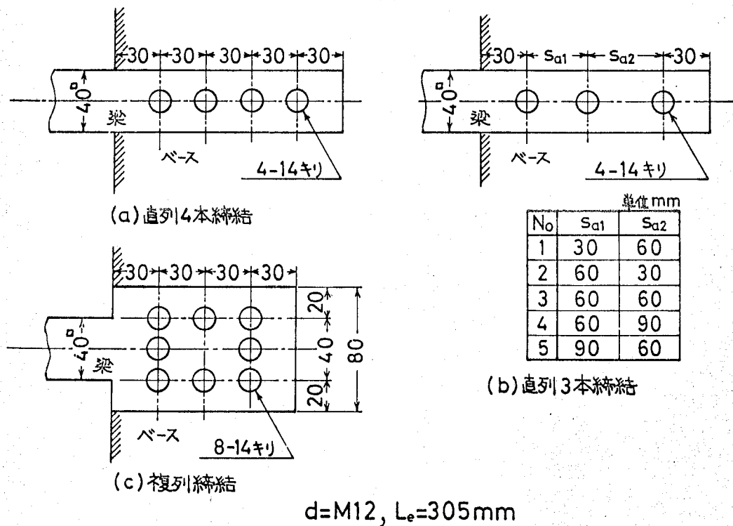
図2-46 締結ボルトの配列位置
