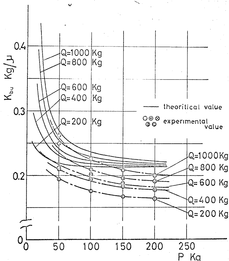
図5-15 曲げ荷重依存性の理論値と実験値の比較(1) d=M12, z_n=2, s_a=60\text{ mm}, b=h=40\text{ mm}, L_c=305\text{ mm}
