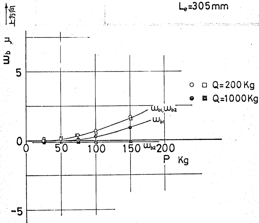
図 2-10 締結ボルトの伸び
