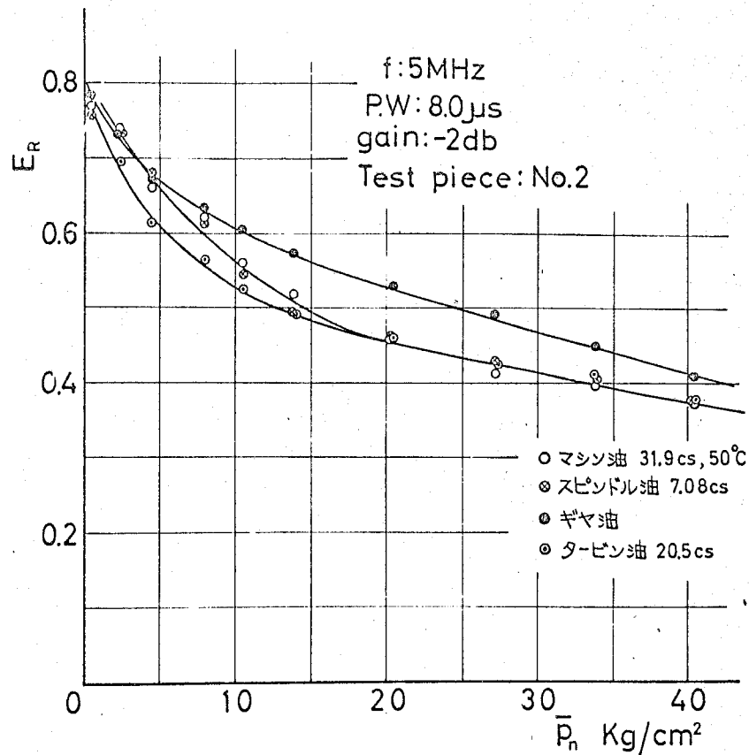
附図-10 発振子塗付油の反射波高比に及ぼす影響
