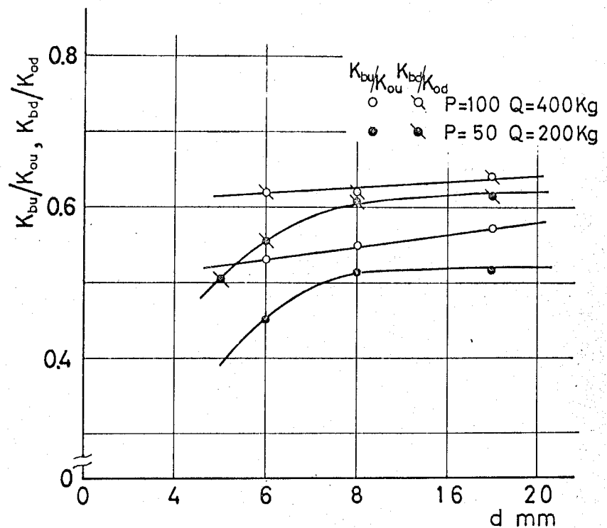
図 2-19 曲げ剛性比に及ぼす締結ボルト径の影響 s_a=40\text{mm} , L_e=305\text{mm} , h=40\text{mm} , b=40\text{mm}
