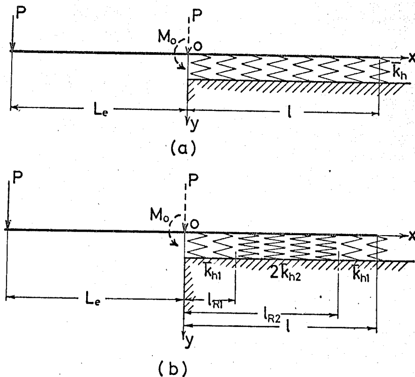
図5-39 横曲げにおける直列二本ボルト締結梁の近似モデル
