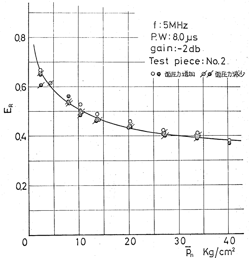
附図-15 接触面圧力の増減による反射波高比の変化
