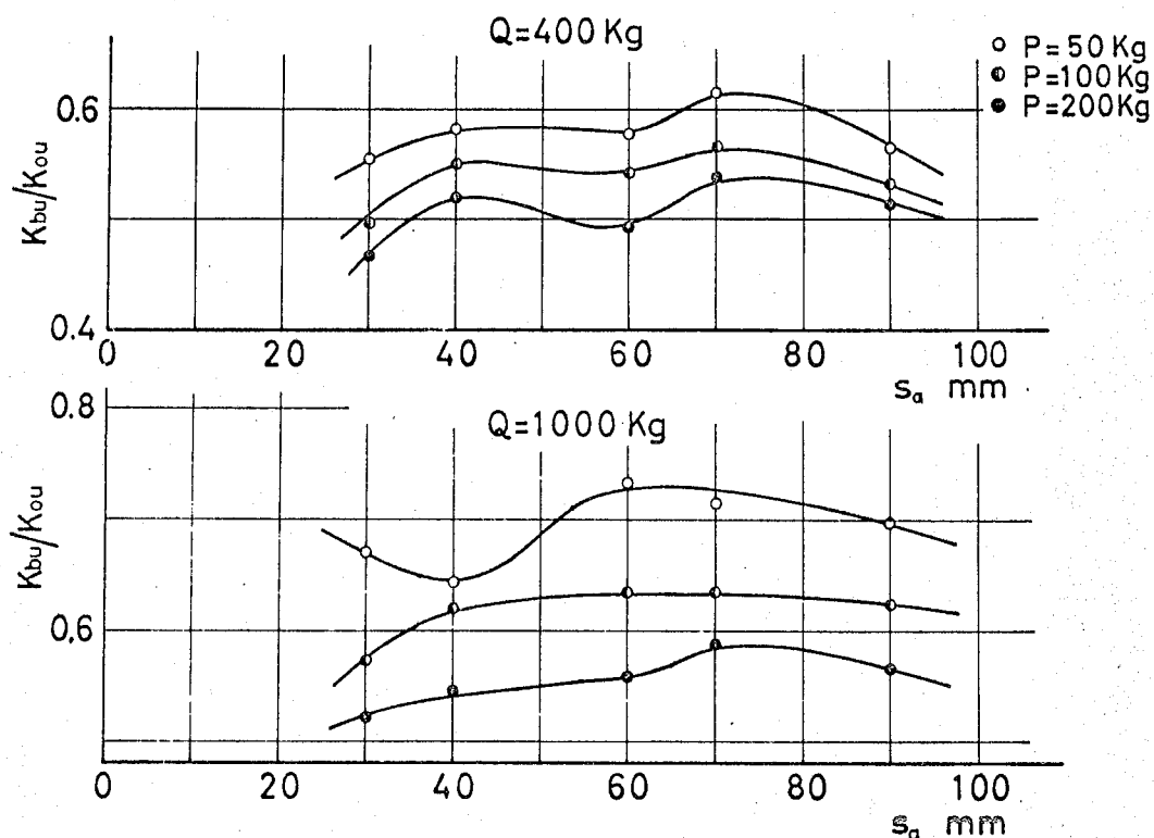
図 2-17 上方向曲げ剛性比に及ぼす締付間隔の影響 d=M12, h=40\text{mm}, b=40\text{mm}, L_e=305\text{mm}
