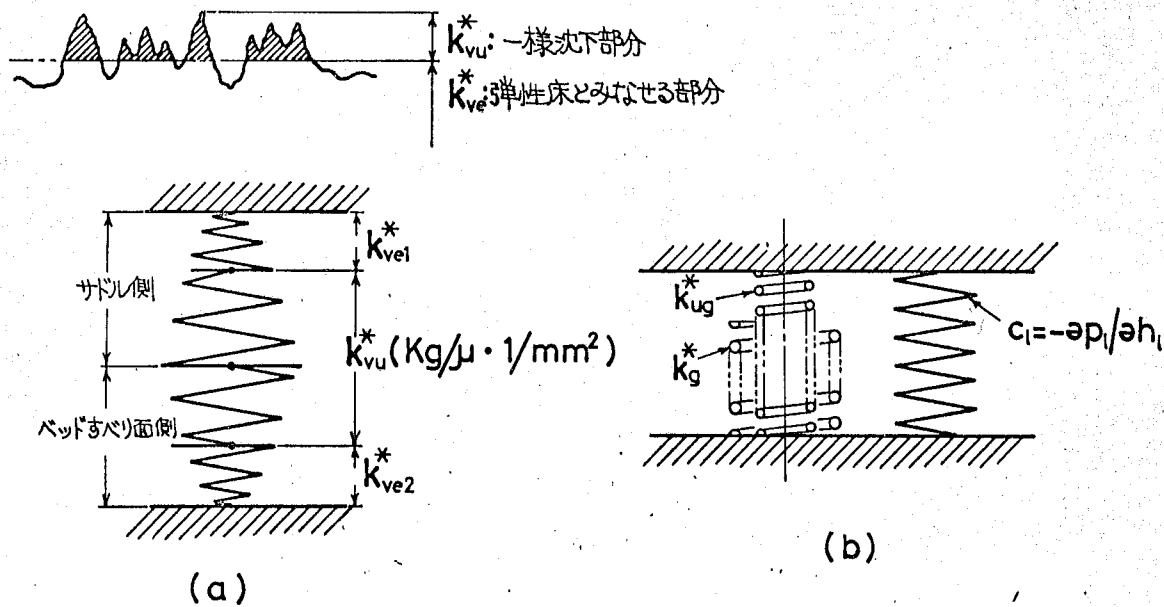
図3-20 二平面接合部のばね作用並びに接合部のモデル
