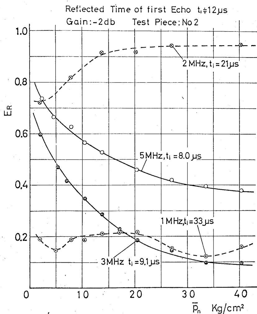
附図-17 \phi 1 反射波戻り時間と送信パルス幅の関係
