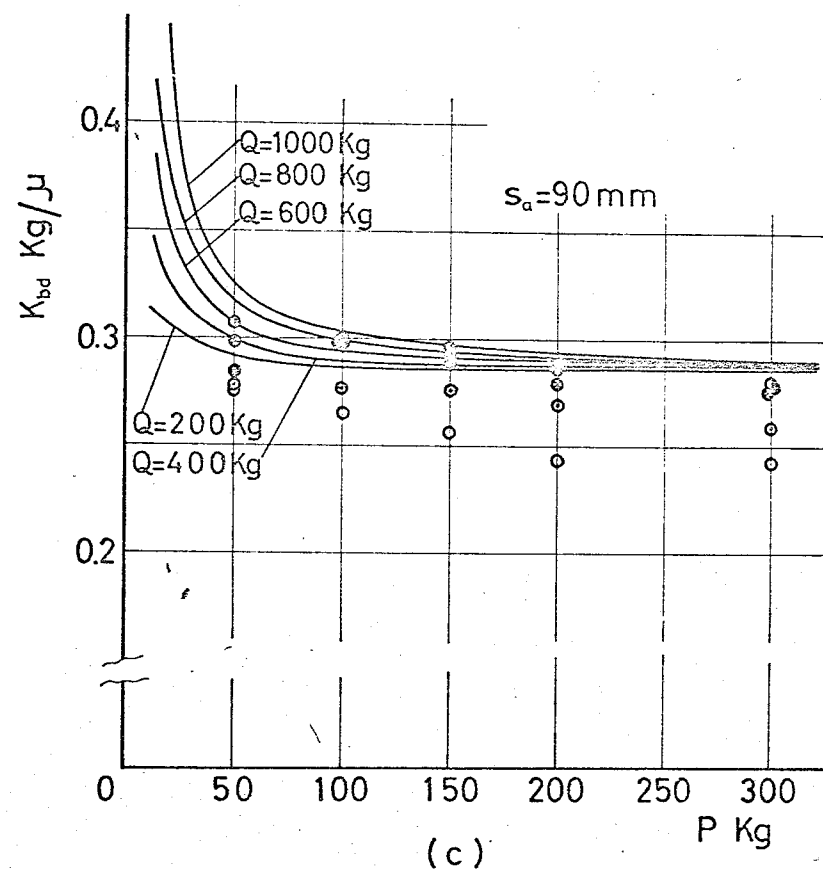
図5-17 曲げ荷重依存性の理論値と実験値の比較(2) d=M12 , b=h=40\text{mm} , L_e=305\text{mm}
