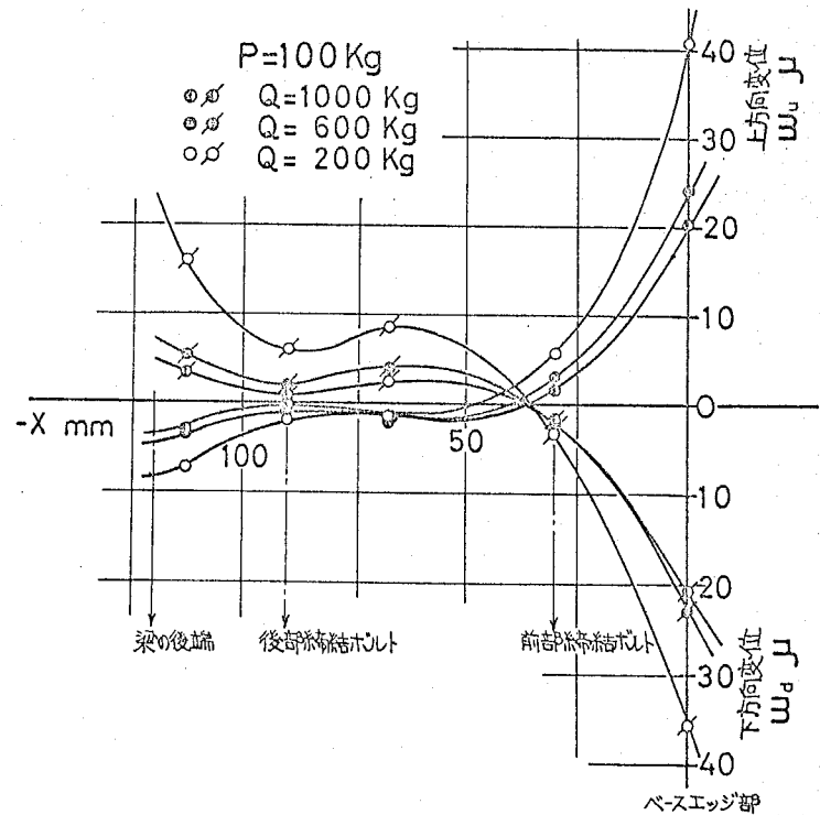
図5-2 結合面に於ける直列二本ボルト締結梁の変形状態 d=M12 , s_a=60\text{mm} , b=h=40\text{mm} , L_e=305\text{mm}
