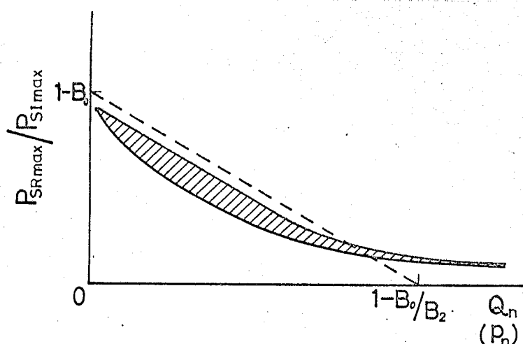
附図-4 反射波音圧と接触面圧力の定性的関係
