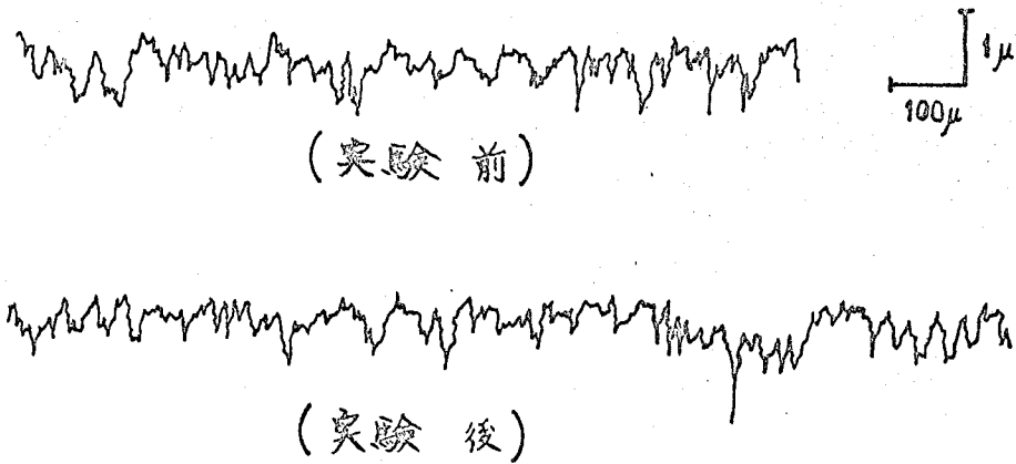
図4-10 荷重の前,後に於ける表面粗さの変化(研削仕上面)
