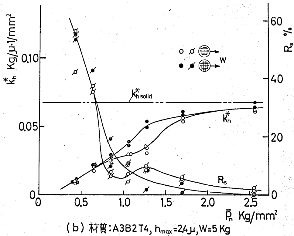
図4-16 材質が異なるときの研削方向の影響
