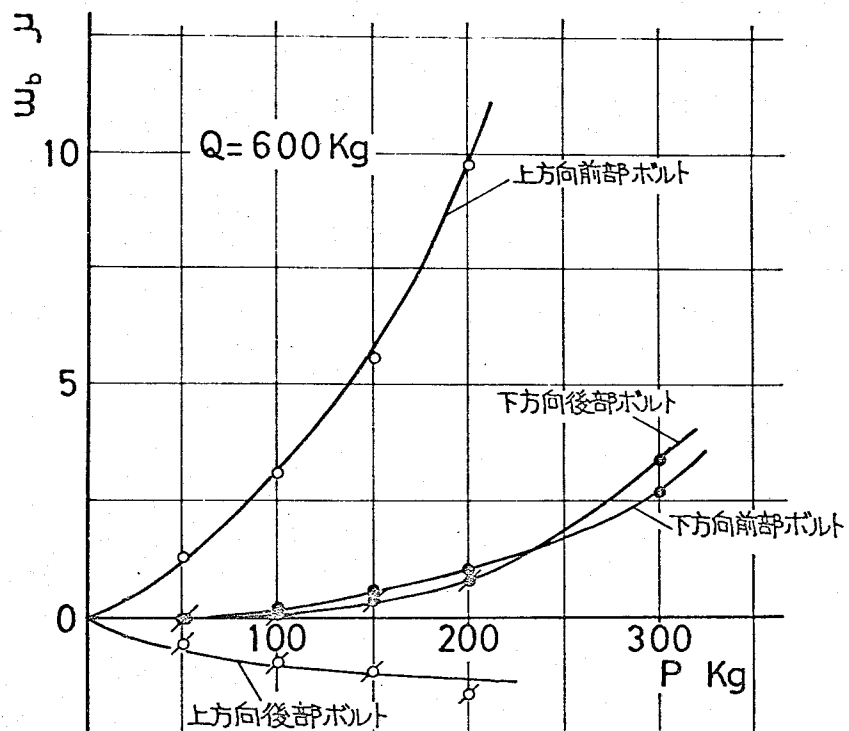
図 2-13 上方向曲げに於ける締結ボルトの伸び d=M12 , s_a=60\text{mm} , b=h=40\text{mm} , L_e=305\text{mm}
