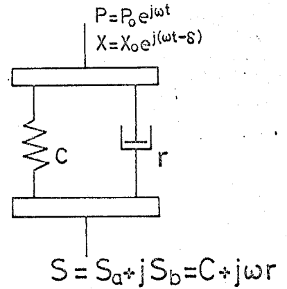
図 1-5 結合面動剛性の定義 (Corbach による)
