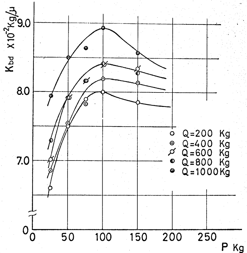
図 2-9 曲げ荷重による下方向静剛性の変化 d = \text{M12} , h = 24\text{mm} , b = 40\text{mm} , s_a = 60\text{mm} , L_e = 305\text{mm}
