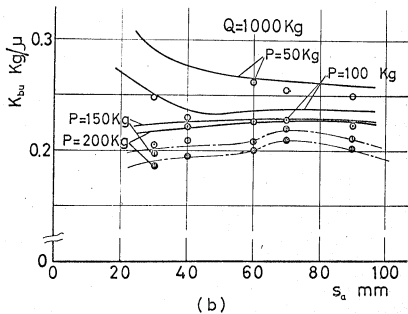
図5-28 曲げ静剛性の締付間隔依存性の理論値と 実験値の比較(1)
