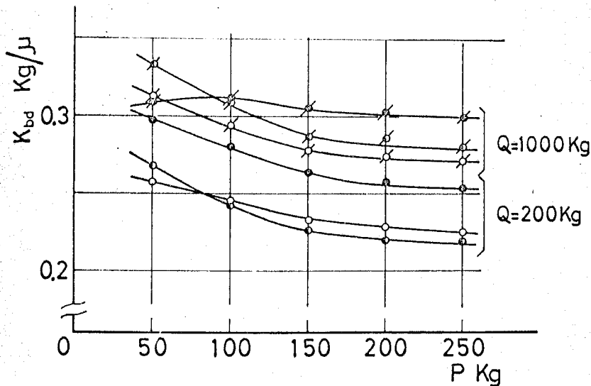
図 2-27 下方向曲げ静剛性に及ぼすベースの厚さの影響 (締結条件, 図中の記号は図 2-26 と同じ)
