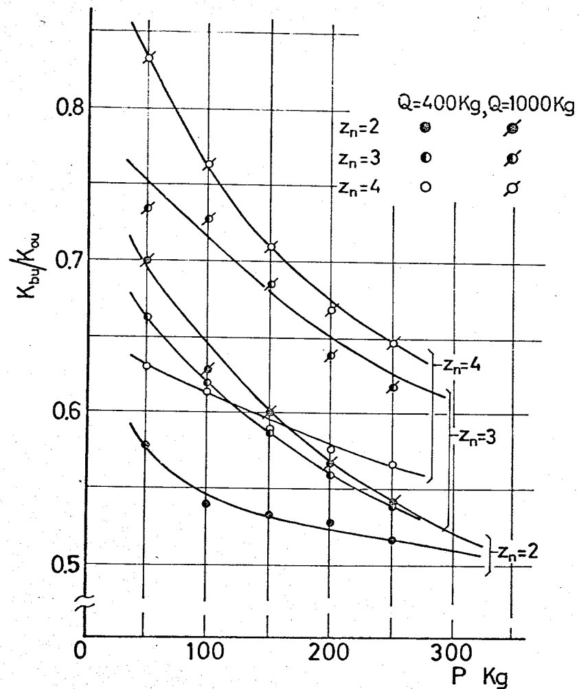
図 2-53 締結本数による上方向曲げ剛性比の変化 (直列多数締結の場合)
