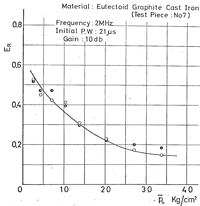
附図-21 材質による反射波高比の変化(3)
