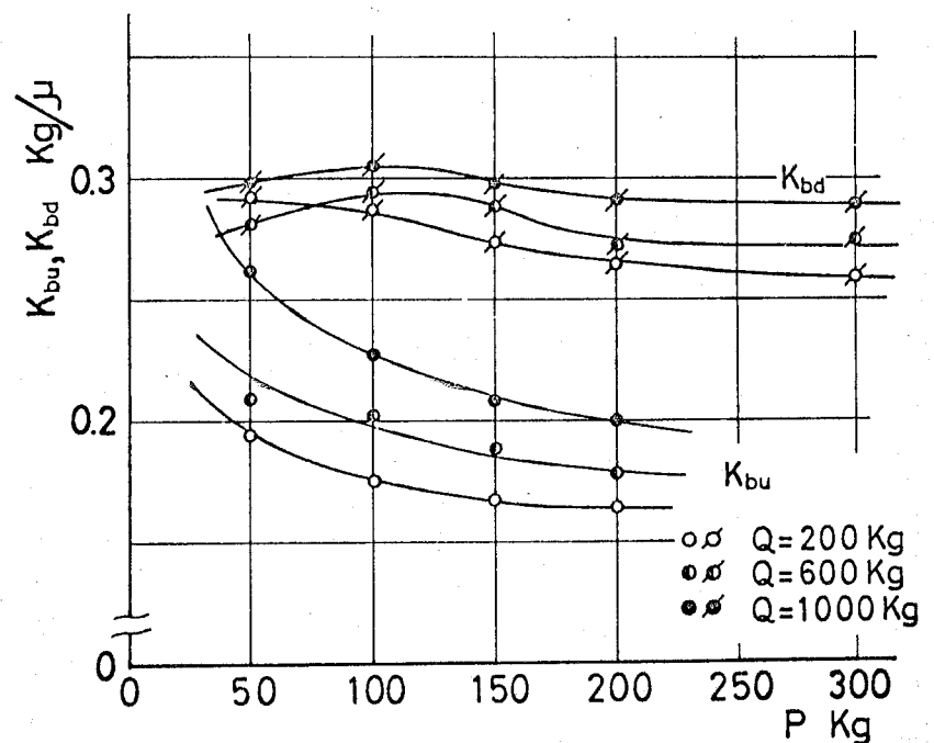
図 2-8 曲げ静剛性に及ぼす曲げ荷重の影響
