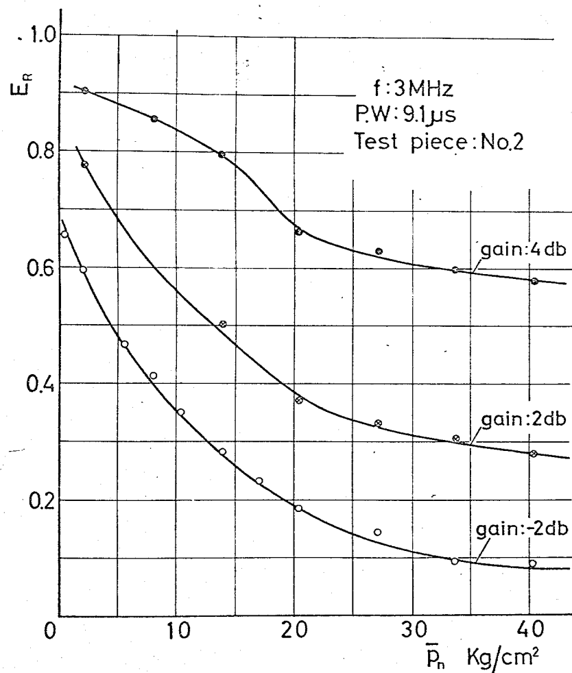
附図-11 発振子出力の反射波高比に及ぼす影響
