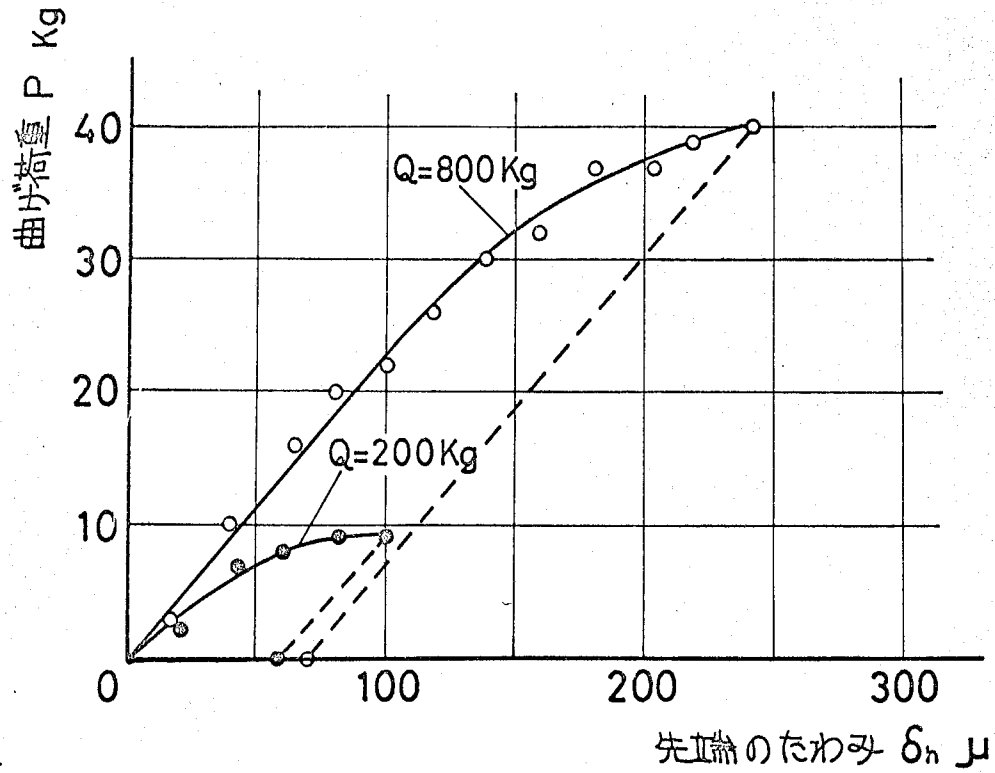
図 2-32 曲げ荷重によるたわみの挙動
