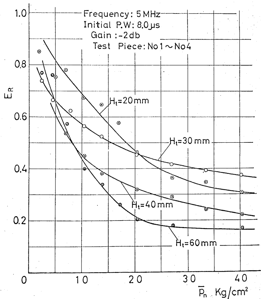
附図-18 試験片の厚さによる反射波高比の変化
