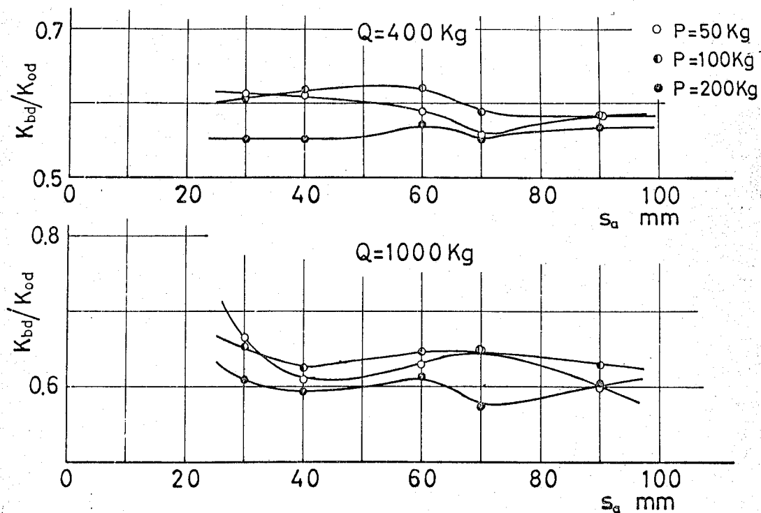
図 2-18 下方向曲げ剛性比に及ぼす締付間隔の影響 d=M12 , h=40\text{ mm} , b=40\text{ mm} , L_e=305\text{ mm}
