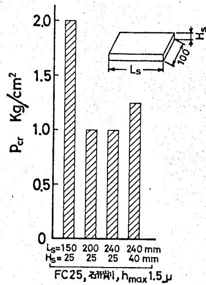
図 3-16 サドルの形状による限界面圧力の変化
