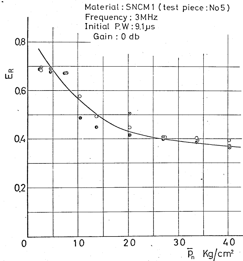
附図-19 材質による反射波高比の変化(1)
