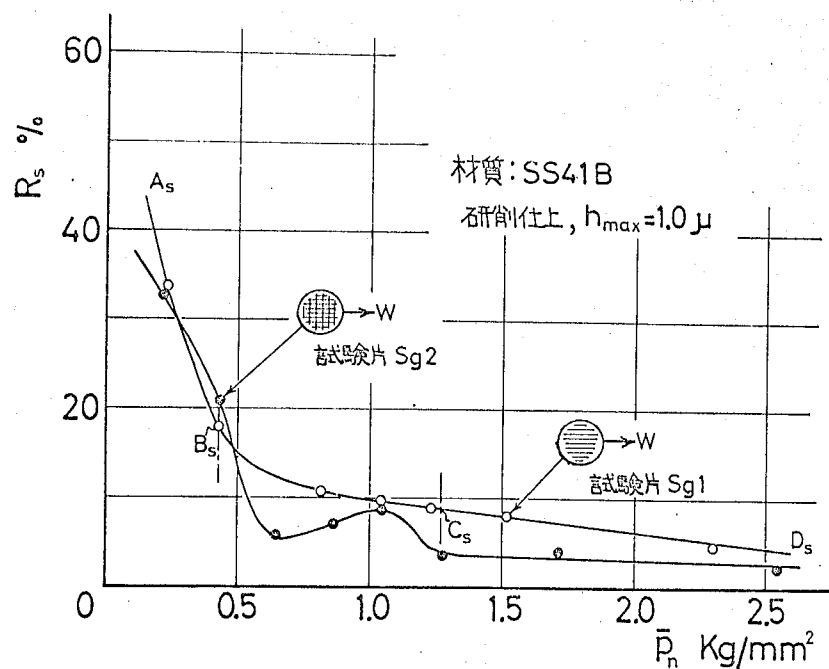
図4-8 すべり変位率に及ぼす平均接触面圧力の影響
