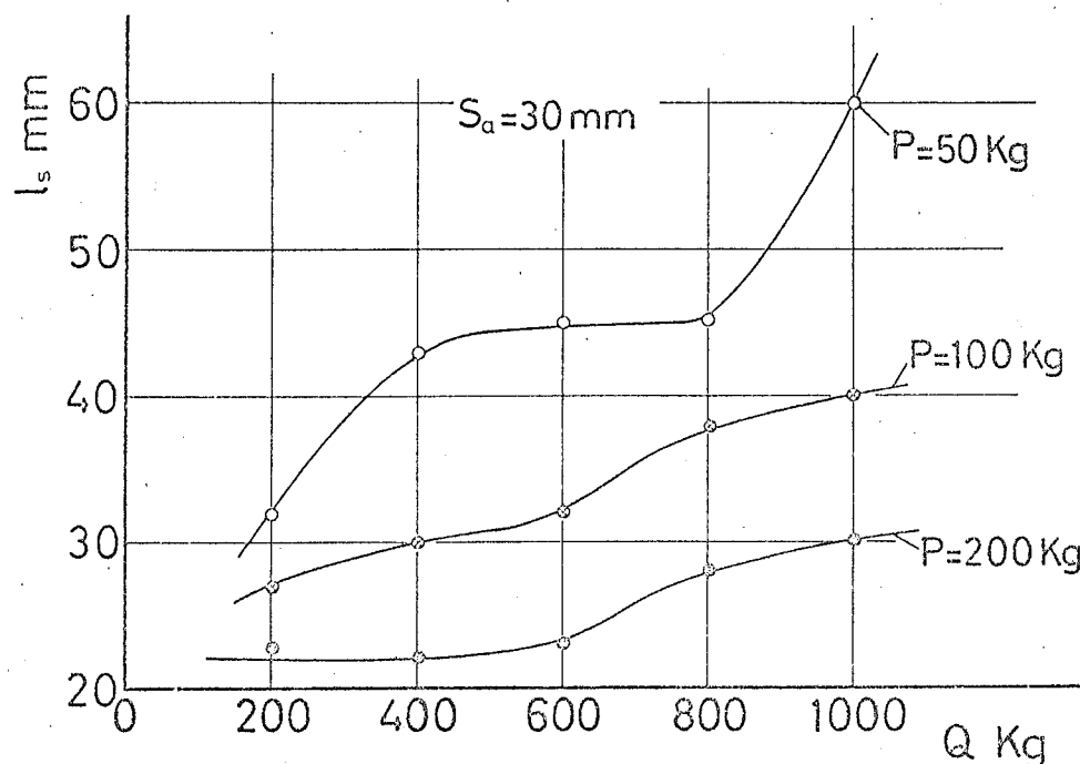
図5-10 ベースエッジ部における梁の接触長さ l_s (下方方向曲げ)
