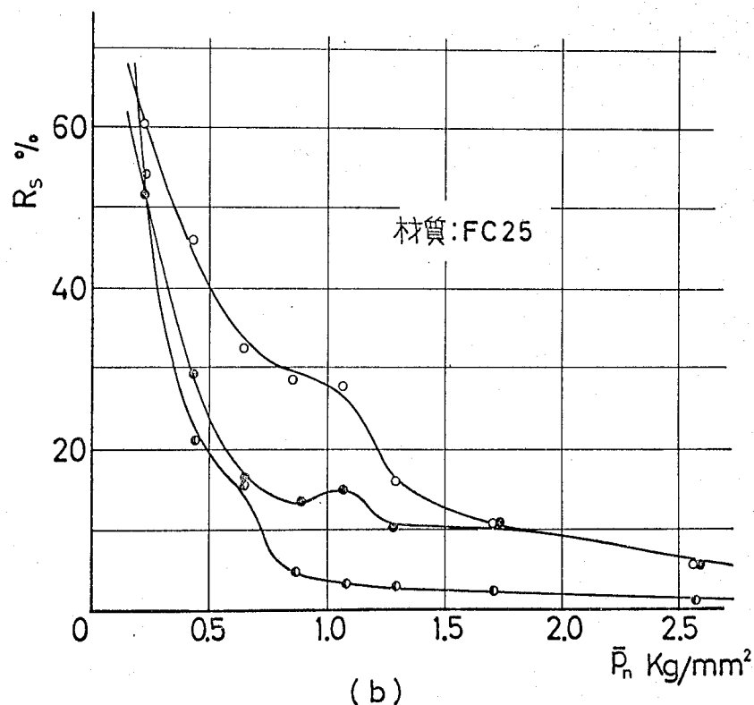
図 4-12 表面仕上状態の横方向接触剛性としべり変位率に及ぼす影響
