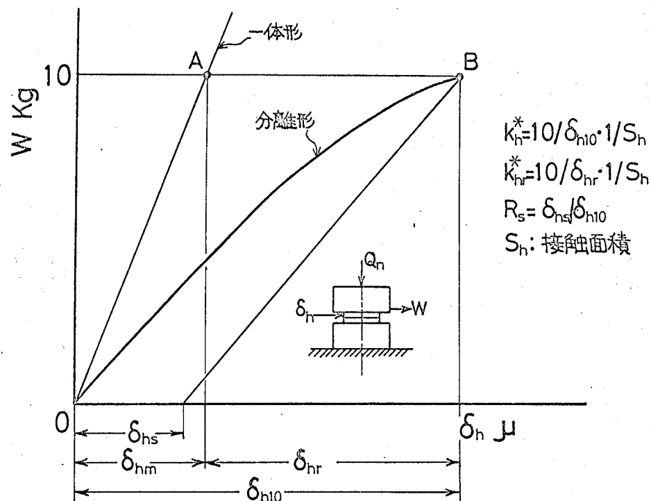
図4-5 横方向接触剛性とすべり変位率の定義
