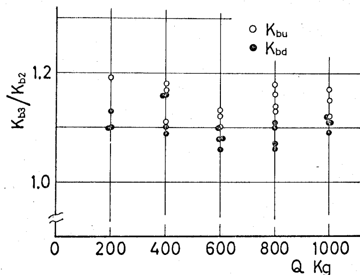
図2-47 曲げ静剛性の増加に及ぼす中間ボルトの効果
