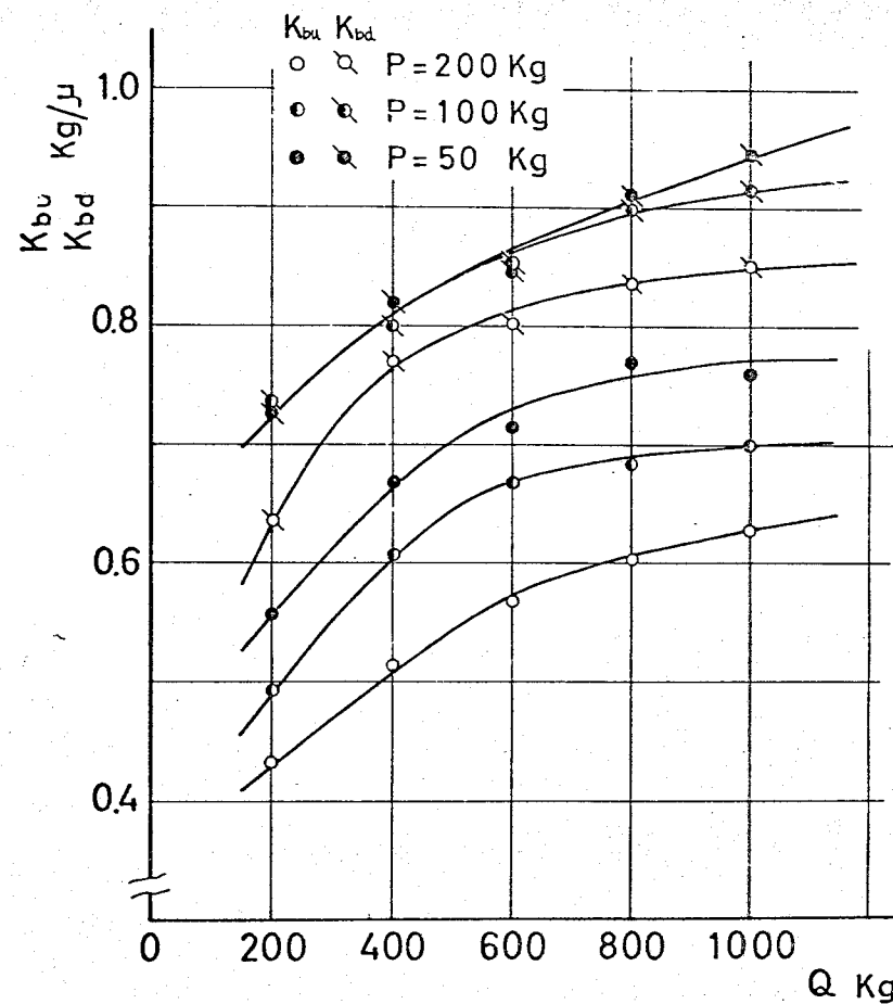
図 2-14 曲げ静剛性に及ぼすボルト締付力の影響 d=M12 , s_a=60\text{mm} , h=40\text{mm} , b=40\text{mm} , L_e=200\text{mm}
