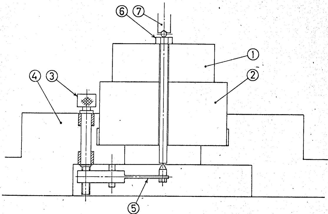
図3-21 実験装置
