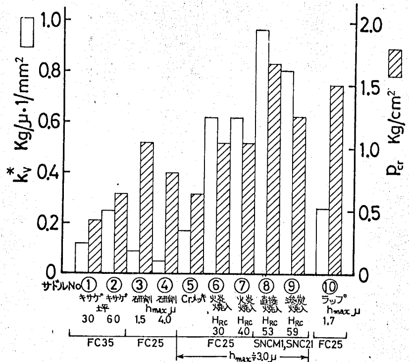
図3-14 床の弾性係数と限界面圧力の測定値 (ベッドすべり面 No1: ラップ仕上面)
