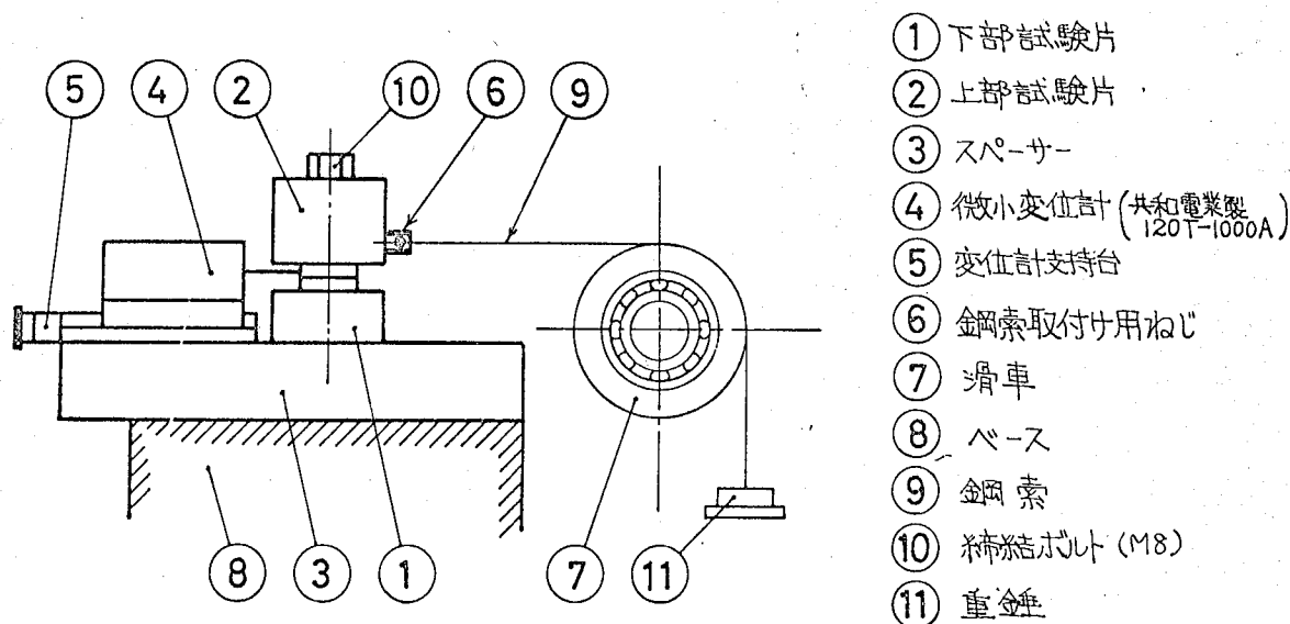
図4-1 横方向接触剛性, すべり変位測定装置の概略図
