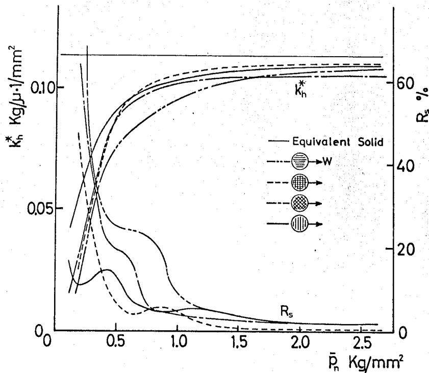
図4-15 横方向接触剛性とすべり変位率に及ぼす研削方向の影響 (材質:FC25, 研削仕上, h_{max}=1.0\mu )
