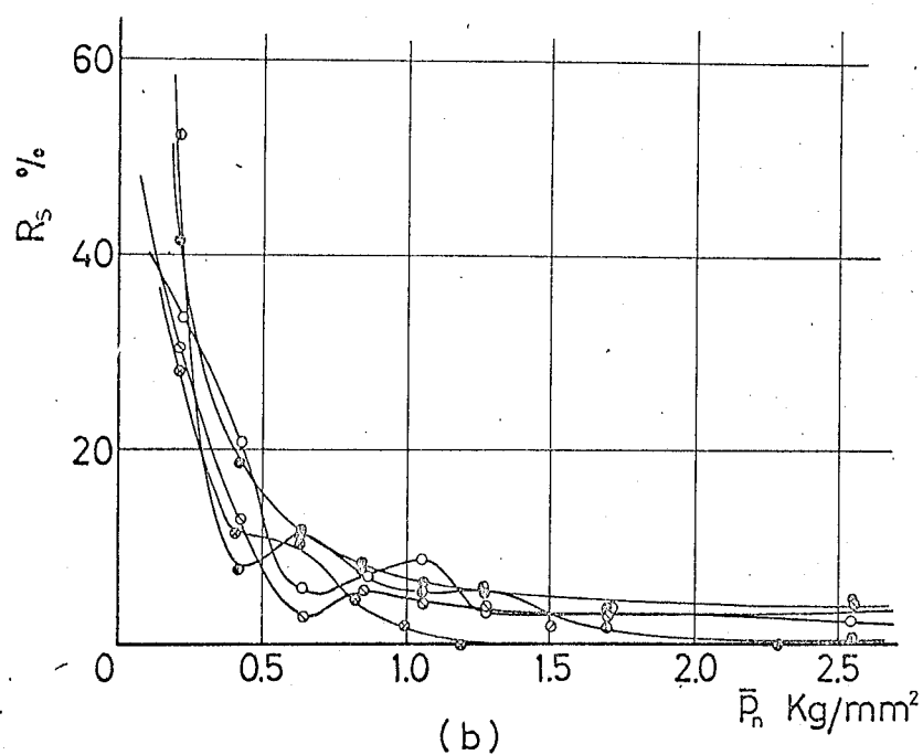
図4-11 表面仕上状態の横方向接触剛性および変位率に及ぼす影響
