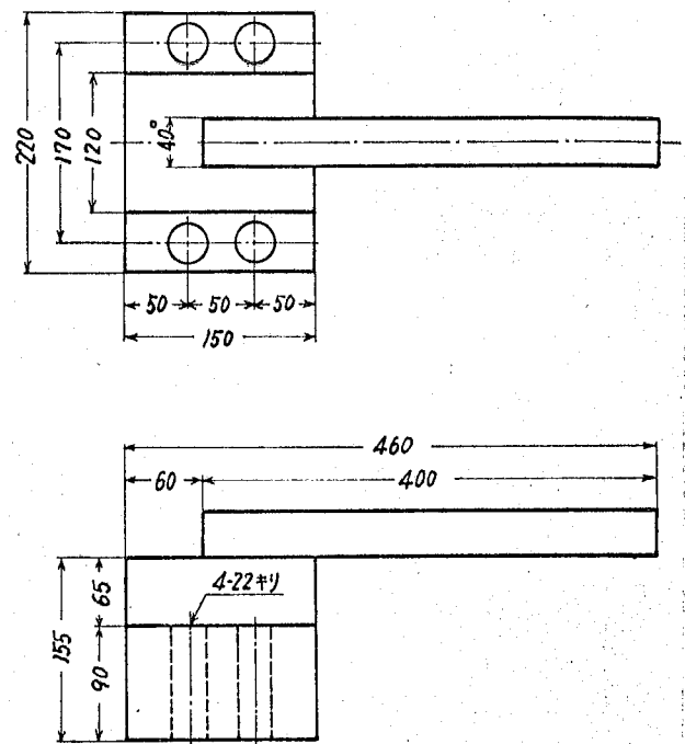
図 2-15 一体形試験片の形状 材質: SS41B
