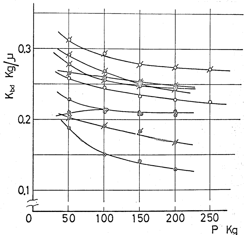
図2-29 下方向曲げ静剛性に及ぼす介在物の影響 (締結条件、図中の記号は図2-28と同じ)
