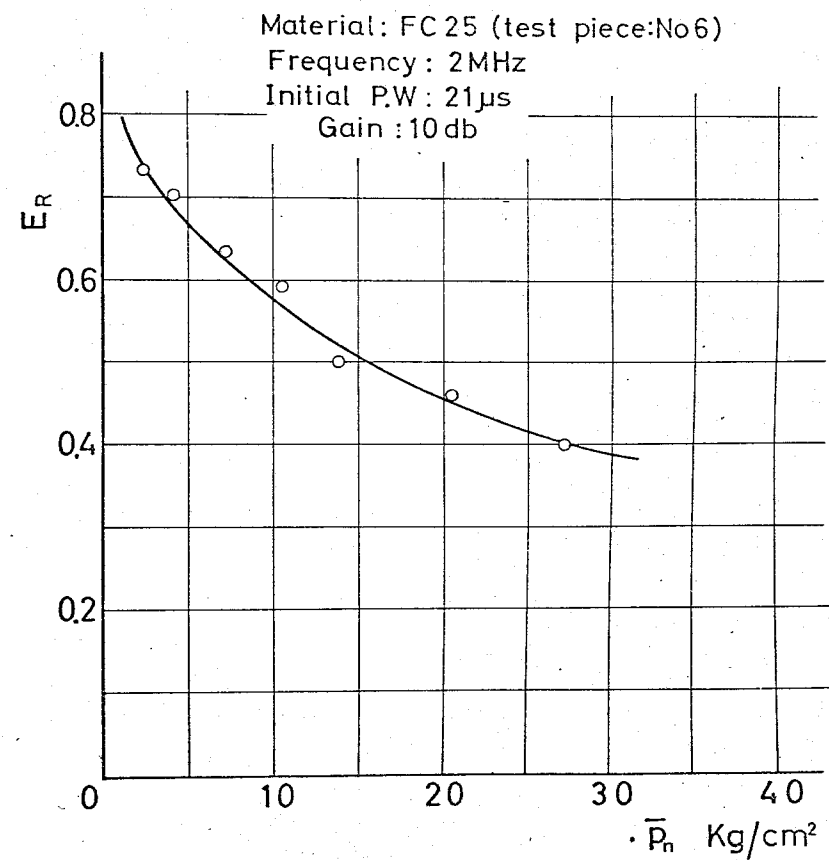
附図-20 材質による反射波高比の変化(2)
