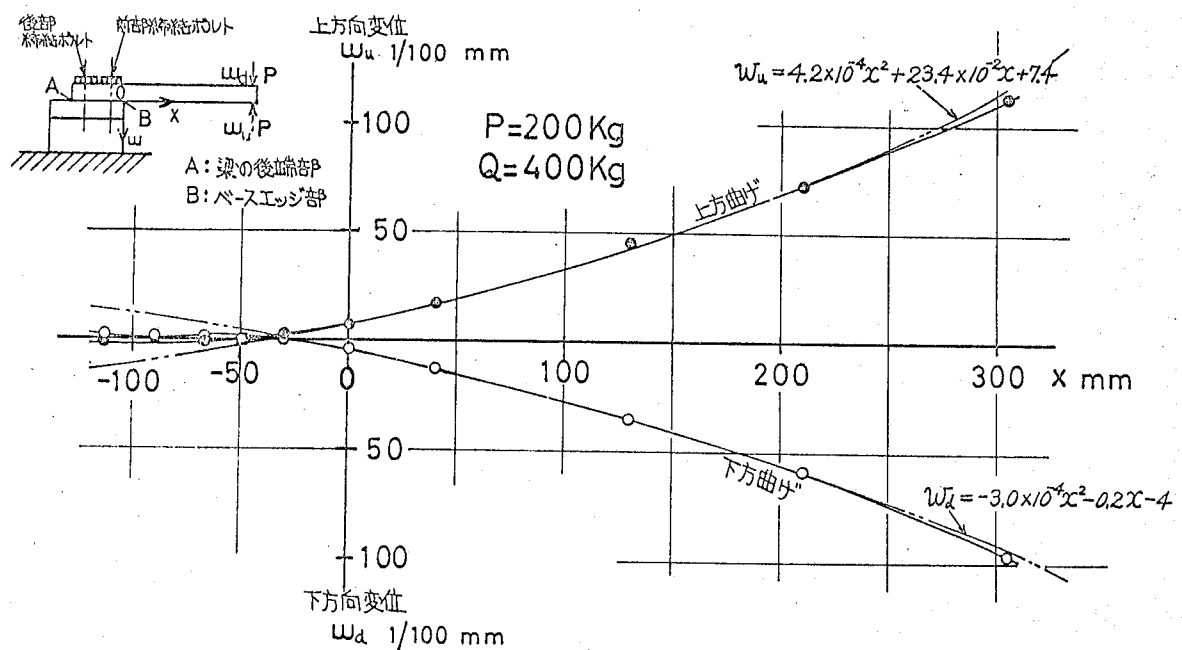
図5-1 直列二本ボルト締結梁の変形曲線
