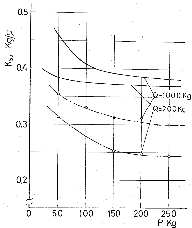
図 5-26 多数ボルト締結時の曲げ荷重依存性の理論値と実験値の比較 d=M12
