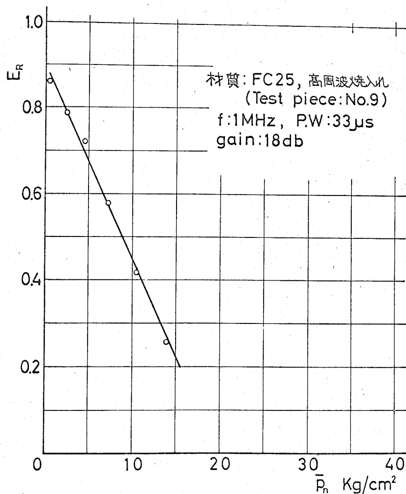
附図-23 材質による反射波高比の変化(5)
