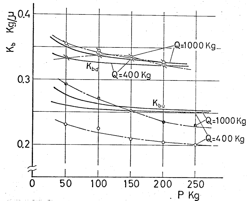
図5-24 多数ボルト締結時の曲げ荷重依存性の理論値と実験値の比較 d=M12, s_a=30\text{ mm}, L_e=305\text{ mm}
