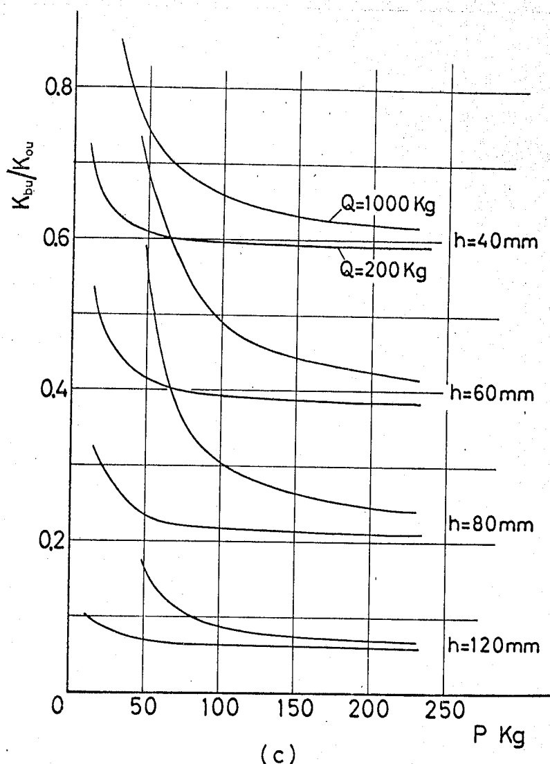
図5-34 梁の厚さによる曲げ剛性比の変化 d=M12 , s_a=60\text{ mm} , b=40\text{ mm}
