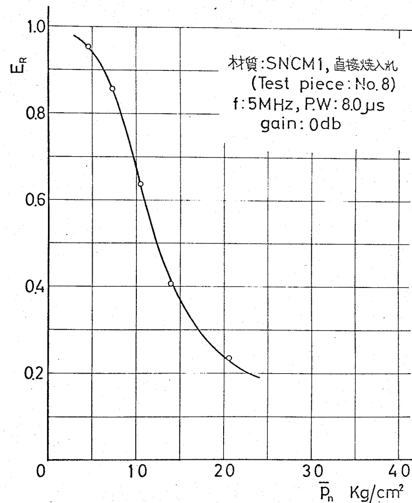
附図-22 材質による反射波高比の変化(4)
