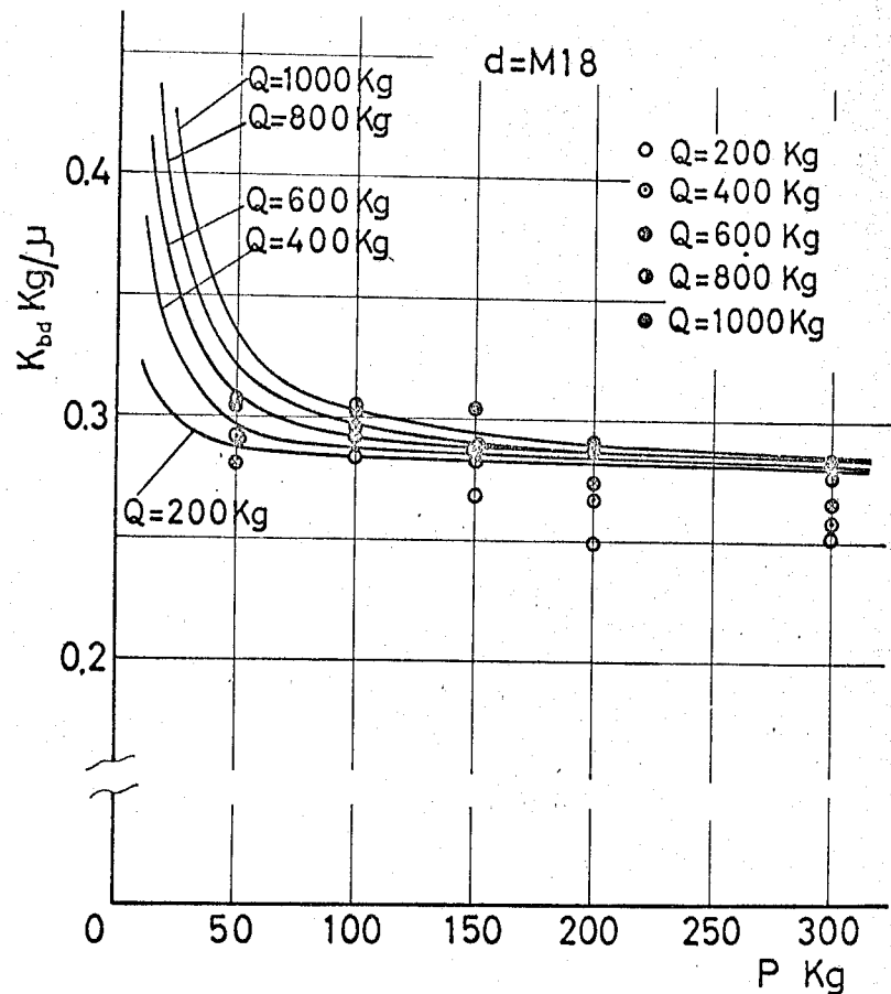
図5-32 締結ボルト径を変えたときの曲げ荷重依存性(2) s_0=40\text{mm} , b=h=40\text{mm} , L_e=305\text{mm}
