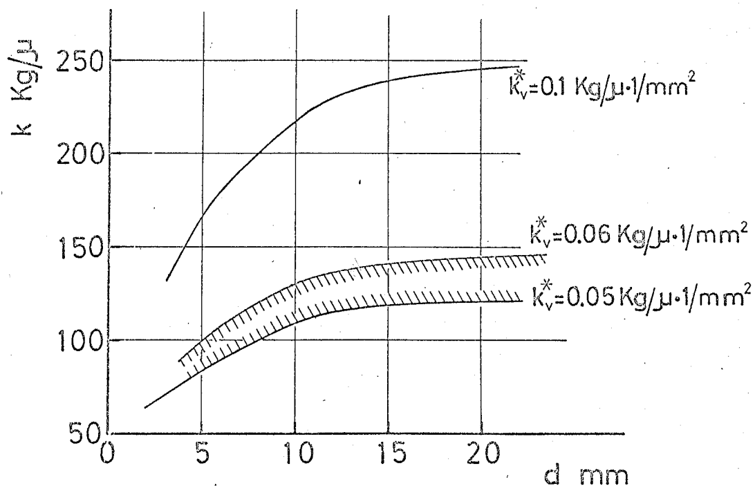
図5-8 ベースの等価ばね定数 b=h=40\text{mm}
