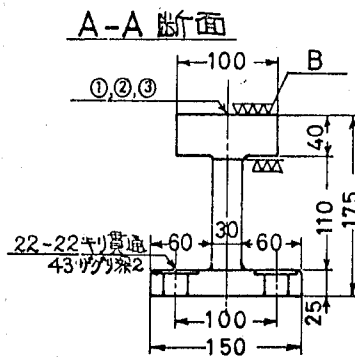
図3-6 ベッドすべり面の寸法と形状
