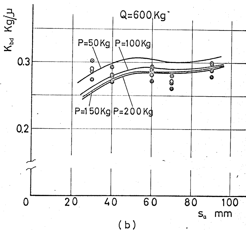
図 5-29 曲げ静剛性の締付間隔依存性の理論値と 実験値の比較 (2) d=M12 , b=h=40\text{mm} , L_e=305\text{mm}
