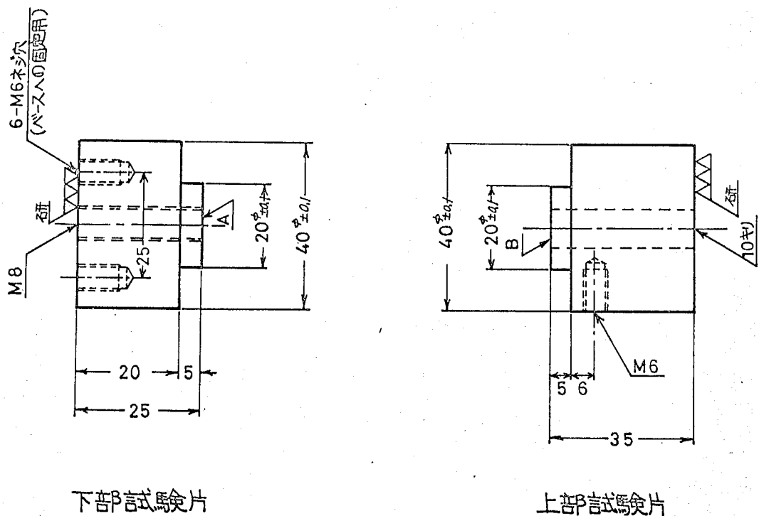
図4-2 試験片の寸法と形状
