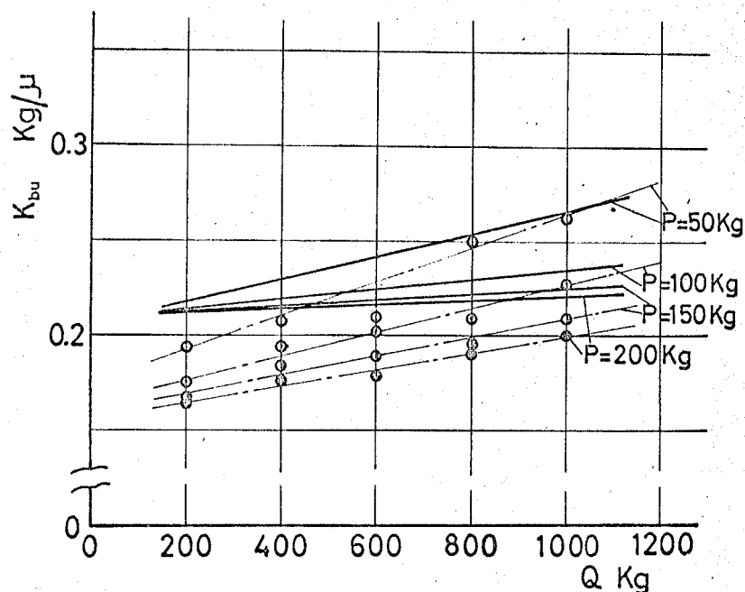
図5-22 締付力依存性の理論値と実験値の比較
