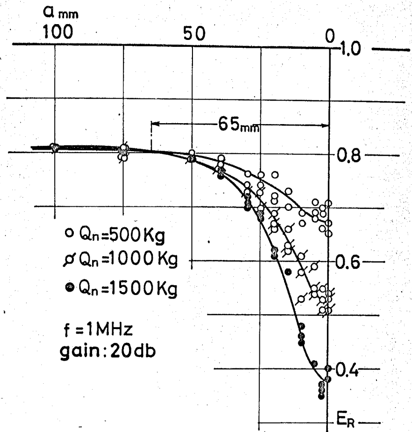
図3-11 反射波高比分布の測定例 サドル: No3, ベッドすべり面: No1
