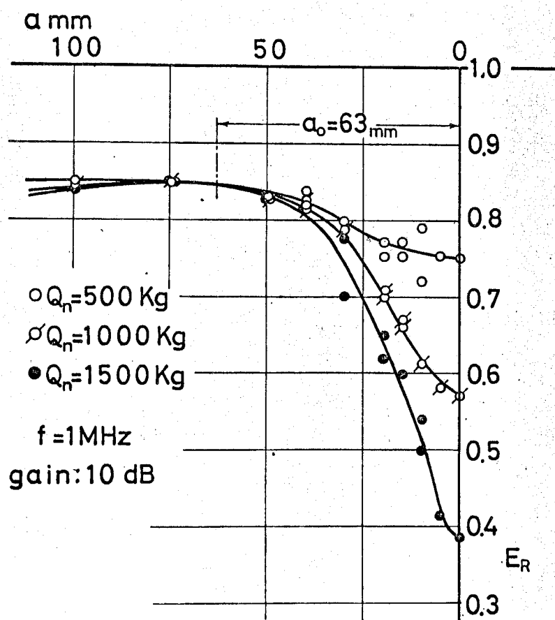
図3-13 日時を経た後の反射波高比分布 サドル:No3, ベッドすべり面:No1
