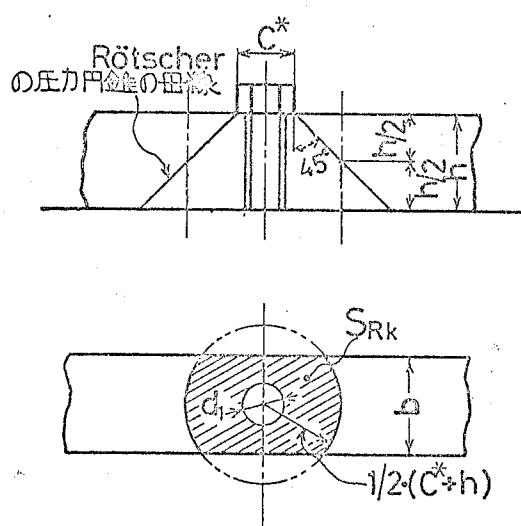
図5-7 Rötischerの説により定まる接合面がボルト結合部のばね作用に關係する範囲
