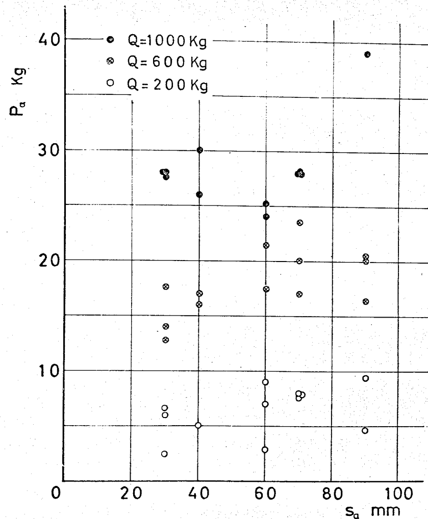
図 2-39 ボルト締付間隔による限界曲げ荷重の変化 締結条件は図 2-38 と同じ
