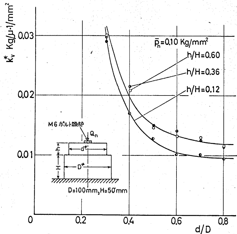
図3-22 垂直方向接触剛性の試片寸法依存性 材質 S45C, 研削仕上面, h_{max}=5.0\mu
