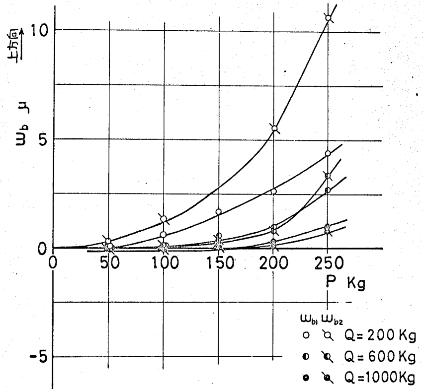
図 2-11 下方向曲げに於ける締結ボルトの伸び (図 2-8 の場合)
