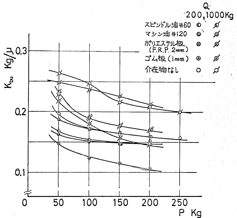
図2-28 上方向曲げ静剛性に及ぼす介在物の影響 d=M12, H=85\text{mm}, s_a=60\text{mm}, b=h=40\text{mm}, L_e=305\text{mm}
