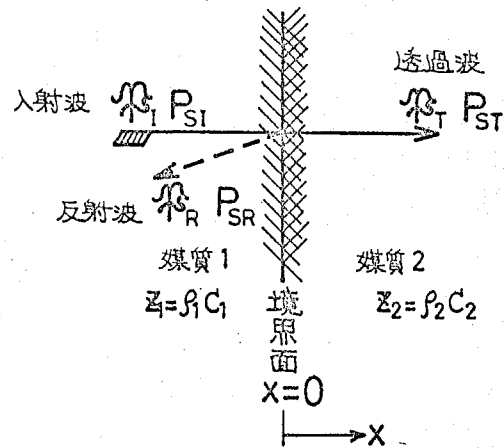
附図-1 境界面に於ける平面波の反射
