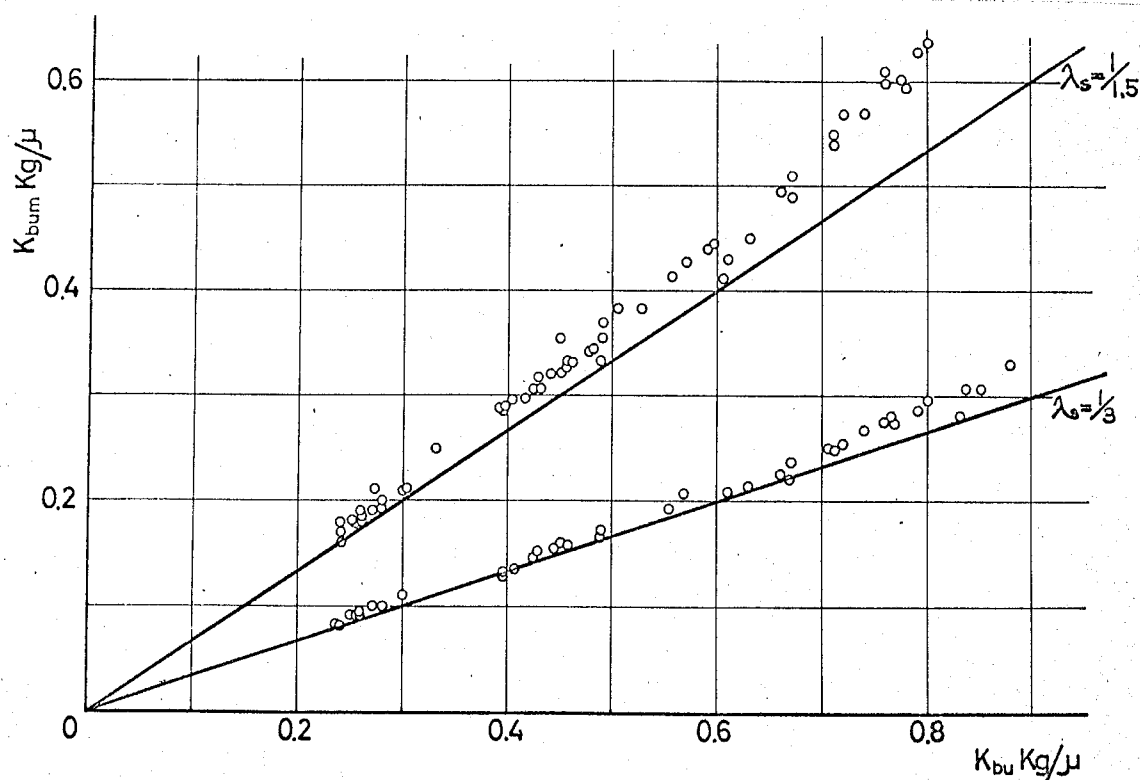
図6-3 模型則の理論値と実験値の比較（上方向曲げ静剛性）
