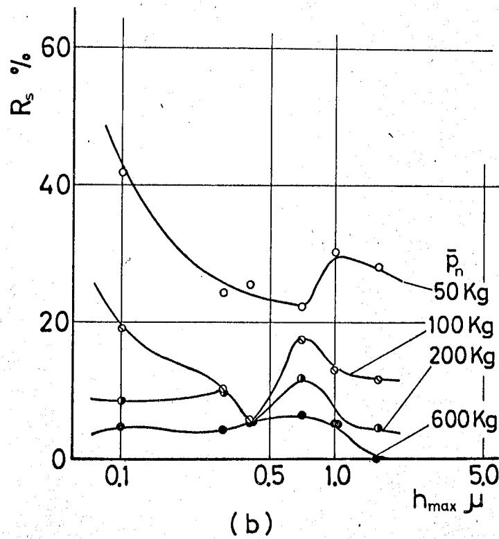
図 4-17 横方向接触剛性とすべり変位率に及ぼす表面粗さの影響 (材質: SS41B, ラップ仕上面)
