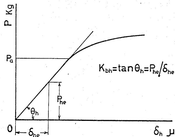
図 2-34 横剛性値の定義の説明図
