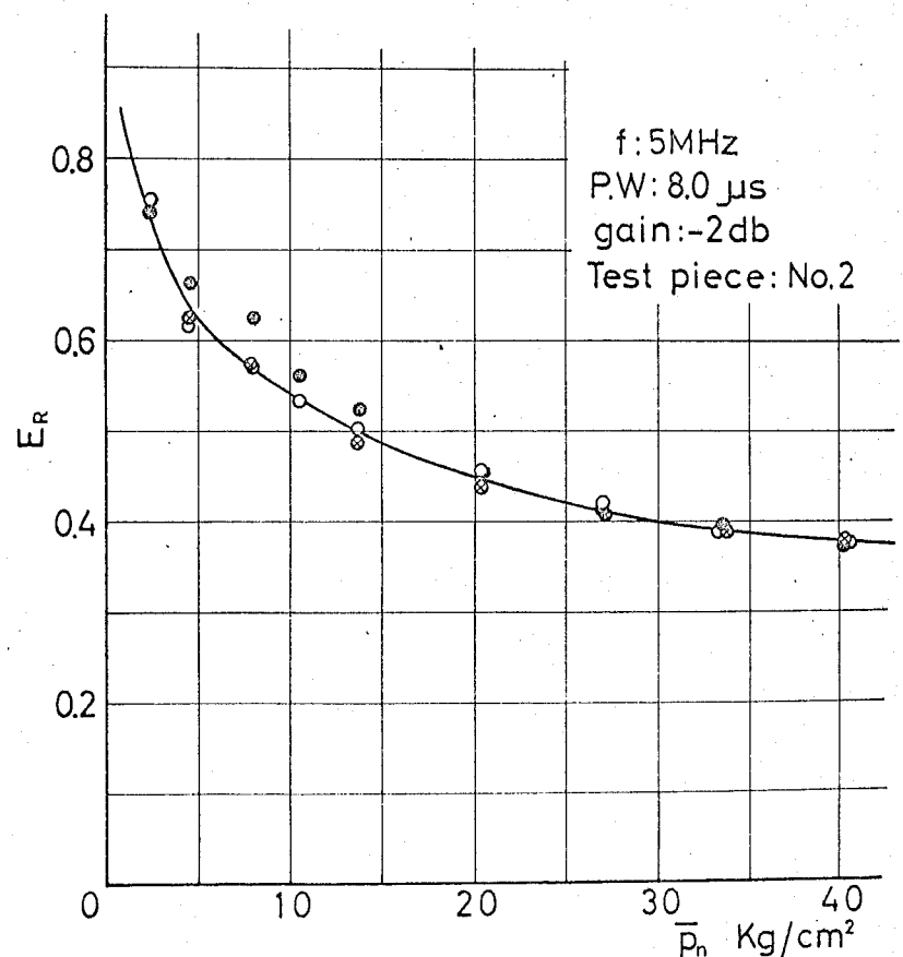
附図-14 繰返し測定精度
