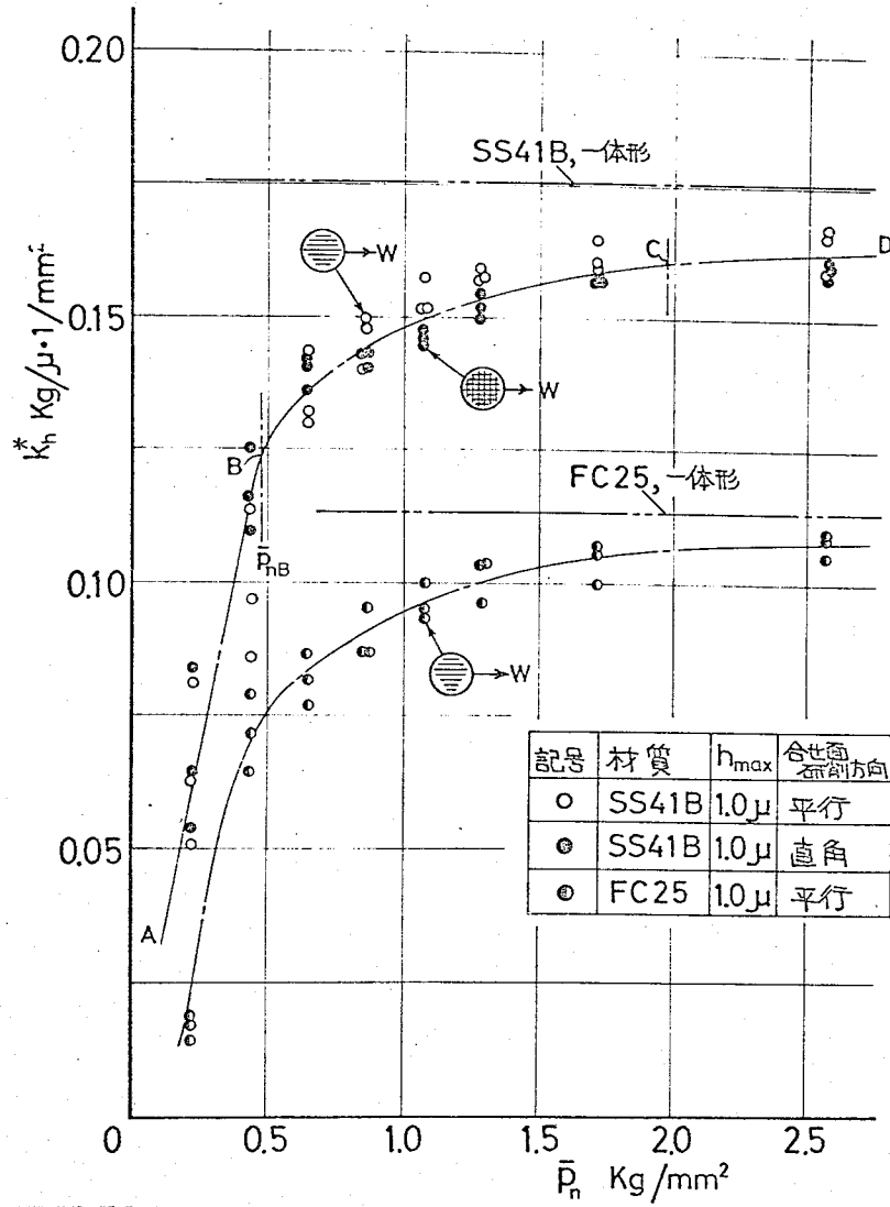
図 4-6 みがけの横方向接触剛性に及ぼす平均接触面圧力の影響
