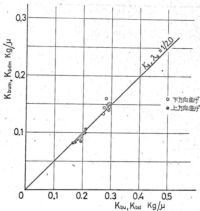
図6-6 垂直曲げ静剛性の模型実験の結果 (実物を締結ボルトM12とした場合), \lambda_s = K_s = 1/2.0
