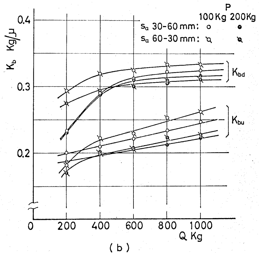
図2-48 曲げ荷重依存性, 締付力依存性に及ぼす中間ボルトの影響
