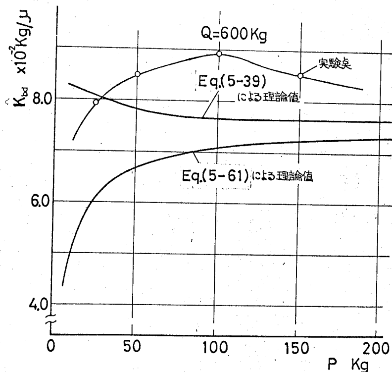
図5-36 結合面が離れないことを考慮したときの曲げ荷重依存性 d=M12, s_a=60\text{mm}, b=40\text{mm}, h=24\text{mm}, L_e=305\text{mm}
