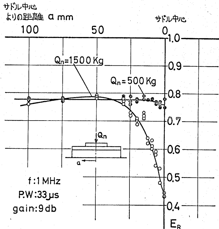
図3-9 集中荷重による反射波高比分布の変化
