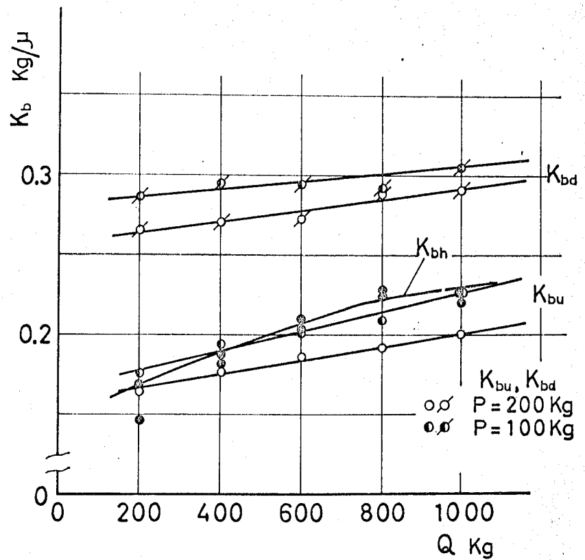
図 2-36 垂直曲げ静剛性と横剛性値の比較
