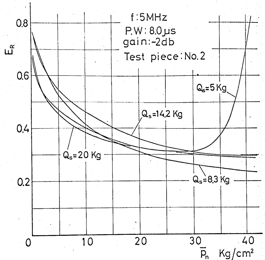
附図-9 発振子押えばね力の反射波高比に及ぼす影響
