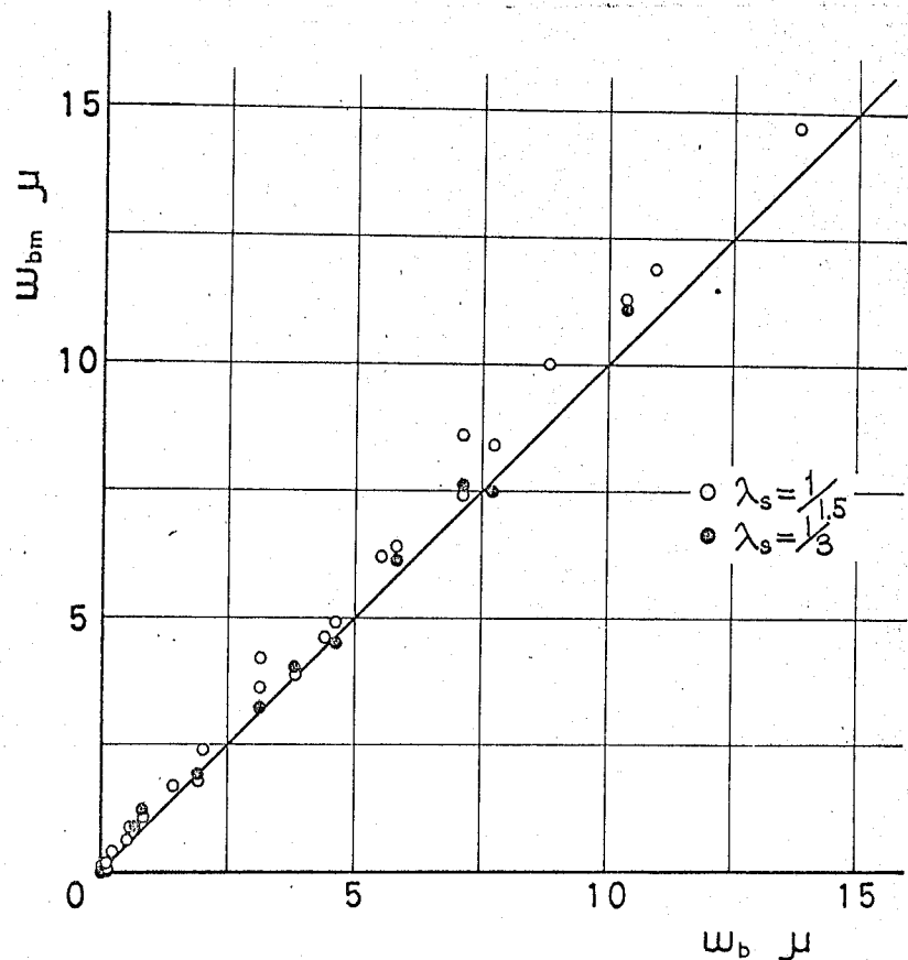
図 6-5 前部締結ボルトの伸びに因る模型実験の結果（上方向曲げの場合）
