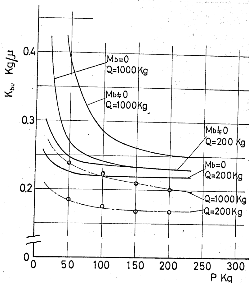
図5-31 ボルト頭部抵抗モーメントの曲げ静剛性に及ぼす影響
