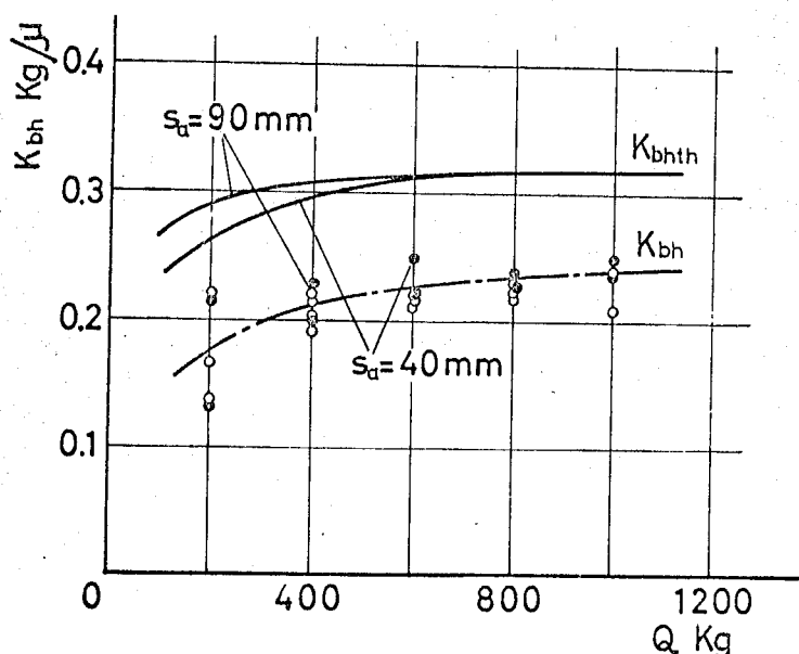
図5-40 横剛性値の理論値と実験値の比較 d=M12, z_n=2, h=40\text{mm}, b=40\text{mm}, L_e=305\text{mm}
