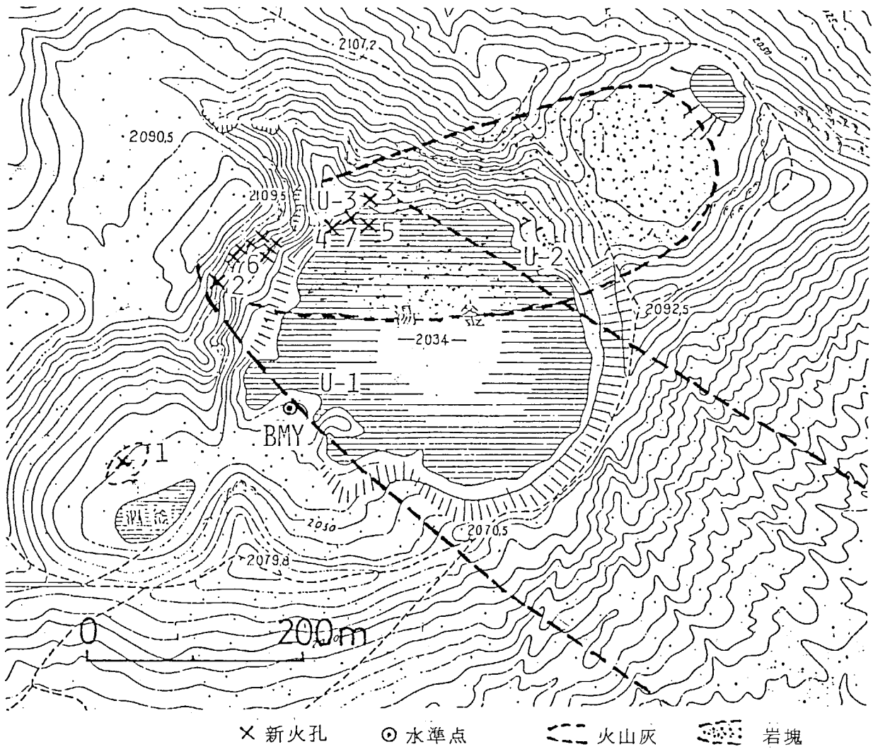
図4-12 1982年10月26日の噴火による山頂付近における固形噴出物の分布範囲と新火孔
