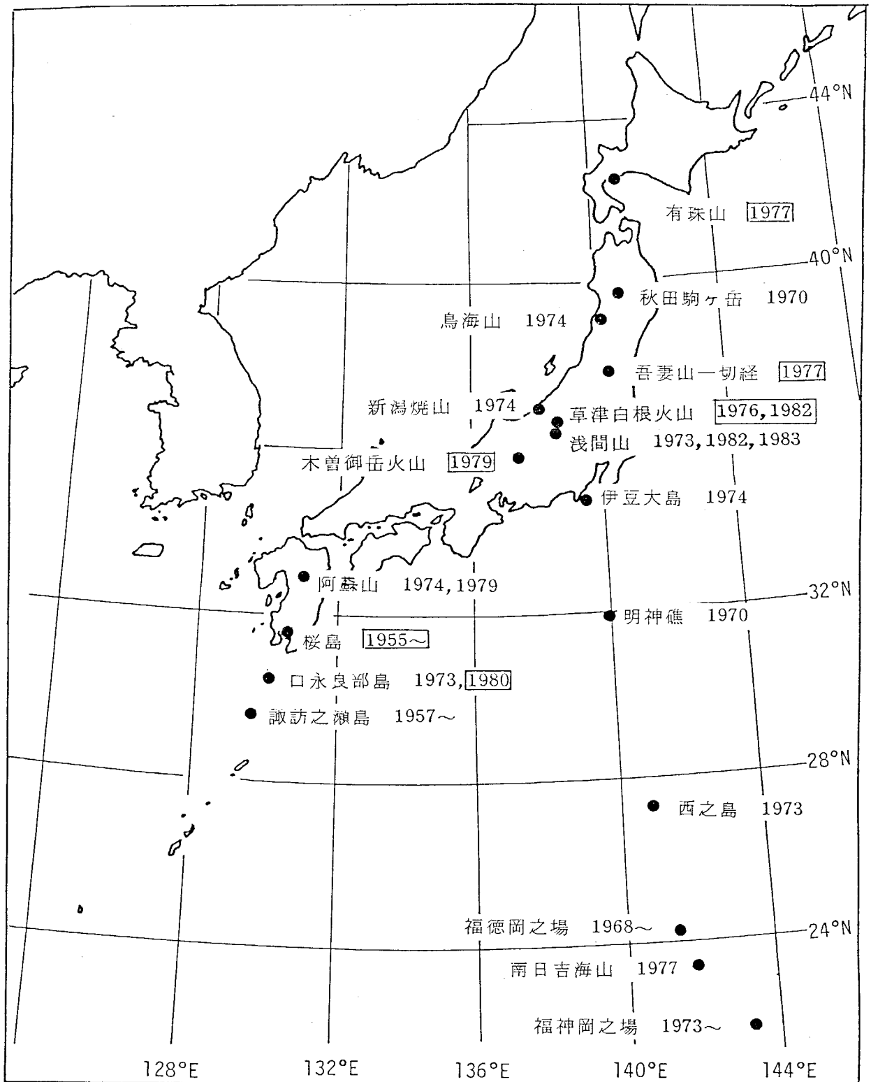
図1-1 1970年以降噴火した火山(●印), および本研究で対象とした火山(□印)
