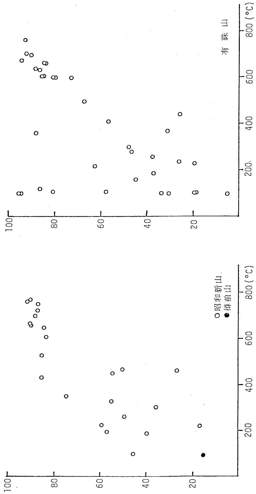
図2-4a 噴気孔温度とH 2 含有量
