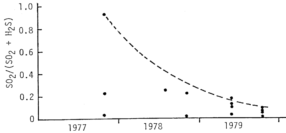
図5-6 噴気孔カスの \text{SO}_2/(\text{SO}_2 + \text{H}_2\text{S}) の変化
