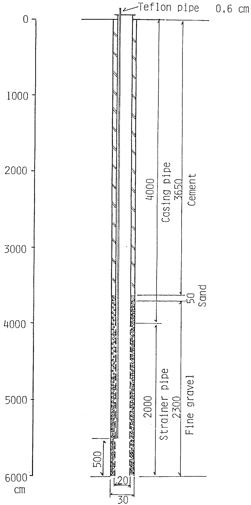
図3-19 ホーリング孔 (A孔) の断面図
