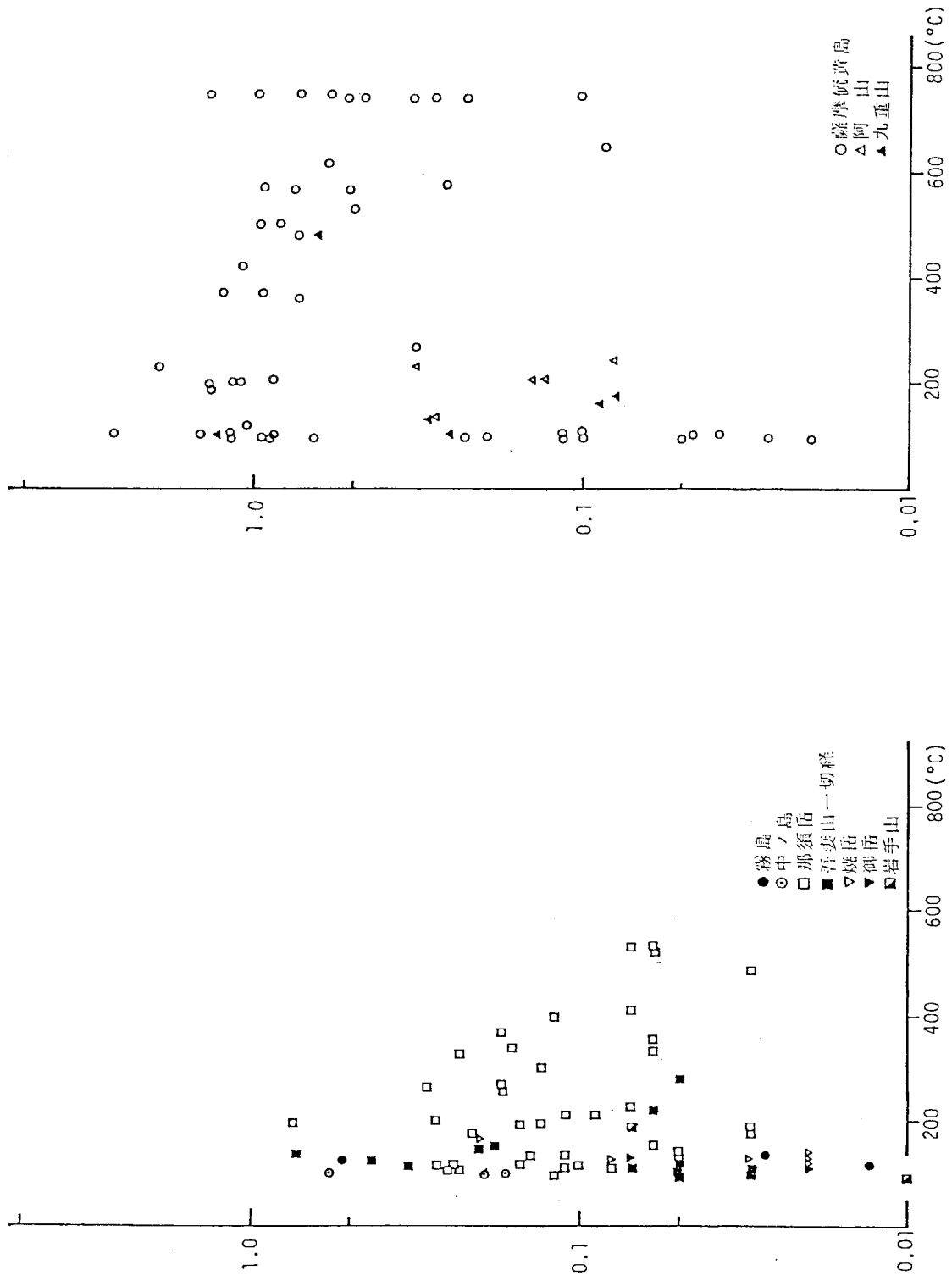
図2-2a 噴気孔温度と HCl/(SO_2 + H_2S)
