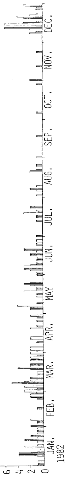
図3-21 A3LにおけるH 2 , Heの日変化と日別爆発回数
