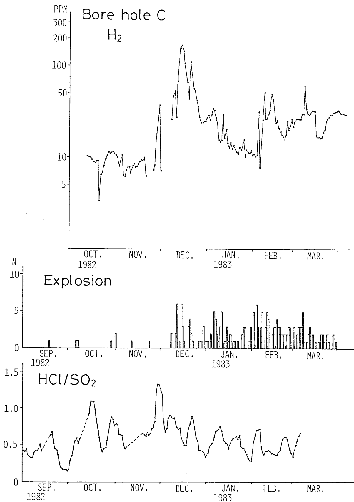
図3-22 C孔における H_2 の日変化と日別爆発回数 および 春田山における大気中カスの HCl/SO_2 の日変化
