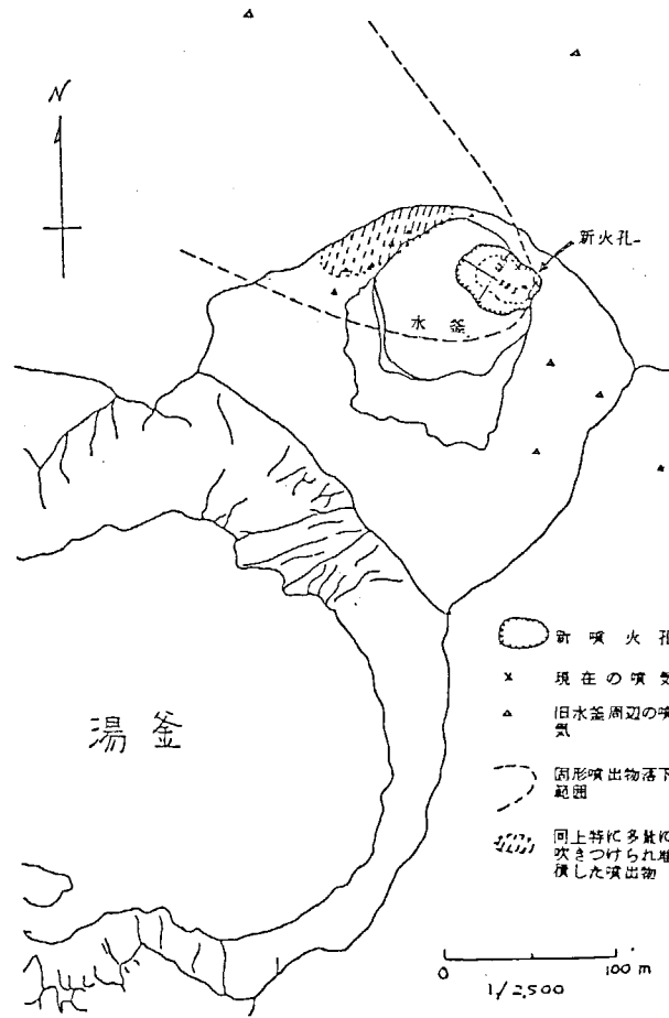
図4-10 草津白根火山水釜付近および 1976年噴火の新火孔および噴出物の 分布範囲
