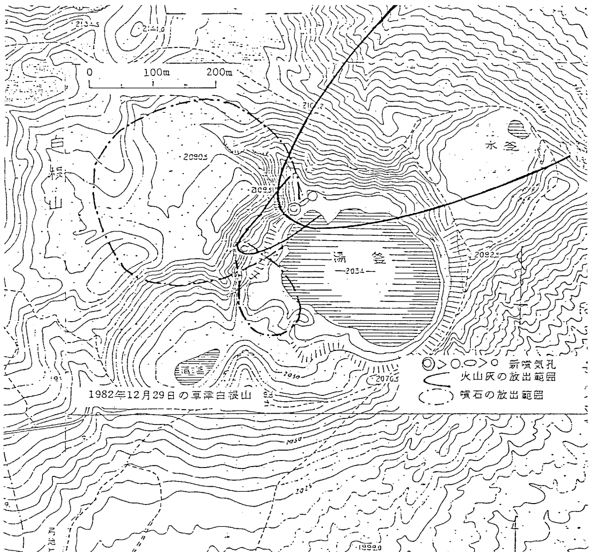
図4-14 1982年12月29日の噴火で放出された円形噴出物の分布範囲
