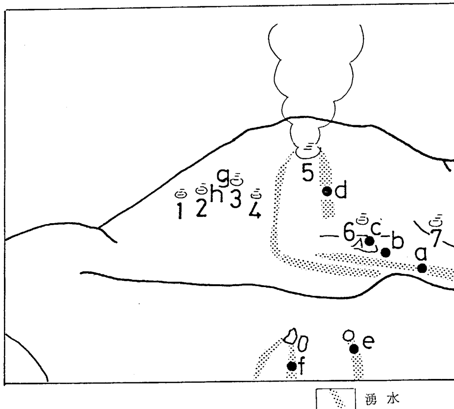
図5-5 吾妻火山一切経山大穴付近山頂見取図
