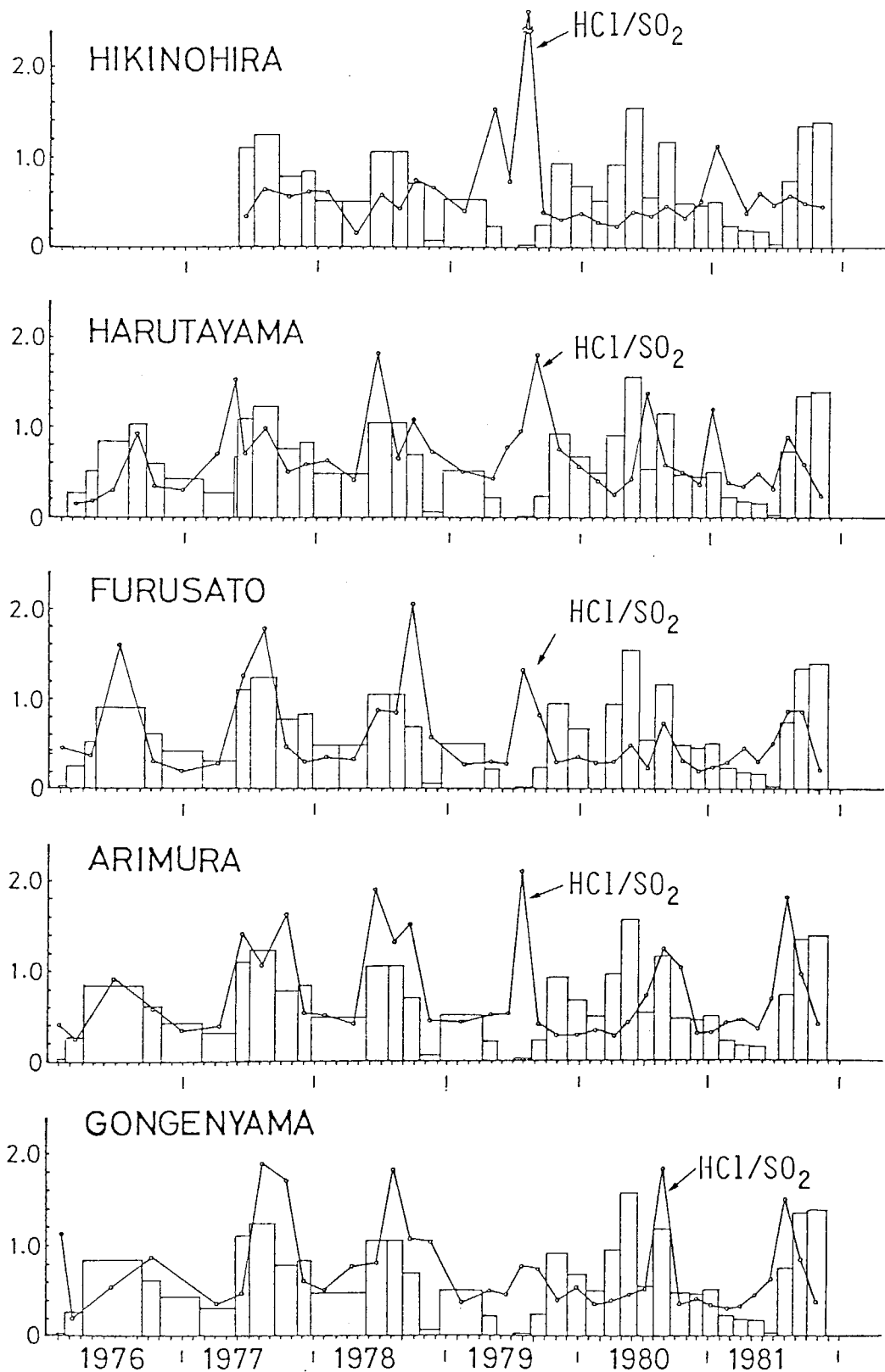
四 3-10 各観測点における \text{HCl}/\text{SO}_2 とアルカリ吸収液設置 期間ごとの日平均爆発回数
