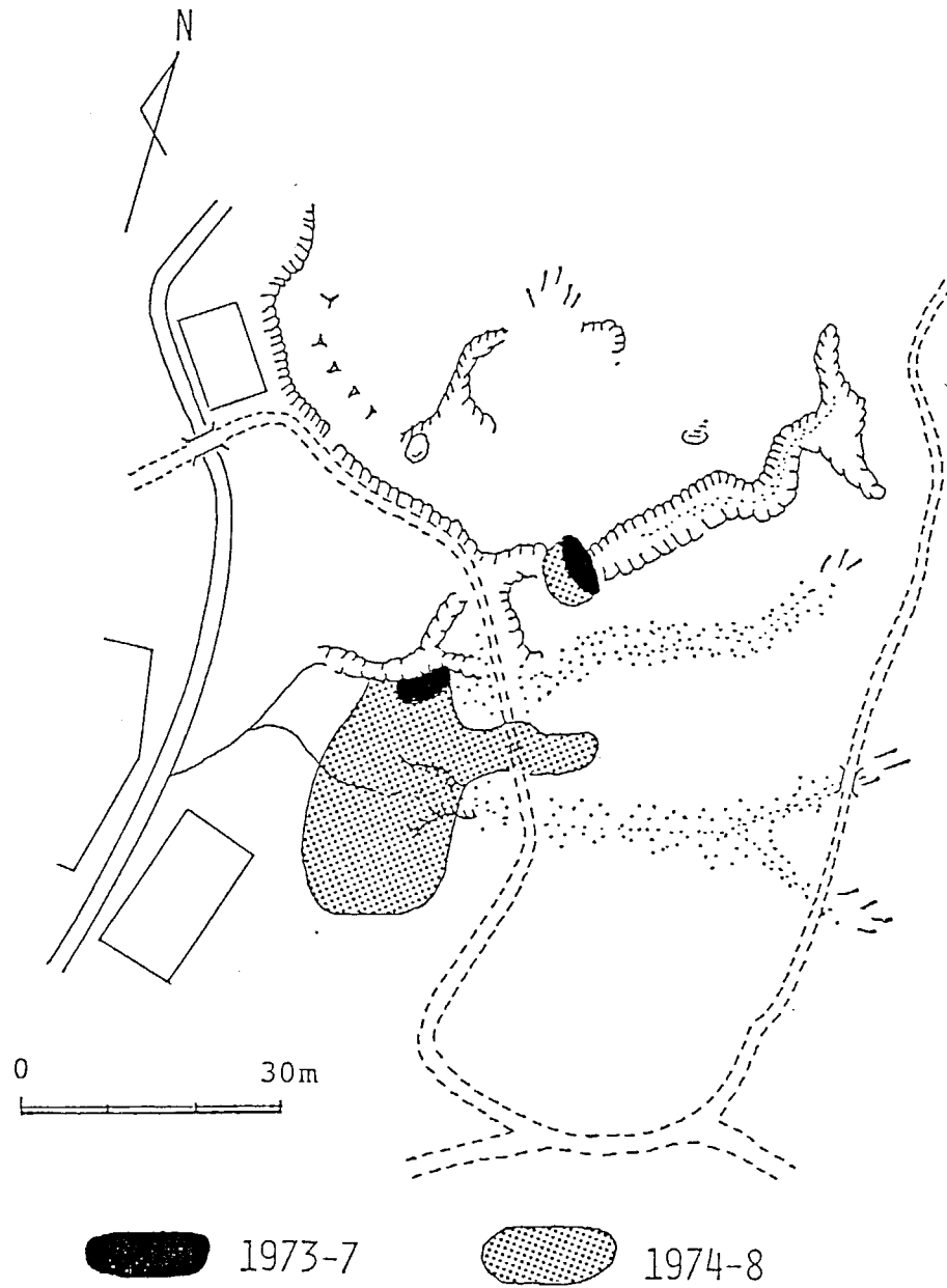
図3-8 万座地域における H_2S 高濃度分布範囲
