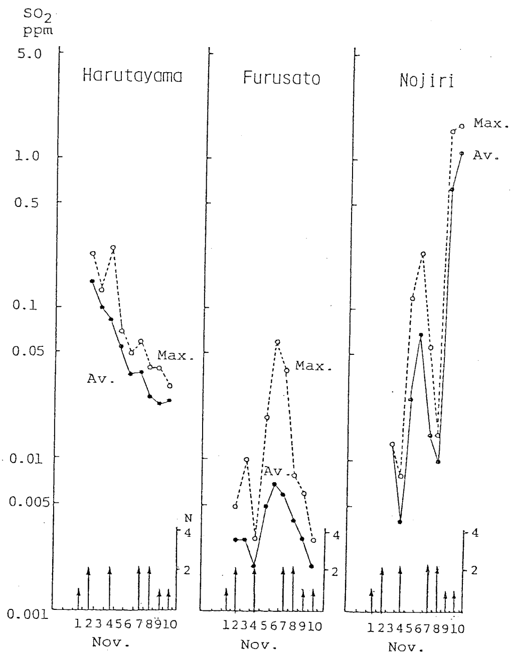
図3-13 春田山，古里，野尻の3観測点における同時連続 観測による大気中のSO 2 濃度の日変化と日別爆発回数
