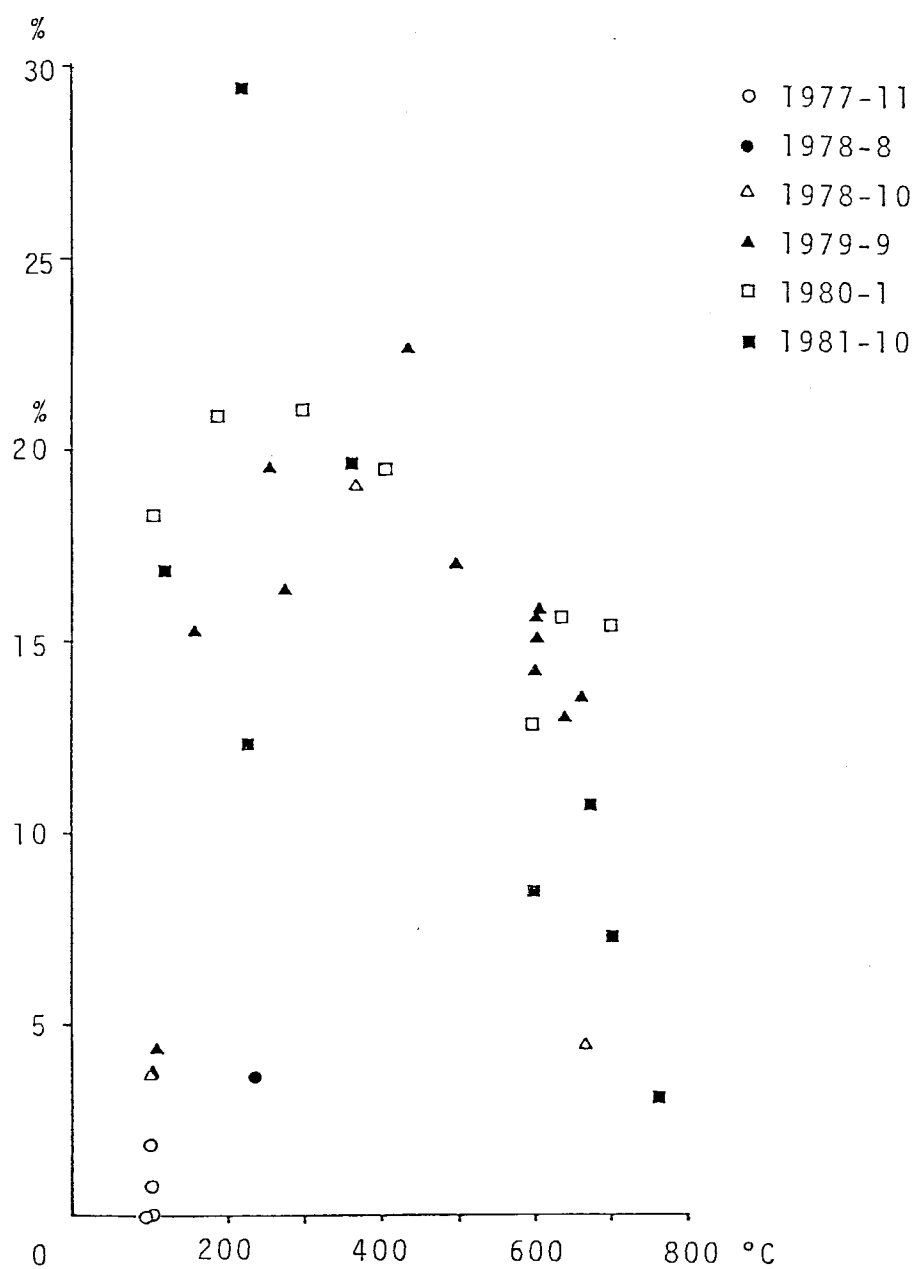
図5-12 噴気孔温度とH 2 S含有量
