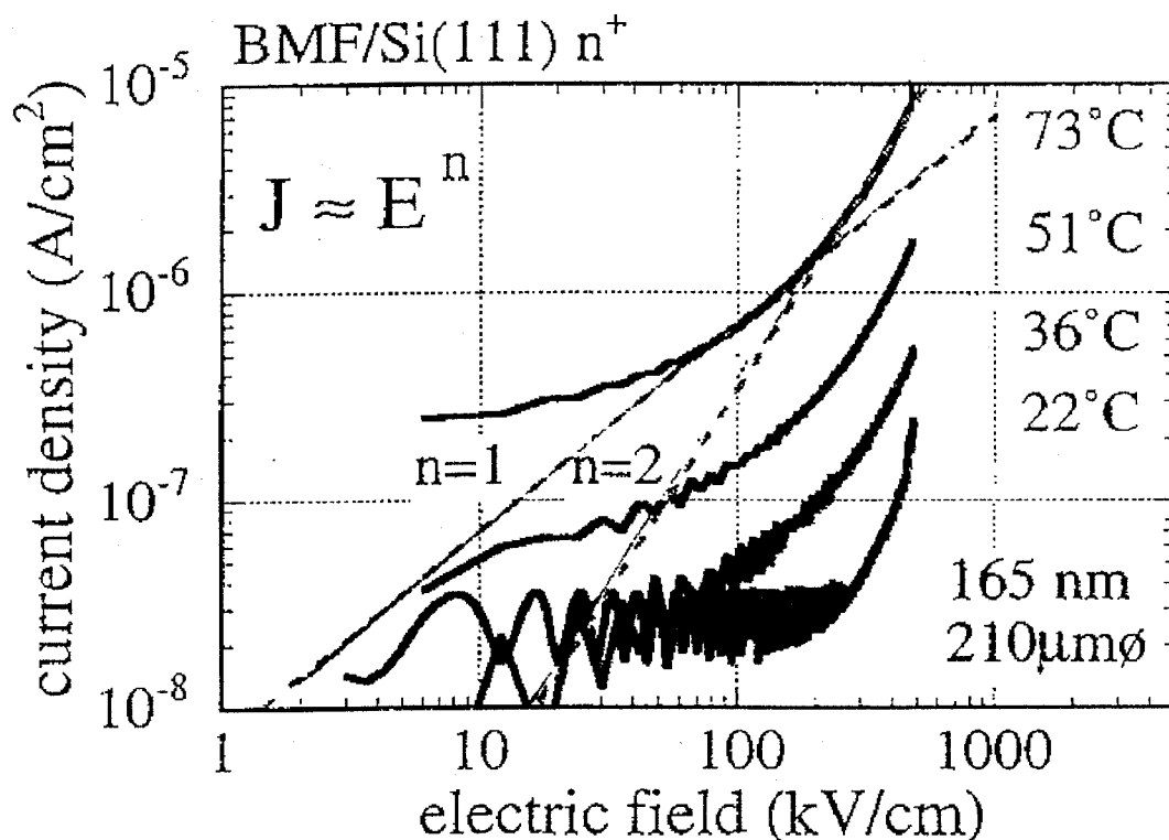
図 5-17 各測定温度 ( 22^\circ\text{C} 、 36^\circ\text{C} 、 51^\circ\text{C} 、 73^\circ\text{C} ) に対する J - E 特性
