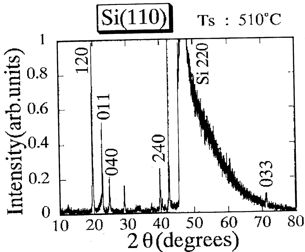
図 4-28 MBE 法を用いて Si (110) 基板上に基板温度 510°C で堆積した BaMgF 4 膜の X 線回折パターン。
