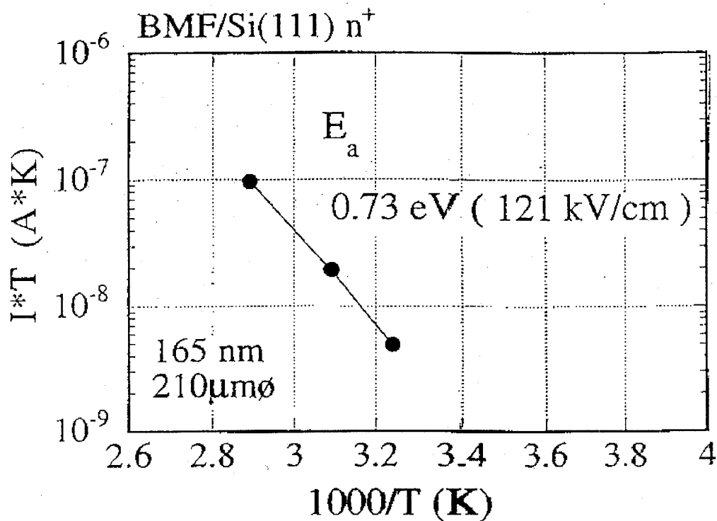
図 5-20 電界強度 121 \text{ kV/cm} における電流密度 J と測定温度 T との積 ( J \times T ) の測定温度に対するアレニウスプロット。
