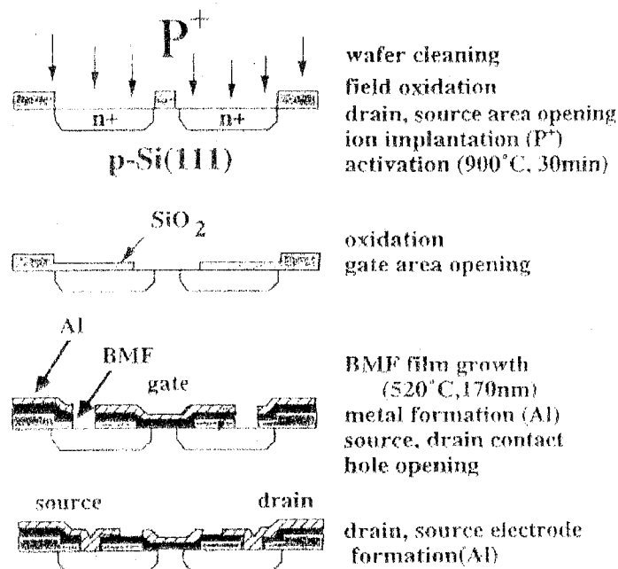
図5-37 BaMgF 4 /p-Si(111)構造によるnチャネル電界効果トランジスタの作製手順
