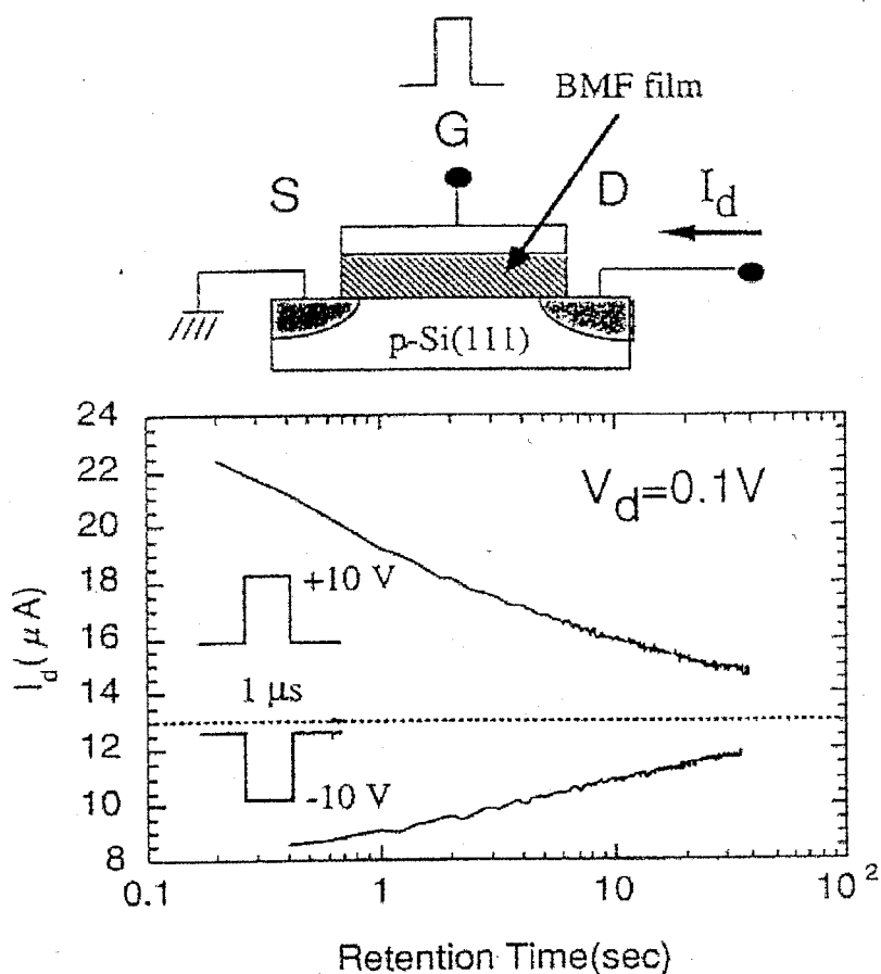
図 5-41 作製した電界効果トランジスタのゲート電極に幅 1ms、電圧 \pm 10\text{V} の単一のパルス電圧を印加した後に V_d = 0.1\text{V} および V_g = 0\text{V} に保持した状態で測定したドレイン電流 I_d の時間変化（記憶保持特性）。点線はパルス電圧を印加する前の初期状態でのドレイン電流の値である。
