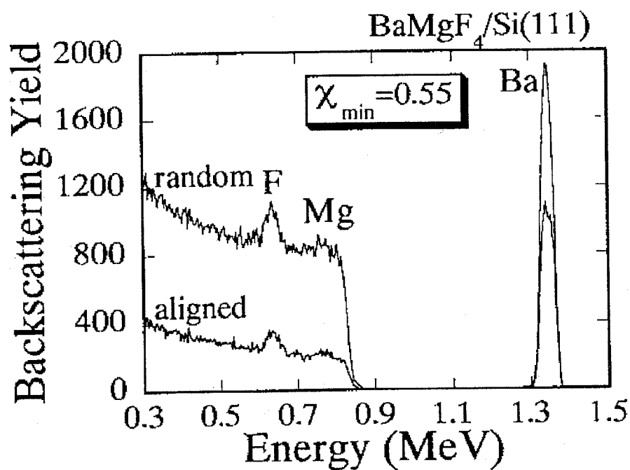
図 4 - 1 9 S(111) 基板上に BaMgF 4 膜を 510°C で堆積した試料の RBS スペクトル。
