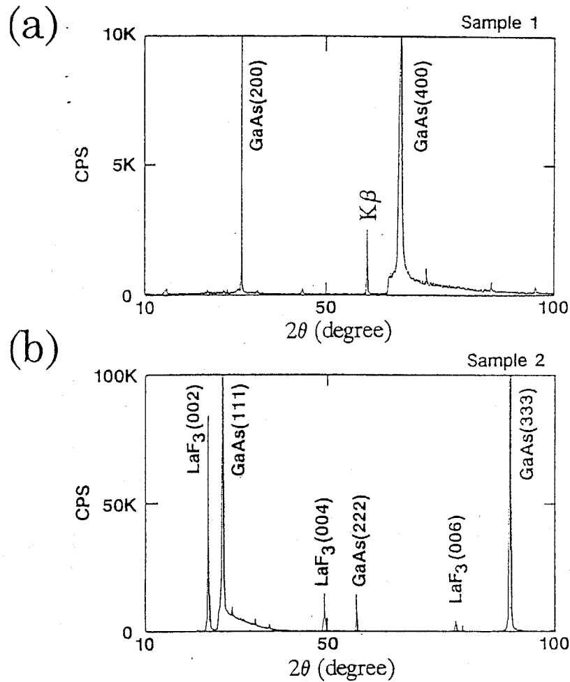
図 3-4 GaAs 基板上の LaF 3 膜の X 線回折パターン (a) LaF 3 /GaAs(100) の試料、(b) LaF 3 /GaAs(111)B の試料
