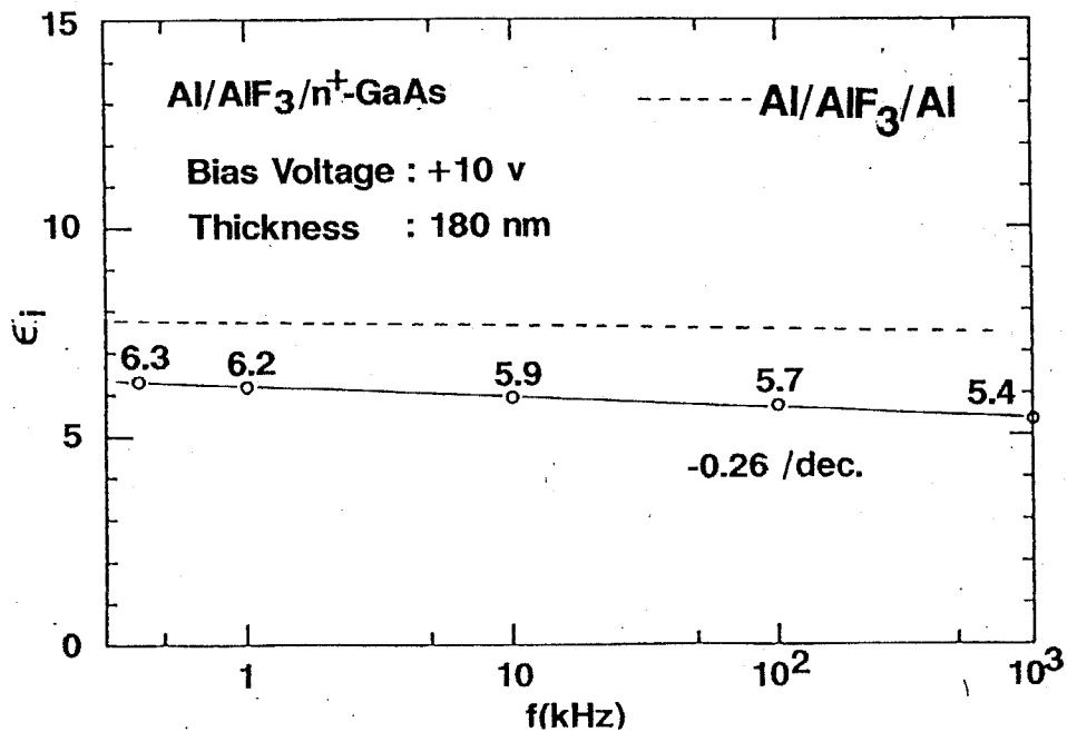
図 2-4 Al/AlF 3 /n + -GaAs(100)構造における AlF 3 膜の比誘電率の周波数特性
