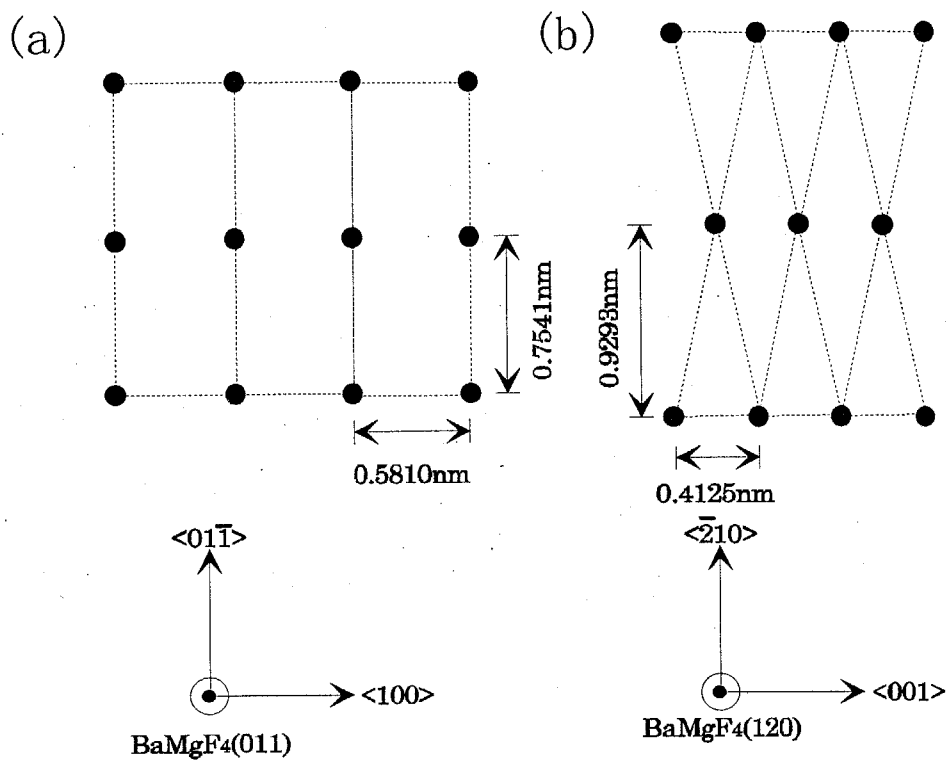
図 4-26 Mg 格子点における、(a) \text{BaMgF}_4(011) 面および (b) \text{BaMgF}_4(120) 面の格子構造図。
