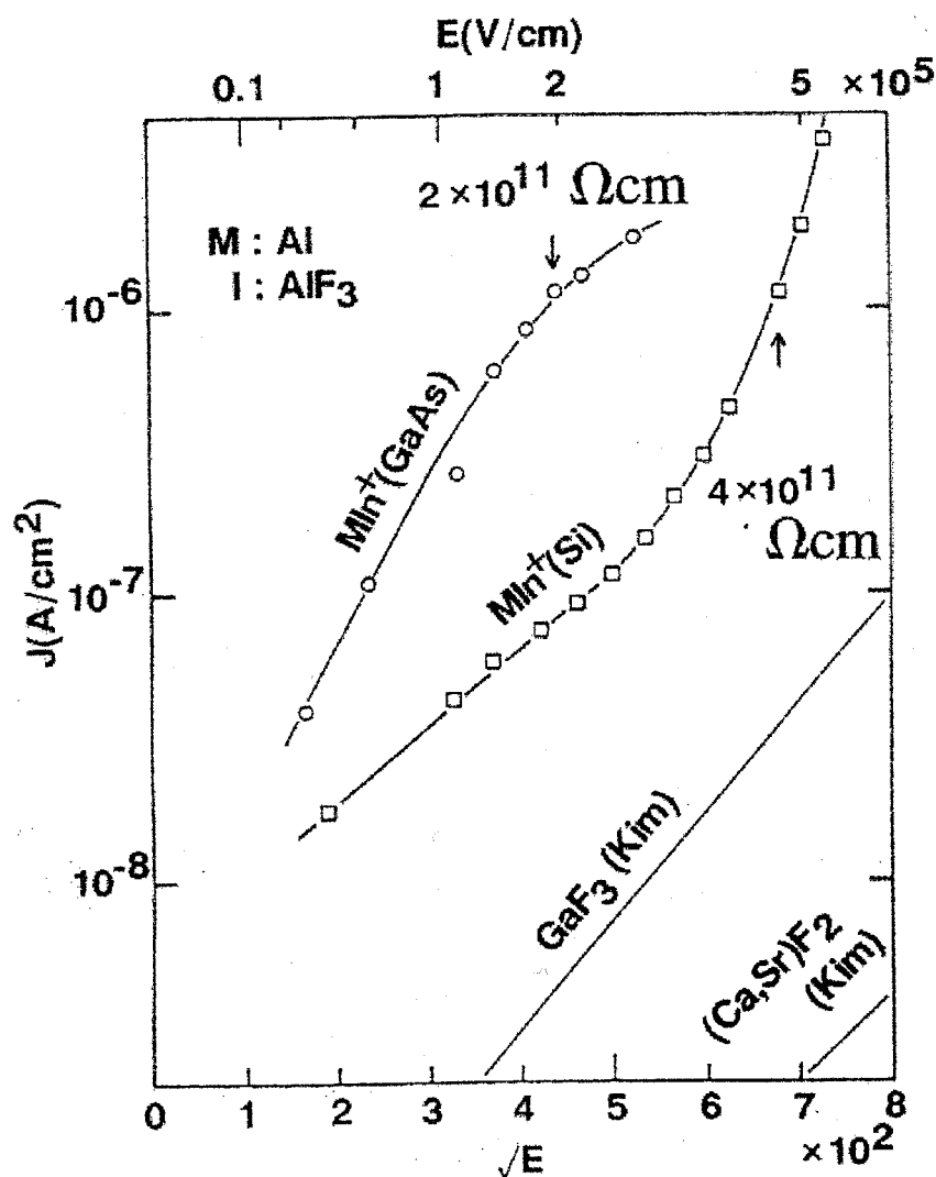
図 2-3 \text{AlF}_3 膜の \sqrt{E} - J 特性
