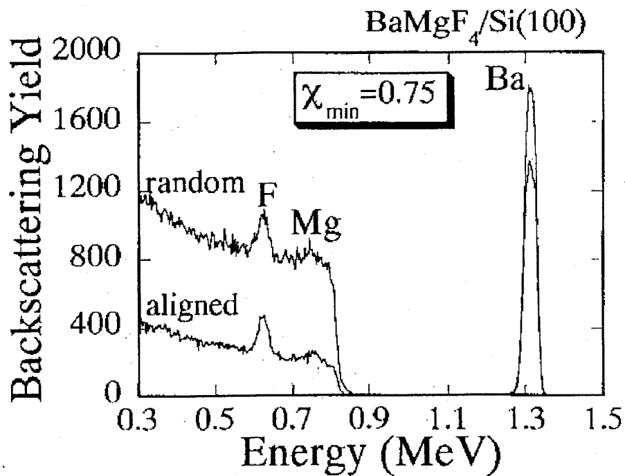
図 4 - 1 8 S(100) 基板上に BaMgF 4 膜を 510°C で堆積した試料の RBS スペクトル。
