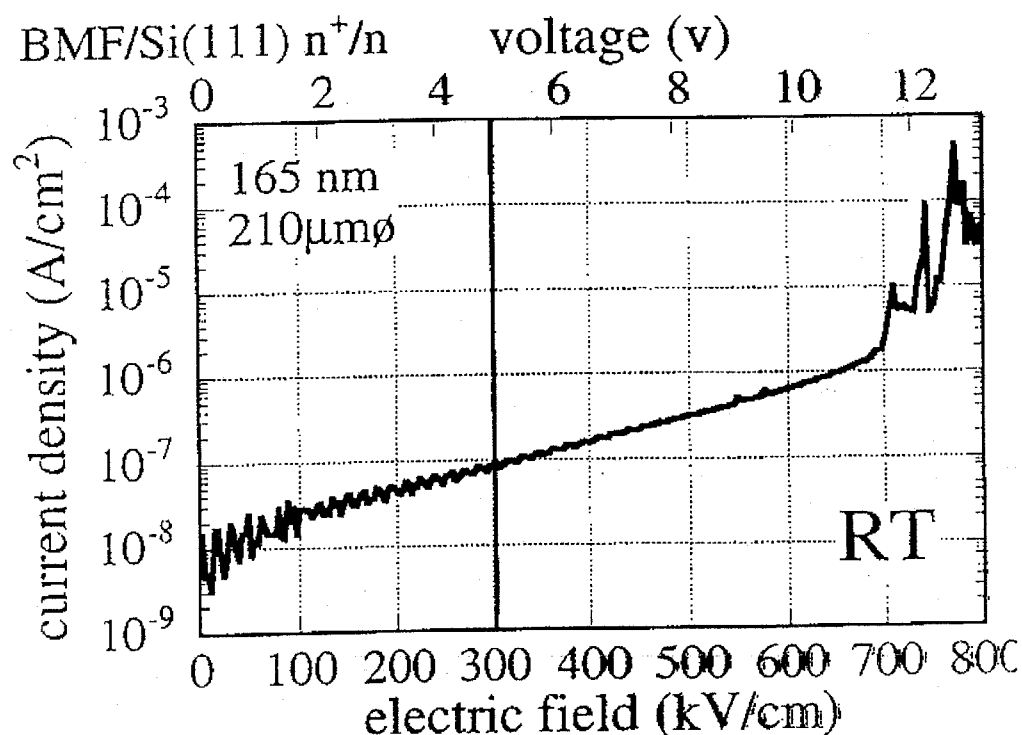
図 5-16 Si (111) 基板上に成長した BaMgF 4 (120) 配向膜 (試料 2) の室温 (300K) における漏れ電流特性
