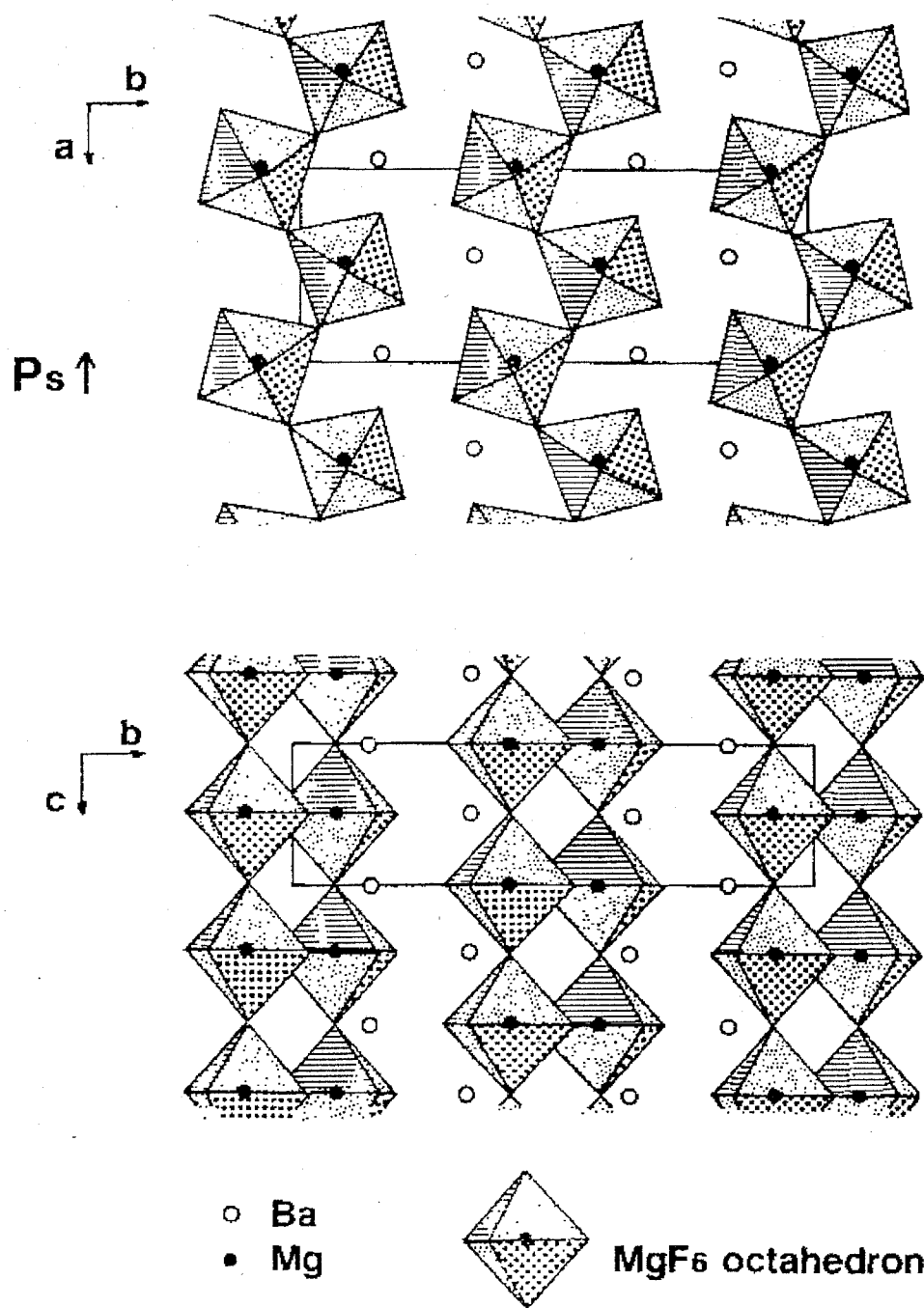
図4-25 \text{BaMgF}_4 の結晶構造。図中の \circ はBa格子点、 \bullet はMg格子点、 \text{MgF}_6 八面体の頂点はそれぞれFの格子点となっている。また四角枠は \text{BaMgF}_4 結晶のユニットセルを表している。
