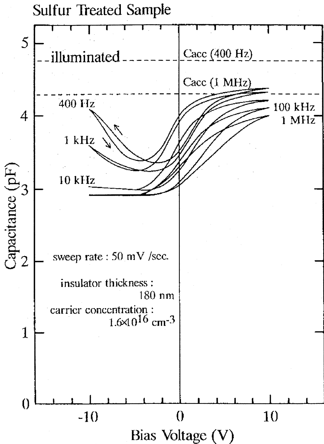
図 2 - 6 硫黄処理した Al/AlF 3 /GaAs(100) 構造 ダイオードの光照射下における C-V 特性
