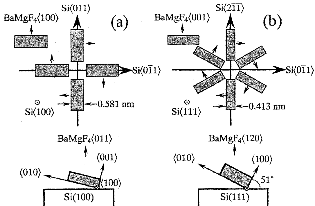
図4-24 Si基板上に成長したBaMgF 4 膜のエピタキシャル方位関係。(a)Si(100)基板上のBaMgF 4 (011)膜の場合、(b)Si(111)基板上のBaMgF 4 (120)膜の場合。
