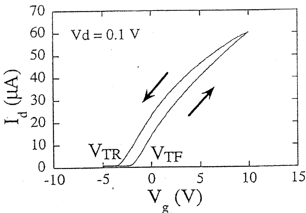
図5-40 作製した電界効果トランジスタの I_d - V_g 特性 ( V_d=0.1\text{V} )。ゲート電圧を 10V 印加した場合のしきい値電圧シフト V_{TF}-V_{TR} は約 1.4V。
