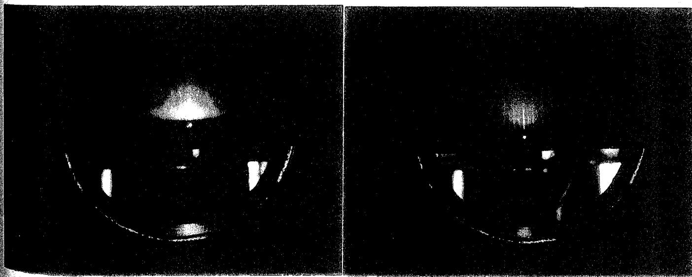
図4-21 Si(111)基板上に作製した試料に対する RHEED 像。電子線の入射方向は \langle 112 \rangle 方向。(a)は BaMgF 4 膜堆積前の RHEED 像、(b)は BaMgF 4 膜堆積後の RHEED 像。
