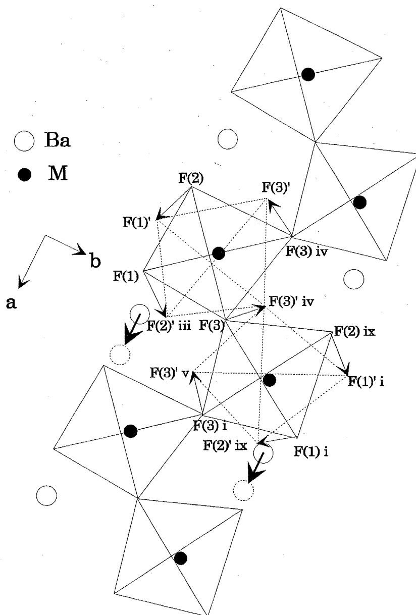
図 4-2 \text{BaMF}_4 の結晶構造と分極の機構
