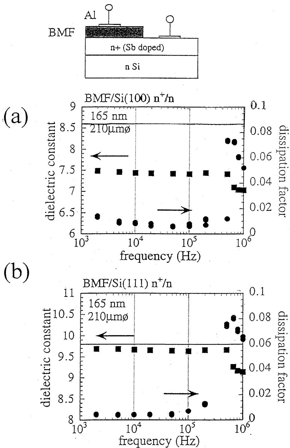
図5-15 Si 基板上に成長した BaMgF 4 配向膜における比誘電率および誘電損失( \tan\delta )の周波数分散特性。
