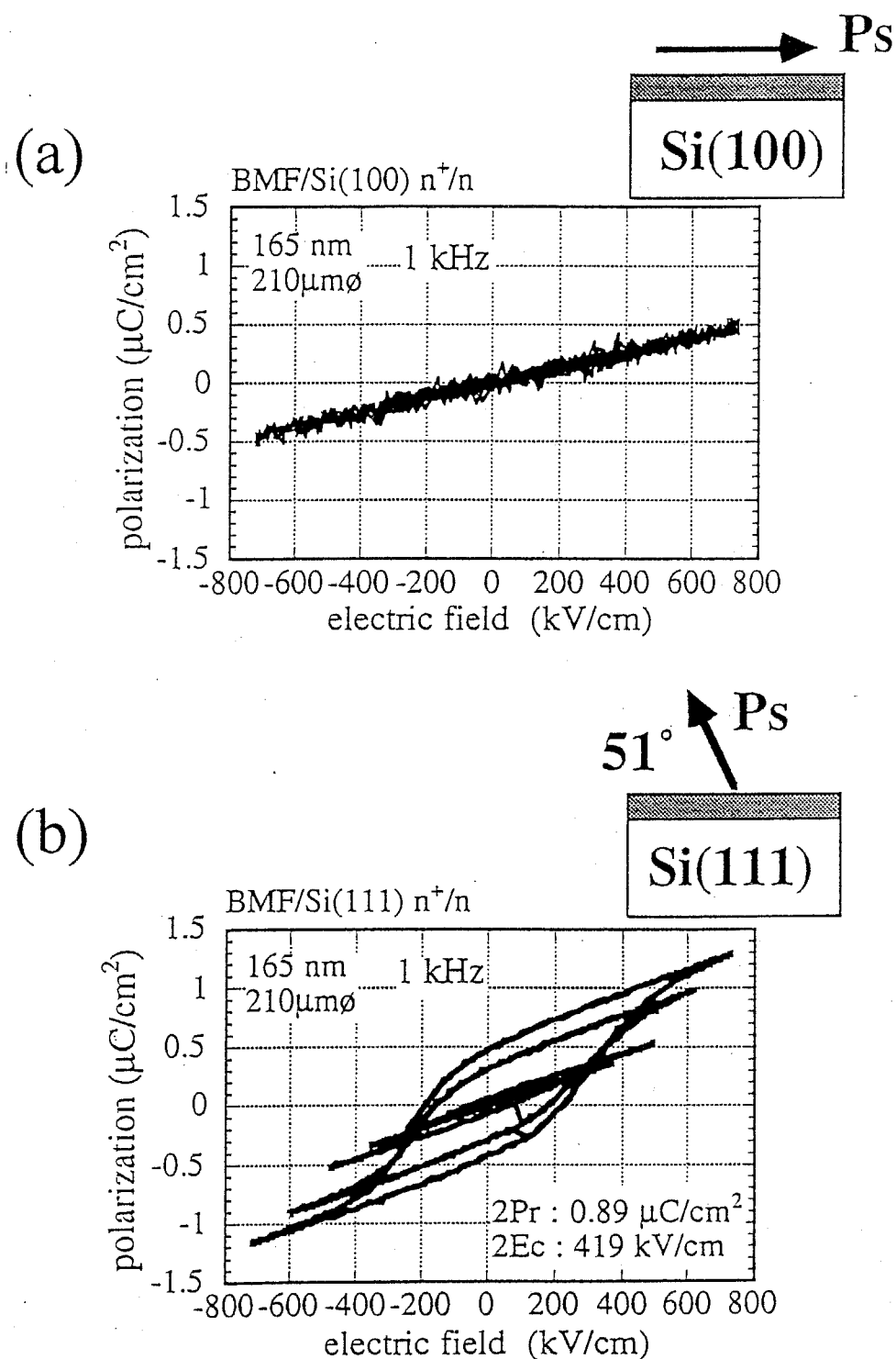
図 5 - 2 2 (a) Si(100)に成長した \text{BaMgF}_4(011) 配向膜 (試料 1) および、(b) Si (111) 基板上 に成長した \text{BaMgF}_4(120) 配向膜の試料 (試料 2) の 1kHz D - E 特性。図中の試料断面図にある矢印は \text{BaMgF}_4 膜中での分極ベクトルの方向を示す。
