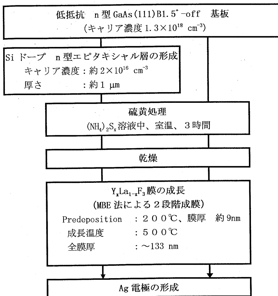
図 3-18 Ag/ \text{Y}_x\text{La}_{1-x}\text{F}_3 /GaAs(111)B MIS ダイオードの作製プロセス
