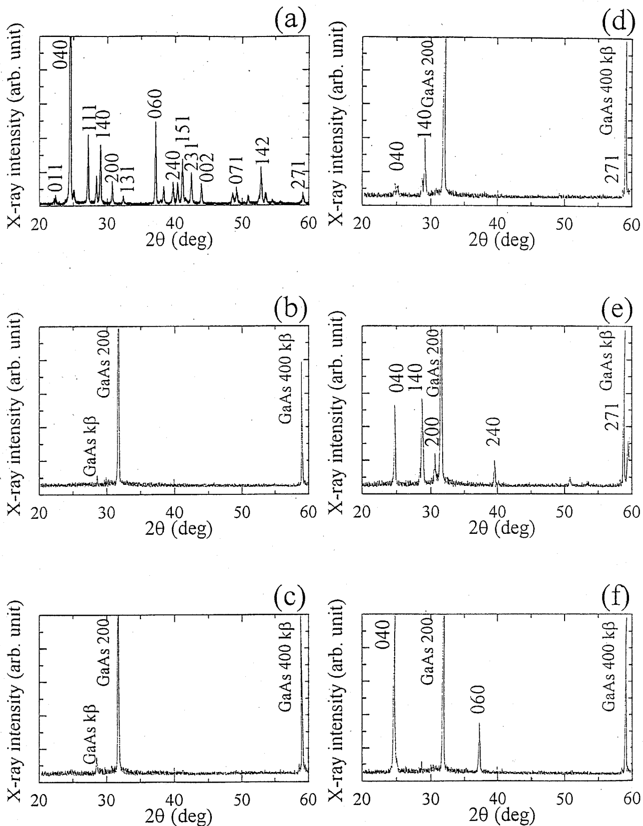
図4-8 GaAs(100)基板上に \text{BaMgF}_4 膜を形成した試料におけるX線回折パターン。(a) : 蒸着源として用いた \text{BaMgF}_4 多結晶のX線回折パターン。(b), (c), (d)および(e) : それぞれ成膜時の基板温度を 300^\circ\text{C} 、 400^\circ\text{C} 、 500^\circ\text{C} 、 600^\circ\text{C} とした場合のX線回折パターン。(f) : 基板温度 300^\circ\text{C} で膜を堆積した後、真空を破らずに続けて 600^\circ\text{C} 、30分の熱処理を行った場合のX線パターン。
