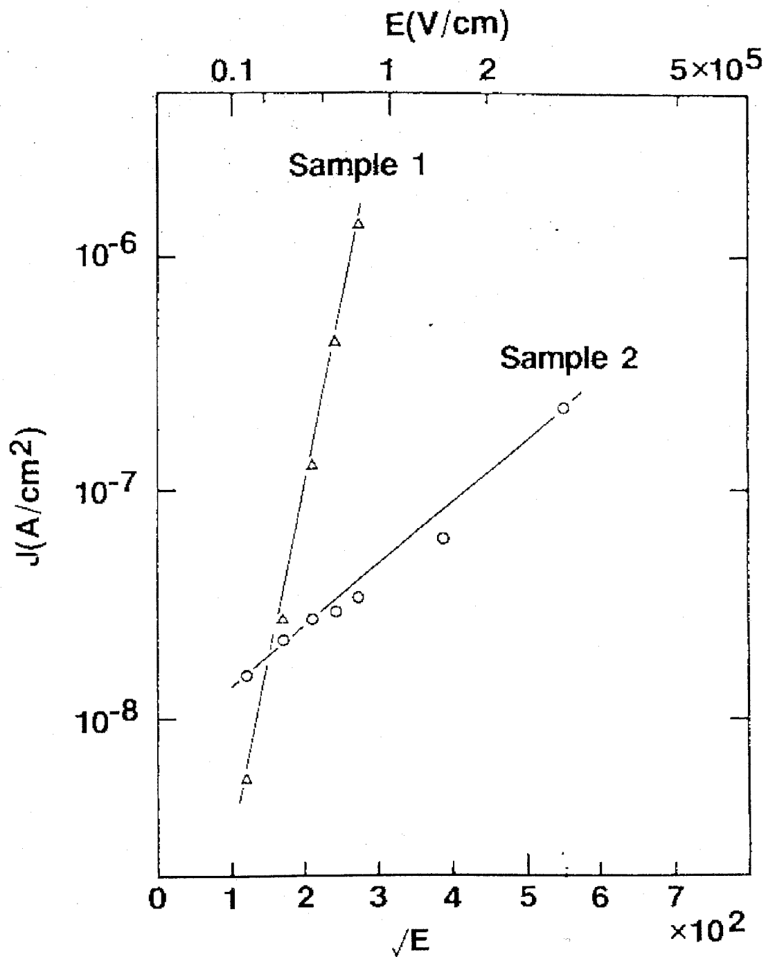
図 3-5 GaAs 上に成膜した LaF 3 膜の漏れ電流特性 [Frenkel-Pool プロット( \sqrt{E} - J )] Sample 1: LaF 3 /GaAs(100) の試料、 Sample 2: LaF 3 /GaAs(111)B の試料
