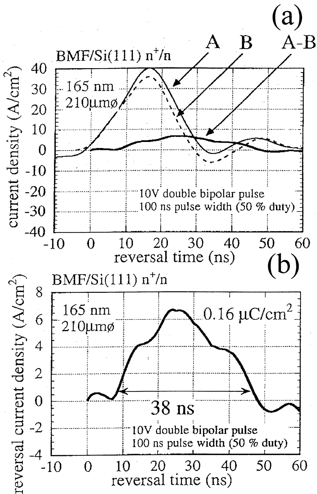
図 5 - 2 5 (a) Si(111) 基板上に成長した \text{BaMgF}_4 (120) 膜のパルス応答波形、(b) 分極反転電流のパルス応答波形
