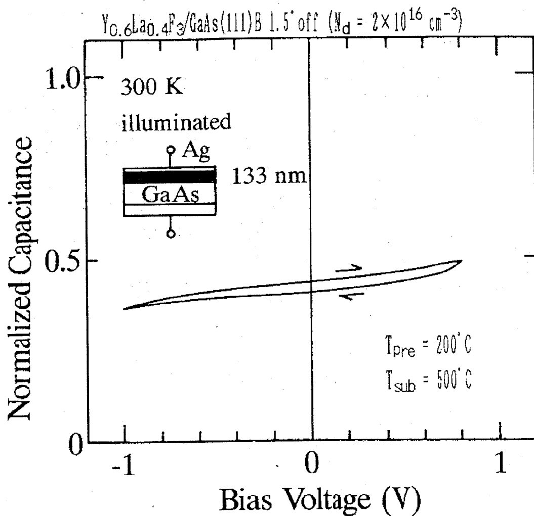
図 3 - 1 9 Ag/ \text{Y}_{0.6}\text{La}_{0.4}\text{F}_3 /GaAs(111)B MIS ダイオードの 1MHz C-V 特性
