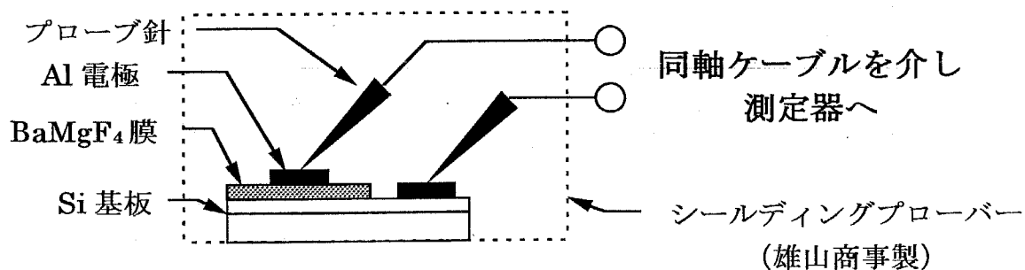
図 5-14 試料測定 of 概略図
