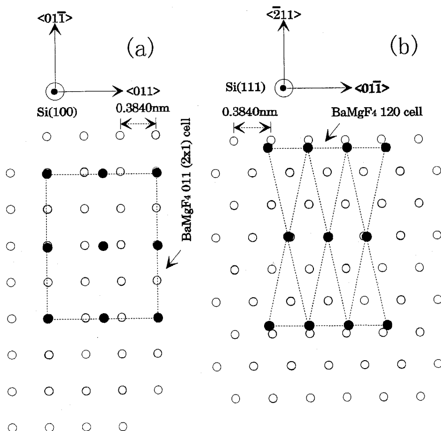
図 4-27 (a) \text{Si}(100) および (b) \text{Si}(111) 最表面での格子構造図。図中 (a) および (b) の点線は \text{BaMgF}_4(011) 面における 2 \times 1 セルおよび \text{BaMgF}_4(120) 面におけるユニットセルを示す。
