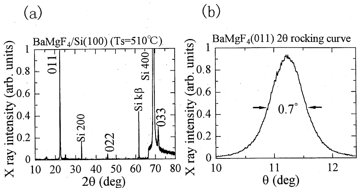
図4-14 Si(100)基板上に 510°Cで作製した試料 (試料 3) におけるX線回折測定の結果。(a)X線回折パターン、(b)BaMgF 4 (011)回折ピークの 2θ ロッキングカーブ。
