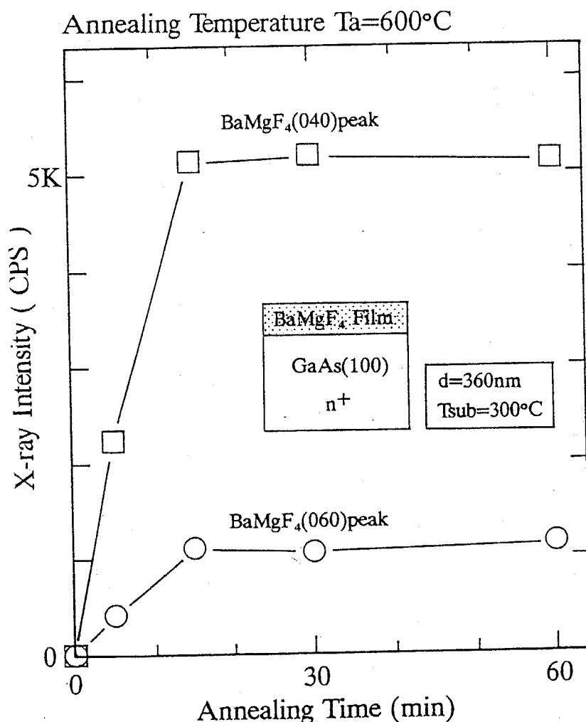
図4-9 基板温度 300^\circ\text{C} で堆積した膜厚 360\text{nm} の \text{BaMgF}_4 膜を真空中で 600^\circ\text{C} で熱処理した場合の \text{BaMgF}_4 (040) および (060) 回折ピークの熱処理時間依存性
