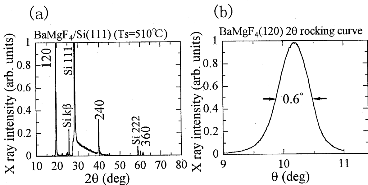
図4-15 Si(111)基板上に 510°Cで作製した試料 (試料 4) におけるX線回折測定の結果。(a)X線回折パターン、(b)BaMgF 4 (120)回折ピークの 2θ ロッキングカーブ。
