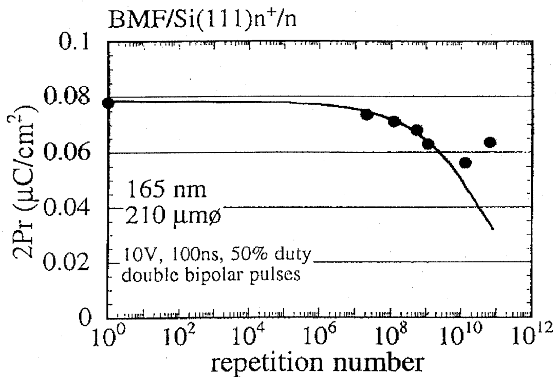
図 5 - 2 7 Si(111)基板上に成長した BaMgF 4 (120)膜の疲労特性
