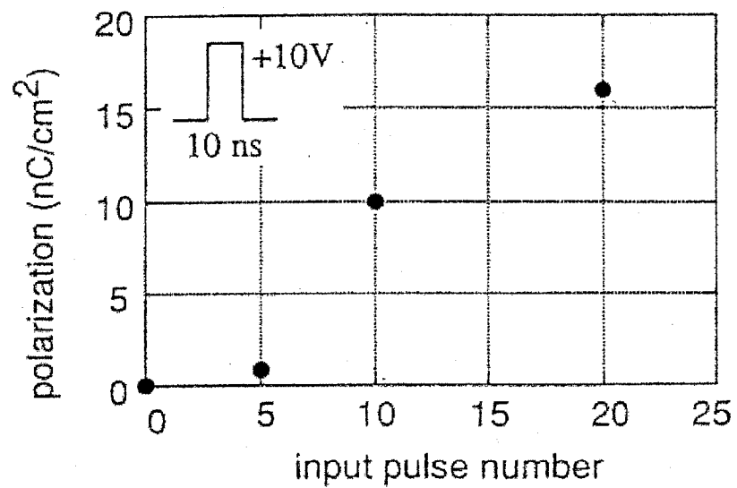
図5-45 入力パルス数に対する分極量の変化。入力パルスには電圧 +10\text{V} 、パルス幅 10\text{ ns} の単一パルスを用いて、 I_d - V_d 特性における飽和ドレイン電流から分極量を見積もった。
