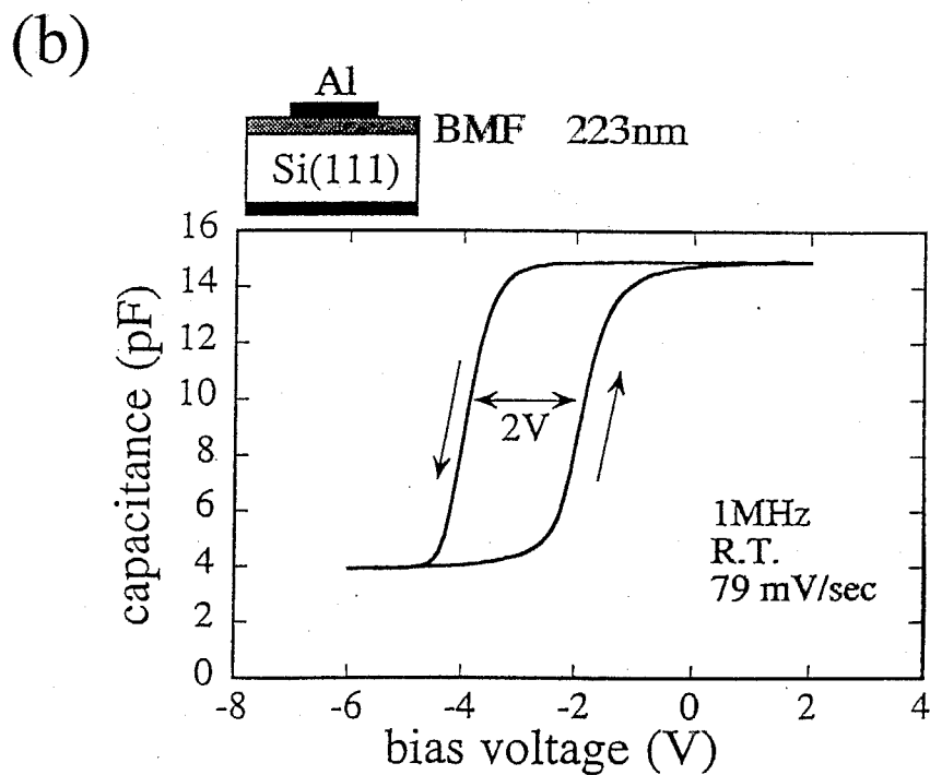
図 5 - 3 3 (a) Si(100) および (b) (111) 基板上に基板温度 500°C で BMF 膜を成長した BMF/Si 構造ダイオードの 1MHz C - V 特性
