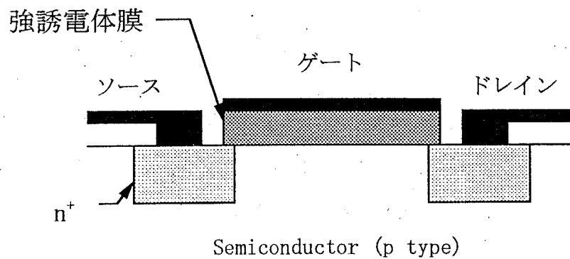
図 1 - 5 基本的な n チャンネル MFSFET の構造
