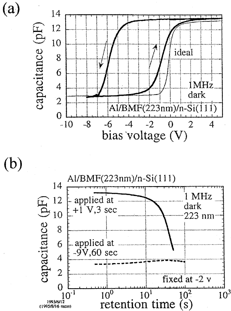
図5-42 (a) Al/BaMgF 4 /n-Si(111) ダイオードにおける 1MHz C - V 特性 (BaMgF 4 膜の厚さ 223nm) および (b) 電極にバイアス電圧 (+5V および -10V) を印加した後、一定のバイアス電圧 (ここでは -2.5V) で保持した場合における容量値の時間変化。
