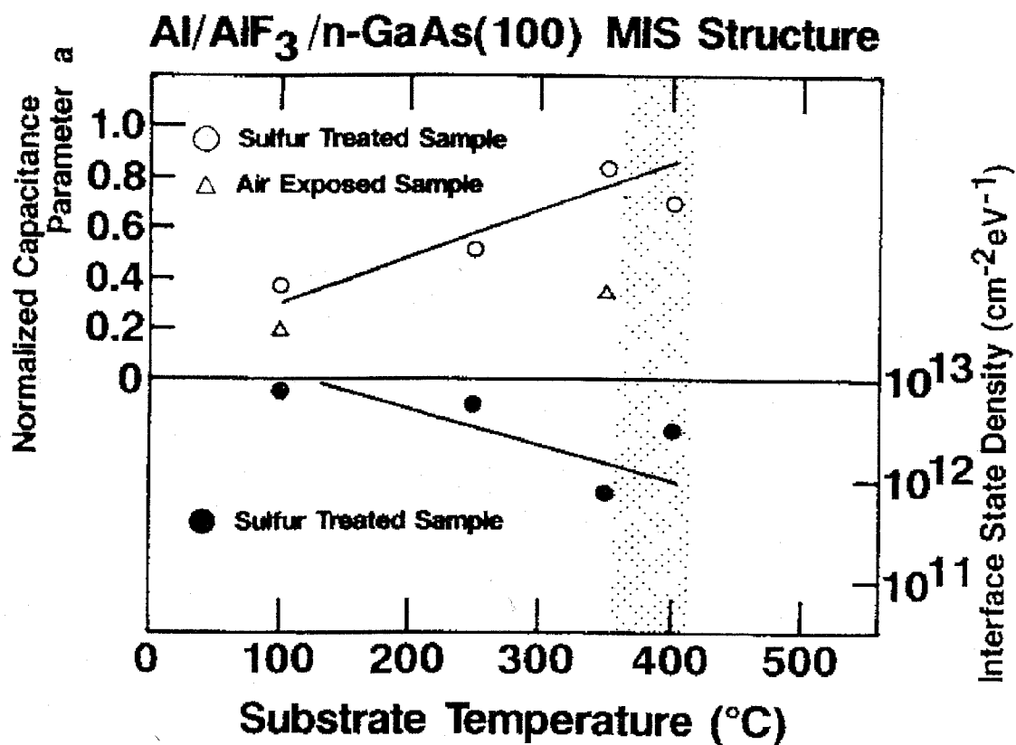
図 2-9 \text{AlF}_3 膜の形成温度に対する界面準位密度およびダイオード測定における規格化容量パラメータ a
