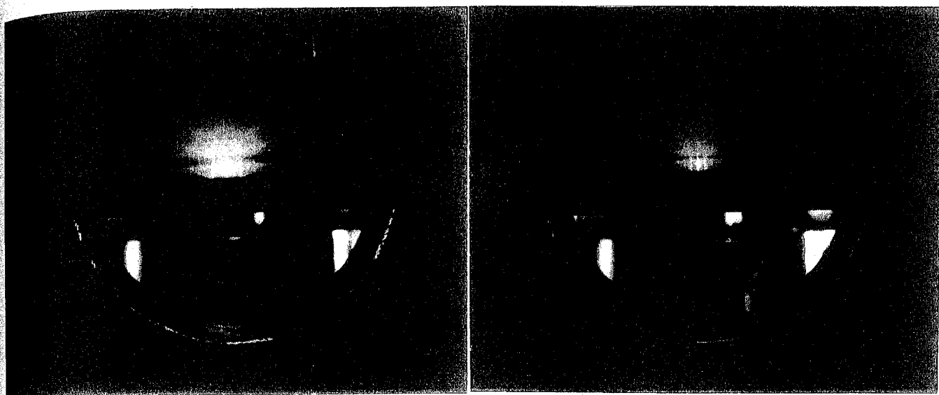
図4-20 Si(100)基板上に作製した試料に対する RHEED 像。電子線の入射方向は \langle 011 \rangle 方向。(a)は BaMgF 4 膜堆積前の RHEED 像、(b)は BaMgF 4 膜堆積後の RHEED 像。
