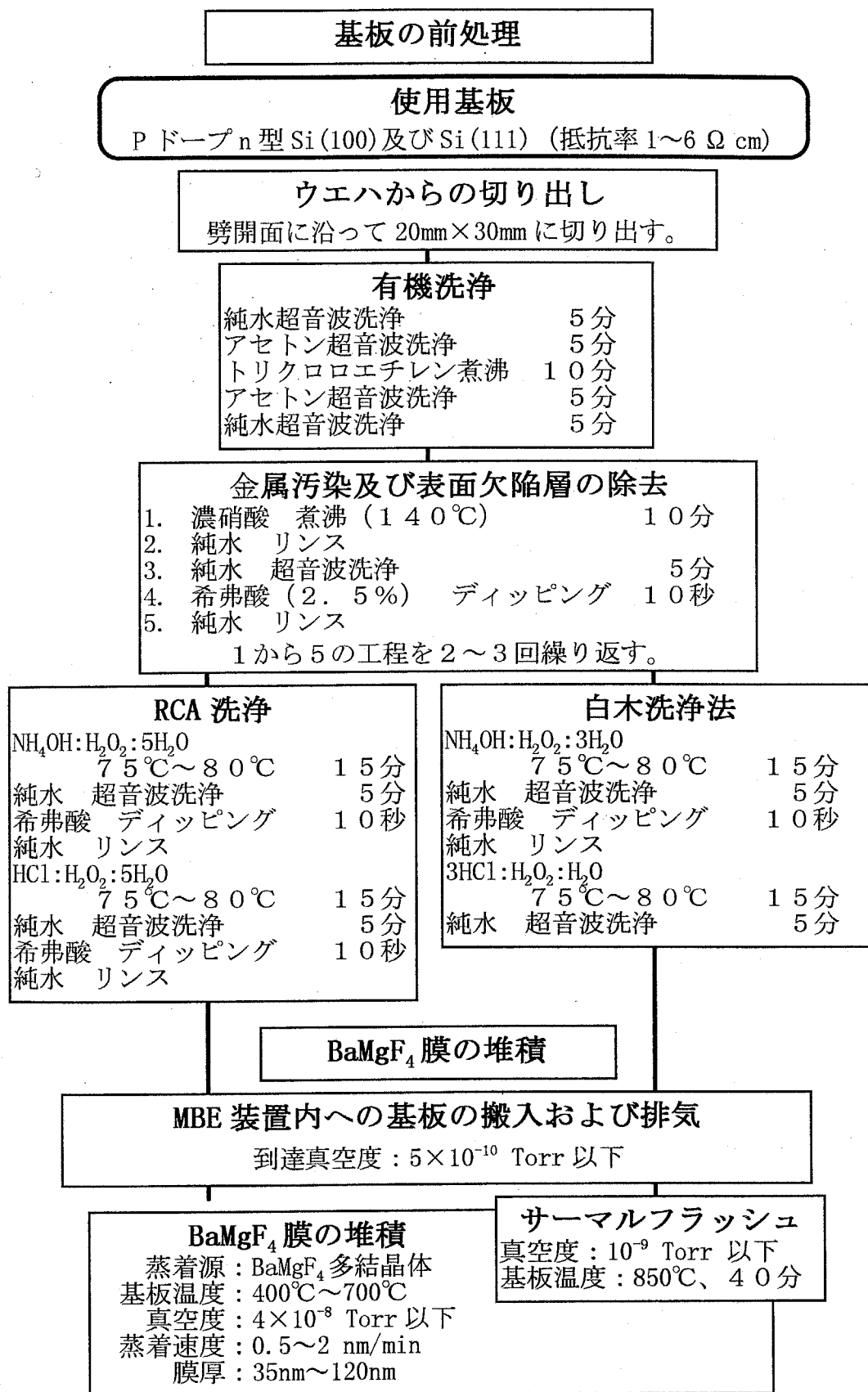
図 4-7 MBE 法による Si 基板上への BaMgF 4 膜形成工程
