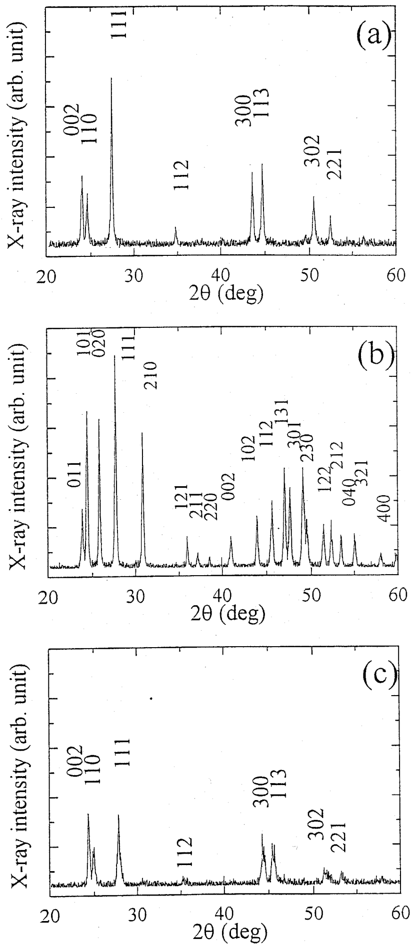
図3-3 蒸着原料のX線回折パターン (a) \text{LaF}_3 粉末、(b) \text{YF}_3 粉末 (c) (\text{Y,Lu})\text{F}_3 焼結体(Y:Lu=2:3)
