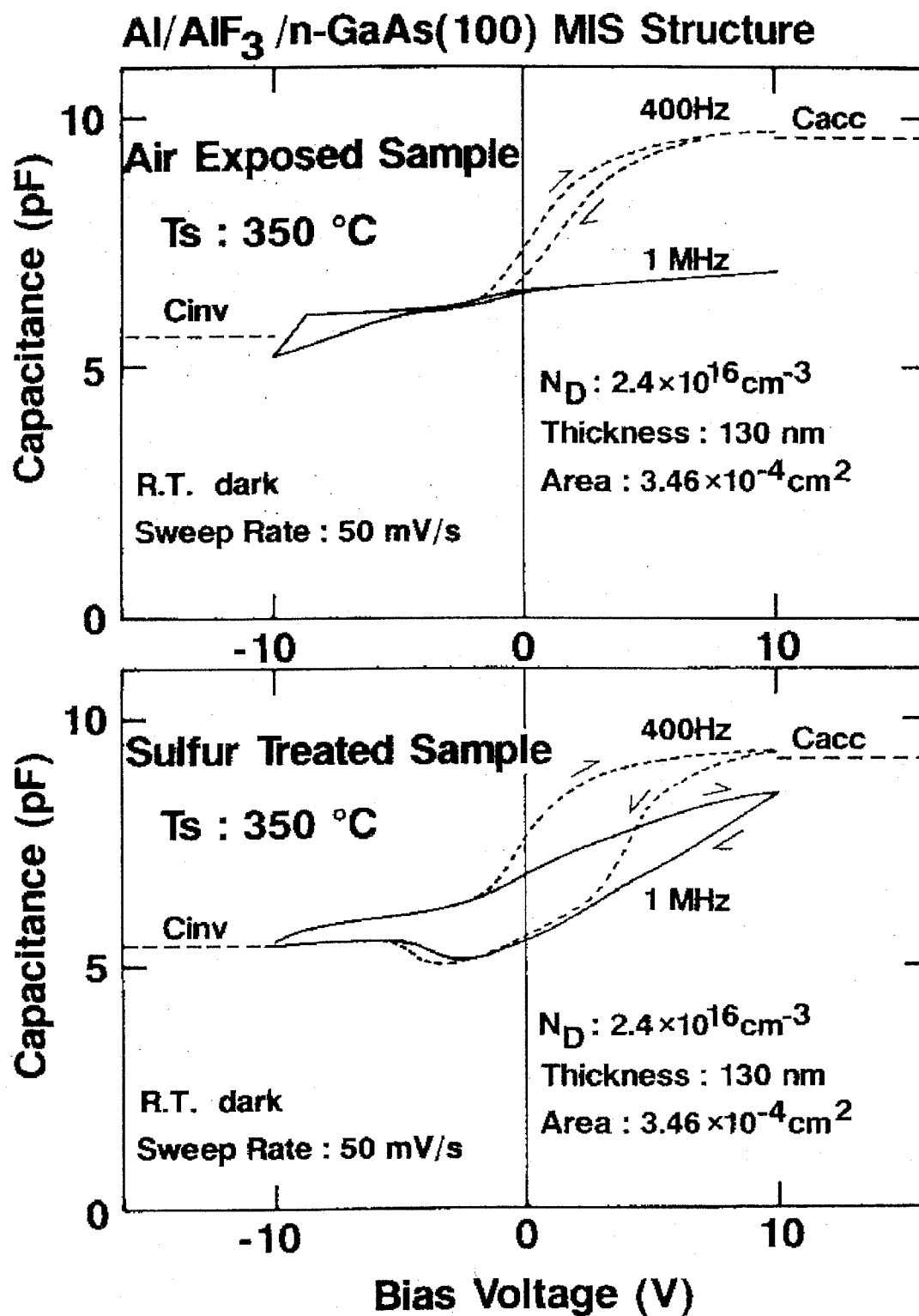
図 2-7 光照射をしない場合の Al/AlF 3 /GaAs(100) 構造ダイオードの C-V 特性。
