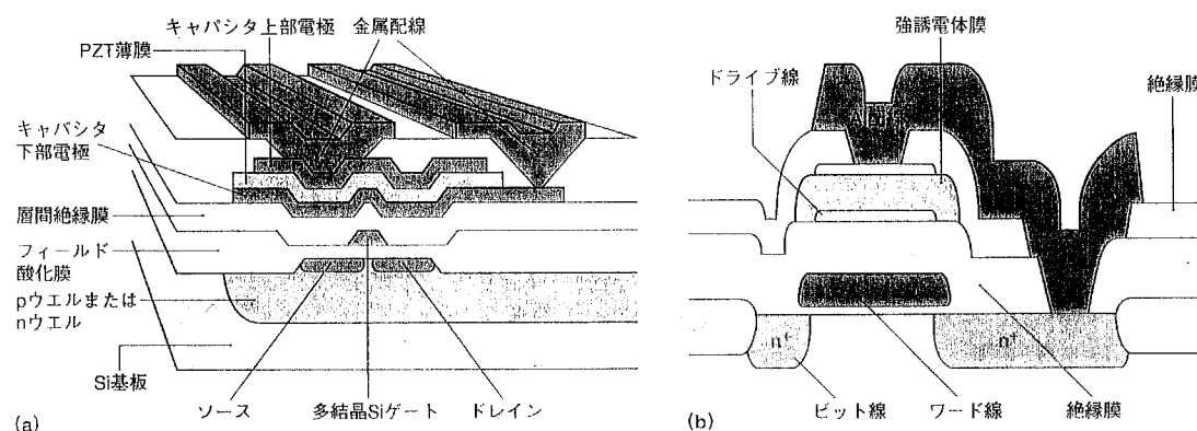
図 1 - 4 1988 年に発表された米 Ramtron 社(a)と米 Krysaliis 社(b)の強誘電体メモリ 20
