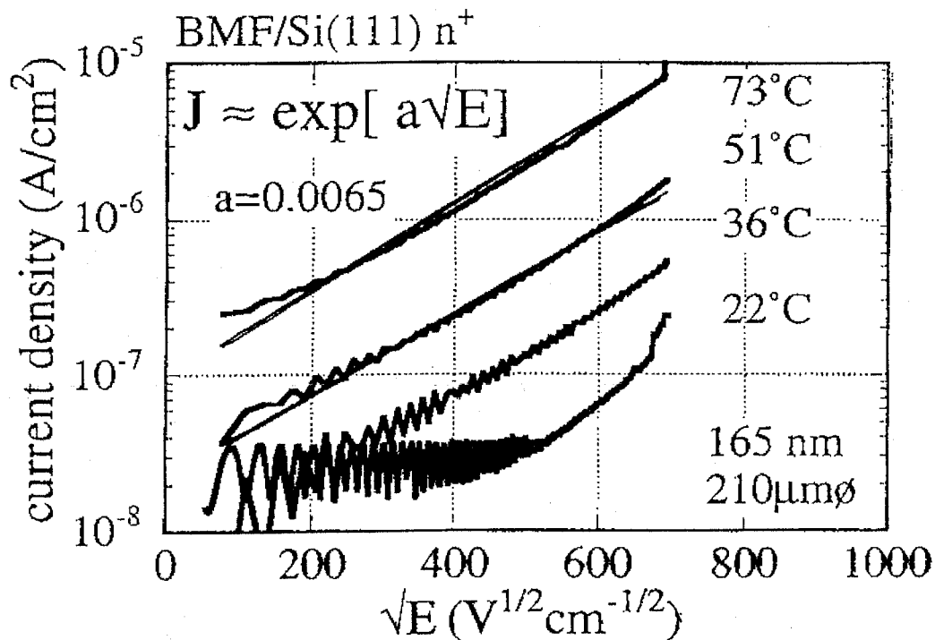
図5-18 漏れ電流特性のショットキープロット ( J-\sqrt{E} )
