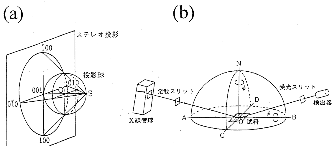
図 3-8 ステレオ投影の概念(a)と極点図形の測定原理(b)
