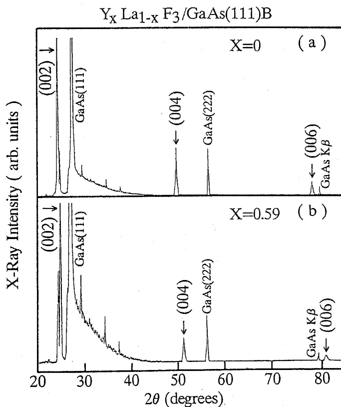
図 3-6 \text{Y}_x\text{La}_{1-x}\text{F}_3/\text{GaAs}(111)\text{B} 構造の X 線回折パターン (a) X=0 の場合、(b) X=0.59 の場合
