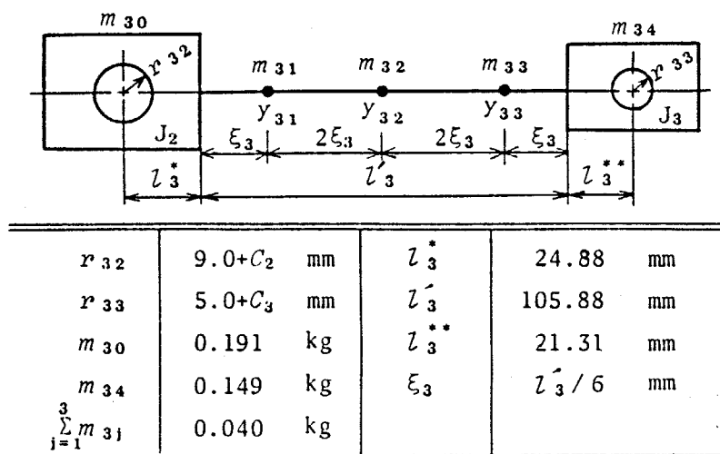
図 4.2.3 弾性節の諸元
