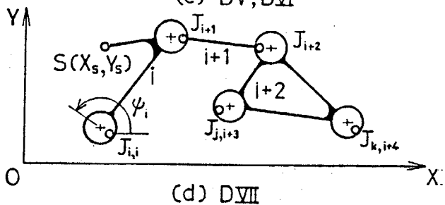
図 2-2-3 基本連節と変位変換関数
