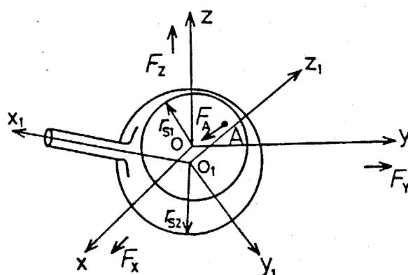
図 2-4-2 球対偶
