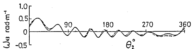
(b) 従動節
