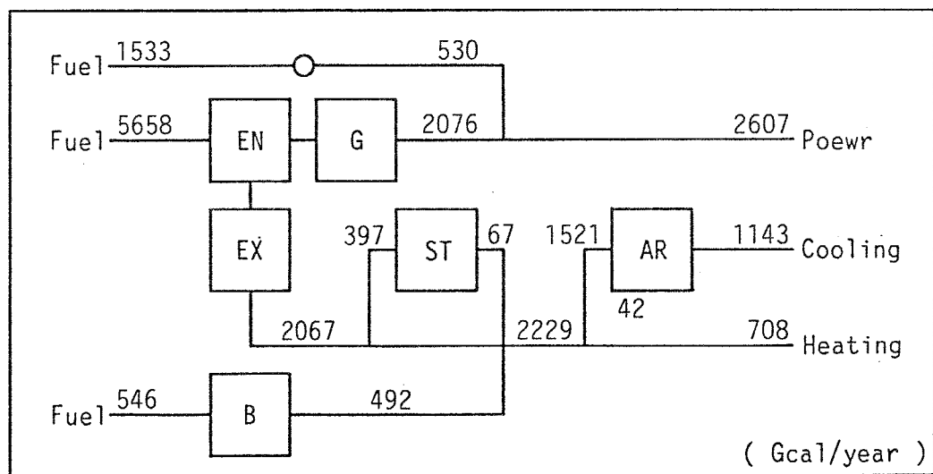
(2) ケースB2
