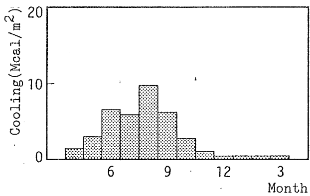
(3) 冷熱需要量
