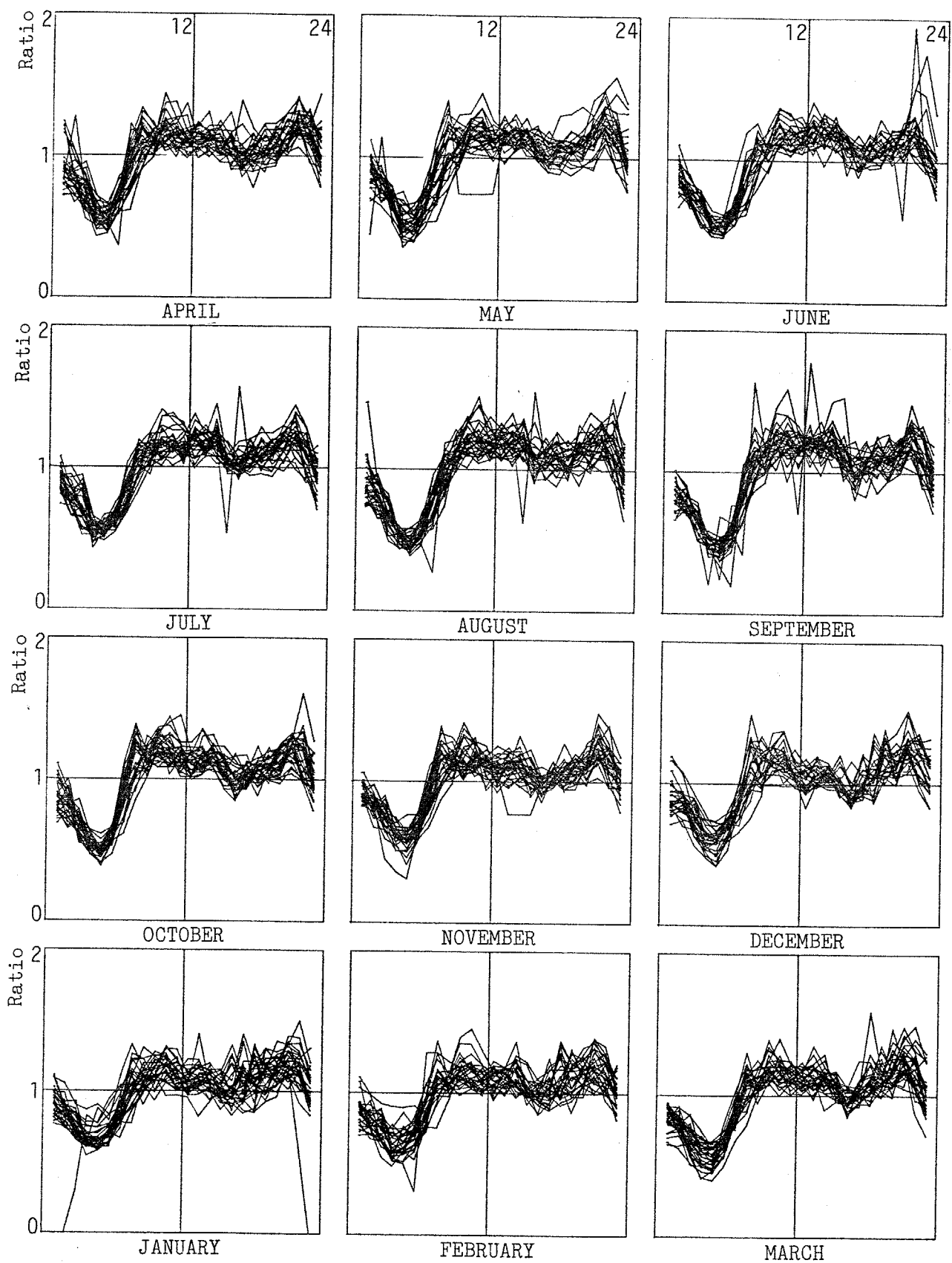
図-3-25 ホテルの温熱需要の時間変動
