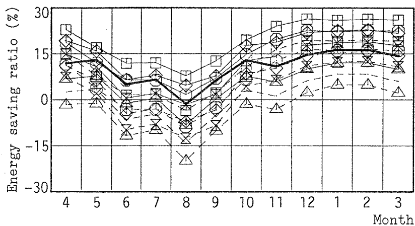
(2) ケースB2
