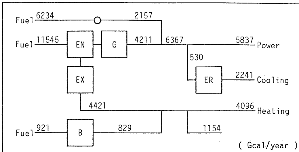
(1) ケースA5
