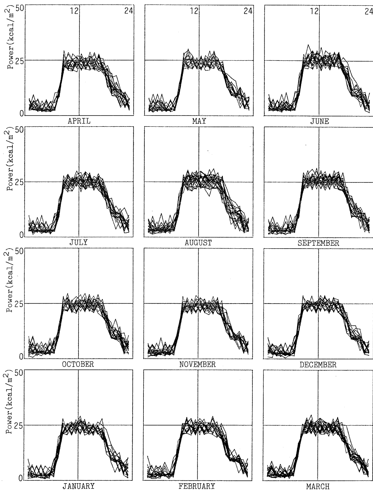
図-3-9 事務所における電力消費量の時間変動(平日)
