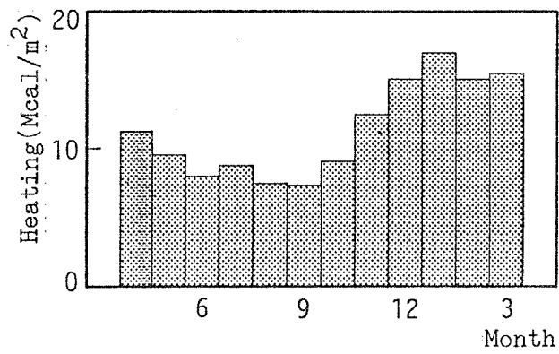
(2) 温熱需要量
