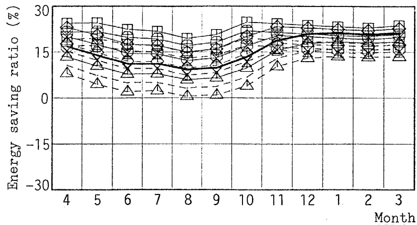
(1) ケースA5
