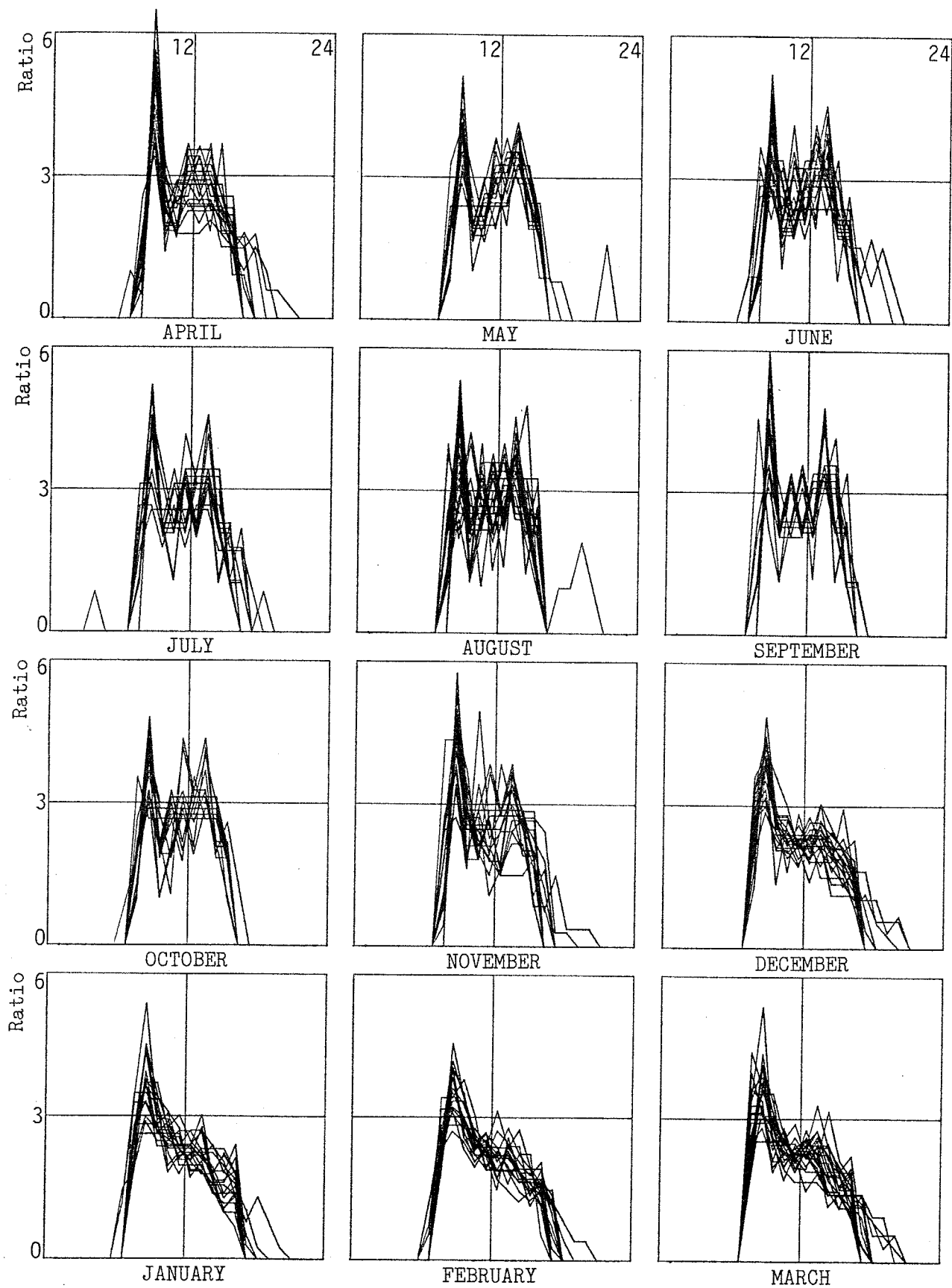
図-3-22 事務所の温熱需要の時間変動
