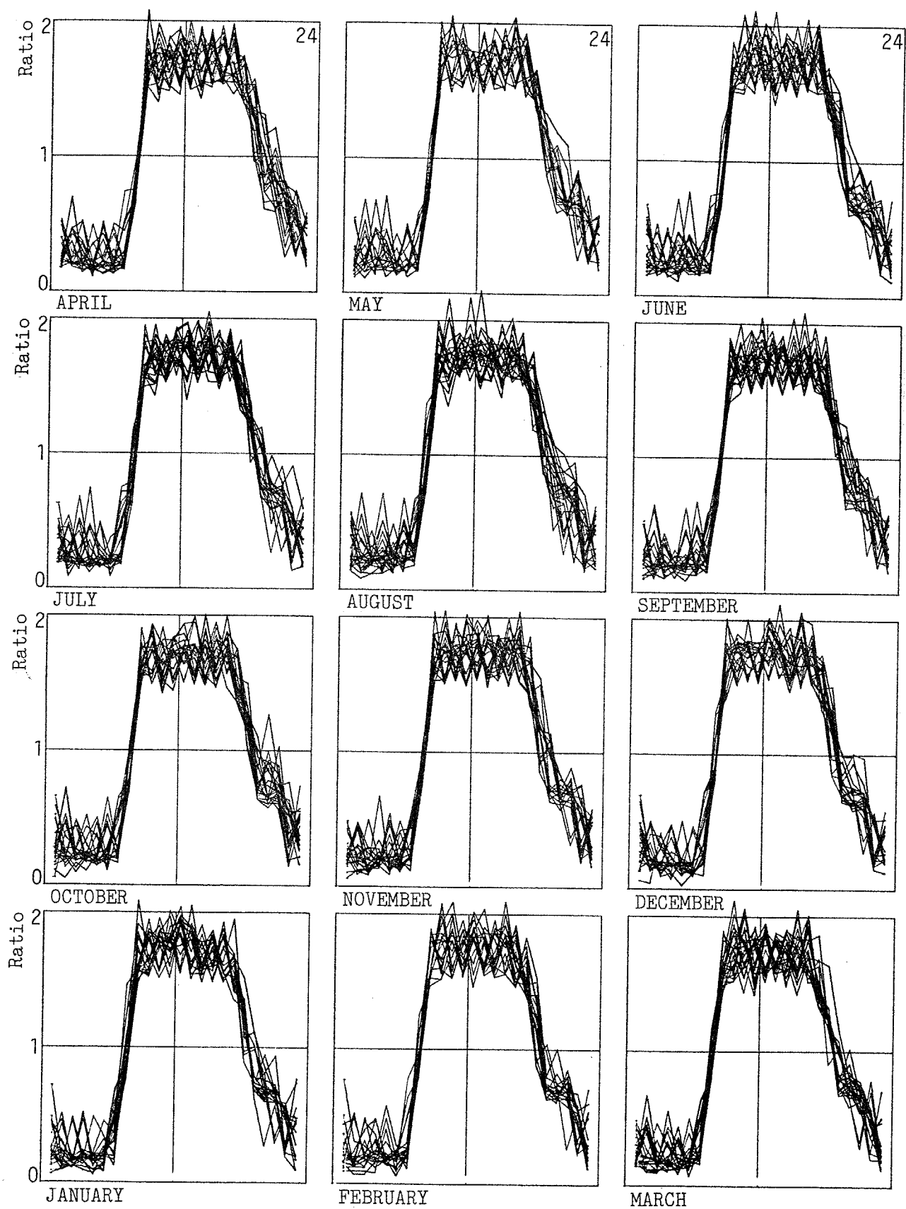
図-3-21 事務所の電力需要の時間変動
