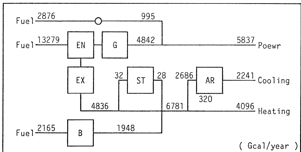
(2) ケースB2
