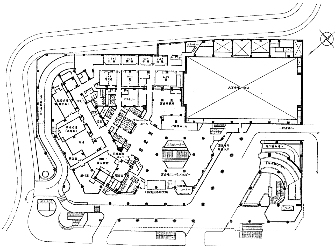
(1) 1階平面図
