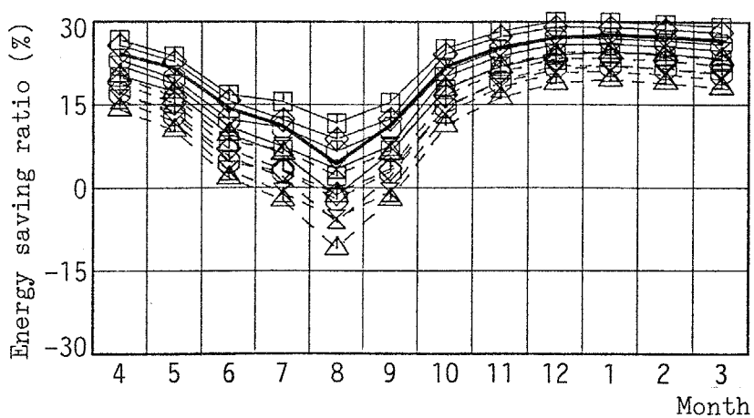
(3) ケースF3
