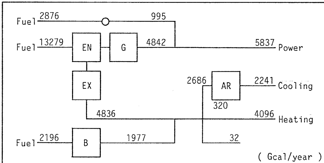
(2) ケースB2
