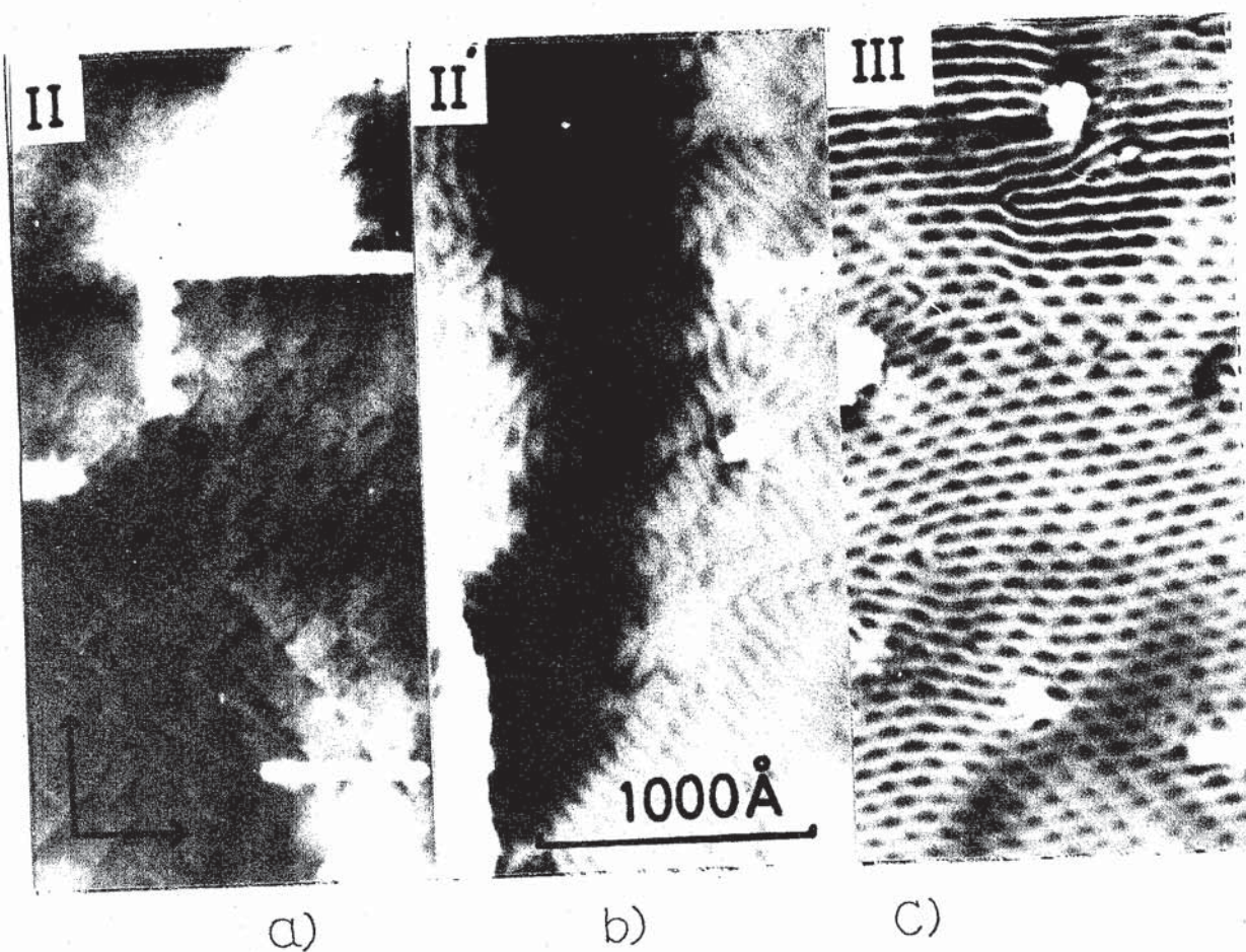
図3-2 PbSe/(001)PbTe ( \sim 200^{\circ}\text{C} ) の成長過程. a) 成長才2段階の始まり, b) 才II段階から才III段階, c) 才III段階, を示す。
