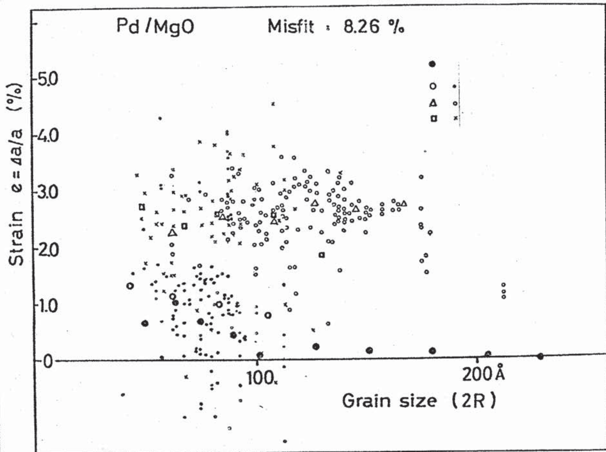
図5-18 Pd/(001)MgO ( \sim 350^\circ\text{C} ) の格子歪.
