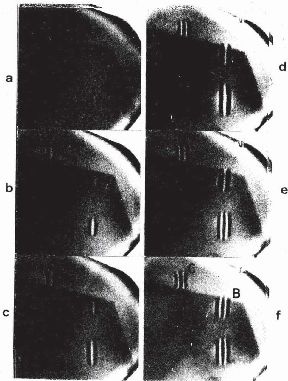
図4-10 80 °C 下地上に固相成長する粒子の成長過程 (a) から (d) にかけて、粒子Aのモアレ縞間隔が増大し、(d) から (e) の間に、モアレ縞の数が増加して、モアレ縞間隔は減少している。粒子BおよびCも同様なモアレ縞巾の変化を示している。(a) の粒子B、C で、すでにモアレ縞が1本見えること、および、粒子輪郭がモアレ縞方向に伸びた扁平楕円形であることに注目。
