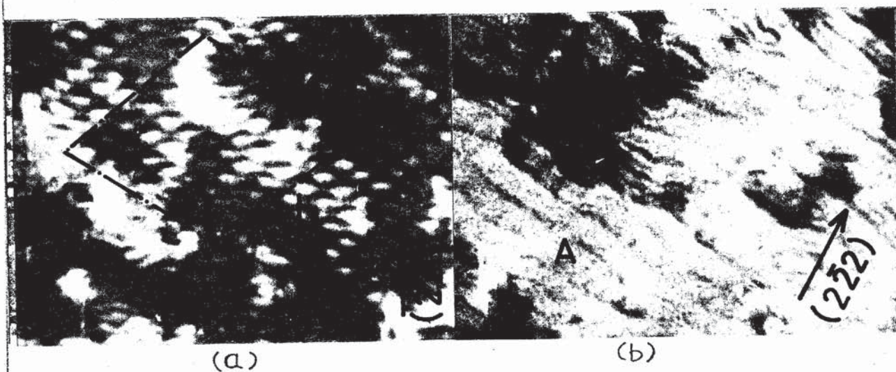
図3-6 (110)膜の刃型段階, 2組の転位 ( l_1 と l_2 ) が網目模様を形成している。それらの一方 ( l_1 ) のコントラストは (2\bar{2}2) 反射を励起した (b) 図で消失している。
