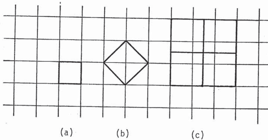
図5-27 イソタクシャル方位と、下地-成長結晶格子の適合。 細い実線が下地結晶格子，太い実線が成長結晶格子 を表わす。(a), a/b = 1 , (b) a/b = \sqrt{2} , (c) a/b = 3/2 の場合.
