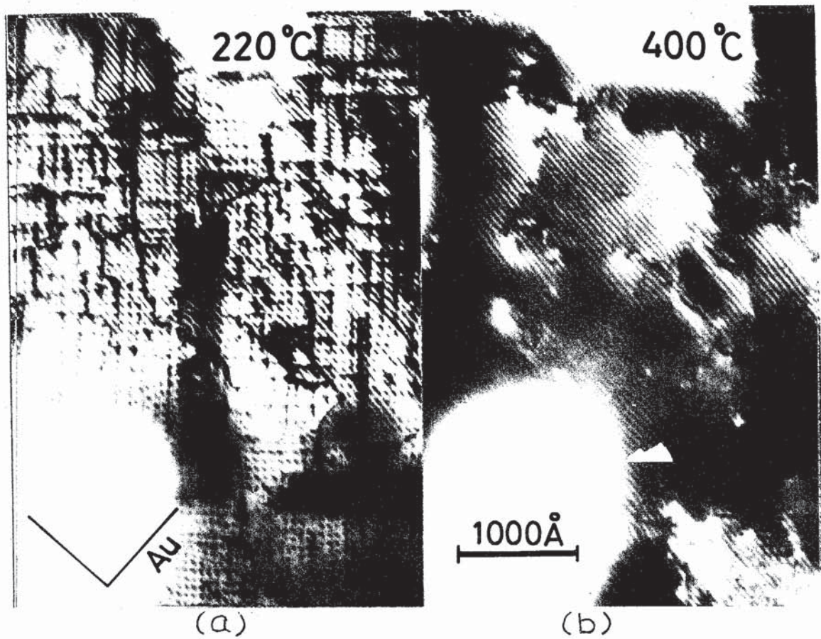
図3-21 Pd/(001)Au(300°C)の加熱による転位の消失
