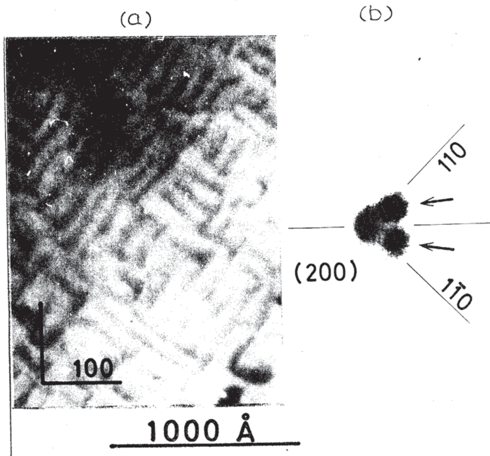
図3-13 PbSe/(001) PbTe (室温)
