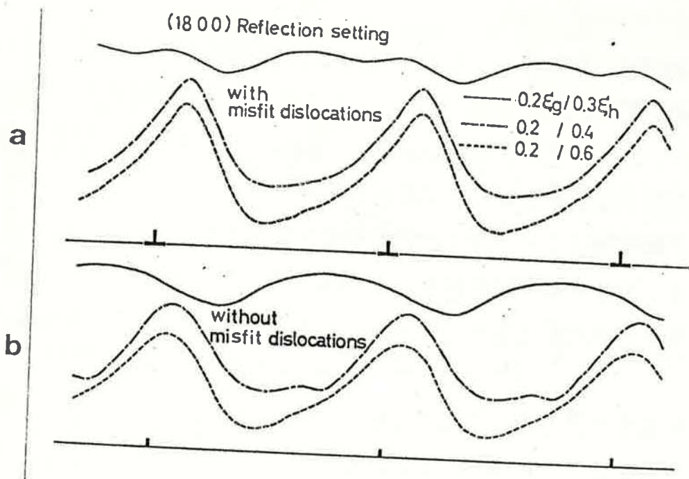
図4-13 (200) 暗視野像の多波動力学回折コントラスト。 (a) 界面にミスフィット転位を含む場合, (b) 含まない場合。 (付録Iを参照) \xi_g, \xi_h それぞれ, 成長, 下地結晶の (200) 反射の消衰距離である。
