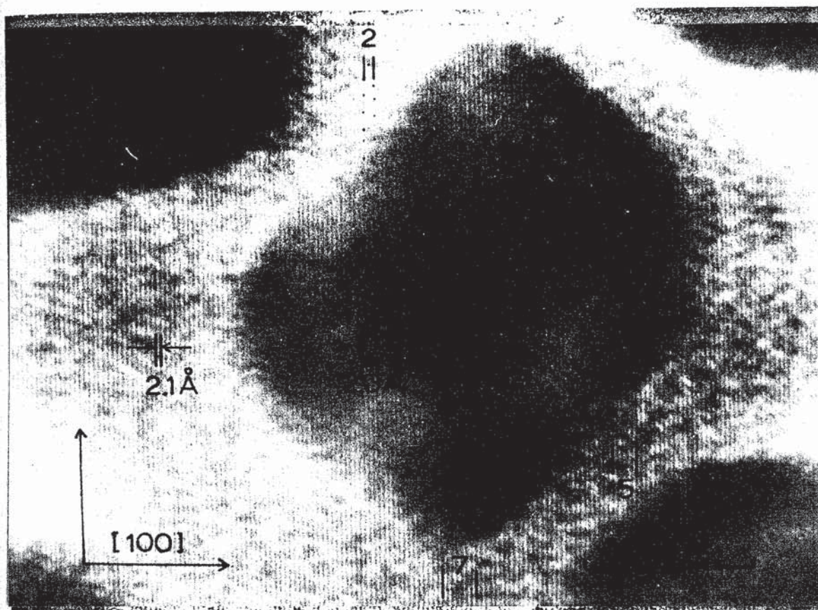
図5-17 Au/(001)MgO (350°C) の格子像写真.
