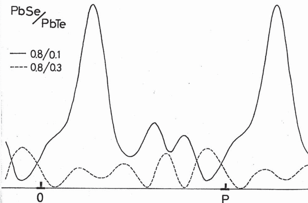
図AI-5 g \cdot b_v = 2 の反射, (220) 反射, による PbSe/PbTe の多波動力学的回折コントラスト. 転位間隔内に 4 つの強度ピークが現われていることに注意せよ. 反射条件は (660) 反射がブラッグ条件を満たすところである. 膜厚はそれぞれの消衰距離を単位として示してある.
