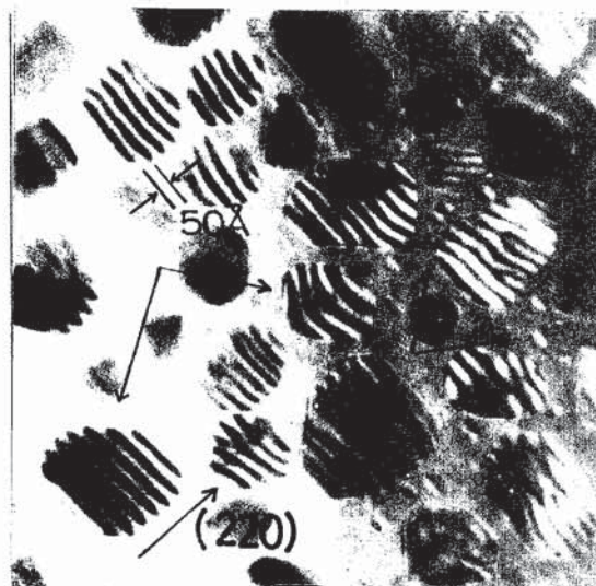
図5-1 300 °C 前後の (001) \text{MgO} 上に成長した Ag 粒子 約 50 Å 間隔のモアレ縞は Ag と \text{MgO} の (220) 反射による。
