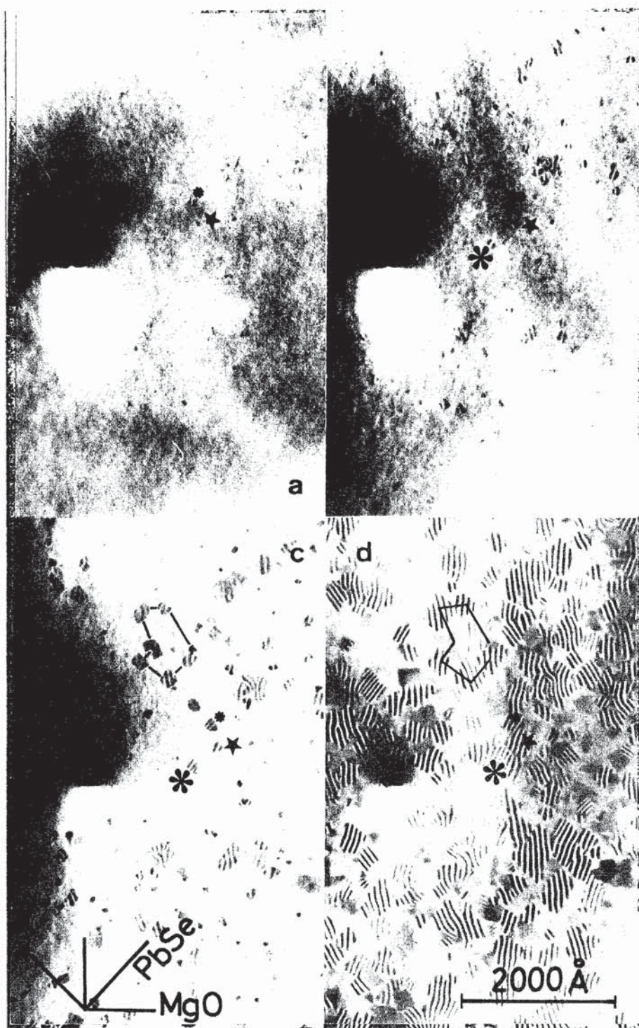
図5-8 PbSe/(001)MgO (150°C)の成長過程の電顕写真記録 PbSeは、ほぼ(001)-R45°方位で成長している。約50 Åの モアレ縞はPbSe(220)とMgO(200)反射による。モアレ 縞を出していない(001)-P方位の粒子も、幾分形成されて いる。初期段階である方向をもって核形成した粒子に、その 成長、合体過程を通して方位変化が、殆んど認められない。
