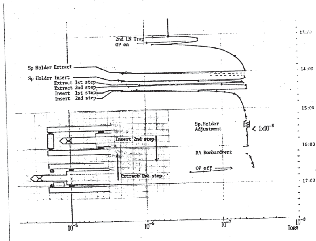
図2-6 JEM 100B 超高真空電顕の排気特性
