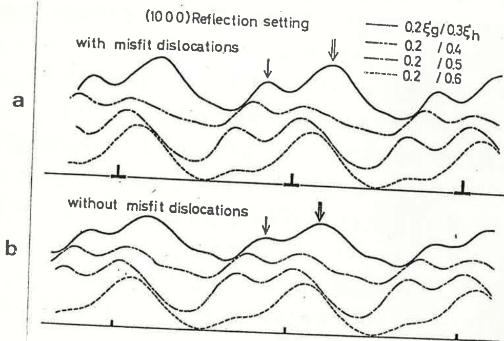
図4-14 (400) 暗視野像の多波動力学的回折コントラスト。 (a) 界面にミスフィット転位を含む場合, (b) 含まない場合。 (a) と (b) でコントラストに定性的差異は認められない。
