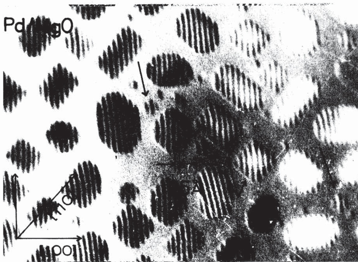
図5-2 300 °C 前後の (001) \text{MgO} 上に成長した Pd 粒子 約 25 Å のモアレ縞は Pd, \text{MgO} の (220) 反射による。 図5-1 と、モアレ縞、粒子輪郭の相異に注意。
