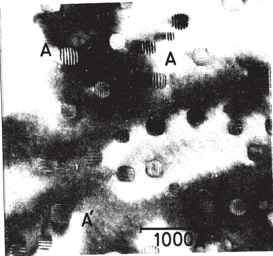
図4-7 180 °Cで液相成長した後に、冷却によって固化した粒子。視野中で(200)反射と(020)反射が同時に励起されている。幅の広い、ほぼ37 Å程のモアレ縞を出している粒子Aは(010) Sn //(001) SnTe , [100] Sn //[100], or [010] SnTe の方位をもち、一方、幅の狭い、ほぼ26 Åのモアレ縞を出している粒子A'は(010) Sn //(001) SnTe [101] Sn //[100] or [010] SnTe の方位をもつ。粒子の輪郭が“角のとれた四角形”であることに注目せよ。(図4-5, 4-6 参照)
