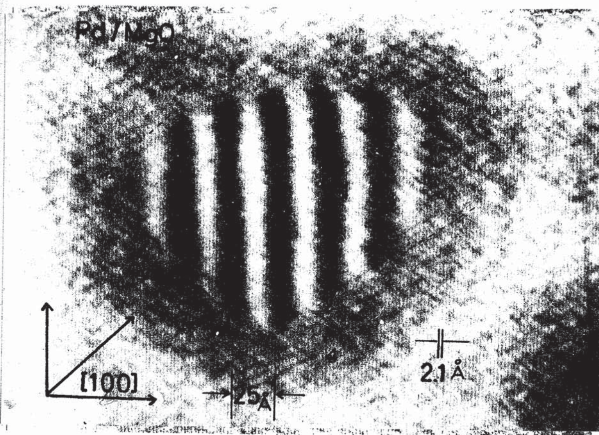
図5-19 Pd/(001)MgO ( \sim 350^\circ\text{C} ) の格子像写真 2.1 Åの格子縞は MgO(200)格子像である。 点線で示した粒子輪郭は、その場蒸着直後の粒子 輪郭とあまり相異していない。これらの粒子の 格子歪は、図5-18の小さい黒丸印のプロット を与えた。
