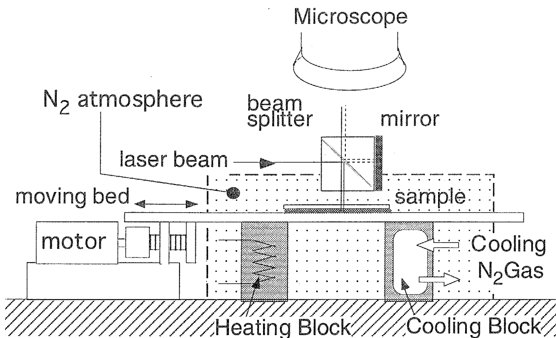
図 5-3-1 方向性凝固実験装置
