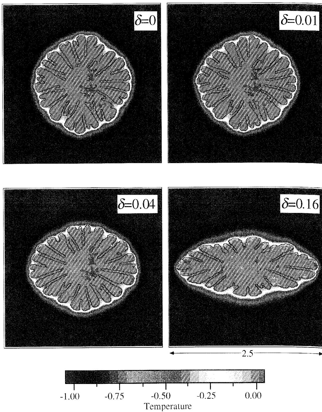
図 5-4-9 異方性の度合いによる凝固形状の変化
