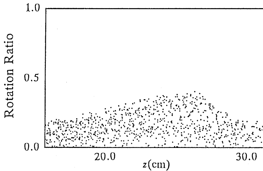
図 4 - 1 9 B_{\text{applied}} \Delta z = 0.01 \text{ Tesla} \cdot \text{m} の磁場を加えた場合の回転速度比分布
