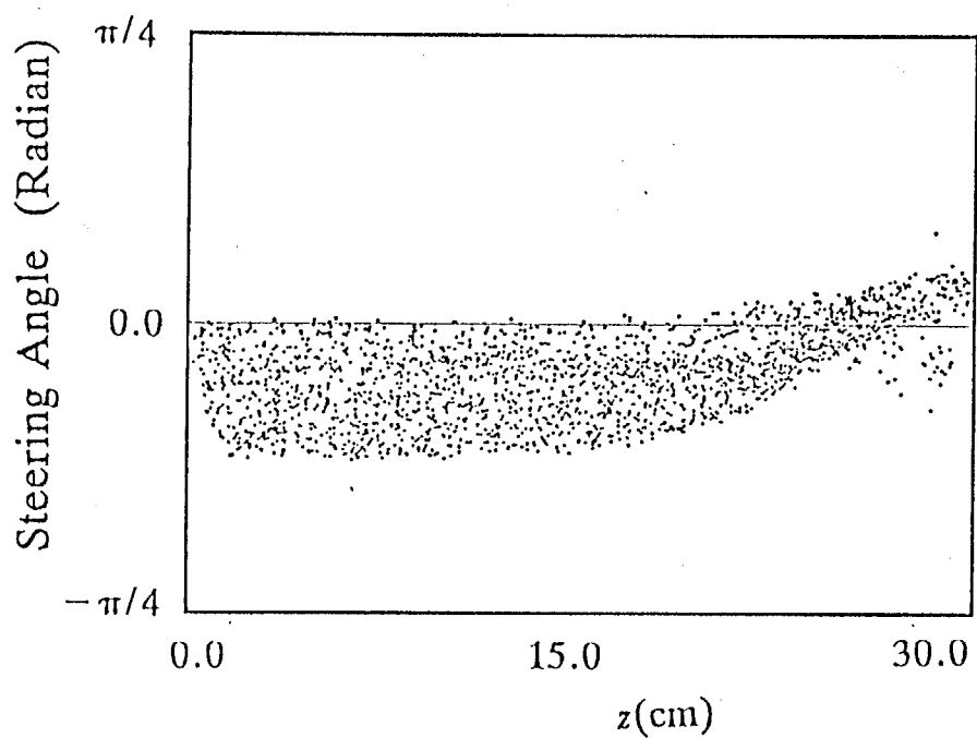
図 4 - 1 8 B_{\text{applied}} \Delta z = 0.01 \text{ Tesla} \cdot \text{m} の磁場を加えた場合の Steering Angle の分布
