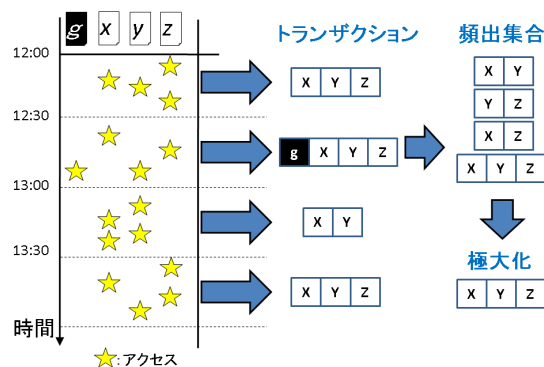
図 1: ファイル集合の発見
