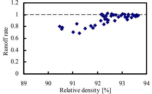
図-11 流出率の相対湿度依存性 (7時間移動平均値)
