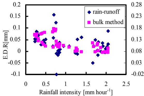
図-12 降雨中蒸発量の降雨強度依存性 (7時間移動平均値)
