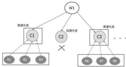
図 3：引用数優先探索手法
