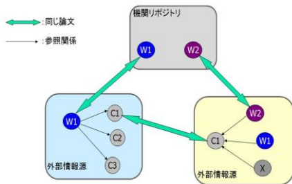
図1: アプローチ
