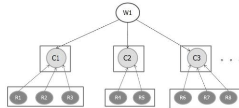
図2: 全探索手法
