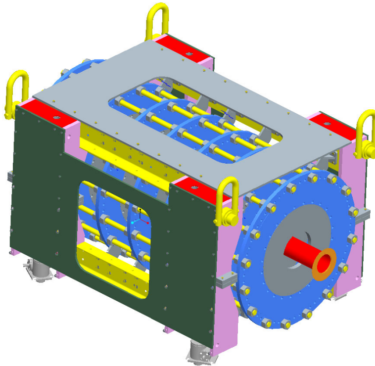
図 4-1-10 : 電磁石の構造図
