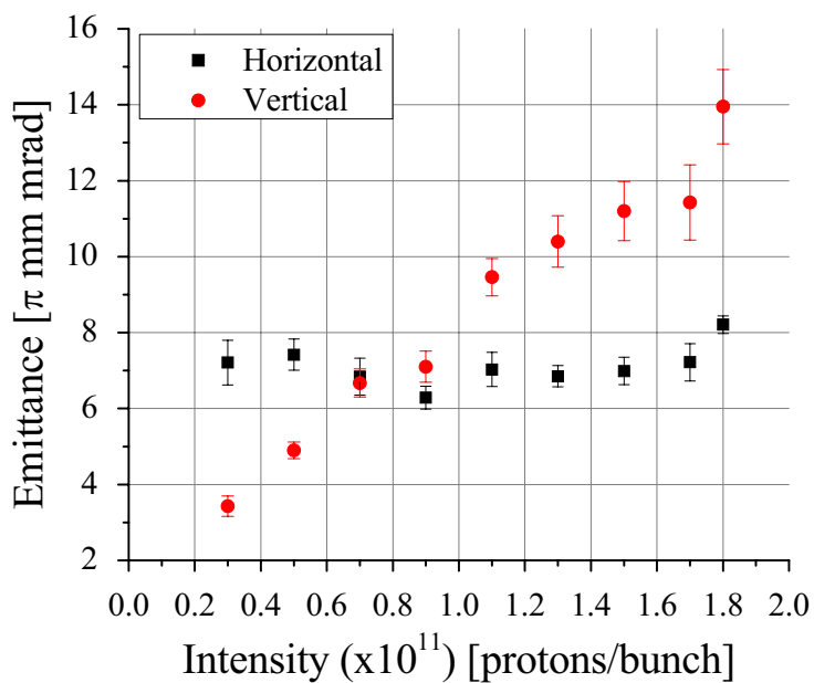
図 6-3-22 : Vert. Scraper を用いたときの T=100ms におけるエミッタンスとビーム強度
