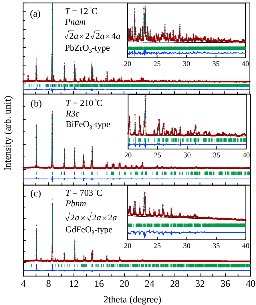
図 3.7 (a) 12^\circ\text{C} 、(b) 210^\circ\text{C} 、(c) 703^\circ\text{C} における \text{Bi}_{0.9}\text{Sm}_{0.1}\text{FeO}_3 の放射光粉末 X 線回折パターン (+) および計算回折パターン (実線)、実測と計算の差分 (最下段)、計算から求められたピーク位置 (中段)。波長 \lambda = 0.41766 \text{ \AA} 。
