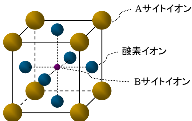
図 1.8 ABO_3 ペロブスカイト構造
