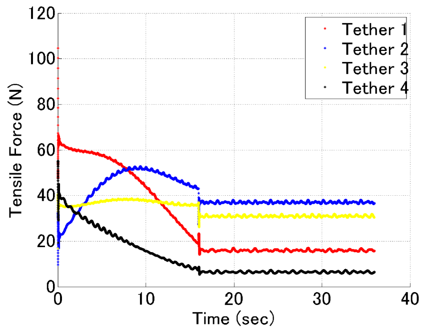
Fig. 3.12 数値解析結果 (テザー張力)
