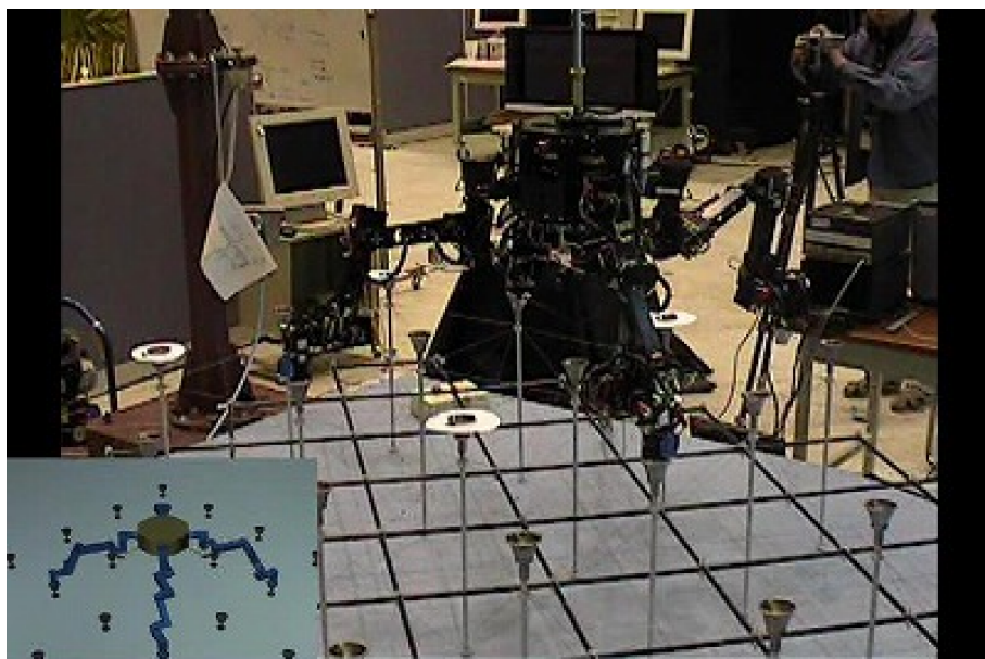
Fig. 1.15 再構成型歩行宇宙ロボット RBR
