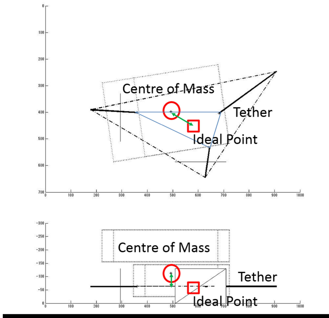
Fig. 5.15 REX-J 重心位置
