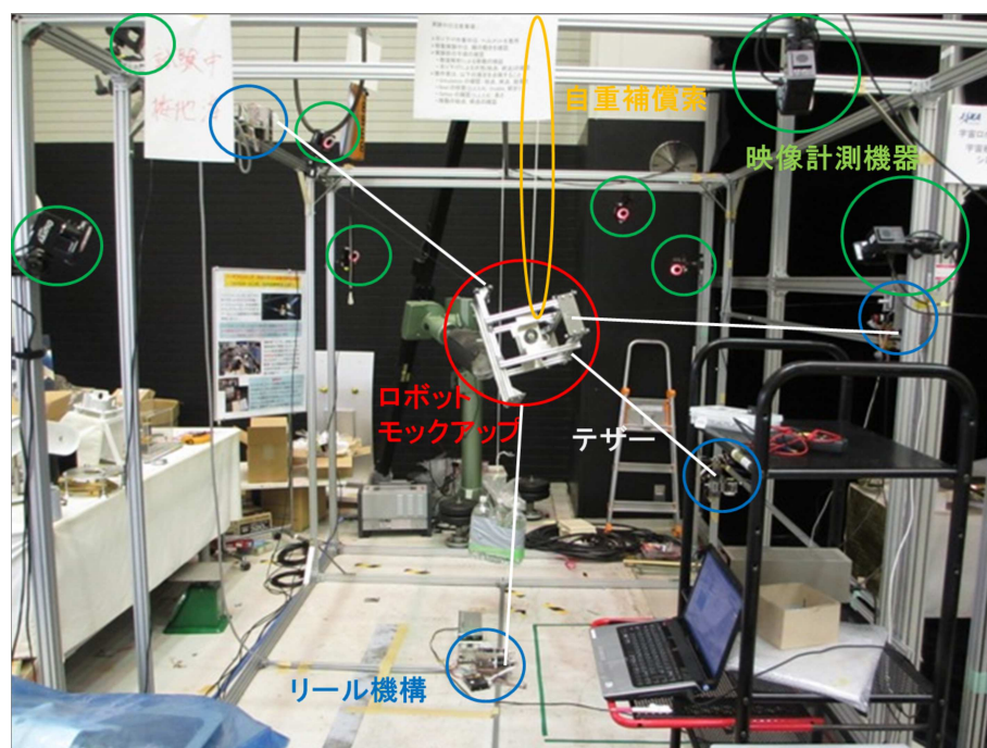
Fig. B.1 実験装置全景
