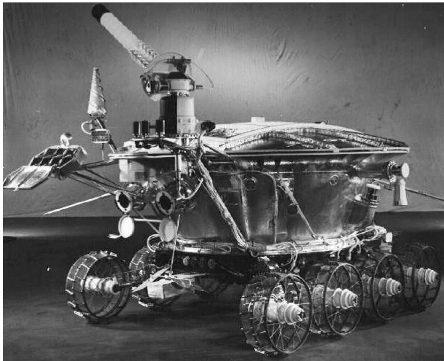
Fig.1.3 月面車 ルノホート
