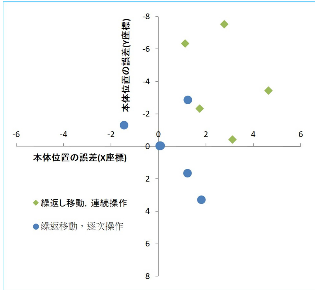
Fig. 5.31 繰返し移動の検証 誤差の比較
