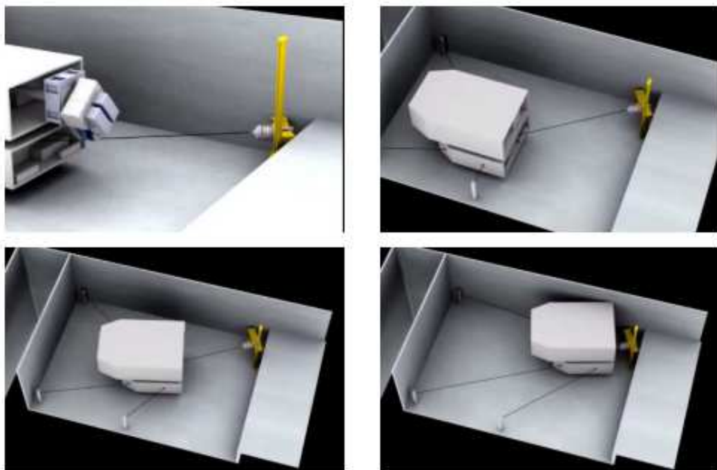
Fig. 5.4 テザーフックのハンドレールへの取り付け
