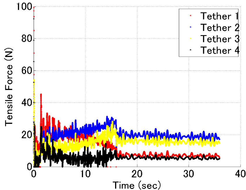
Fig. 3.26 数値解析結果 (テザー張力)
