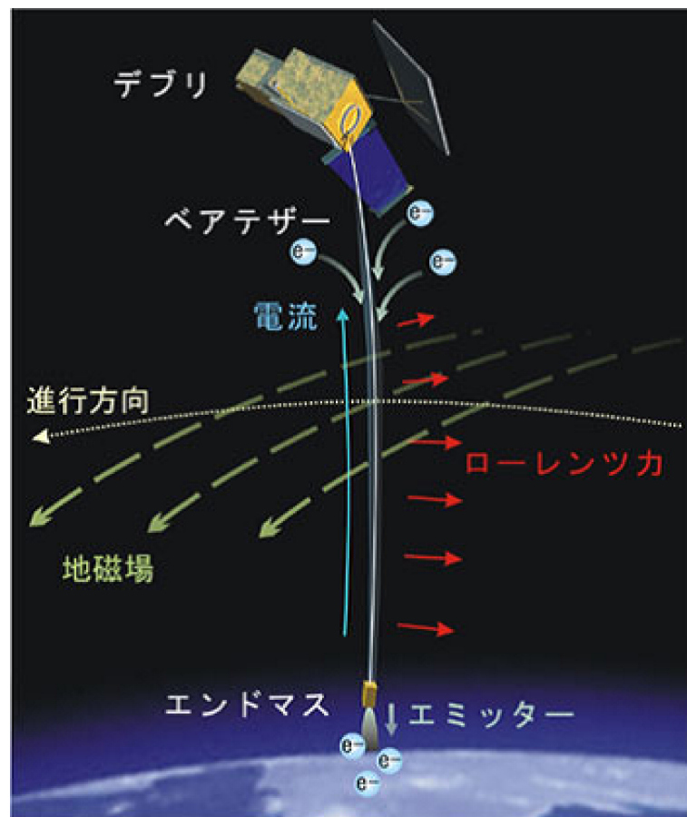
Fig. 2.2 導電性テザー [22]
