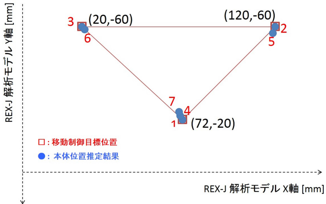
Fig. 5.30 繰返し移動の検証 移動履歴と位置精度 (逐次操作)
