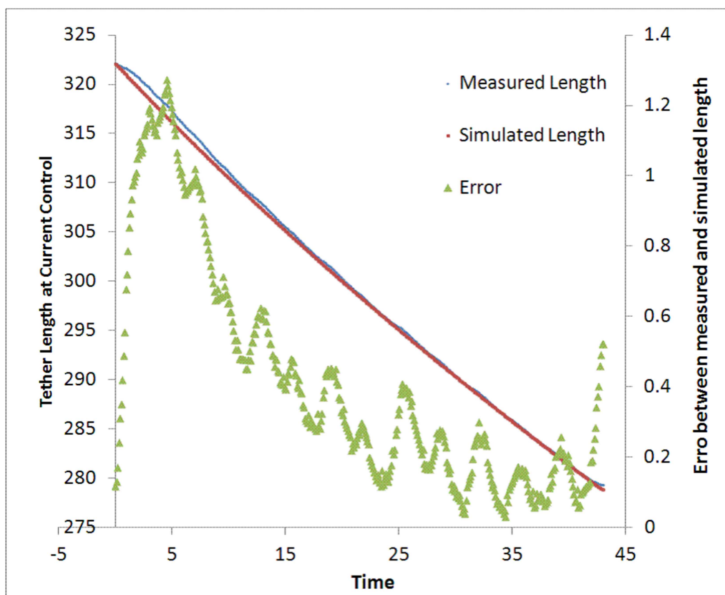
Fig. 5.25 定負荷移動制御の検証 電流制御の伸展長履歴と解析モデルとの比較
