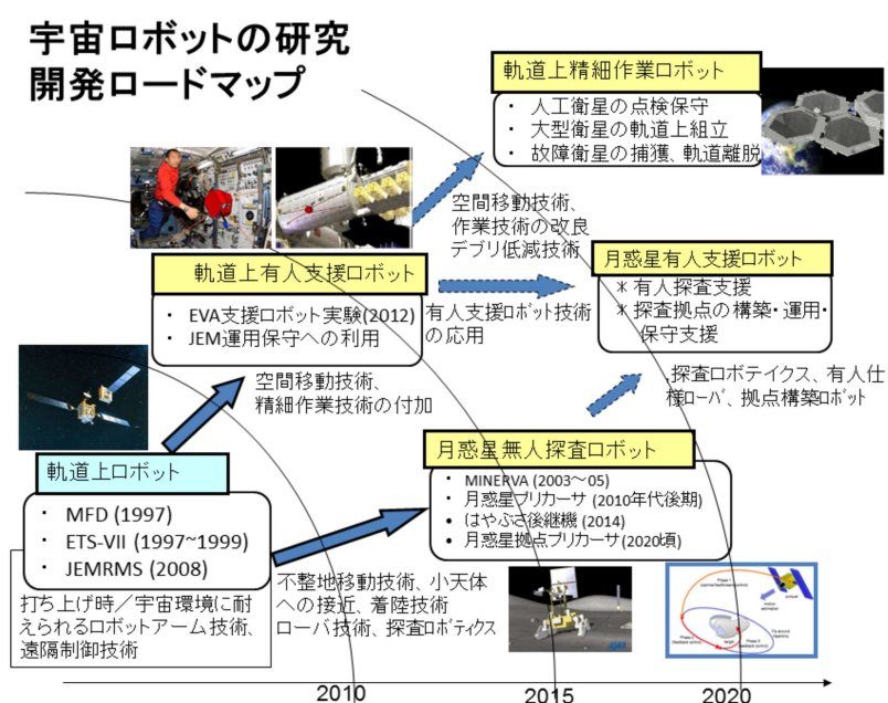
Fig. C.1 宇宙ロボットの研究ロードマップ (C) JAXA
