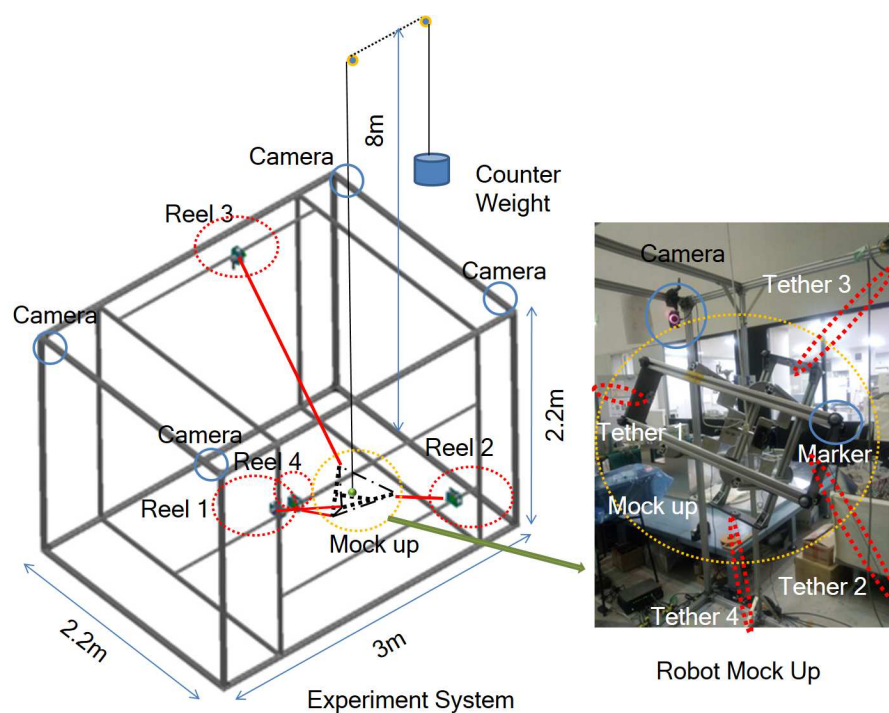
Fig. 4.3 実験装置 外観図
