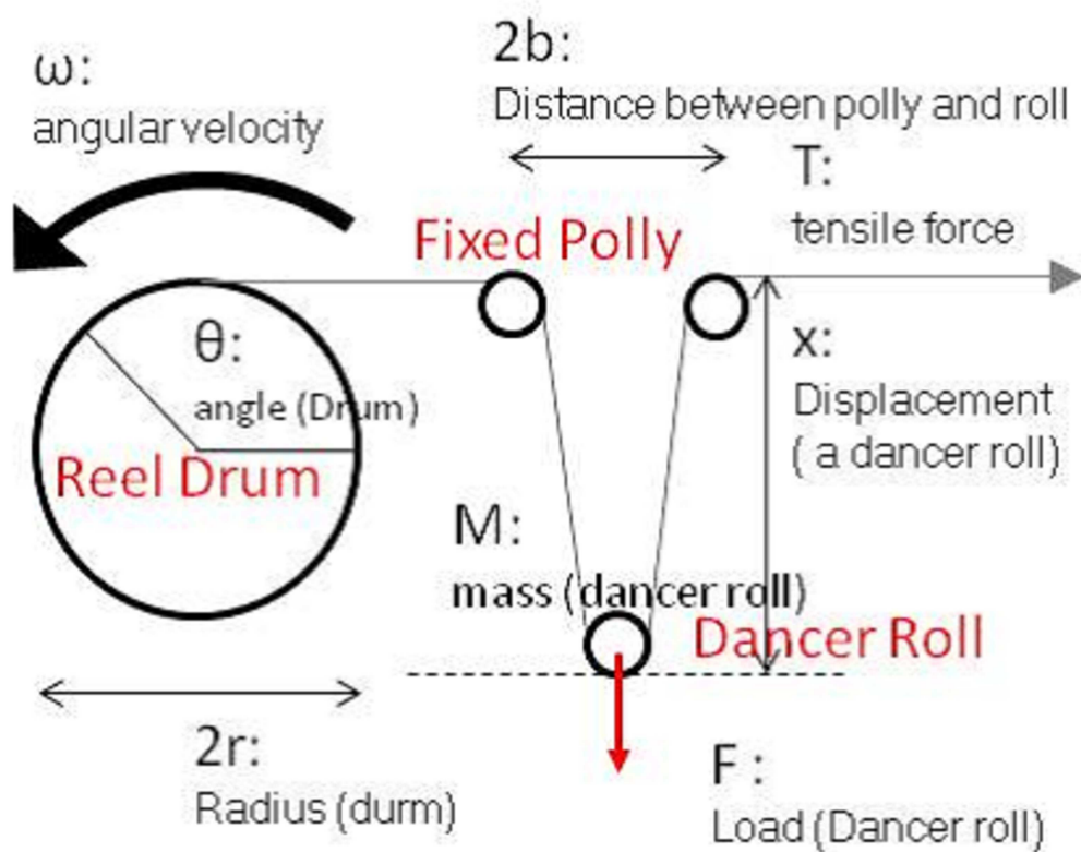
Fig. B.3 ダンサーロール方式 概略図
