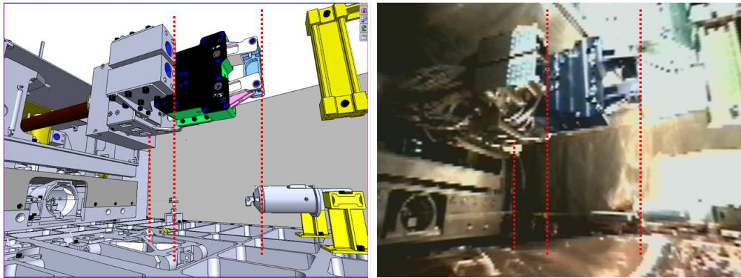
Fig. 5.23 定負荷テザー制御の検証 視野解析
