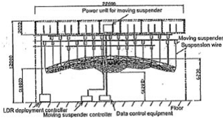
Fig. 4.1 ETS-VIII 搭載用大型展開アンテナの地上展開試験 [65]
