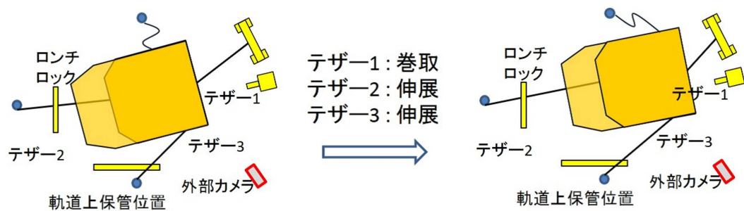
Fig. 5.13 テザー支持→本体移動→テザー支持
