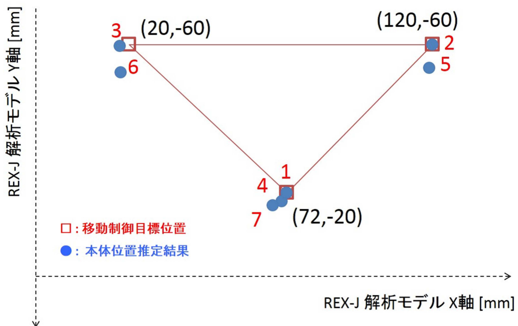
Fig. 5.28 繰返し移動の検証 移動軌跡
