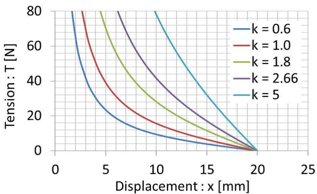
Fig. B.6 バネ変位-張力のモデル
