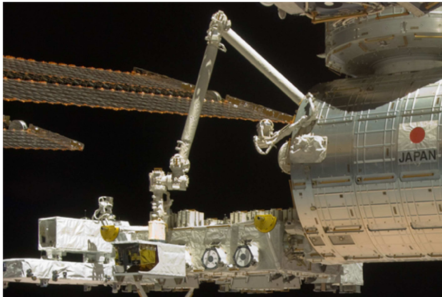
Fig. 1.7 「きぼう」ロボットアーム
