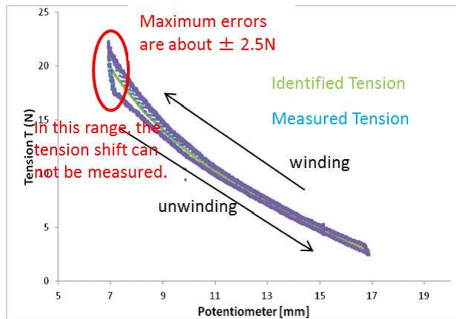
Fig. B.9 張力計測結果
