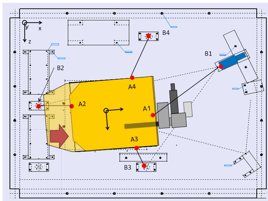
Fig. 5.10 REX-J 移動実験 (模式図)
