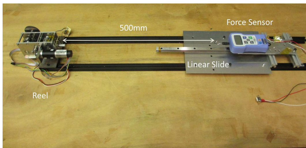
Fig. B.8 リール機構 実験装置
