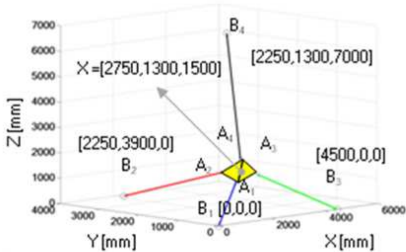
Fig. 3.4 シミュレーションモデル
