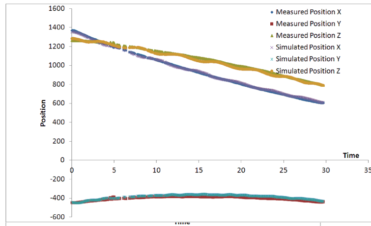
Fig. 4.6 地上実験 移動軌跡 (計測値, 解析解)
