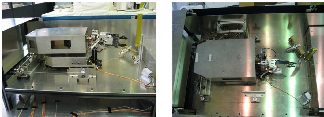
Fig. 5.15 REX-J 重心位置
