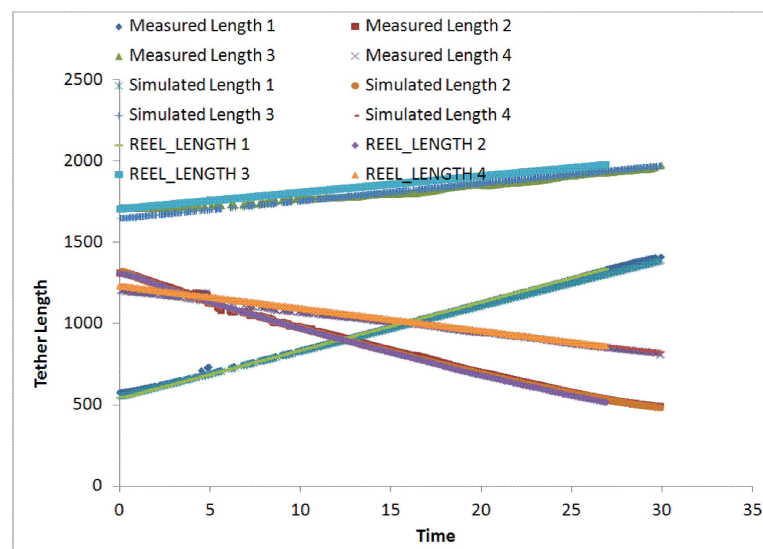
Fig. 4.7 地上実験 テザー長 (計測値, 解析解, リール算定値)
