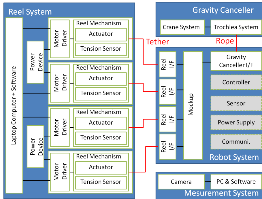
Fig. 4.2 地上模擬装置の概念図
