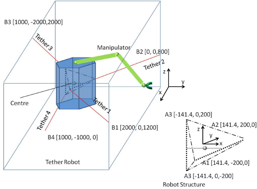
Fig. 3.9 シミュレーションモデル
