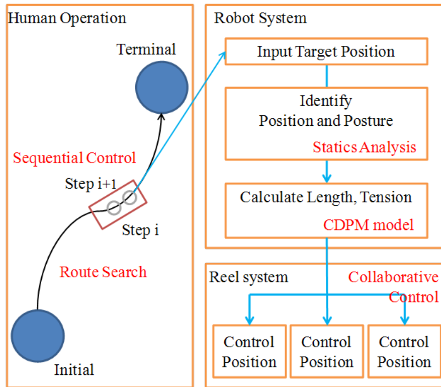
Fig. 3.7 作業空間による逐次テザー制御手法
