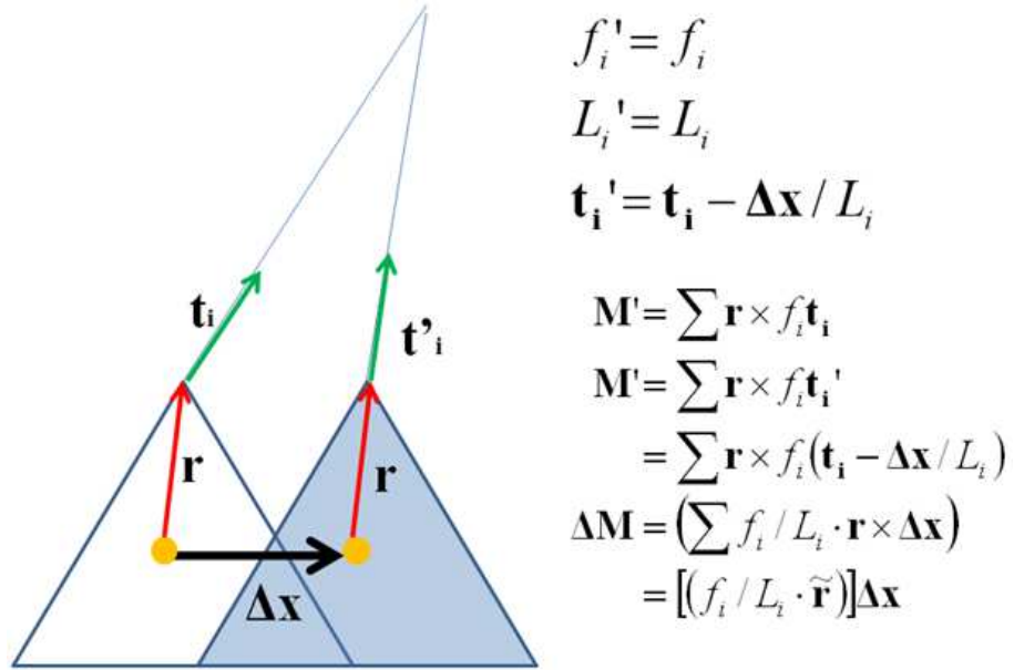
Fig. 3.3 姿勢指定の反復方法
