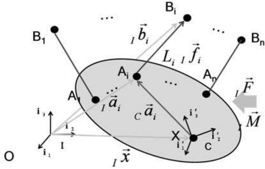
Fig. 2.13 CDPM 数理モデル
