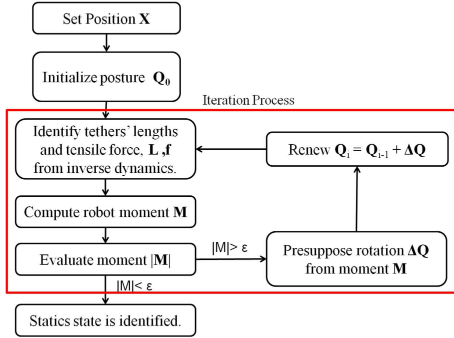
Fig. 3.2 静安定解析の反復法 (位置)
