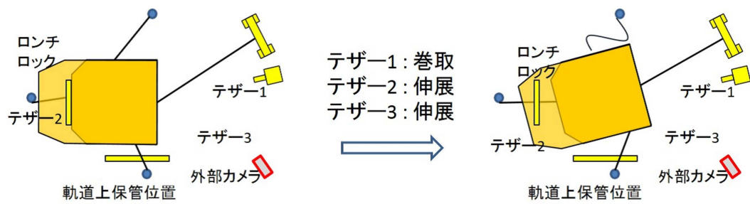
Fig. 5.11 壁面支持→本体移動→テザー支持
