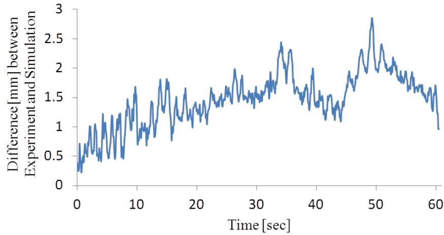
Fig. 5.20 数値解析との比較 (重心位置との偏差)
