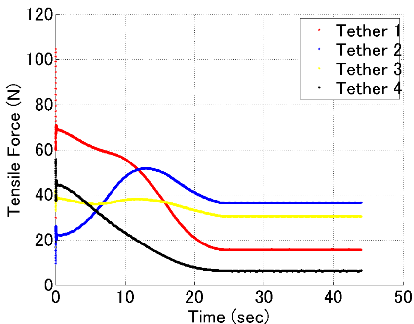
Fig. 3.15 数値解析結果 (テザー張力)
