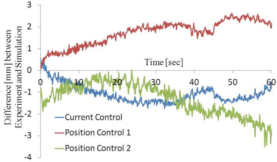
Fig. 5.21 数値解析との比較 (テザー長との偏差)
