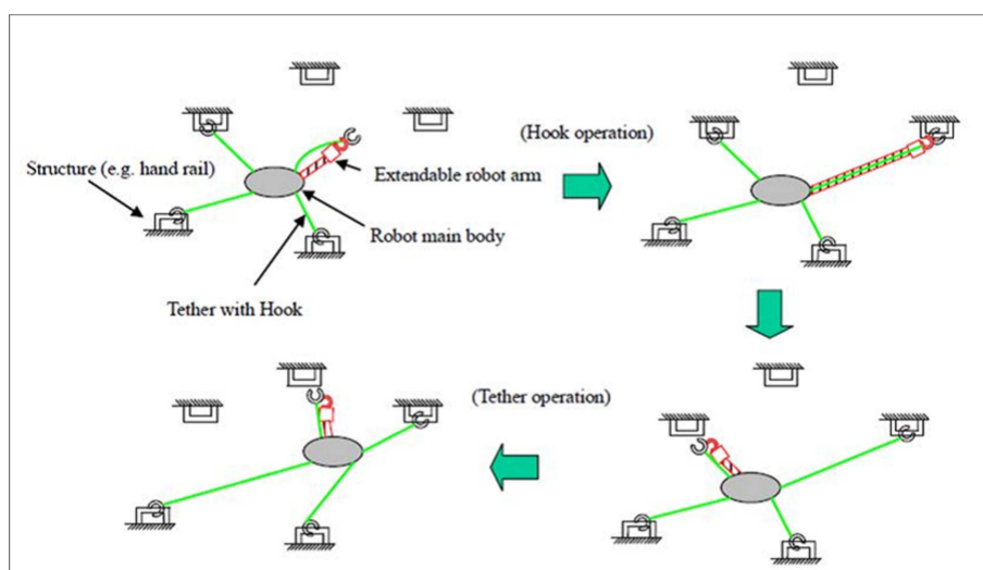
Fig. 2.1 Astrobot Support Robot の移動手法
