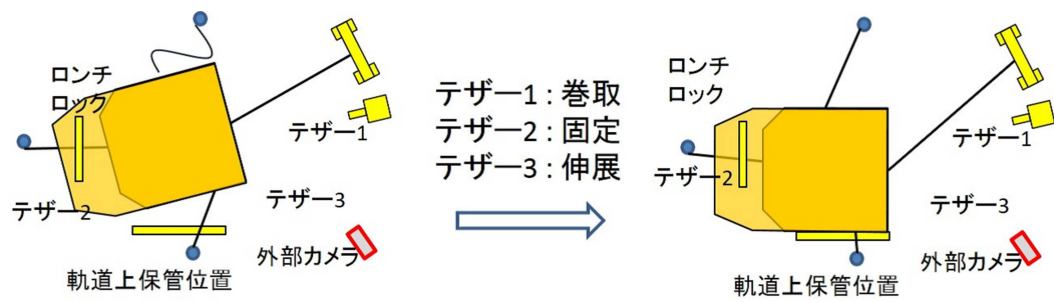
Fig. 5.12 テザー支持→本体移動→壁面支持
